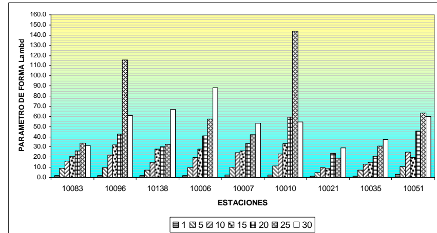
Figura D-6. Comportamiento de los parámetros de escala y forma por el método de Momentos, estaciones de la sub-región sub-húmeda de la RH-36.
