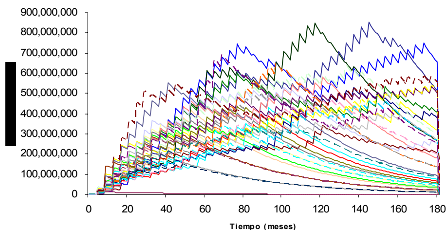
Figura V.9. Perfiles de producción de gas del proyecto.
