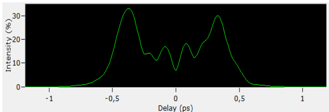
Figura 3.29. Gráfica correspondiente al peor valor del coeficiente de PMD (1527-1620 [nm]) del enlace del sitio C-sitio D. Fibra 2. PMD: 0.395 [ps], Coeficiente de PMD: 0.0364 [ps/km 0.5 ], PMD de segundo orden: 0.0694 [ps/nm] (0.0901 [ps 2 ]), Segundo coeficiente de PMD: 0.0006 [ps/nm*km] (0.0008 [ps 2 km]).
