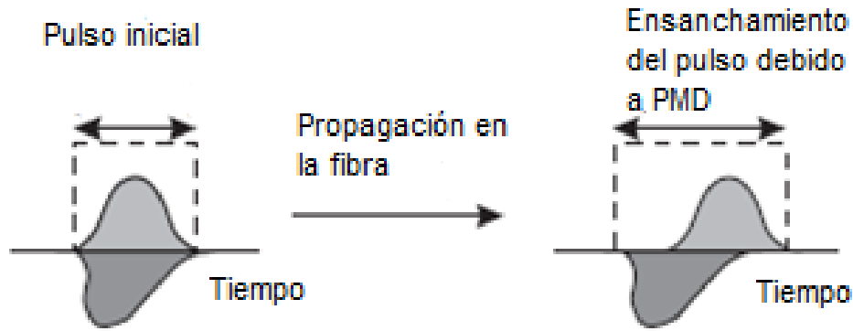
Figura 1.4. Ensanchamiento de un pulso debido a PMD [11].
