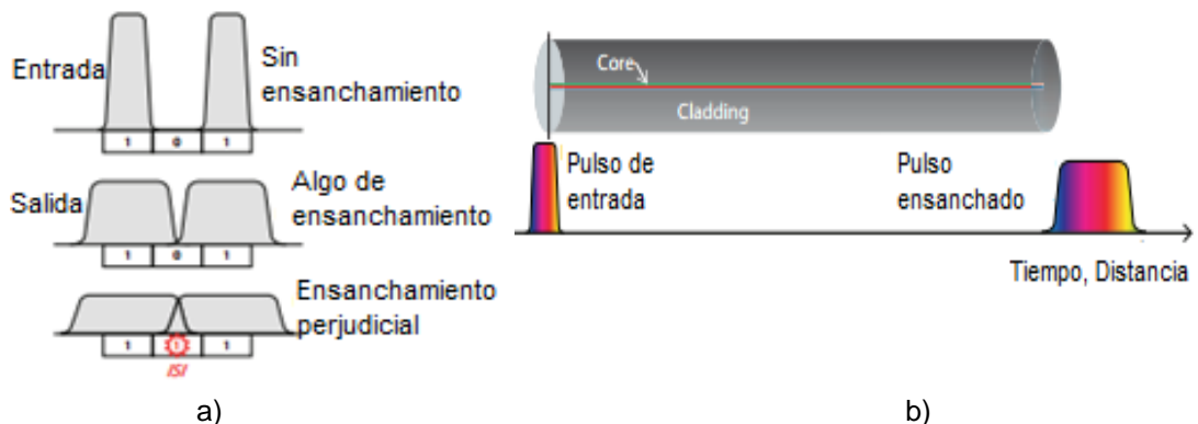
Figura 1.3. a) Interferencia intersimbólica debida a ensanchamiento. b) Diferentes longitudes de onda viajando a diferentes velocidades. [10].
