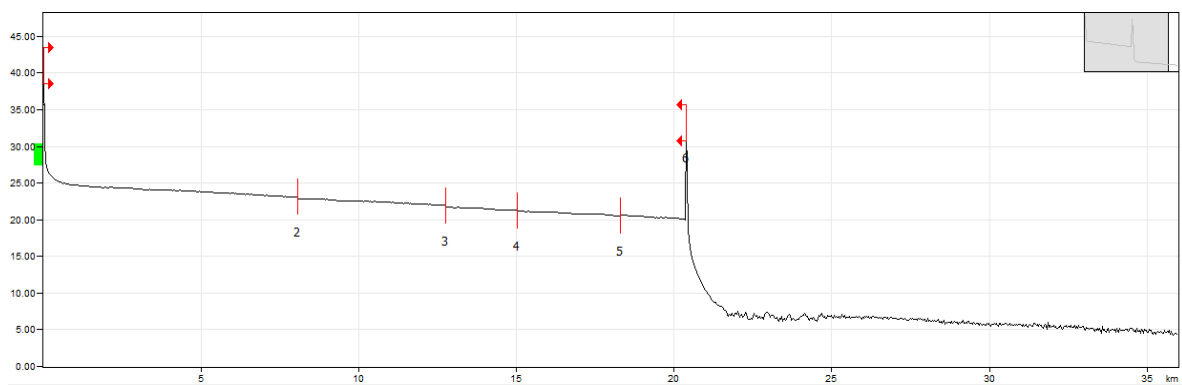
Figura 3.16. Trazo del enlace del sitio G-sitio H. Fibra 1.
