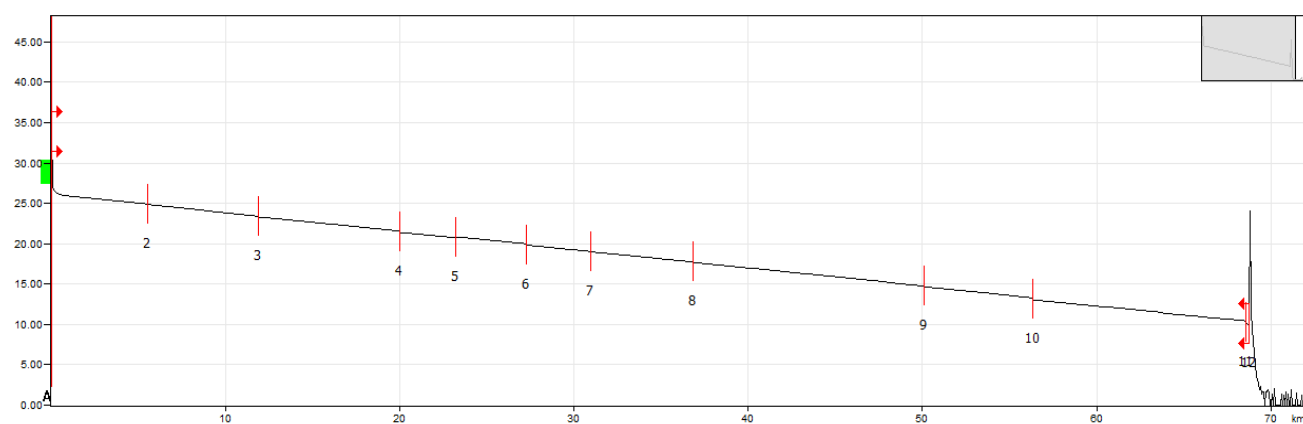
Figura 3.3. Trazo del enlace del sitio A-sitio B. Fibra 1.
