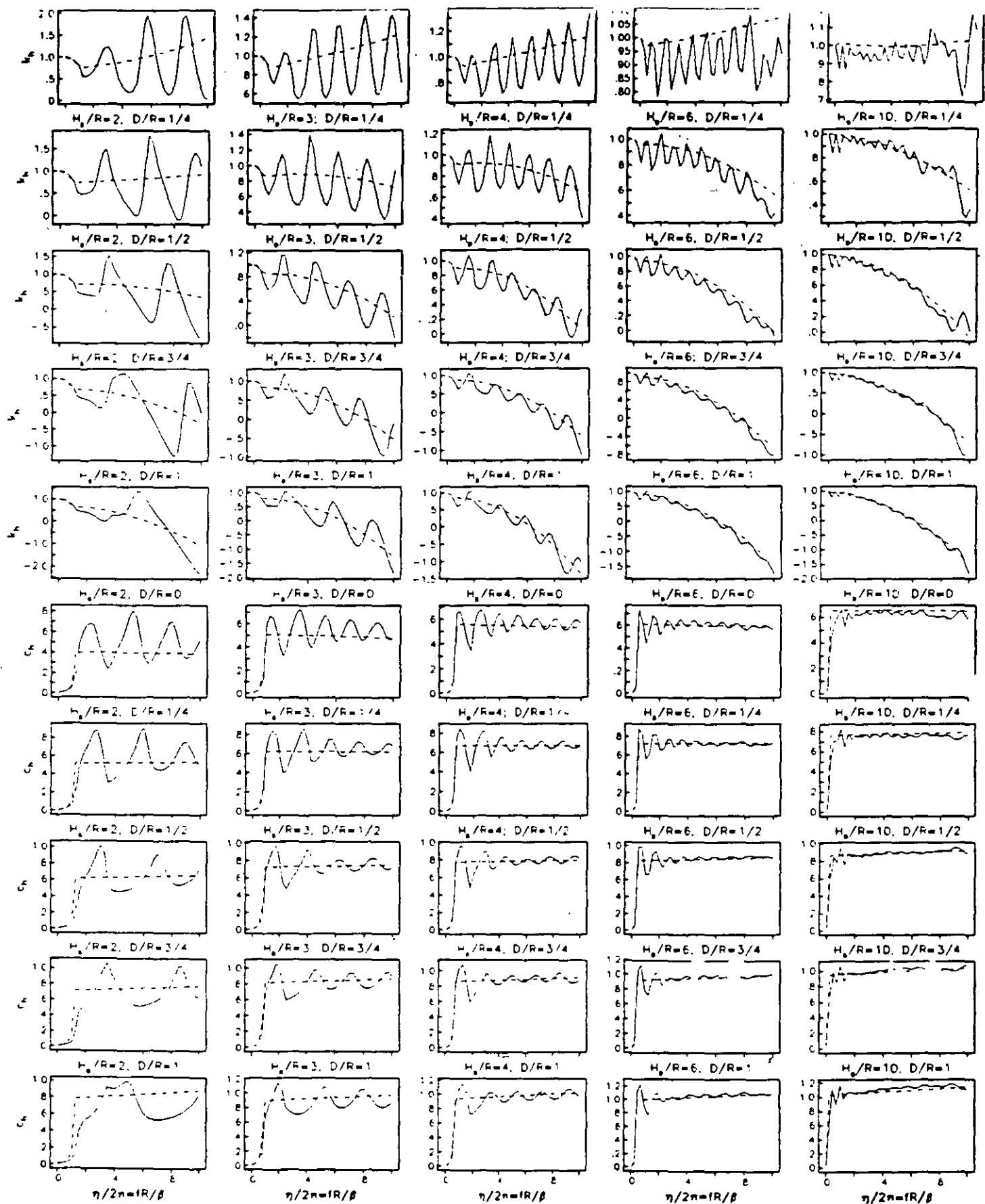
Fig 2.3.1 Coeficientes de rigidez k_n y amortiguamiento c_n para \nu=1/2 ; funciones rigurosas (linea continua), funciones aproximadas (linea discontinua)
