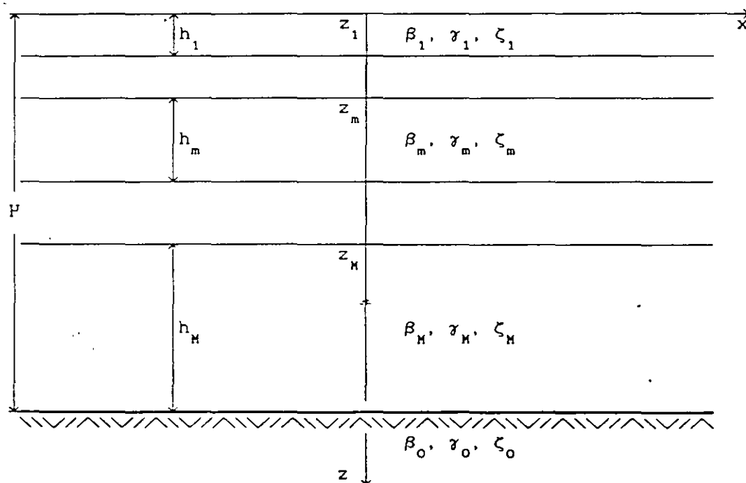
Fig. 1 Depósito estratificado horizontalmente
