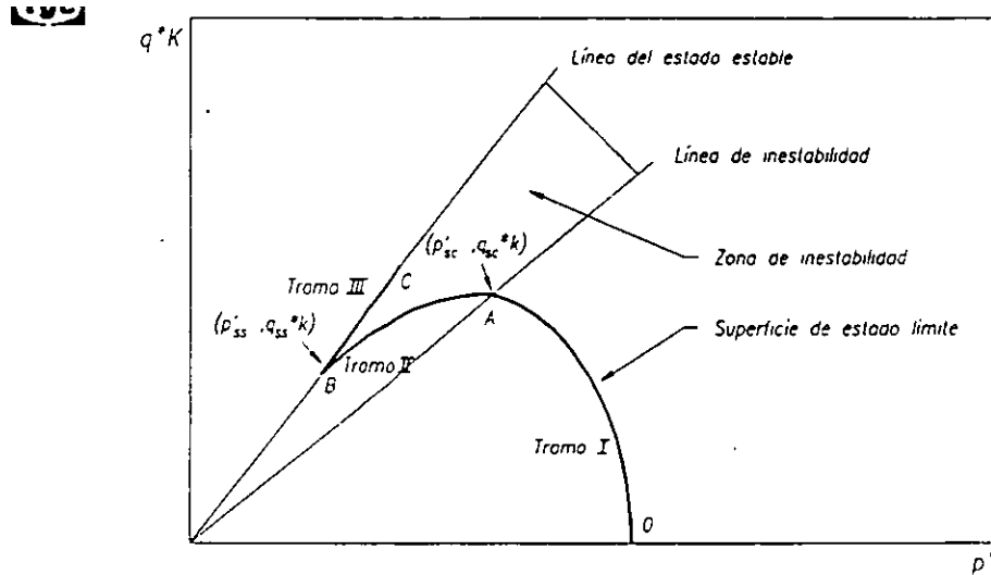
Fig 18 Identificación de la superficie de estado límite y la zona de inestabilidad
