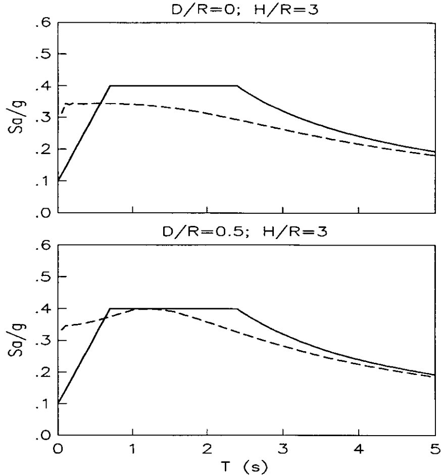
Fig. 21. Espectros de diseño para el sitio SCT con (---) y sin (—) efectos de interacción
