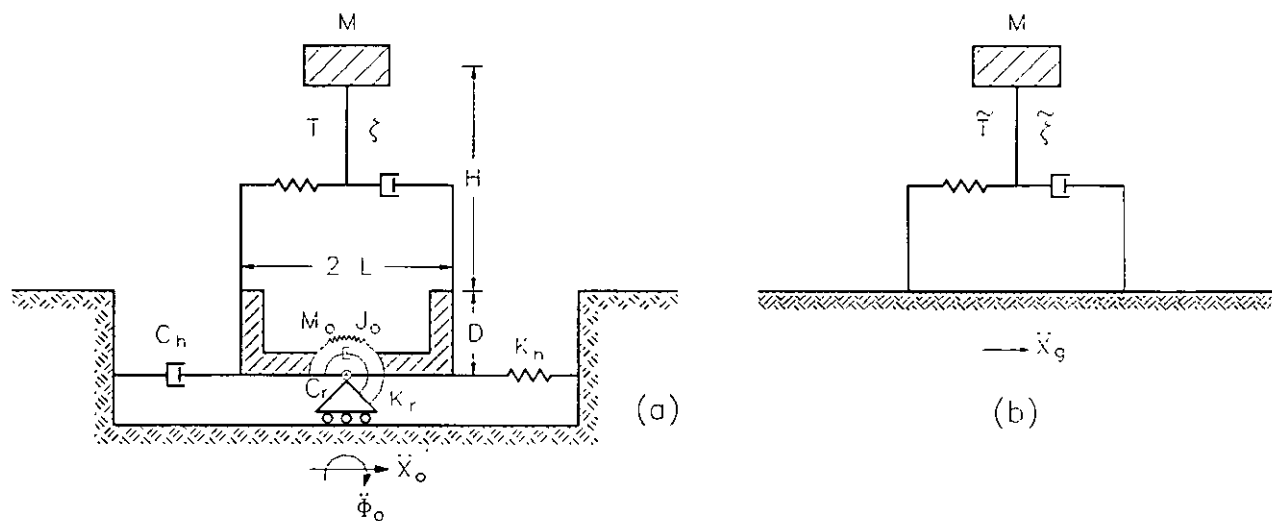
Fig. 9. (a) Sistema suelo-estructura sujeto al movimiento efectivo de la cimentación y (b) oscilador de reemplazo sujeto al movimiento de campo libre
