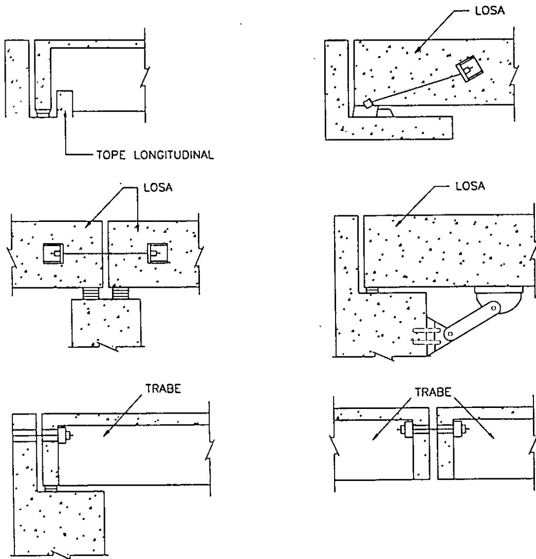
UNIONES ENTRE CLAROS Y ENTRE SUPERESTRUCTURA Y SUBESTRUCTURA
