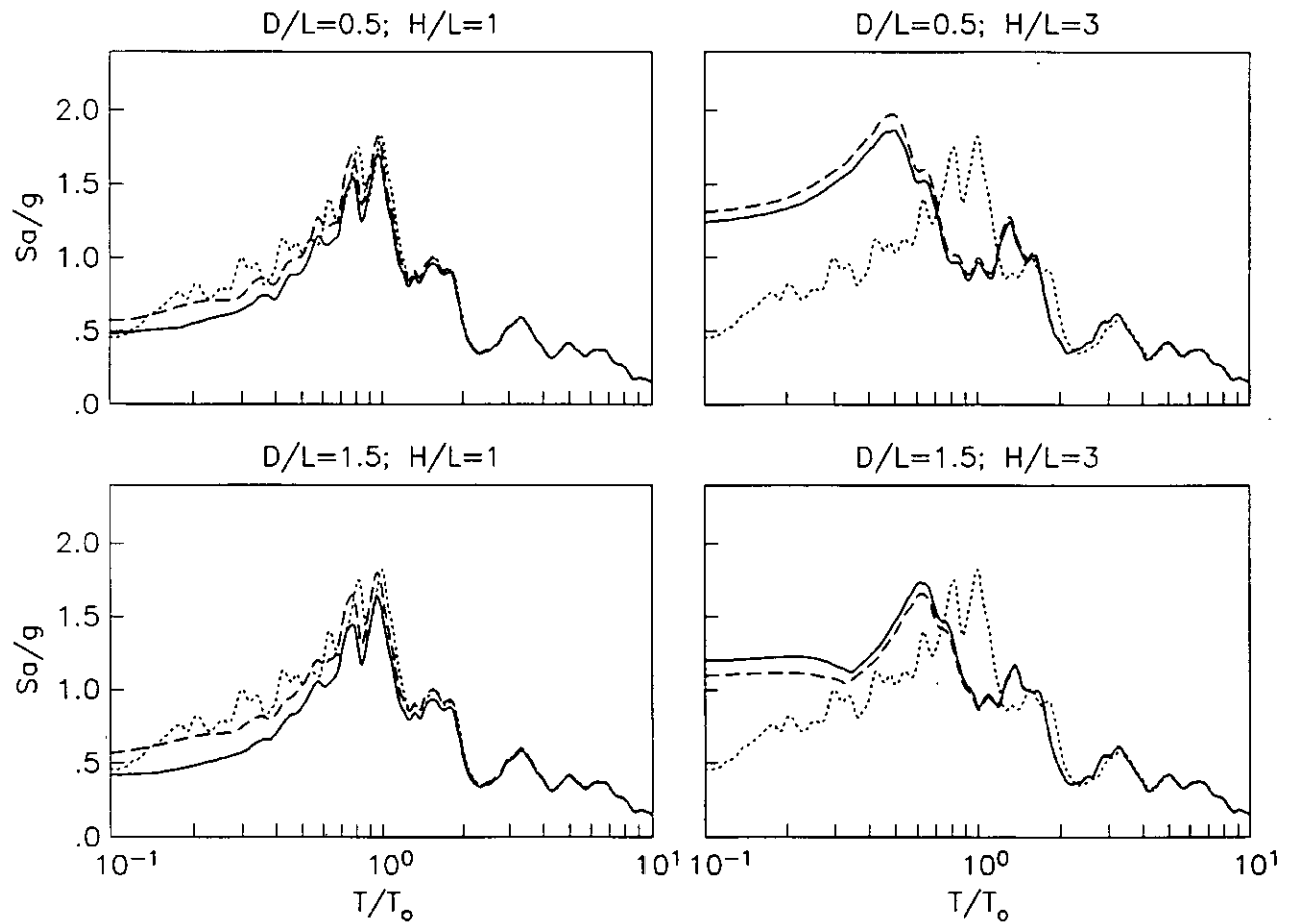
Fig. 15. Espectros de respuesta para L/\beta T_n = 0.08 sin efectos de interacción (.....), considerando sólo la interacción inercial (---) e incluyendo la interacción cinemática (—)
