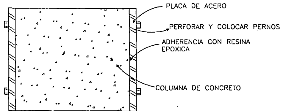
SECCION TRANSVERSAL
