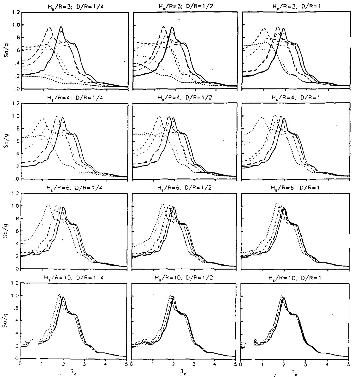
Fig 2 Espectros de respuesta con efectos de interacción cinemática para el sitio SCT. Con línea gruesa cálculos rigurosos y con línea delgada cálculos aproximados
