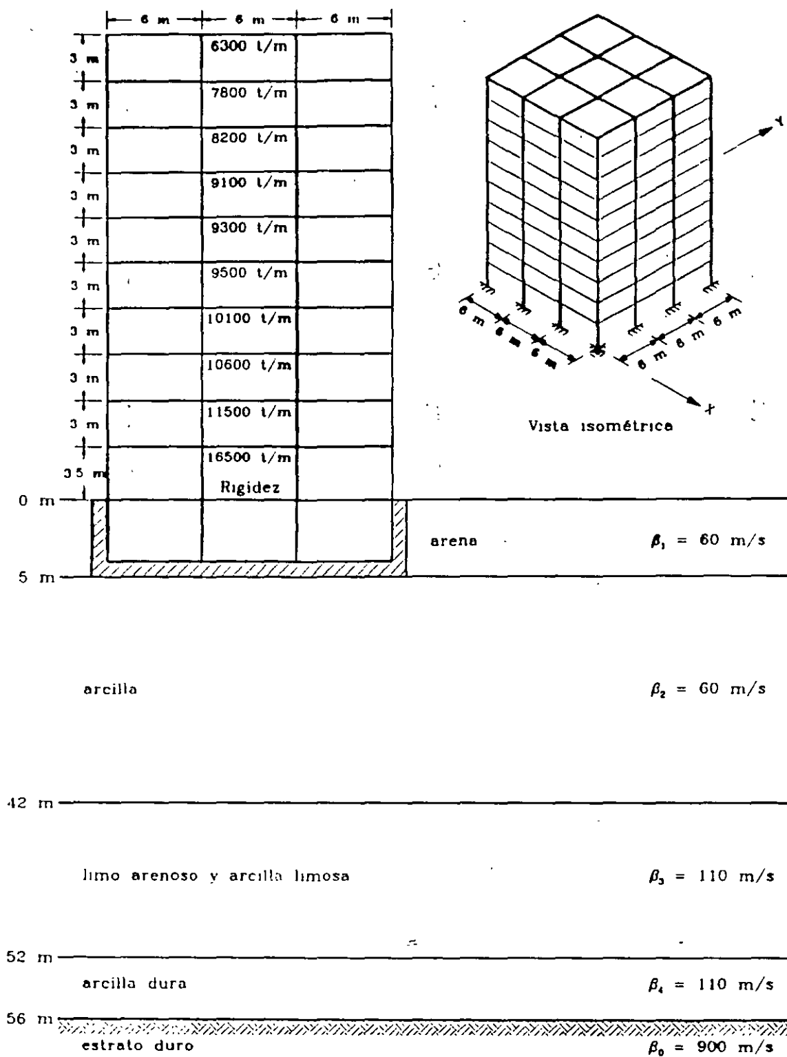
Fig 3.1 Sistema suelo-estructura
