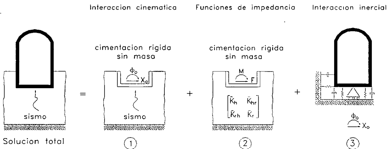
Fig. 2. Solución en tres pasos de la interacción suelo-estructura
