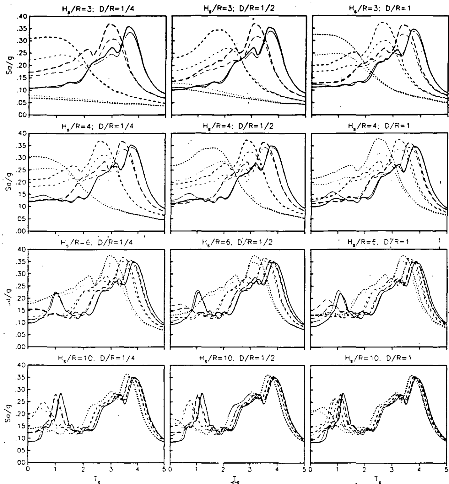
Fig 3 Espectros de respuesta con efectos de interacción cinemática para el sitio CAO Con línea gruesa cálculos rigurosos y con línea delgada cálculos aproximados
