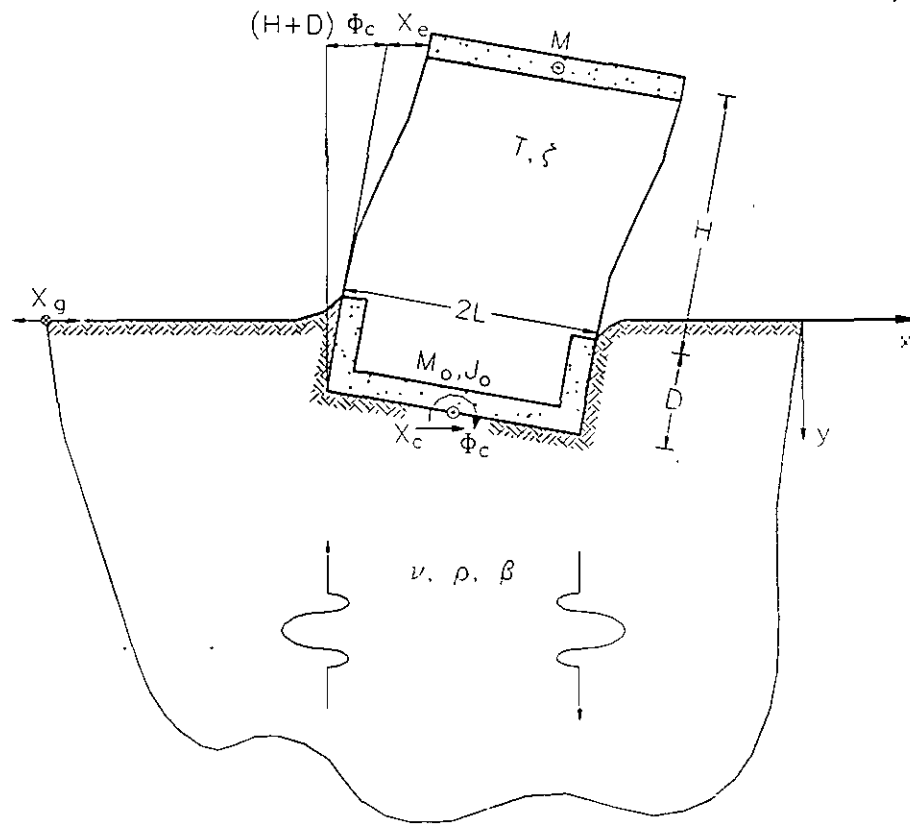
Fig. 8. Modelo para considerar los efectos de interacción suelo-estructura en el modo fundamental
