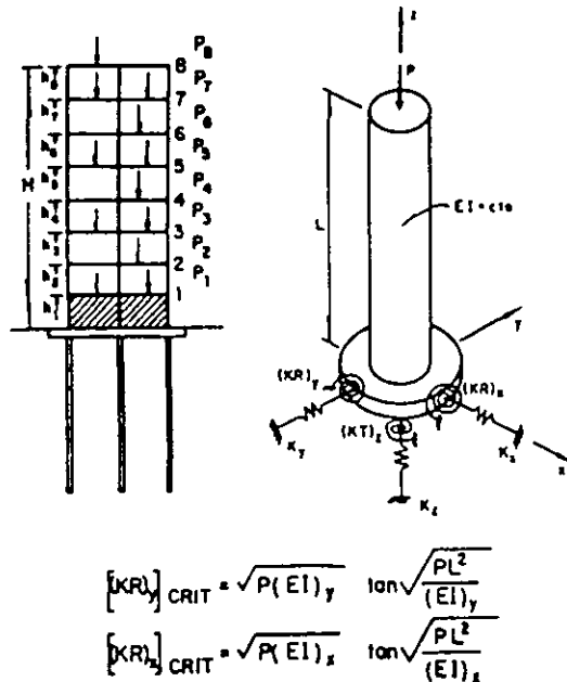
Fig 1. Modelos para estudio de estabilidad de un edificio con efectos de interacción suelo-estructura
