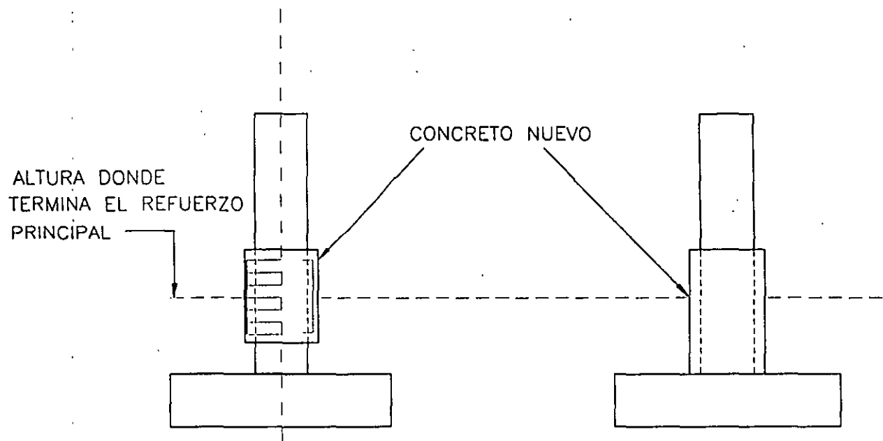
(A) SECCION NUEVA DE CONCRETO
