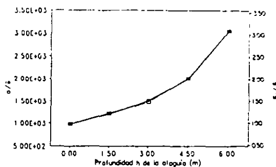
a. Cambio en la rigidez lineal vertical
