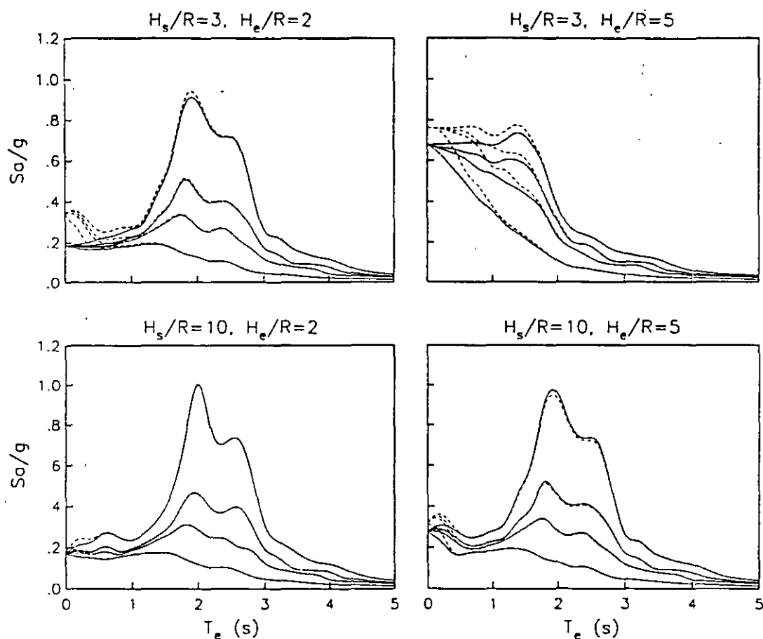
Figura 19. Espectros de respuesta inelásticos de sistemas suelo-estructura con \zeta_s = \zeta_e = 0.05 , v_s = 0.5 y D/R = 1 , en el sitio SCT; se analiza el sistema acoplado (línea continua) y el oscilador de remplazo (línea discontinua).
