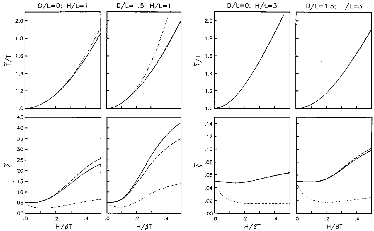
Fig. 12. Periodos y amortiguamientos efectivos para ondas SV con incidencia respecto a la vertical \gamma = 0^\circ (—), 30^\circ (---) y 60^\circ (.....)
