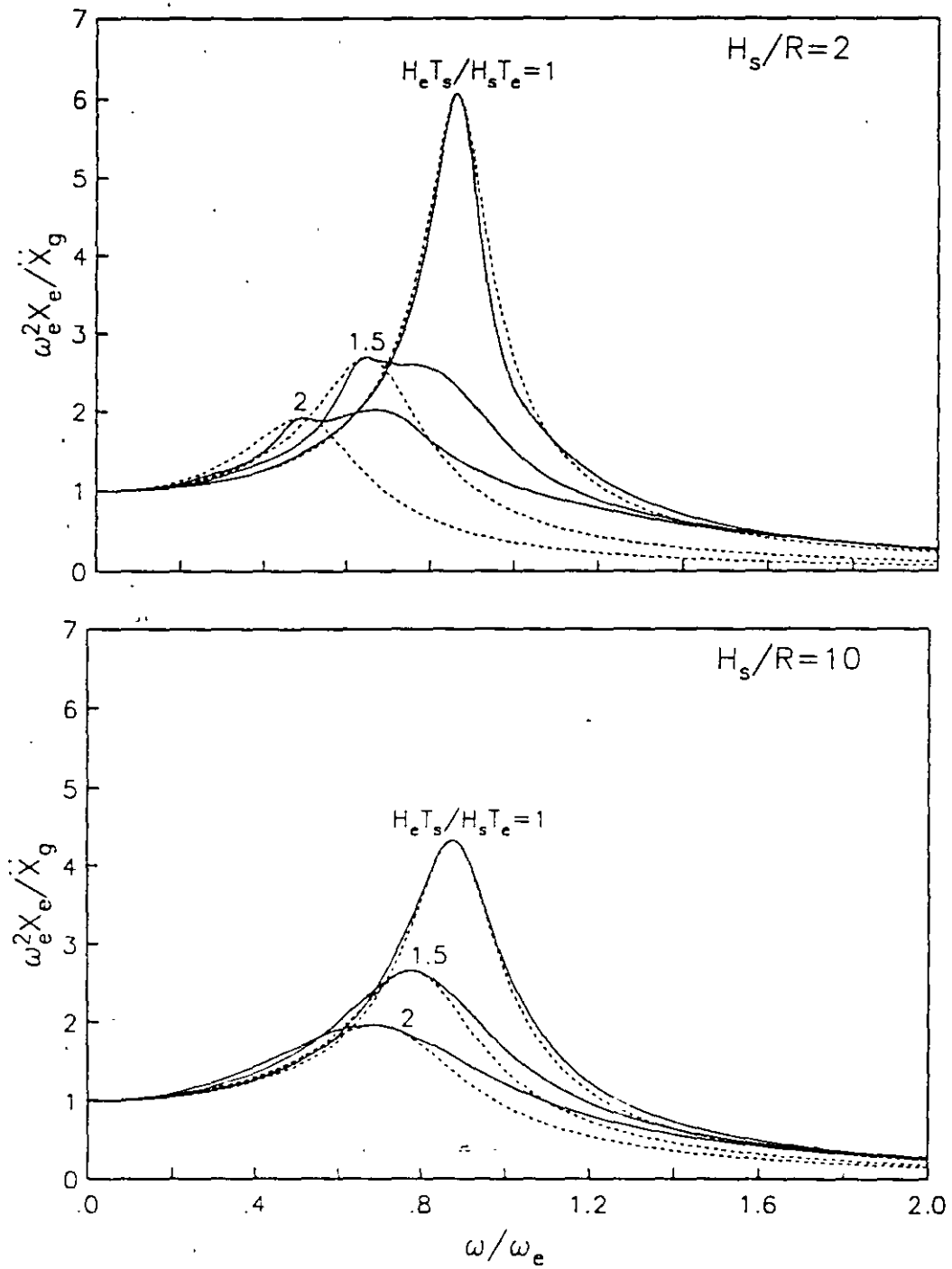
Figura 15. Funciones de transferencia de pseudoaceleración para sistemas acoplados con \zeta_s = \zeta_e = 0.05 , \nu_s = 1/3 , D/R = 1 y H_e/R = 1 , comparadas con las correspondientes del oscilador de reemplazo.
