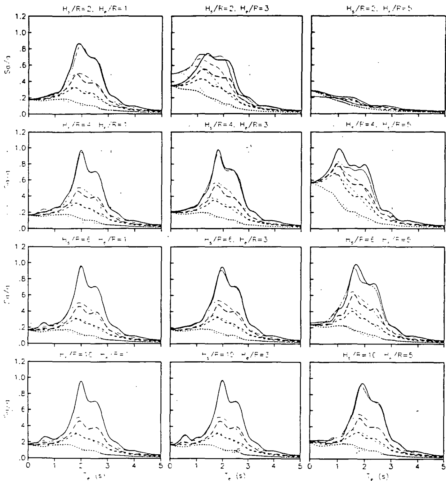
Fig 2 Comparacion de espectros de respuesta inelasticos calculados para configuraciones suelo-estructura con D/R=1 (sitio SCT). Con trazo grueso se indican los espectros calculados mediante integrales de convolucion. Con trazo fino se indican los espectros calculados haciendo uso de un metodo lineal equivalente y de un oscilador de reemplazo; ( — ) \mu=1 , ( --- ) \mu=1.5 , ( ---- ) \mu=2 , ( ..... ) \mu=4 .
