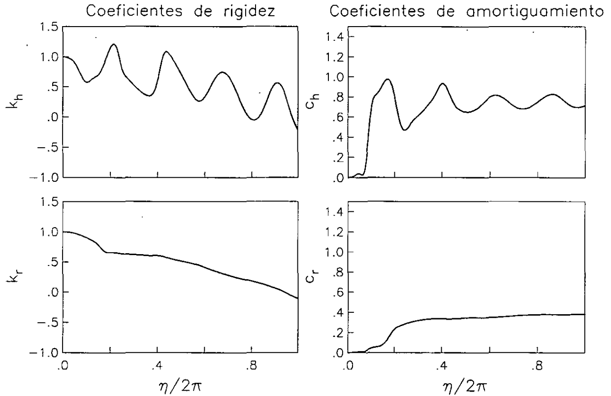
Fig. 6. Coeficientes de rigidez y amortiguamiento para los modos de traslación horizontal (subíndice h ) y cabeceo (subíndice r ) en un estrato de suelo con E/R = 3
