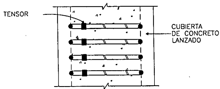
SECCION TRANSVERSAL
