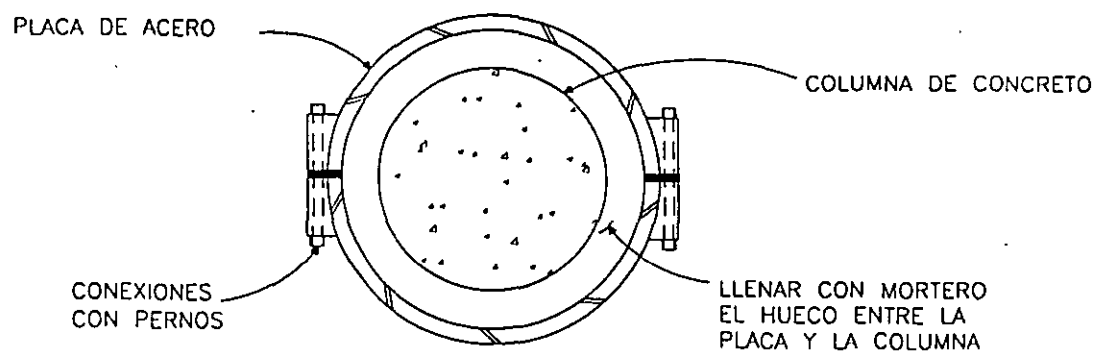
SECCION TRANSVERSAL
