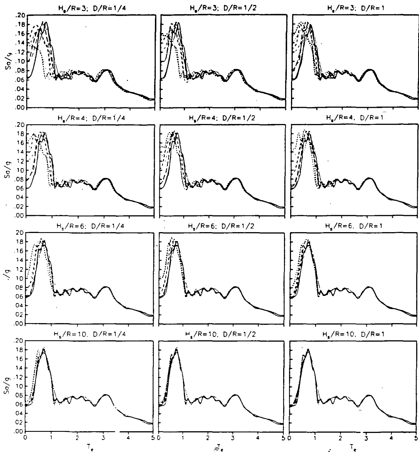
Fig 1 Espectros de respuesta con efectos de interacción cinemática para el sitio VIV. Con línea gruesa cálculos rigurosos y con línea delgada cálculos aproximados
