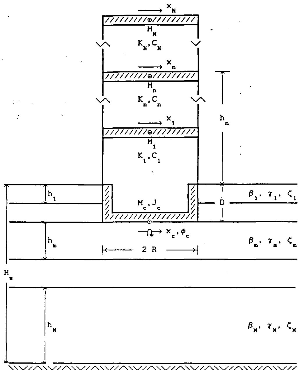
Fig.1 Sistema suelo-estructura
