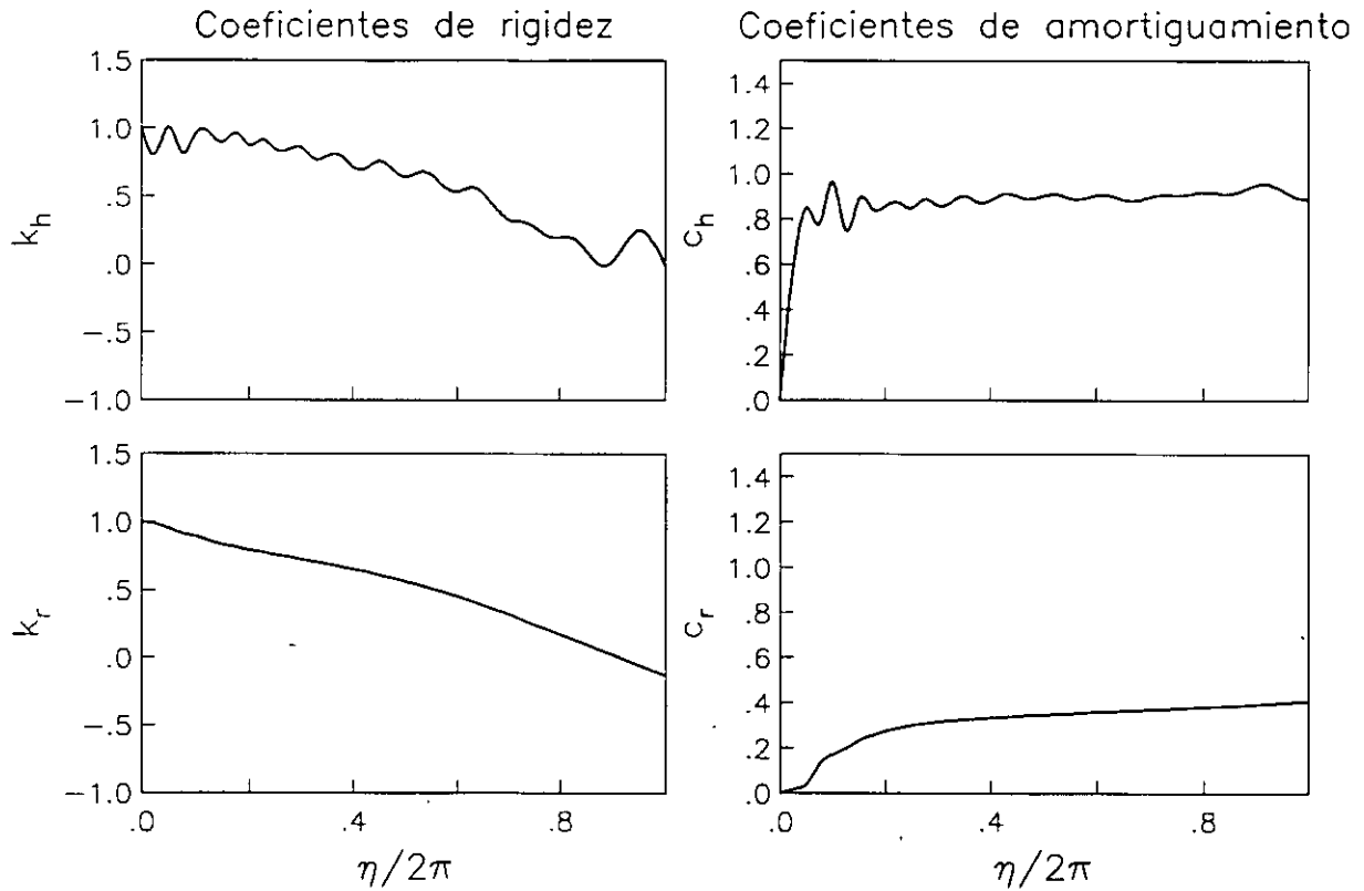
Fig. 7. Coeficientes de rigidez y amortiguamiento para los modos de traslación horizontal (subíndice h ) y cabeceo (subíndice r ) en un estrato de suelo con E/R=10
