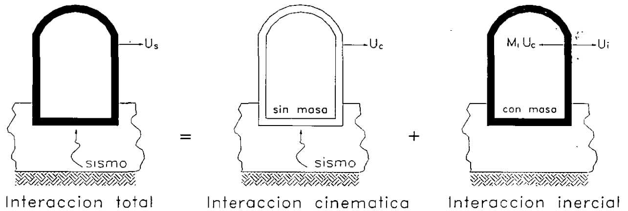
Fig. 1. Teorema de superposición de la interacción suelo-estructura
