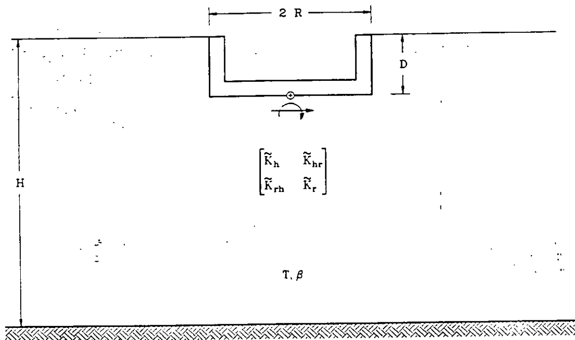
Fig. 3 Sistema suelo-cimentación
