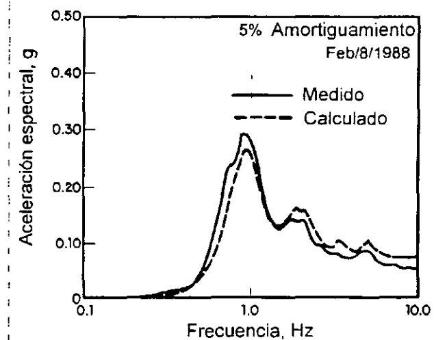
Fig 33. Espectros de respuesta en el sitio D54
