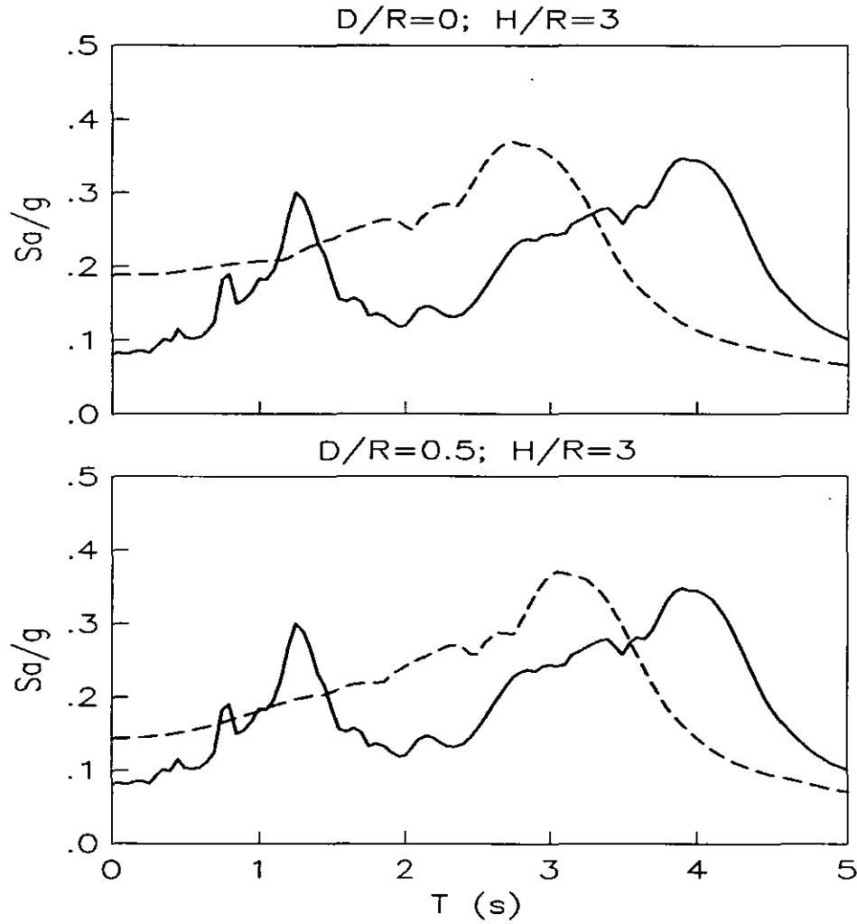
Fig. 19. Espectros de respuesta para el sitio CAO considerando sólo la interacción inercial, para R/\beta = 0 (—) y 0.31 (---) s
