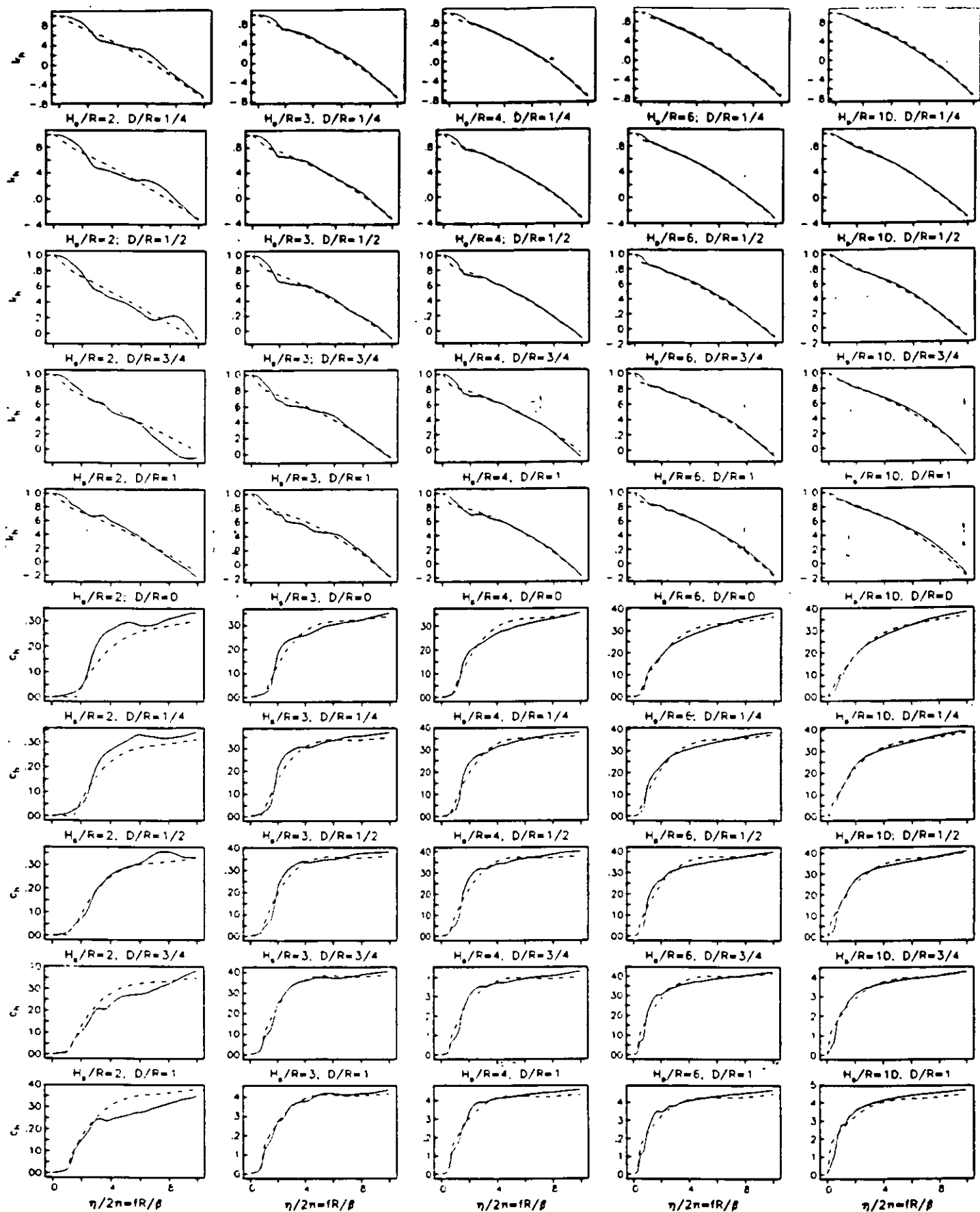
Fig 2.3.2 Coeficientes de rigidez k_r y k_h y amortiguamiento c_r y c_h para \nu=1/2 ; funciones rigurosas (linea continua), funciones aproximadas (linea discontinua)
