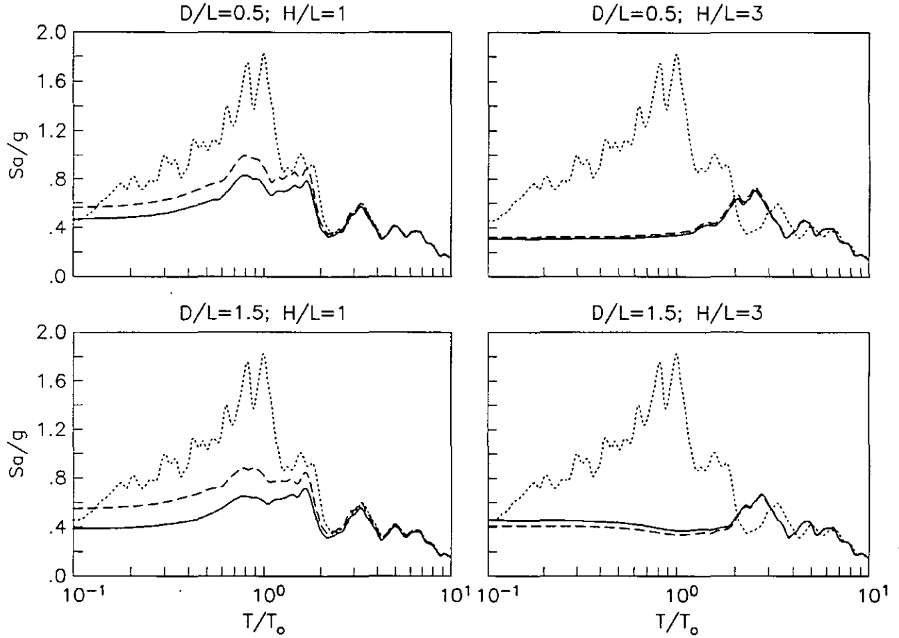
Fig. 16. Espectros de respuesta para L/\beta T_o = 0.2 sin efectos de interacción (.....), considerando sólo la interacción inercial (---) e incluyendo la interacción cinemática (—)
