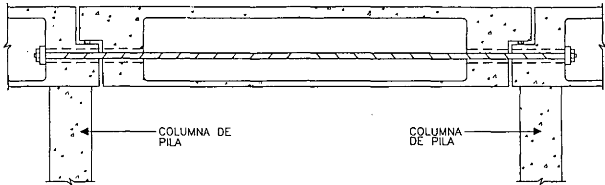
REFUERZO DE UN CLARO SUSPENDIDO
