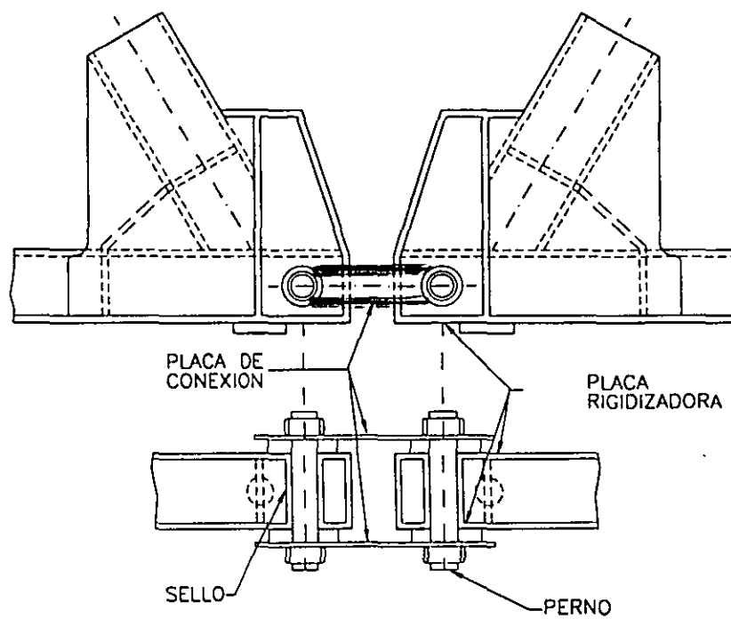
DISPOSITIVO DE CONEXION PARA ARMADURAS
