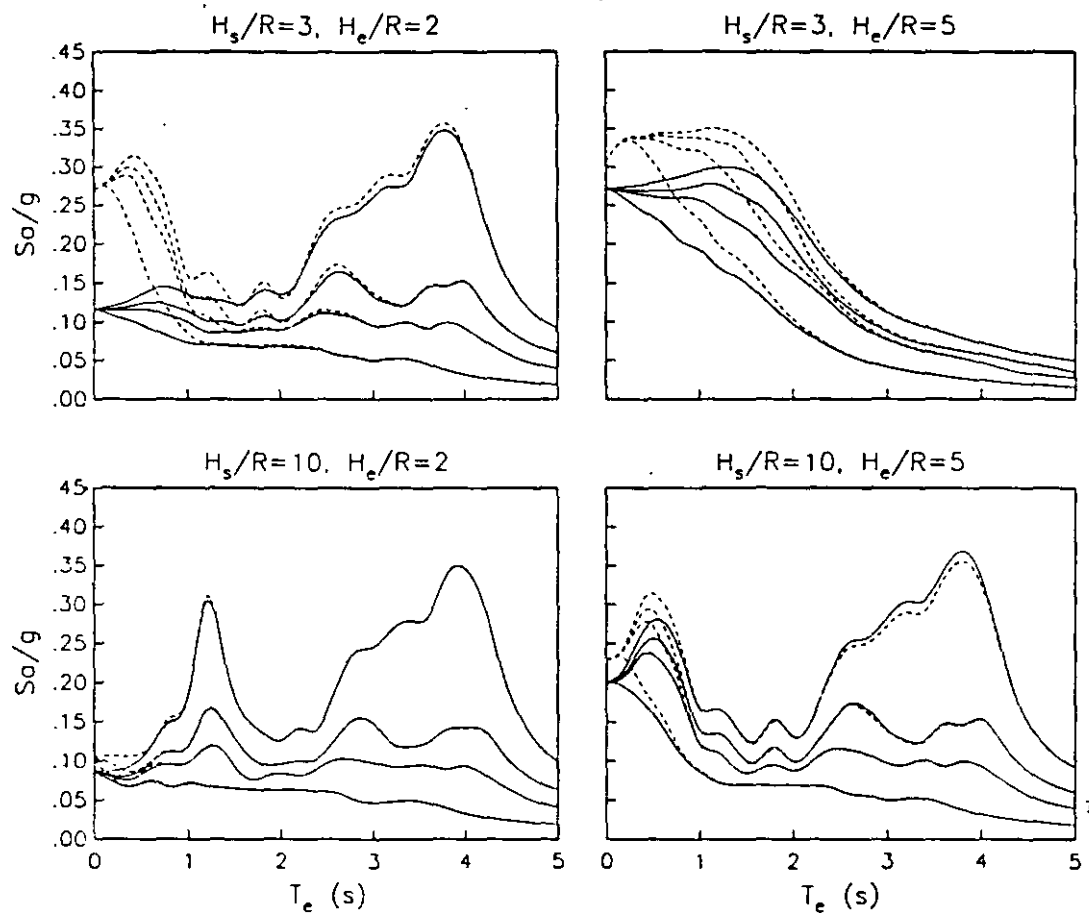
Figura 20. Espectros de respuesta inelásticos de sistemas suelo-estructura con \zeta_s = \zeta_r = 0.05 , v_s = 0.5 y D/R = 1 , en el sitio CAO; se analiza el sistema acoplado (línea continua) y el oscilador de reemplazo (línea discontinua).
