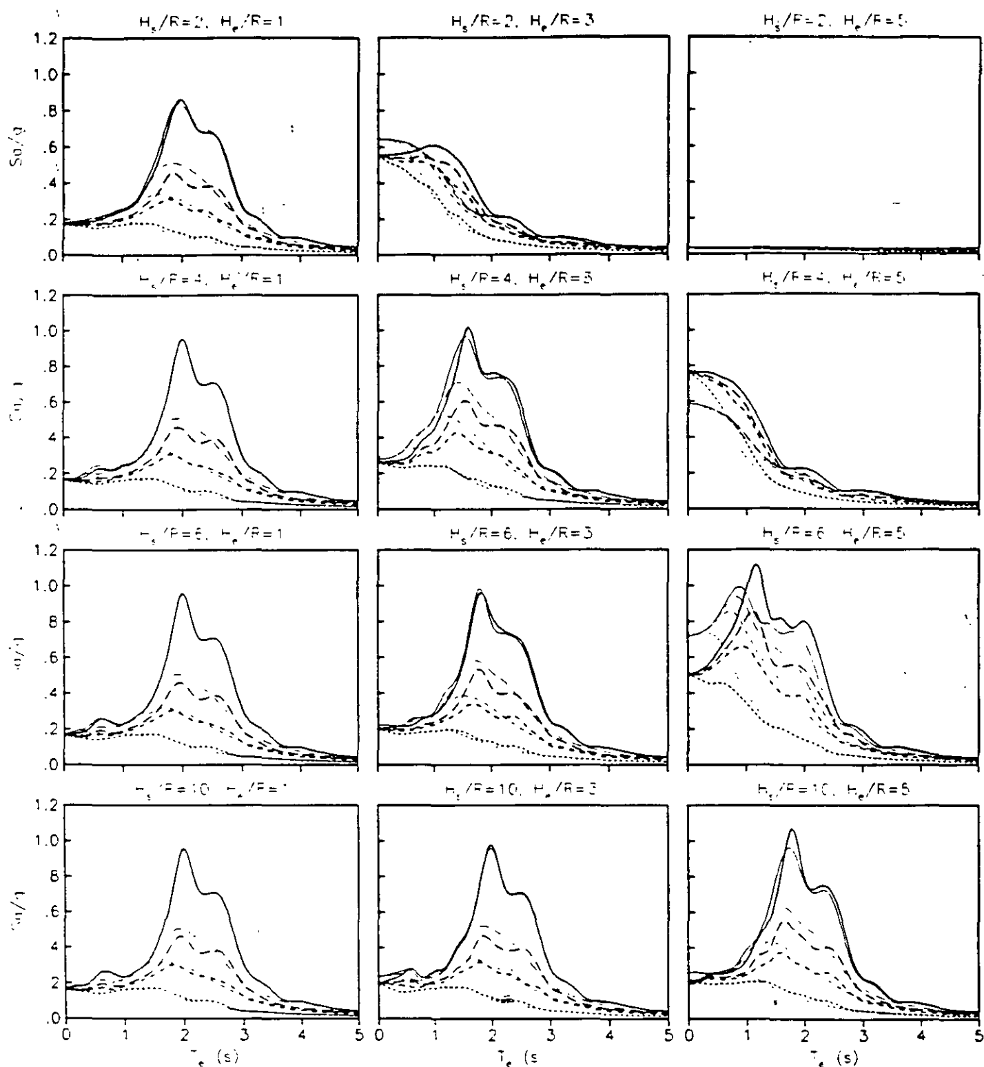
Fig 1 Comparacion de espectros de respuesta inelasticos calculados para configuraciones suelo-estructura con D/R=0 (sitio SCT). Con trazo grueso se indican los espectros calculados mediante integrales de convolucion. Con trazo fino se indican los espectros calculados haciendo uso de un metodo lineal equivalente y de un oscilador de reemplazo; ( — ) \mu=1 , ( --- ) \mu=1.5 , ( -.-.- ) \mu=2 , ( ..... ) \mu=4 .
