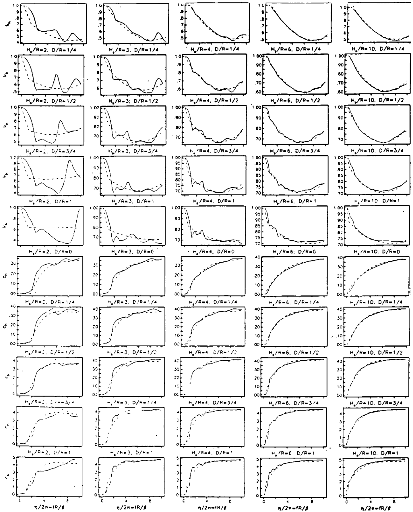
Fig 2.1.2 Coeficientes de rigidez k_r y amortiguamiento c_r para \nu=1/3 ; funciones rigurosas (línea continua), funciones aproximadas (línea discontinua)
