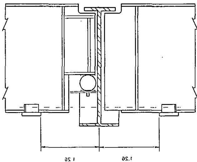
ELEVACION
