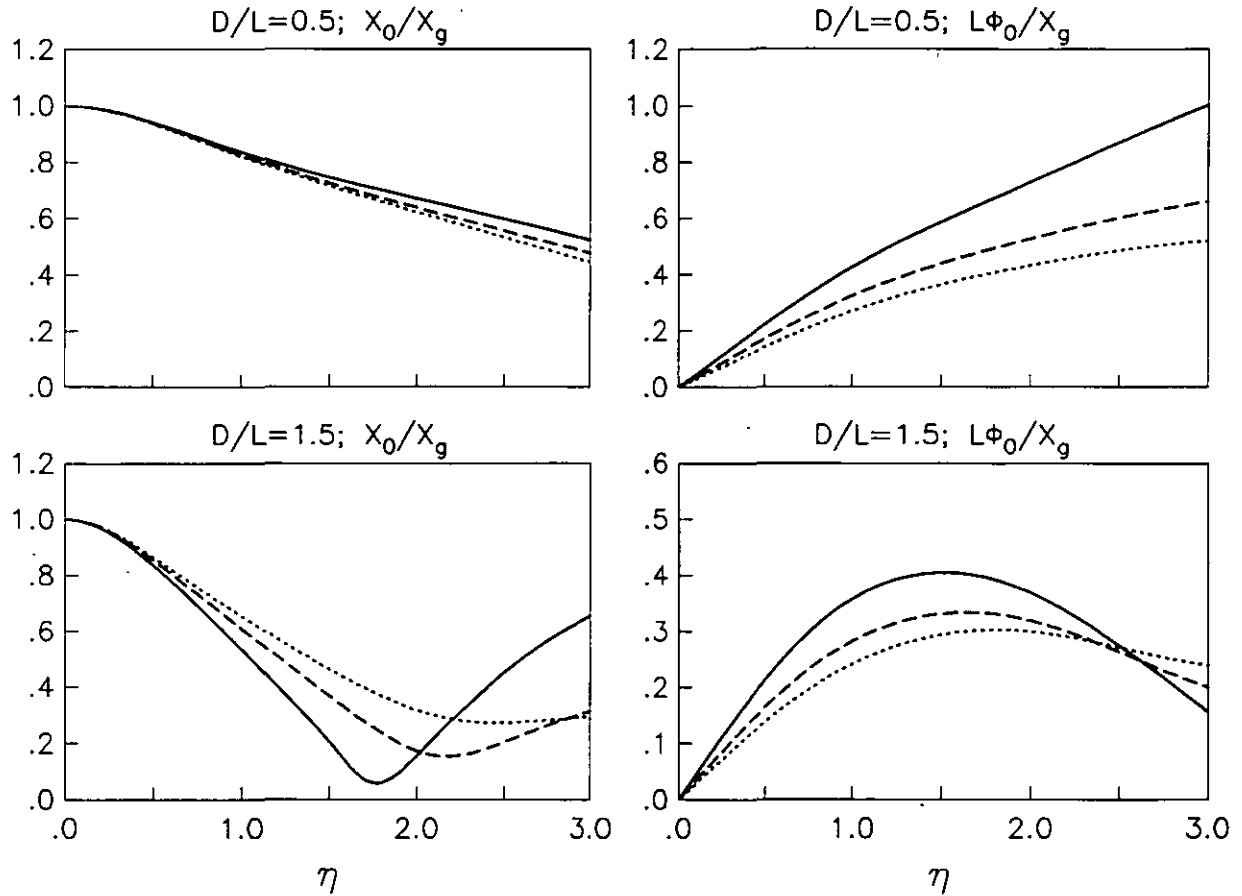
Fig. 4. Amplitud de los movimientos efectivos de la cimentación para ondas P con incidencia respecto a la vertical \gamma = 30^\circ (—), 60^\circ (---) y 90^\circ (.....)
