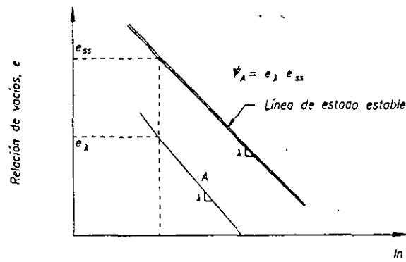
a) Parámetro de estado de Been y Jefferies (1985)
