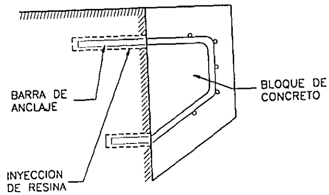
COLOCACION DE BLOQUE DE CONCRETO
