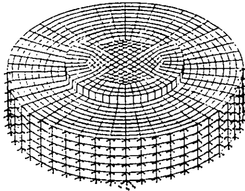
Fig 4. Modelo de elementos finitos seleccionado para representar a una placa circular sobre un semiespacio elástico
