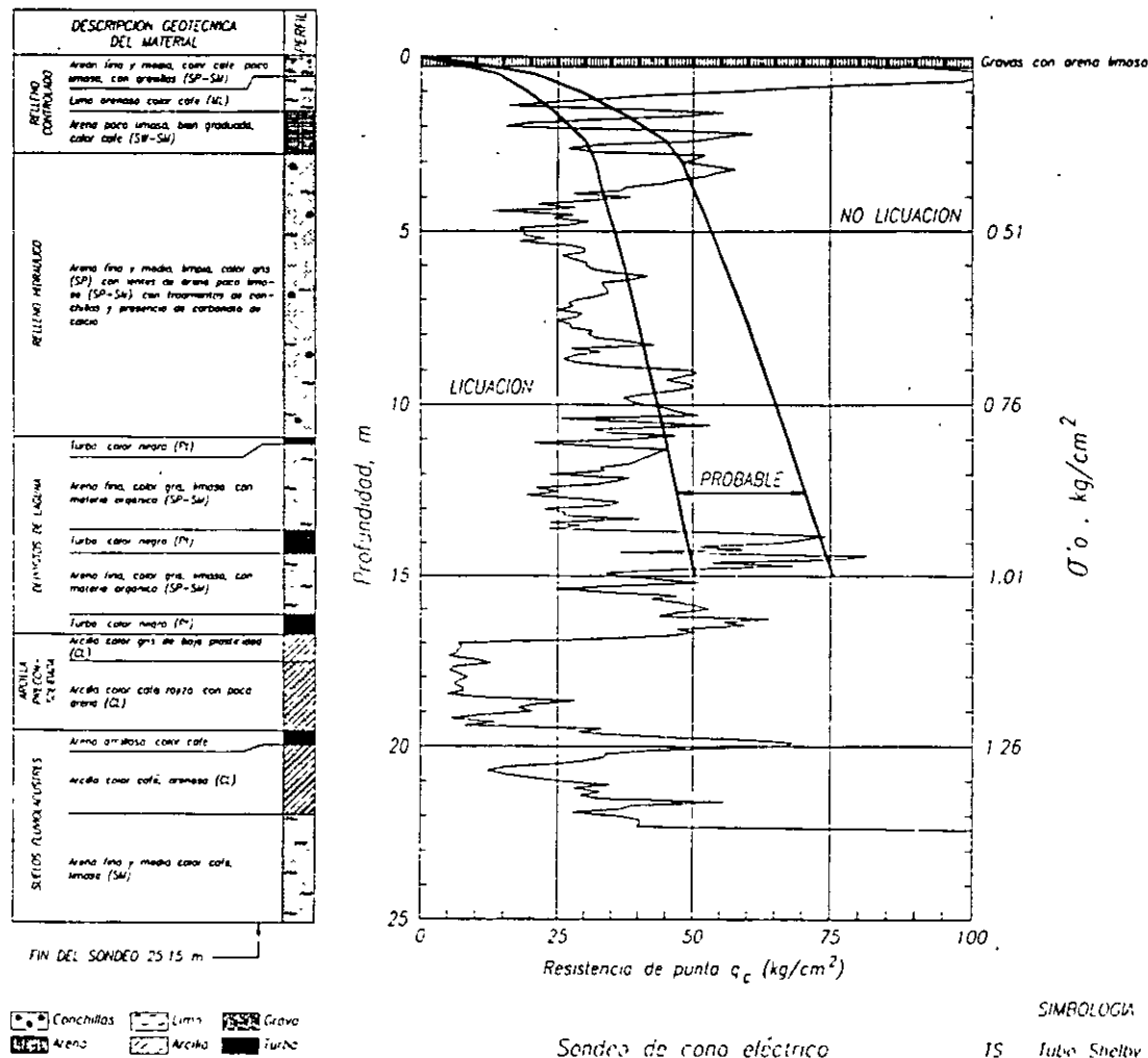
Fig 24 Aplicación del criterio de Robertson (1992)
