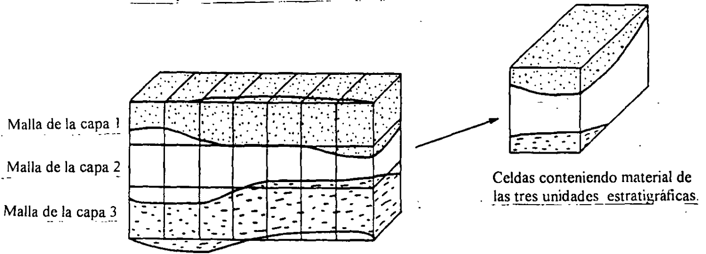
(b) Esquema del acuífero con una malla rectilínea sobrepuesta.
