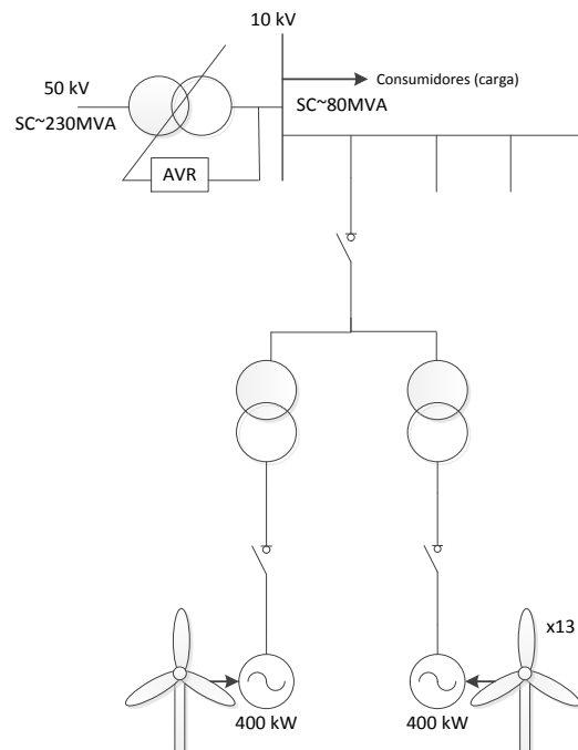
Figura 2. 6 Conexión típica de parque eólico [14]
