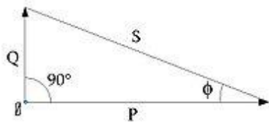
Figura 2. 25 Triángulo de potencias activa (P), reactiva (Q) y aparente (S)
