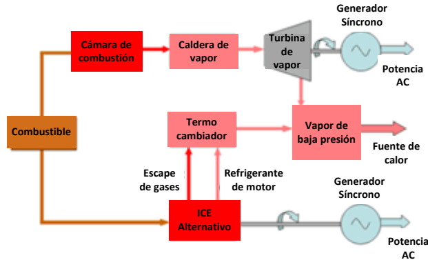
Figura A. 5CHP de recuperación de calor [11]
