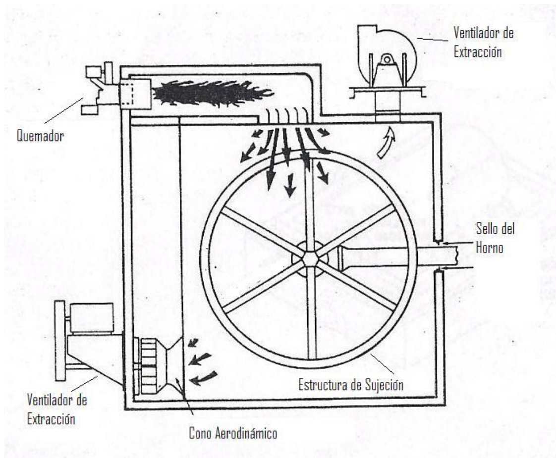
Figura 2.3.C Esquema de un horno de rotomoldeo. [4]
