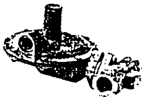
Serie-S100 Entrada Máxima: 125 Psi Presión de Salida: 5.5 a 8.5 C.A. Conexión: 19 mm (3/4") y 25 mm (1") N.P.T.
