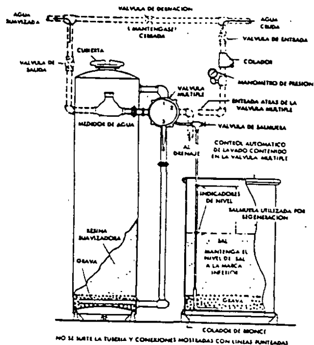
DIAGRAMA DE INSTALACION
