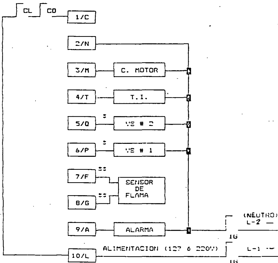
Diagrama eléctrico de alambado exterior
