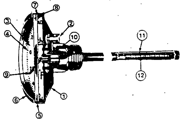
1.- Caja; 2.- Recalibrador; 3.- Carátula; 4.- Escalas; 5.- Cristal; 6.- Bisel; 7.- Empaque; 8.- Separador; 9.- Aguja; 10.- Buje; 11.- Vástago; 12.- Elemento Sensor Bimetálico.
