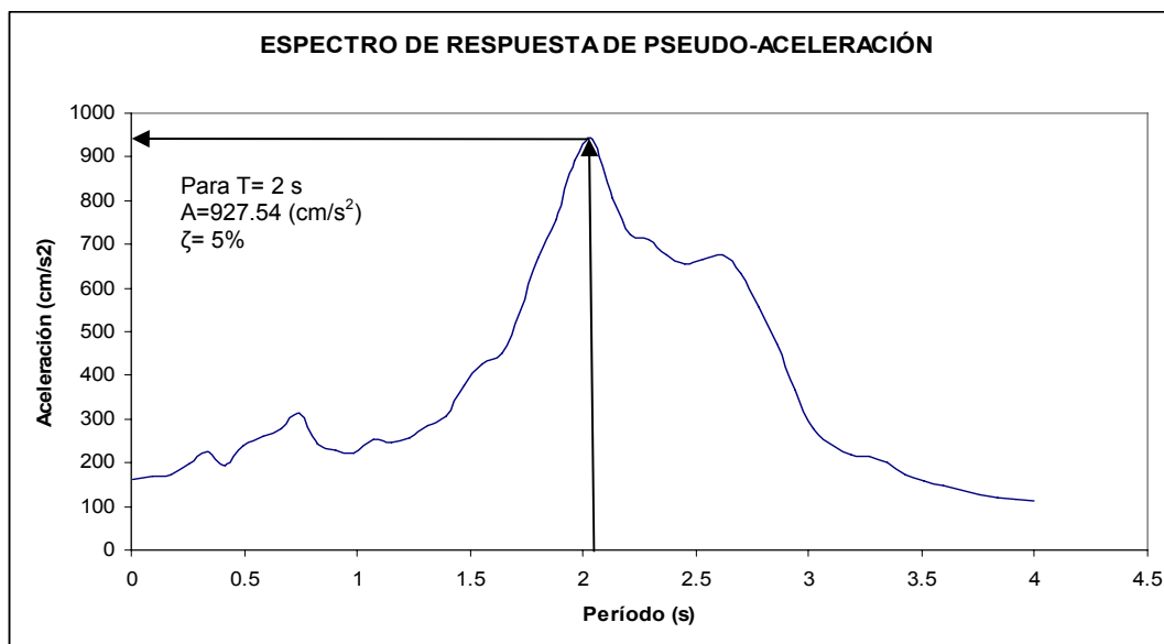
Figura A.4 Espectro de respuesta del registro de la Secretaría de Comunicaciones y Transportes (SCT) del temblor del 19 de septiembre de 1985.
