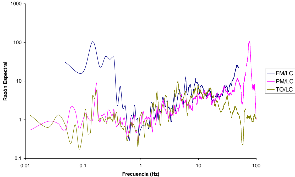
Figura II.6 Funciones de Transferencia para el sismo 23 (V)
