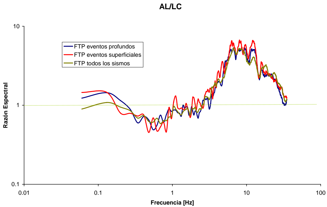
Figura II.10 Comparación de las FTP (L) obtenidas por los dos métodos de cálculo
