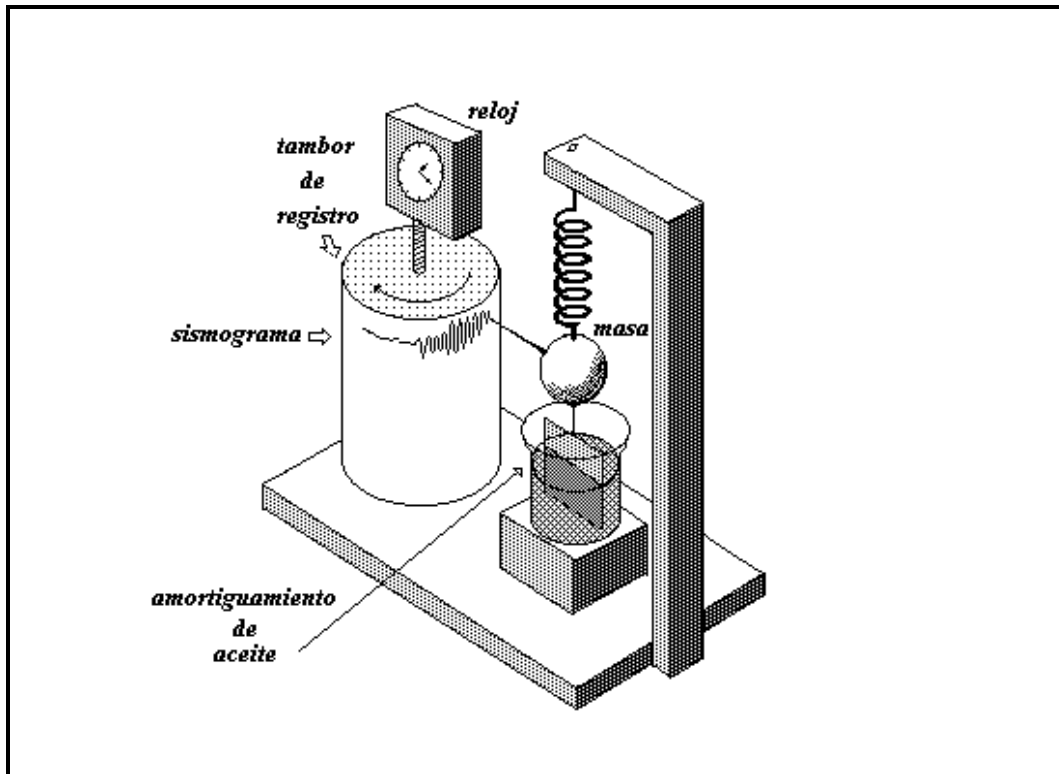
Figura I.1 Principio básico de operación y registro de un sismógrafo (ref. 8)
