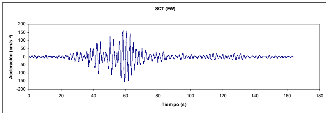
Figura A.1 Registro obtenido en la estación SCT (19/09/1985)
