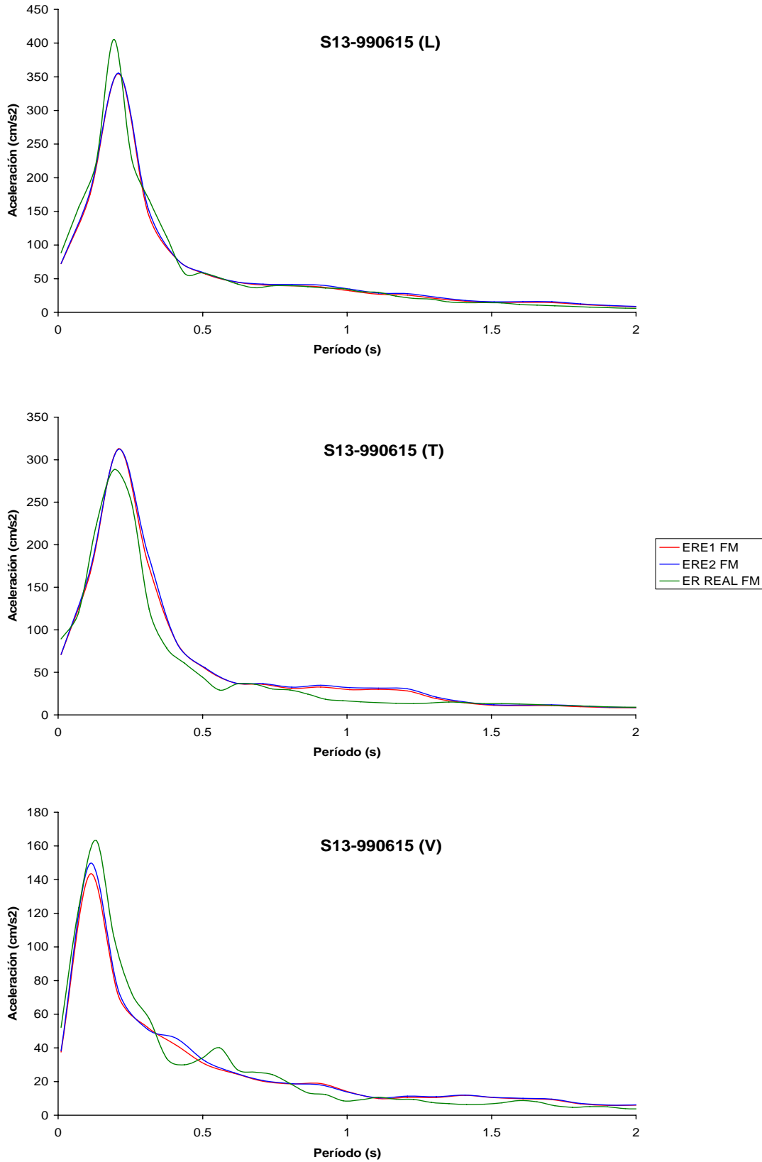
Figura III.13 Comparación de ER estimados con el ER real
