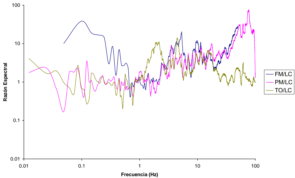
Figura II.5 Funciones de Transferencia para el sismo 23 (T)
