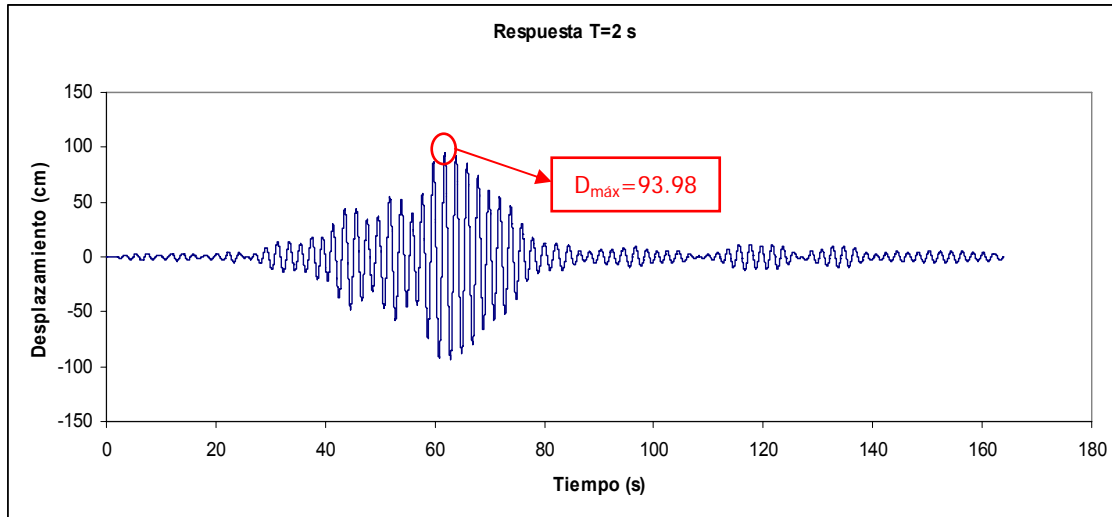
Figura A.3 Solución a la ecuación diferencial de movimiento para un período T=2(s) .
