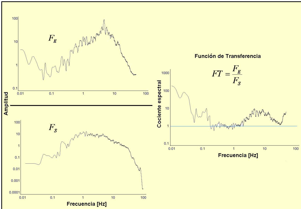
Figura II.3 Cálculo de la FT a partir del cociente espectral
