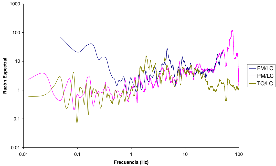
Figura II.4 Funciones de Transferencia para el sismo 23 (L)
