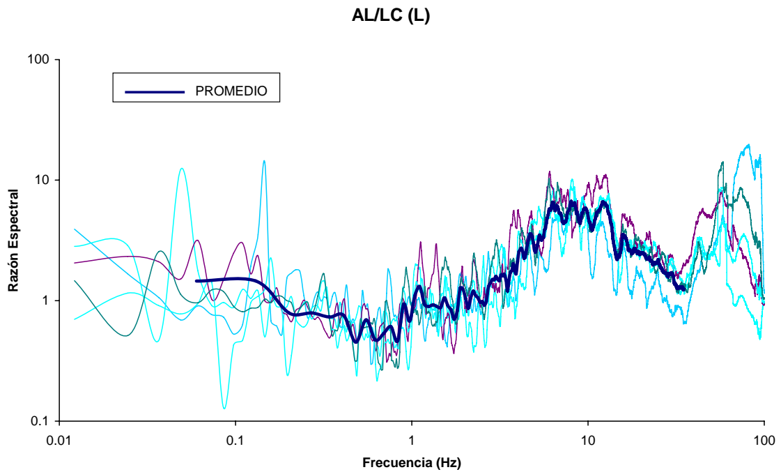
Figura II.7 Función de Transferencia Promedio eventos superficiales, L
