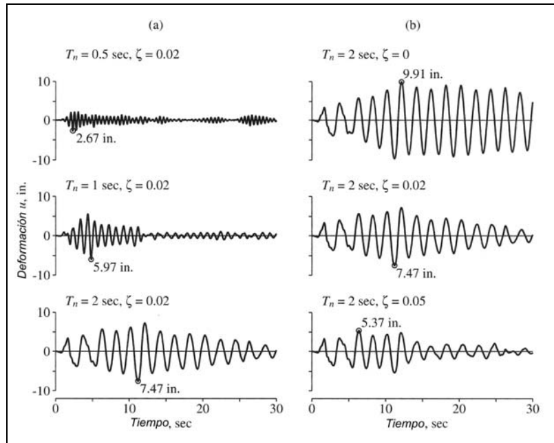
Figura III.4 Respuesta al desplazamiento de sistemas lineales de un grado de libertad (ref. 22)
