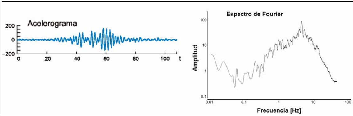
Figura II.2 Cálculo del EF a partir de un acelerograma
