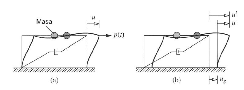
Figura III.2 Sistema de un grado de libertad.
