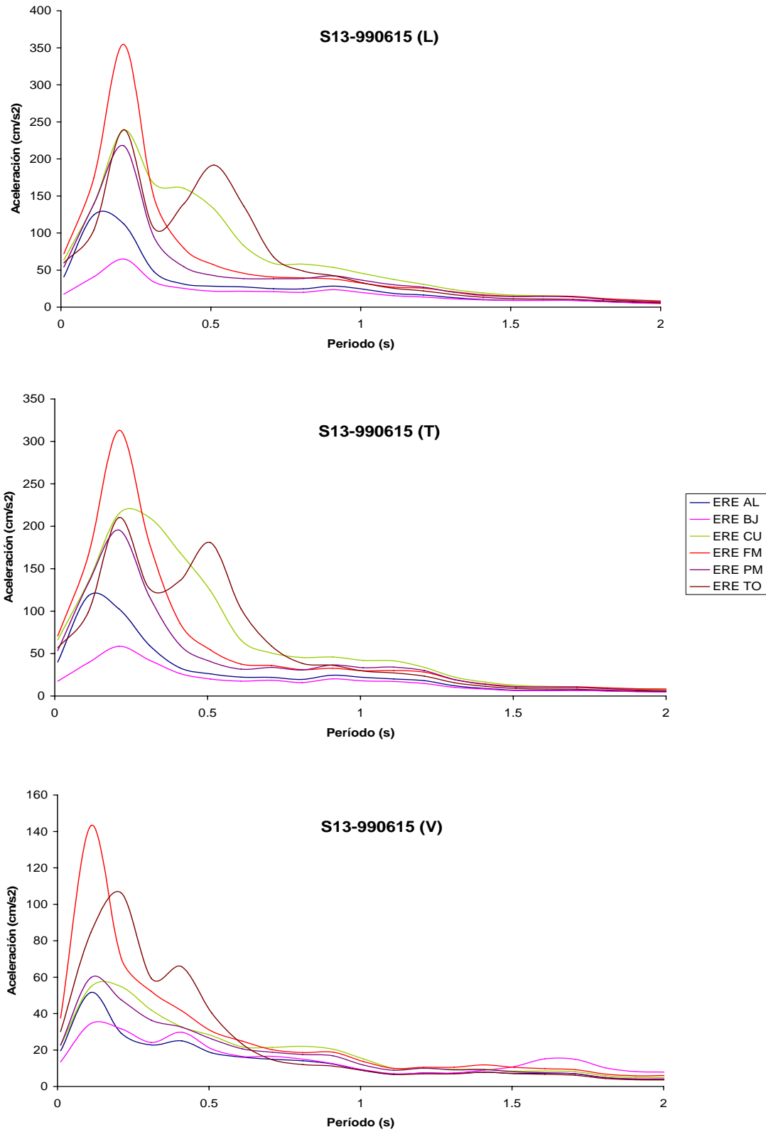
Figura III.11 Espectros de Respuesta Estimados con el primer método de cálculo
