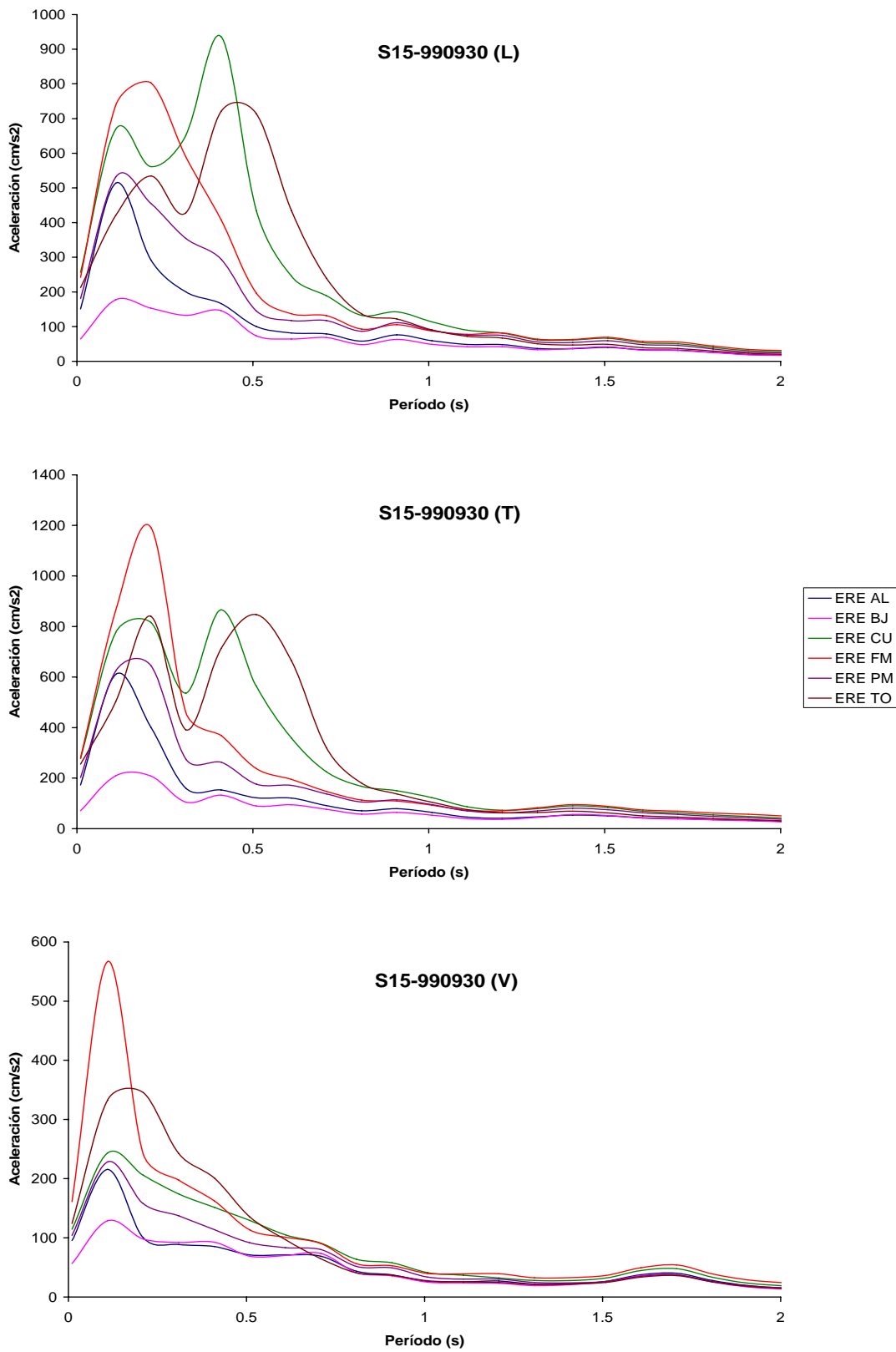
Figura III.15 Espectros de Respuesta Estimados con el segundo método de cálculo
