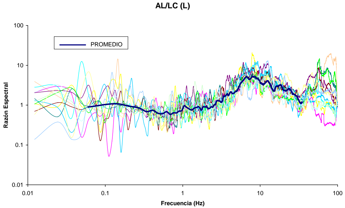
Figura II.9 Funciones de Transferencia para todos los sismos, L
