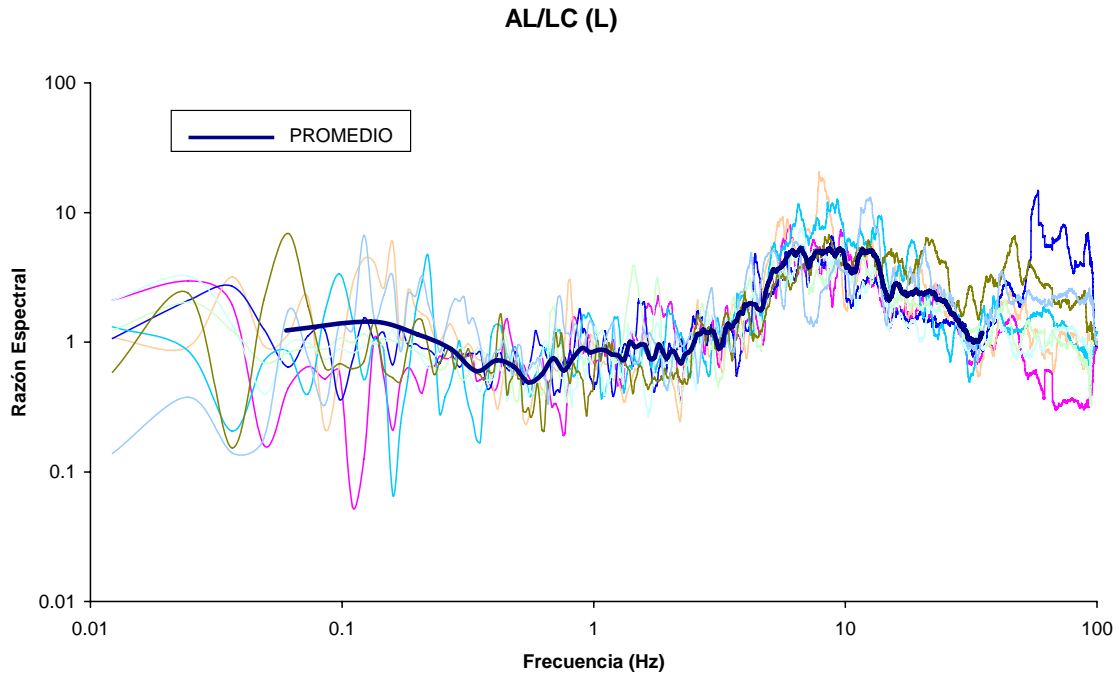
Figura II.8 Función de Transferencia Promedio eventos profundos, L
