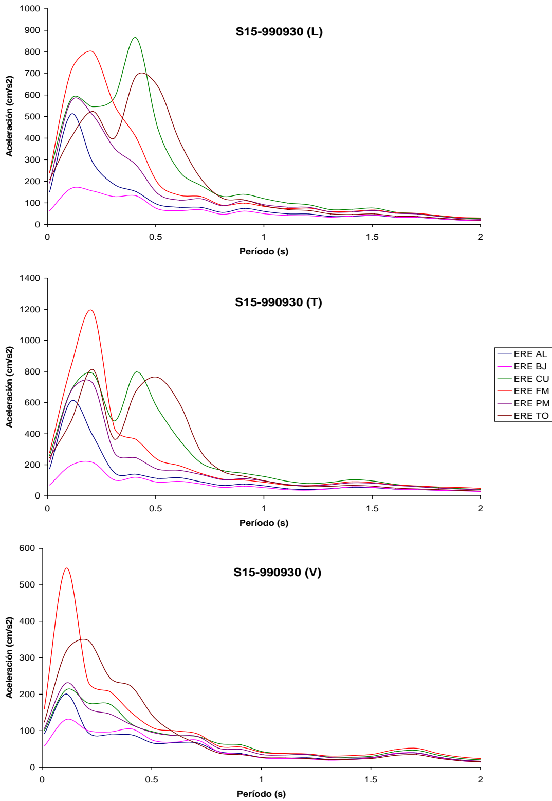
Figura III.14 Espectros de Respuesta Estimados con el primer método de cálculo
