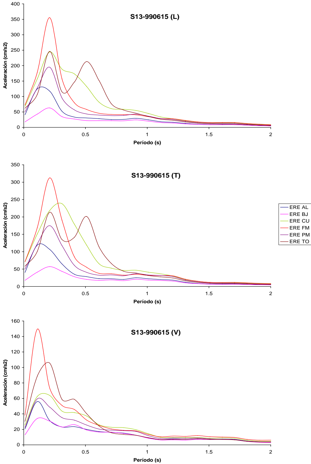
Figura III.12 Espectros de Respuesta Estimados con el segundo método de cálculo
