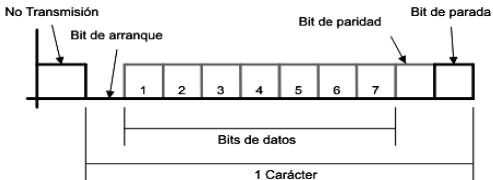
Figura 1.17 Transmisión asíncrona
