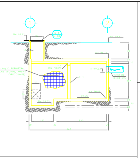
D-4 CORTE B-B' (ELEVACION) SIN ESC. REF.: D-1 y D-2/C-08b
