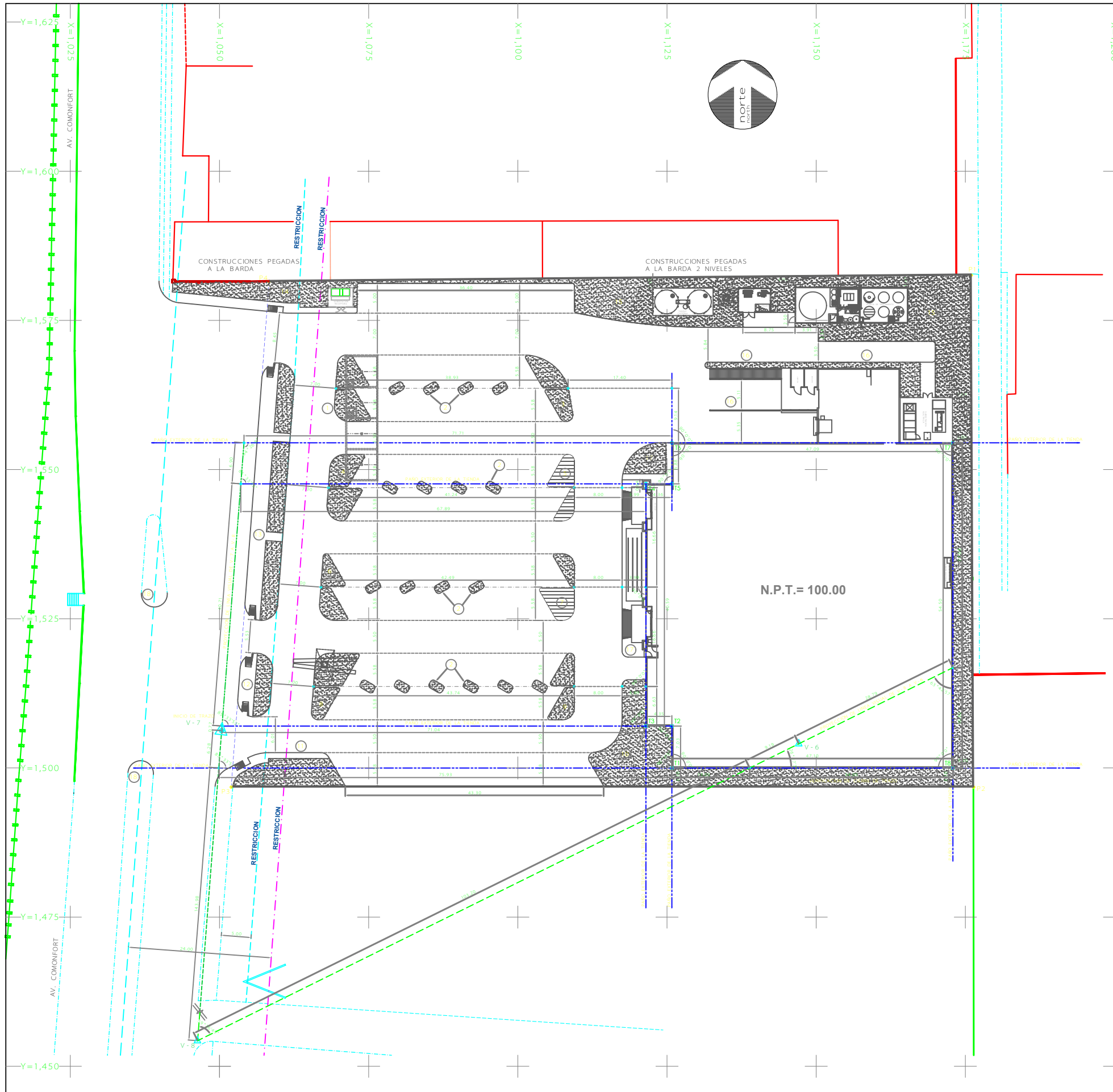
D-1 PLANTA DE TRAZO ESC. 1:250
