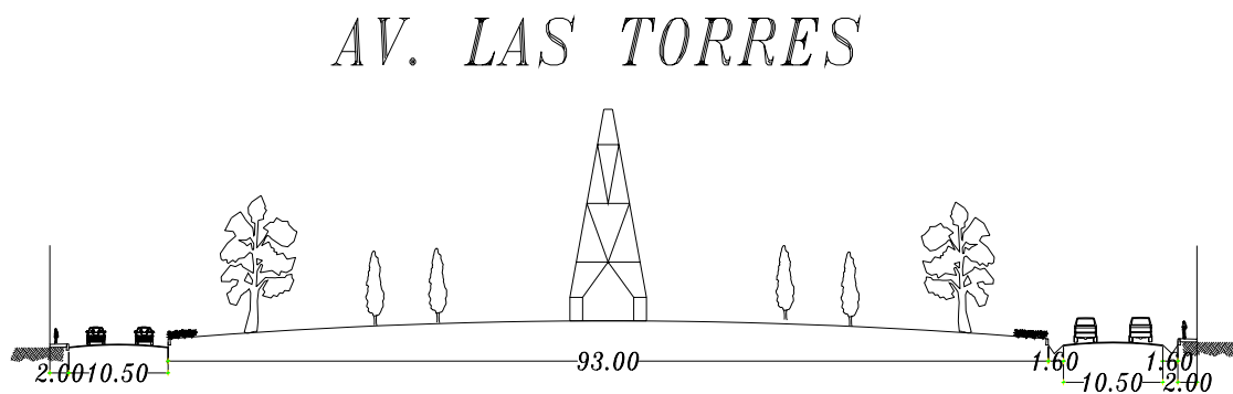
Figura II.4.5 Corte transversal de la Av. Las Torres.
