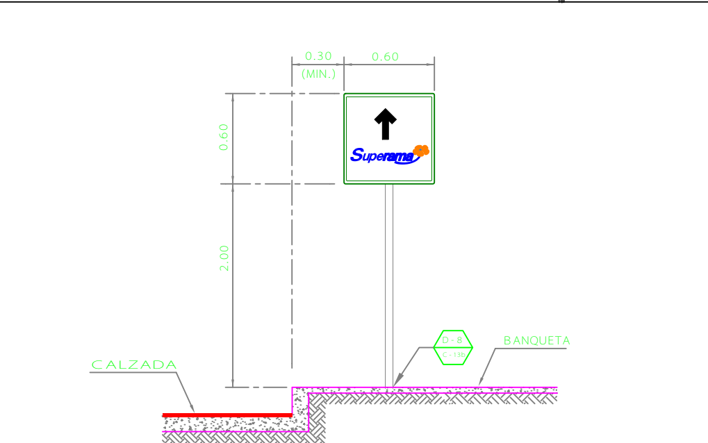
D-3 UBICACION LATERAL DE LETREROS (EN CANDELEROS) Y SEÑAL RESTRICTIVA SIN ESC. REF.: D-1 / C-13b
