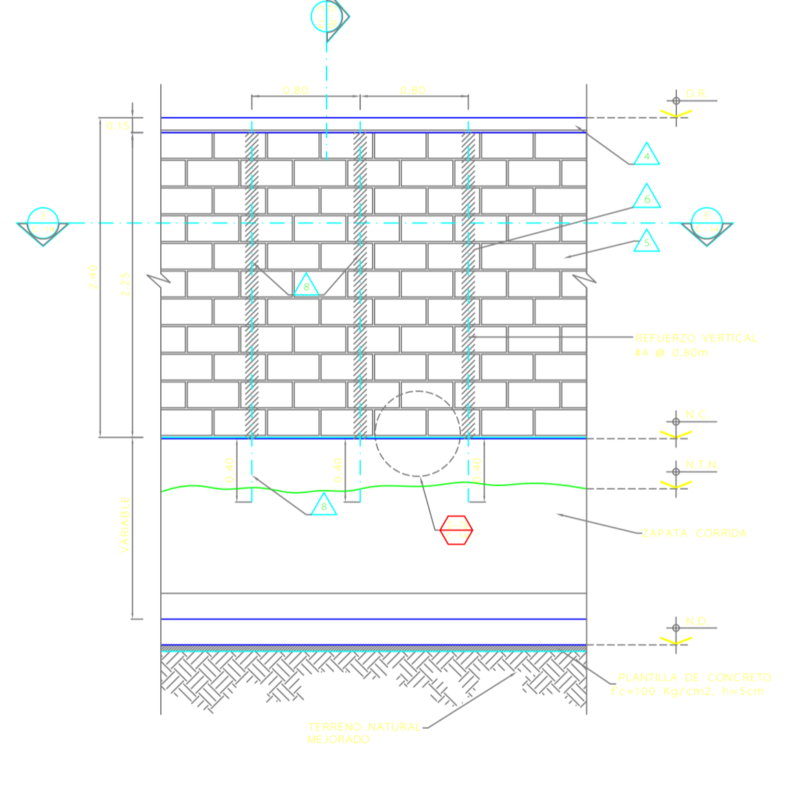
D-7 MURO DE LINDERO (MURO DE BLOCK), EN COUNDANCIA
