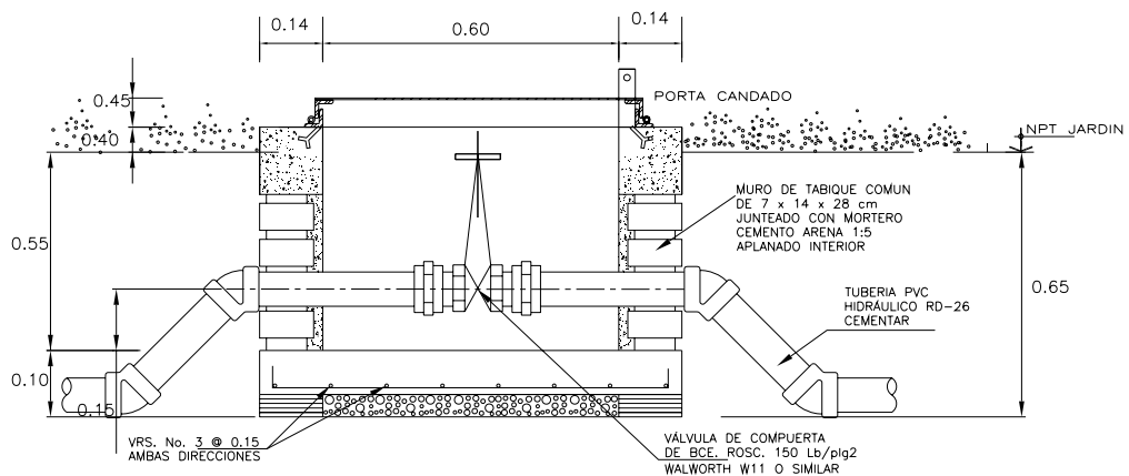
Figura III.7.1.1 Registro de válvulas de red de riego.
