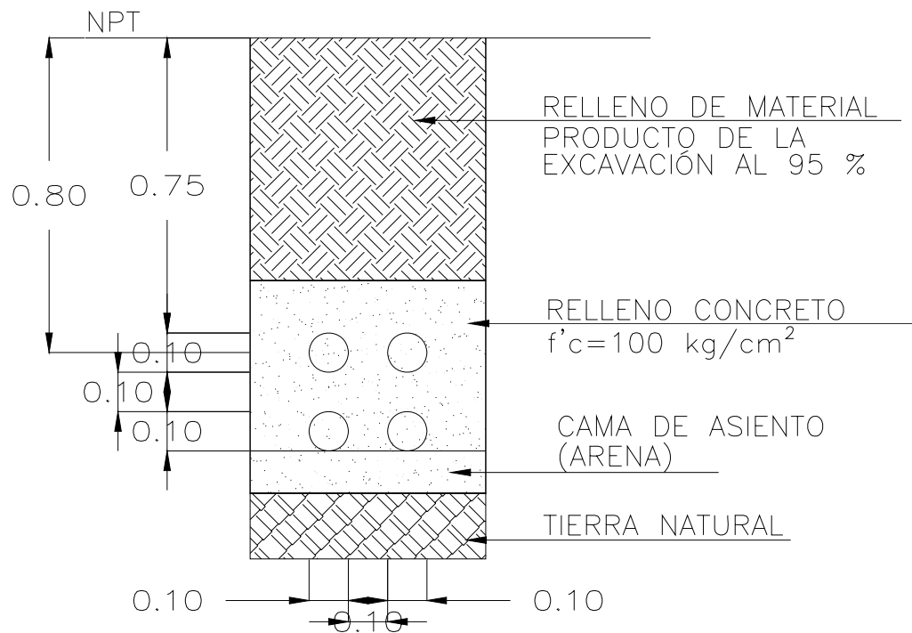
Figura III.5.2.1 Zanja en trancito pesado.
