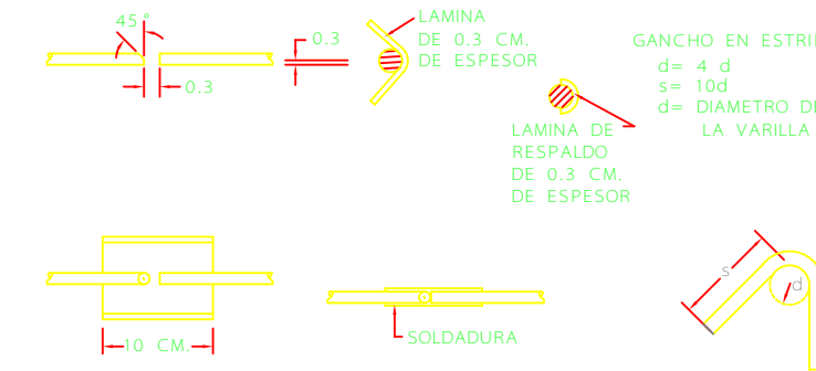
D-5 DETALLES DE REFUERZO
