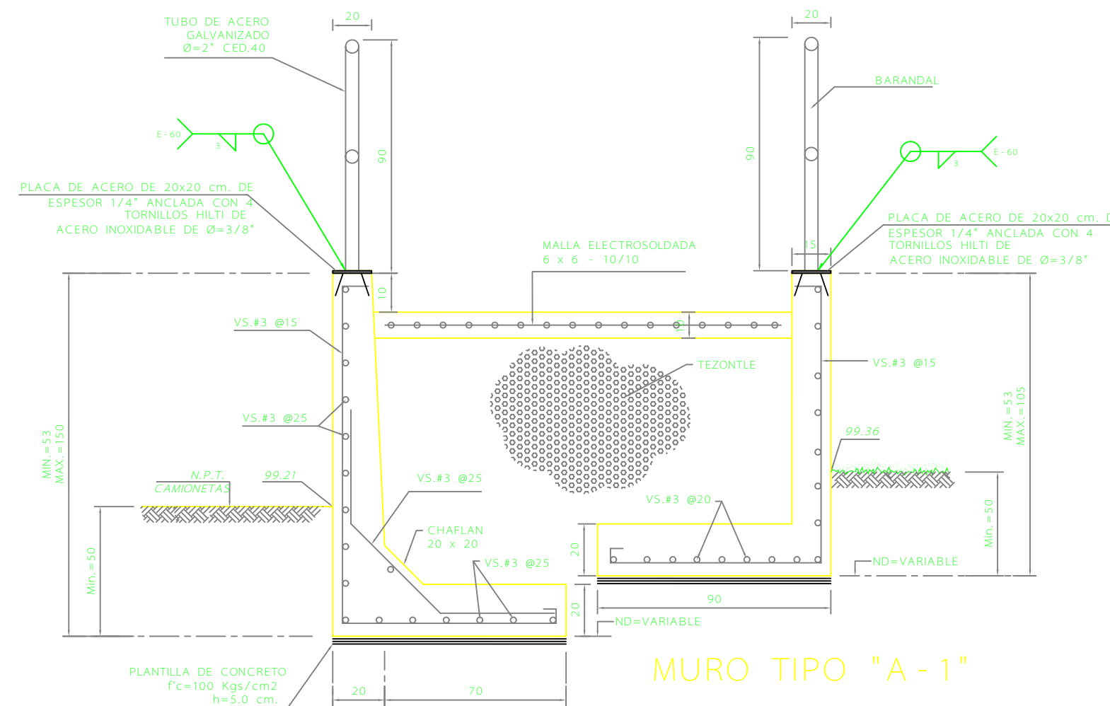
MURO TIPO "A-1"
