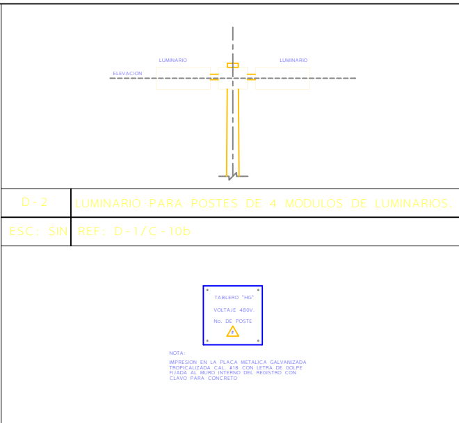
D-3 PLACA METALICA DE 0.10x0.10m. CON LEYENDA DESCRIPTIVA. ESC: SIN REF: D-4/C-10b
