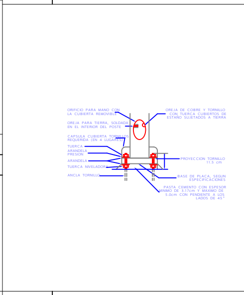
D-12 FIJACION DE ANCLAS. ESC: SIN REF: D-4/C-10b
