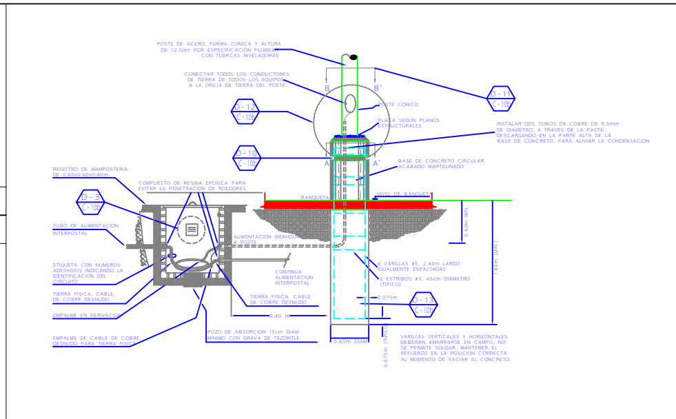
D-4 CIMIENTACION TIPICA POSTES DE ILUMINACION ESTACIONAMIENTO Y CONEXION A REGISTRO. ESC: SIN REF: D-1/C-10b
