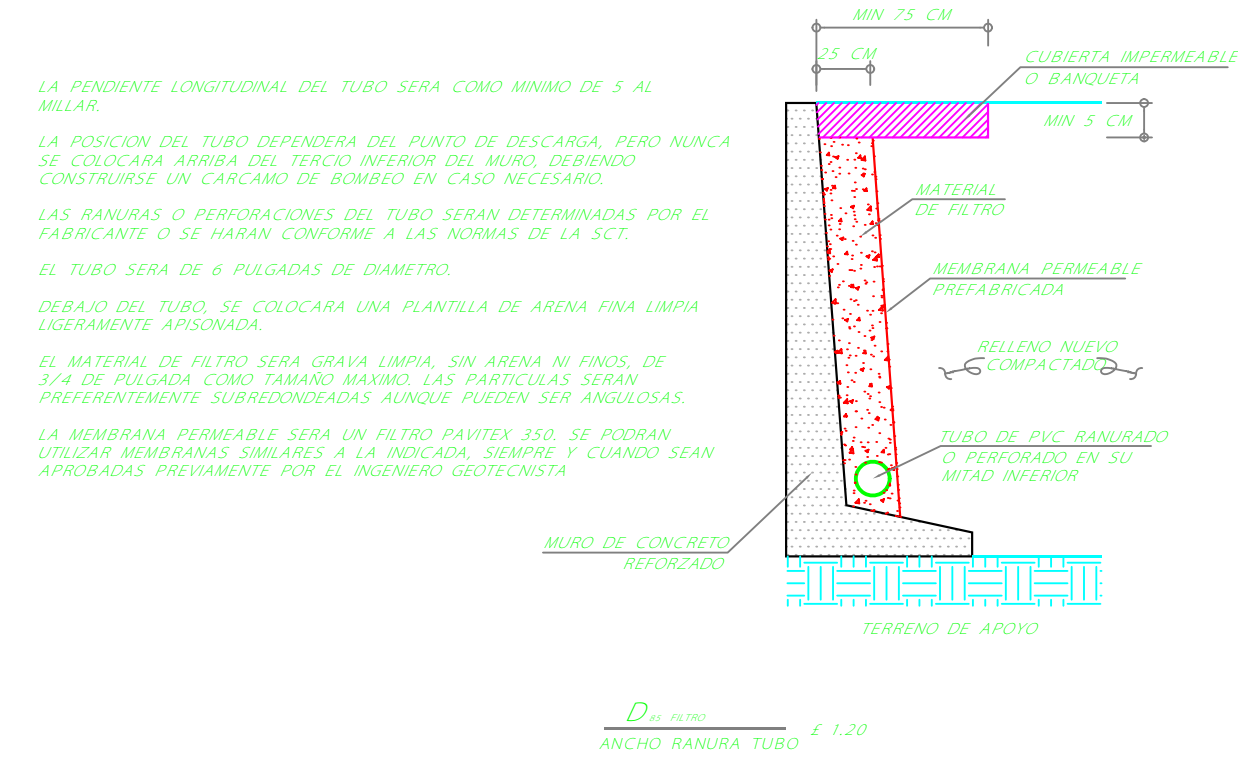
D-3 SISTEMA DE DRENAJE PARA MUROS DE RETENCION
