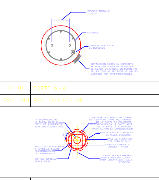
D-11 CORTE B-B' FIJACION DE PLACA DE BASE. ESC: SIN REF: D-4/C-10b
