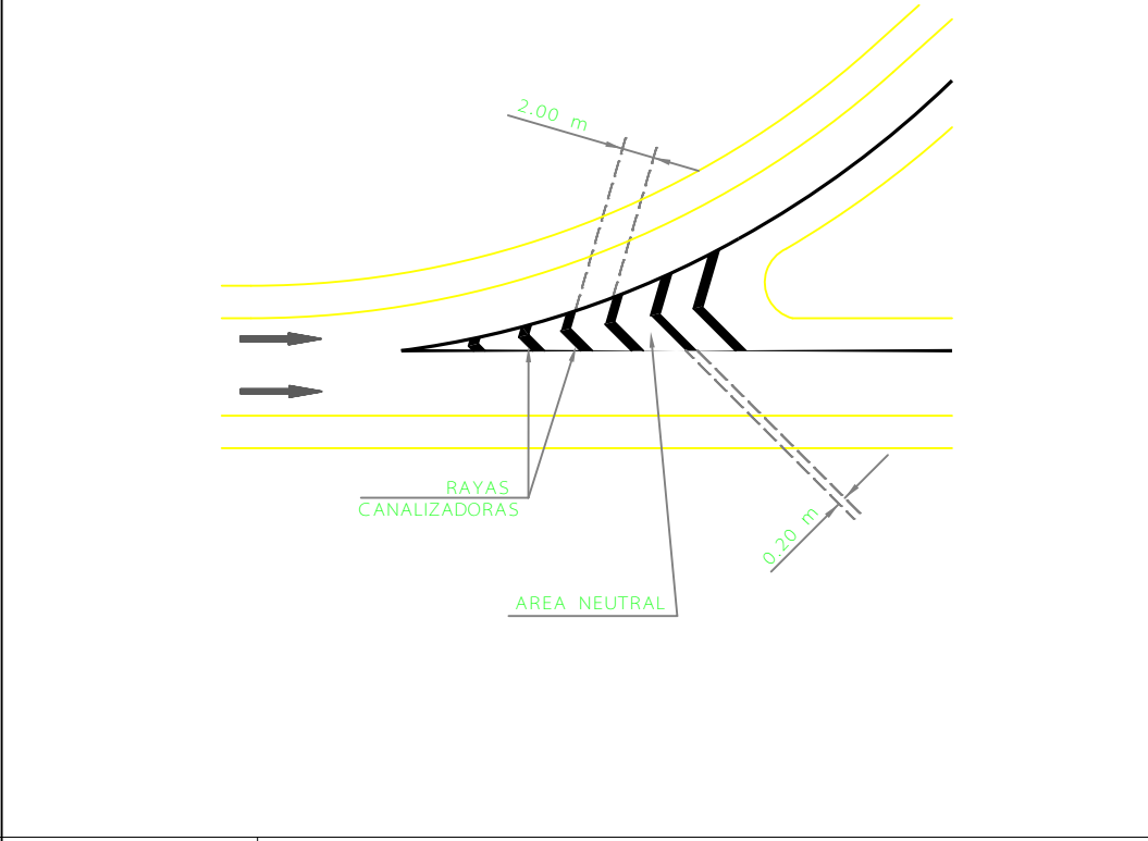
D-6 RAYAS CANALIZADORAS TIPO
