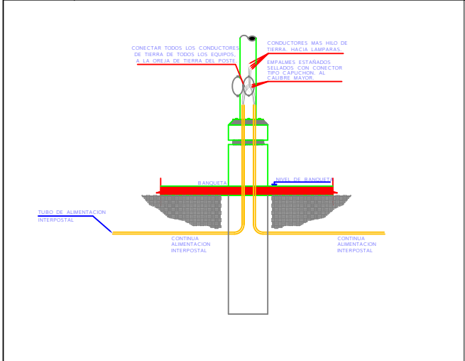
D-5 CIMIENTACION TIPICA DE POSTES DE ILUMINACION ESTACIONAMIENTO Y CONEXION SIN REGISTRO. ESC: SIN REF: D-1/C-10b
