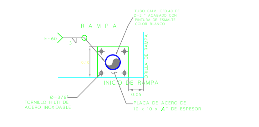
D-12 PLACA DE BARANDAL
