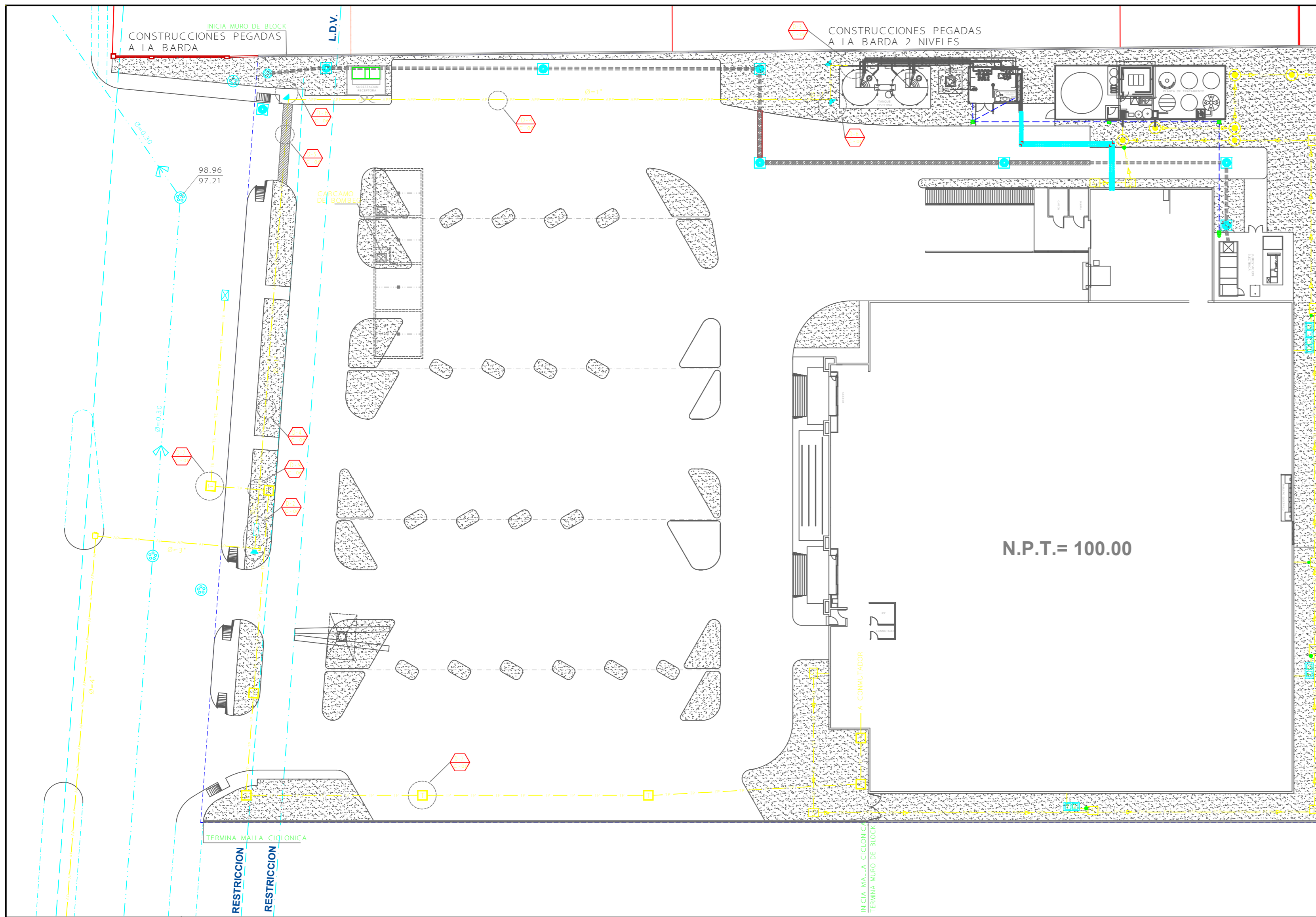
D-1 PLANO DE SERVICIOS GENERALES ESC. 1:250 D-1/C-03
