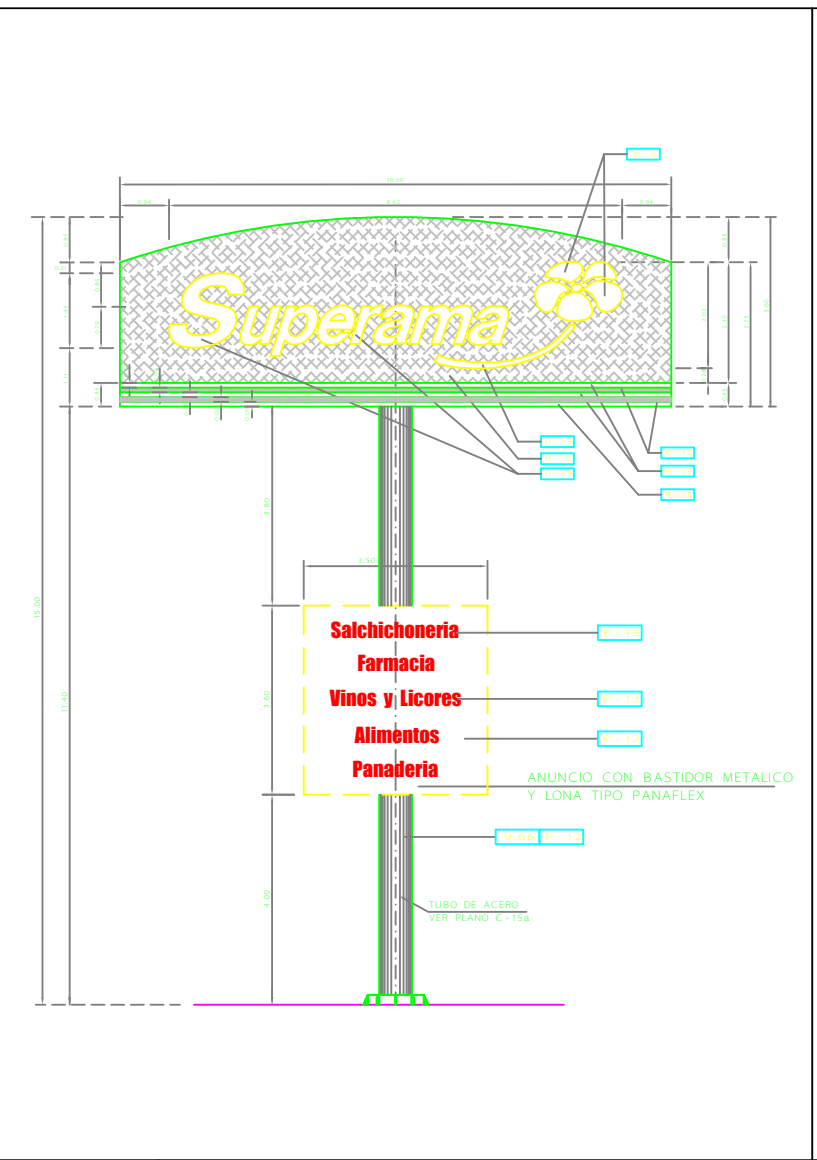
D-2 ANUNCIO ESPECTACULAR (ALZADO FRONTAL) ESC. 1:50 REF.: D-1/C-15
