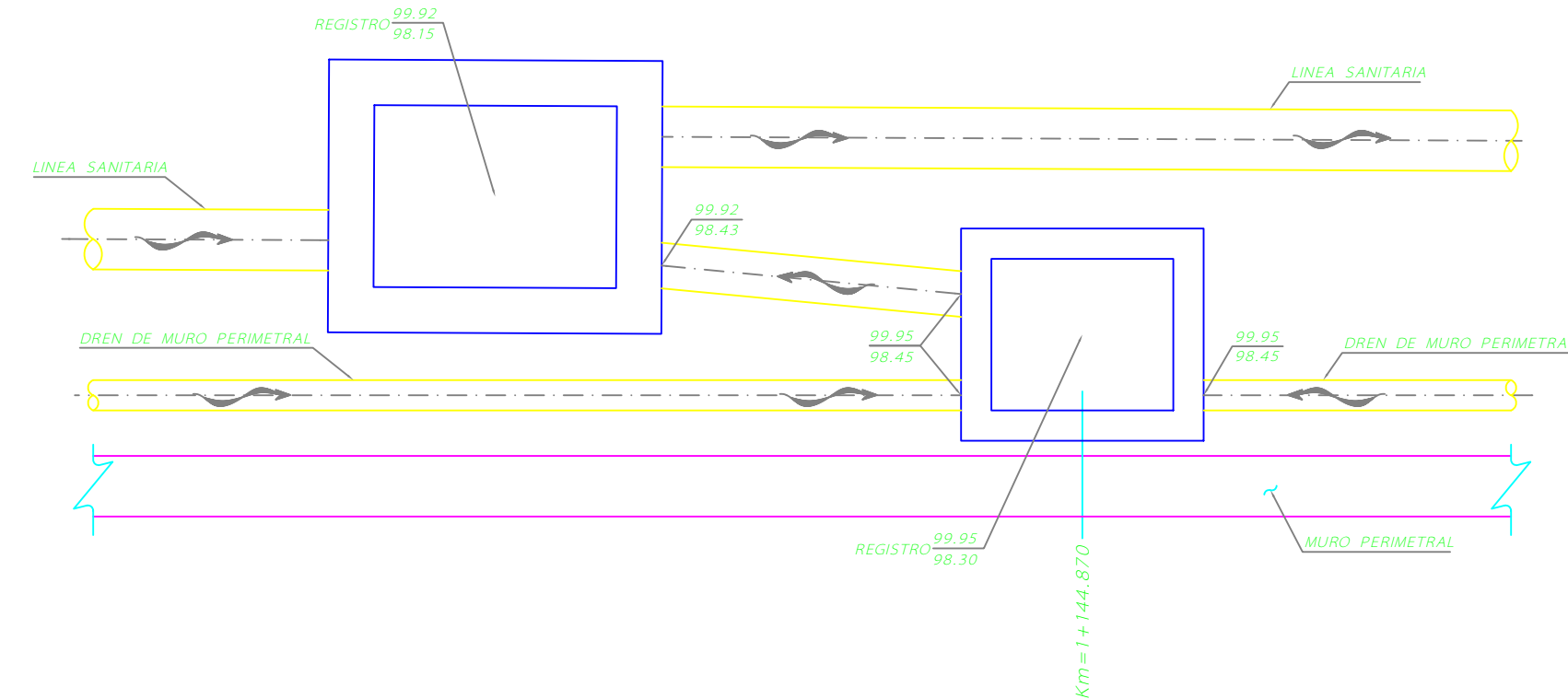
D-2 CONEXION: SANITARIA - DREN DE MURO
