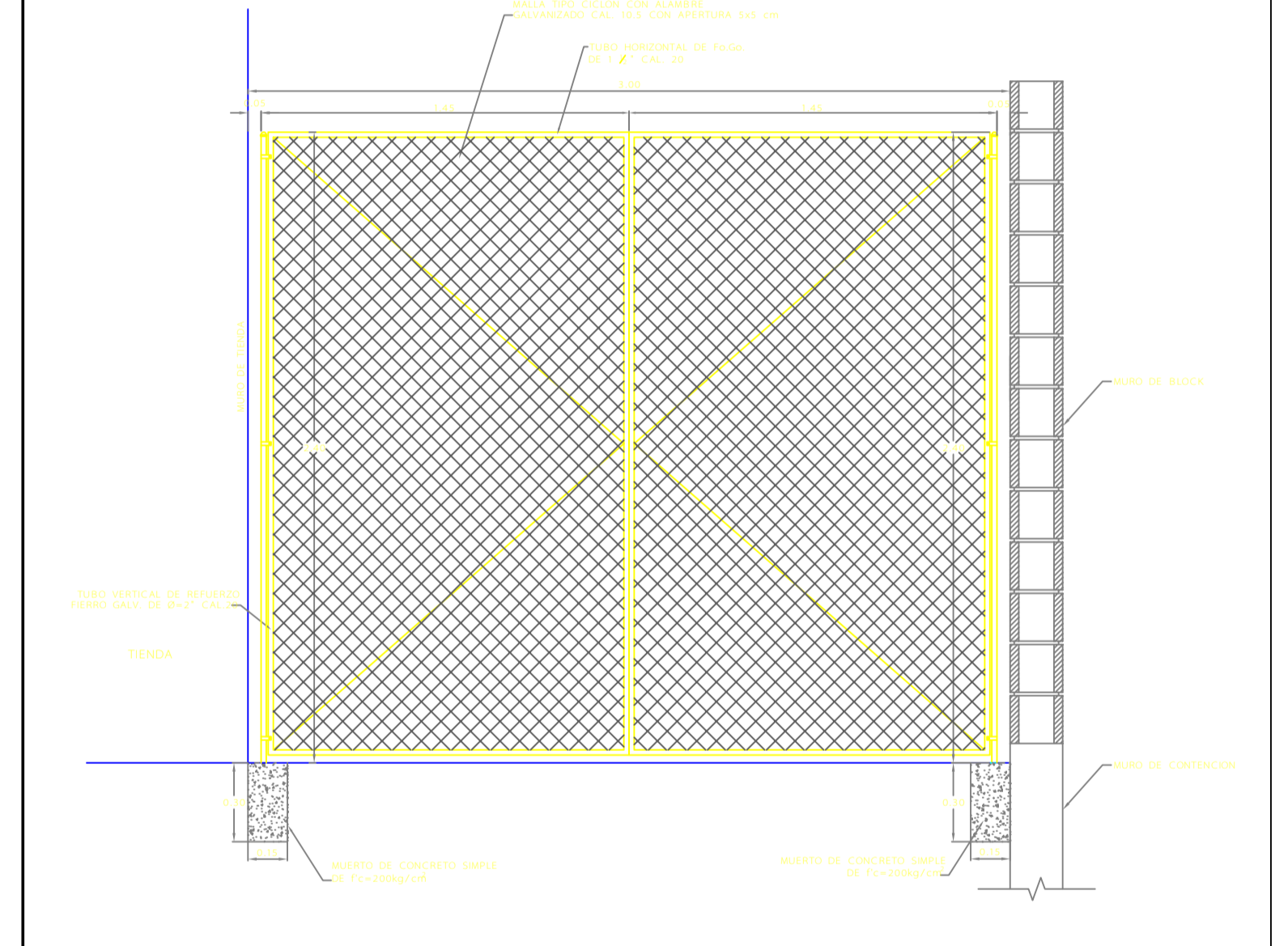
D-5 PUERTA DE MALLA CICLONICA EN LIMITE DE TIENDA CON ESTACIONAMIENTO DE 2.40 m DE ALTURA
