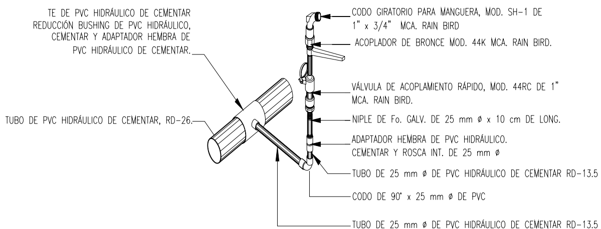
Figura. II.5.3 Detalle típico de válvulas de riego.
