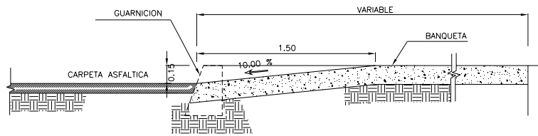
CORTE 2-2''
