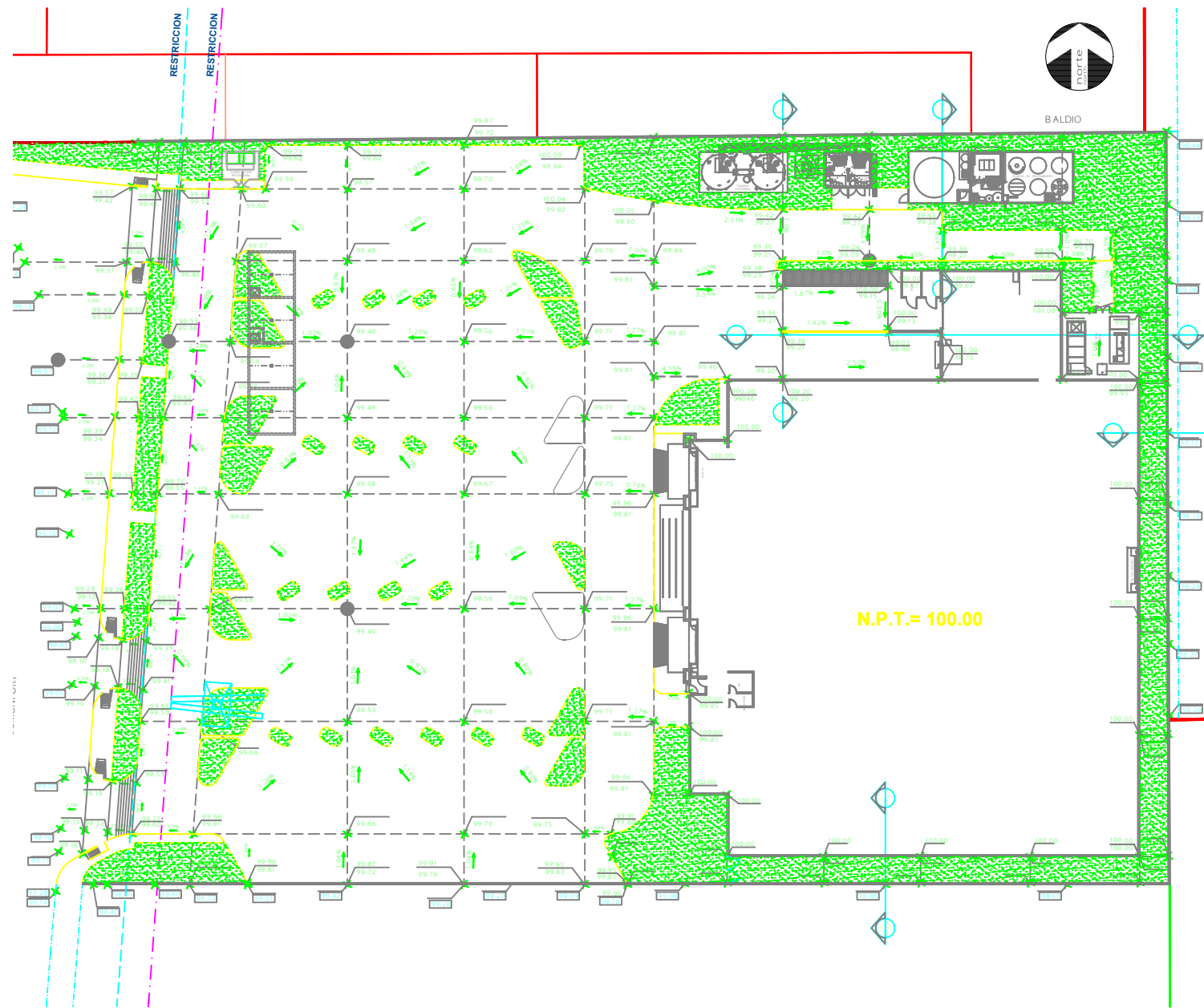
D-1 PLANTA DE NIVELES ESC. 1:250 D-1/C-03
