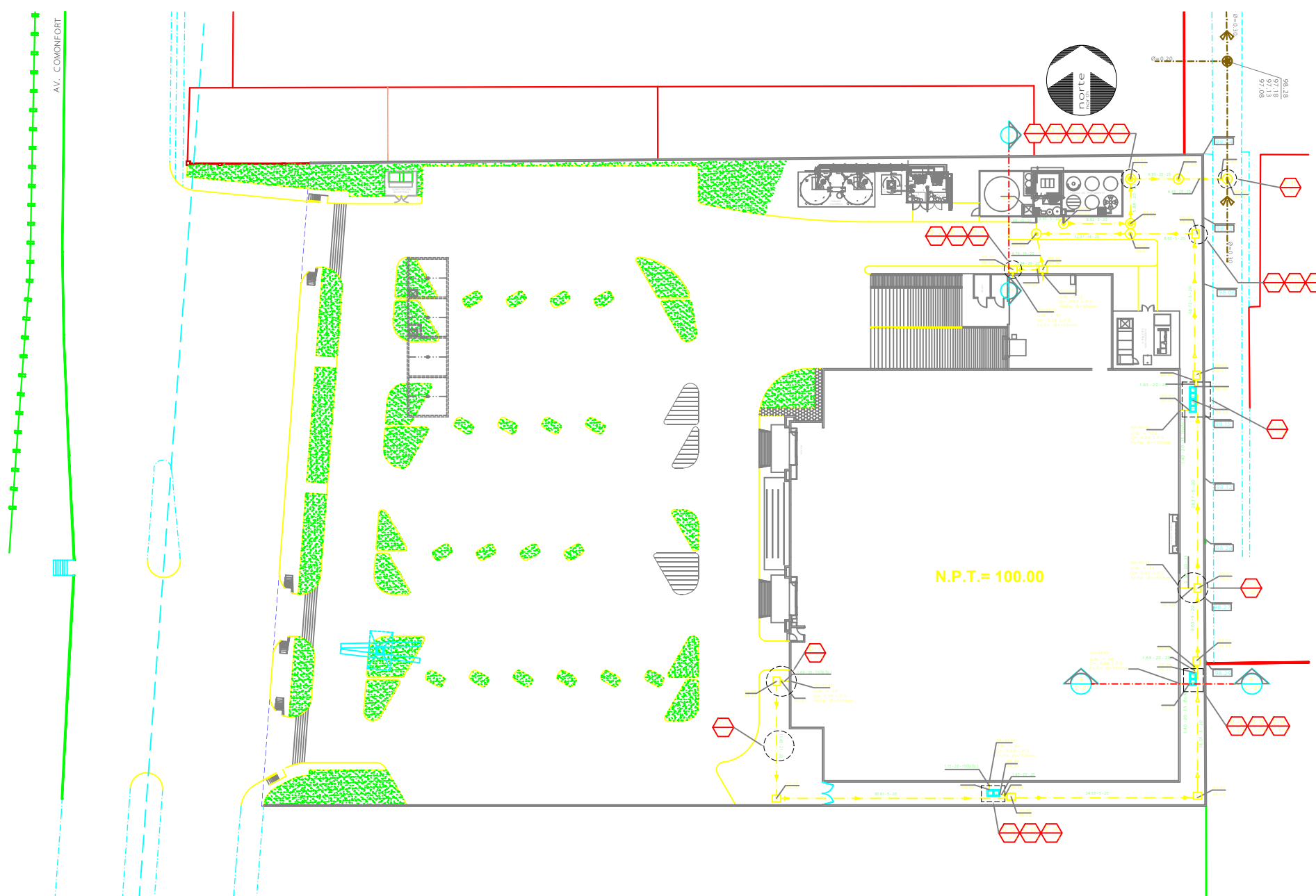
D-1 PLANTA DE DRENAJE SANITARIO ESC. 1:250 D-1/C-03
