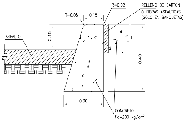
GUARNICIÓN TIPO 1 (TRAPEZOIDAL)
