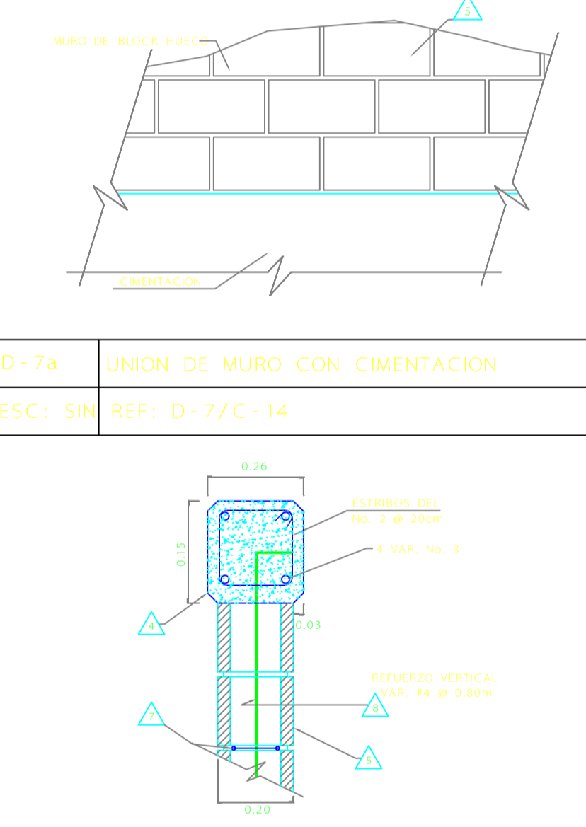
D-7b DALA DE CERRAMIENTO EN MURO BLOCK
