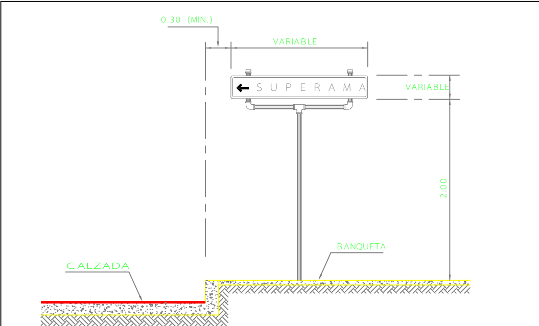
D-2 UBICACION LATERAL DE LETREROS (EN CANDELEROS) EN ZONA URBANA SIN ESC. REF.: D-1 / C-13b
