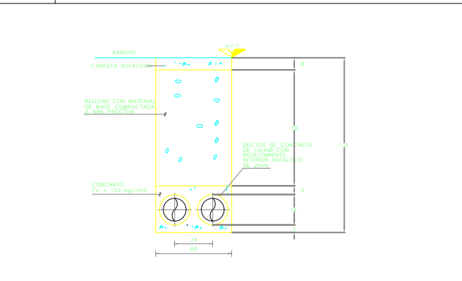
D-4 COLOCACION DE DUCTOS DE ARROYO ESC. S/N REF.: D-1/C-13c ACOT. EN cm
