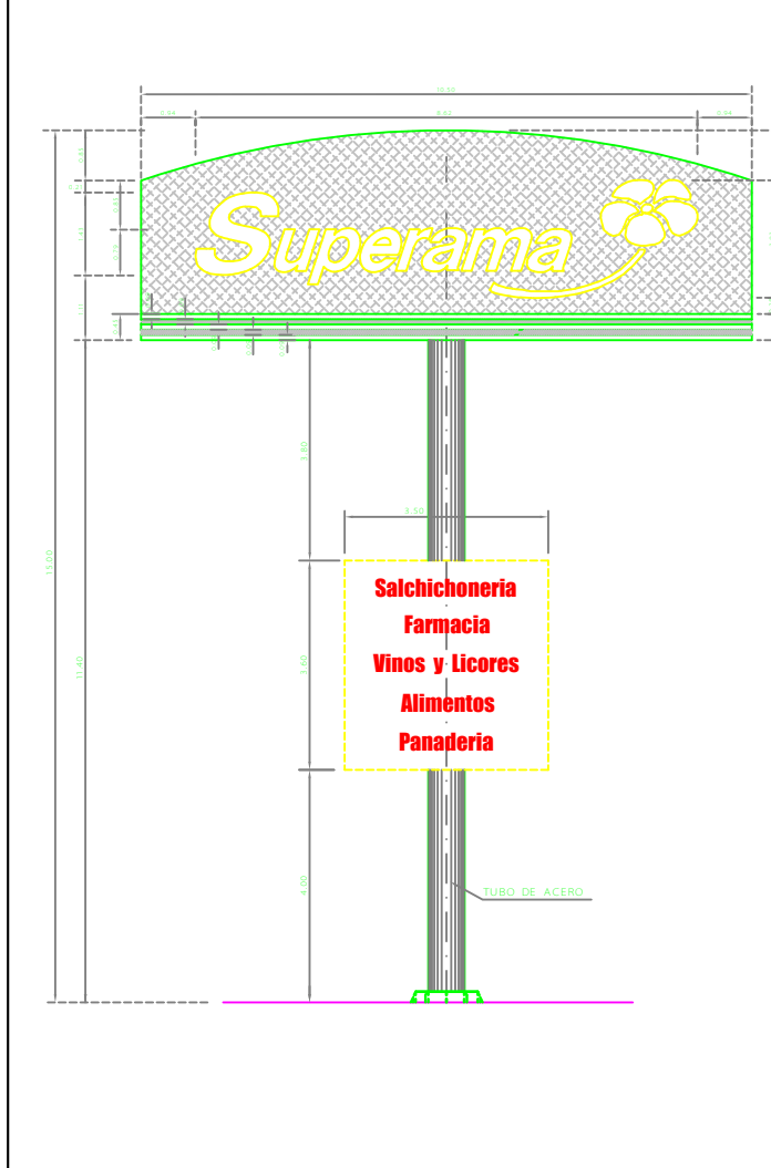
D-5 ANUNCIO ESPECTACULAR (ALZADO FRONTAL) ESC. SIN REF: D-1/C-15
