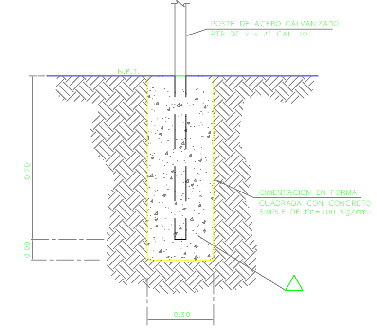
D-8 BASE PARA SEÑALAMIENTO EN EXTERIOR DE TIENDA SIN ESC. REF.: D-5 / C-13b
