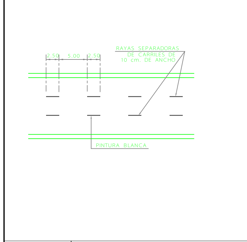
D-1 PLANTA DE SEÑALIZACION ESC. 1:250 REF.: D-1 / C-03
