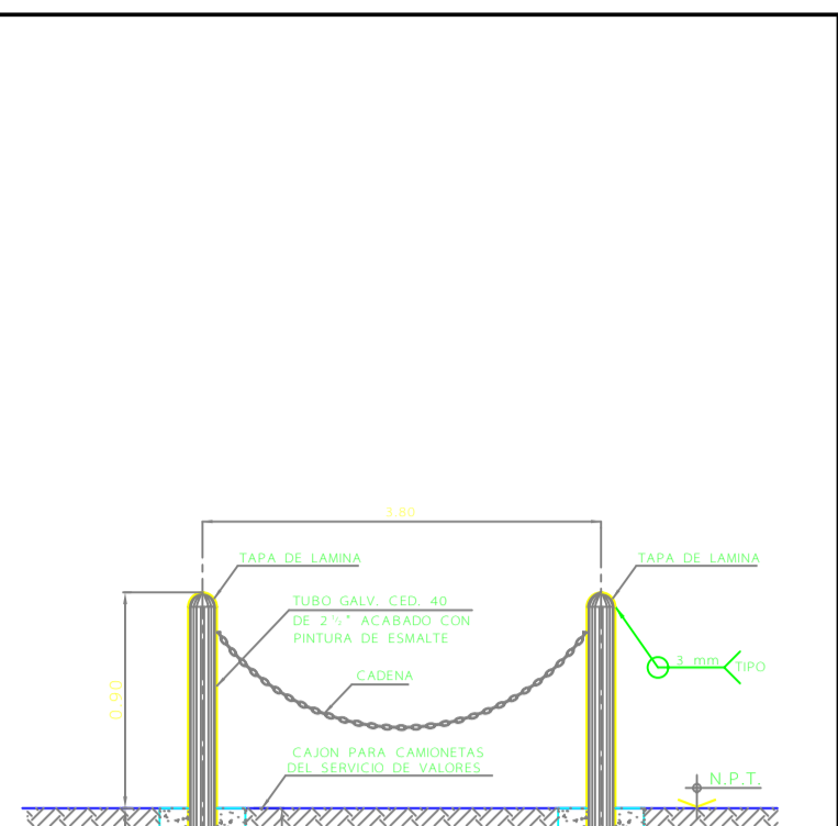
D-2 PROTECCION EN ZONA DE CAMIONETA DE VALDRE
