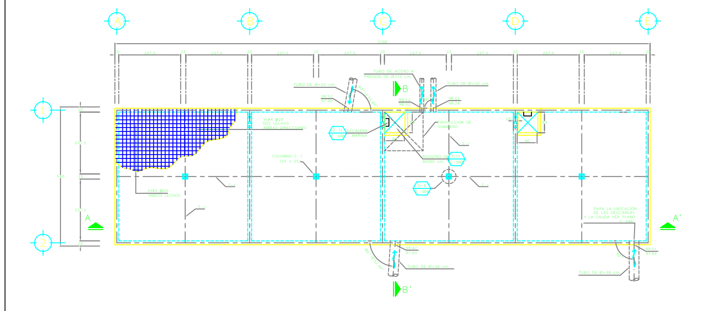
D-2 PLANTA TANQUE DE TORMENTAS (LOSA DE TAPA) SIN ESC. REF.: D-1/C-08
