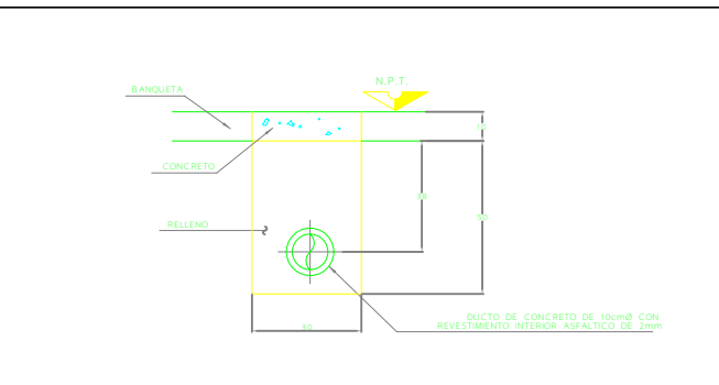
D-3 COLOCACION DE DUCTO EN BANQUETA ESC. S/N REF.: D-1/C-13c ACOT. EN cm
