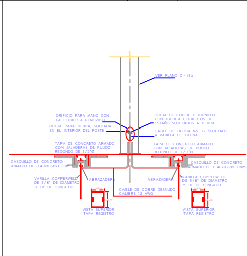
D-7 REGISTROS PARA ELECTRODO DE PUESTA A TIERRA EN ANUNCIO ESPECTACULAR ESC: SIN REF: D-1/C-10
