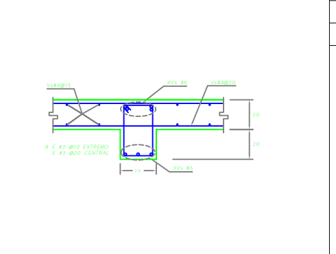
D-7 ARMADO DE T-1 (TRABE) SIN ESC. REF.: D-2/C-08b
