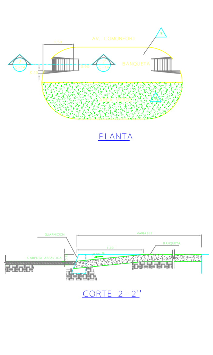
D-6 DETALLE TIPO PARA RAMPA DE DISCAPACITADOS
