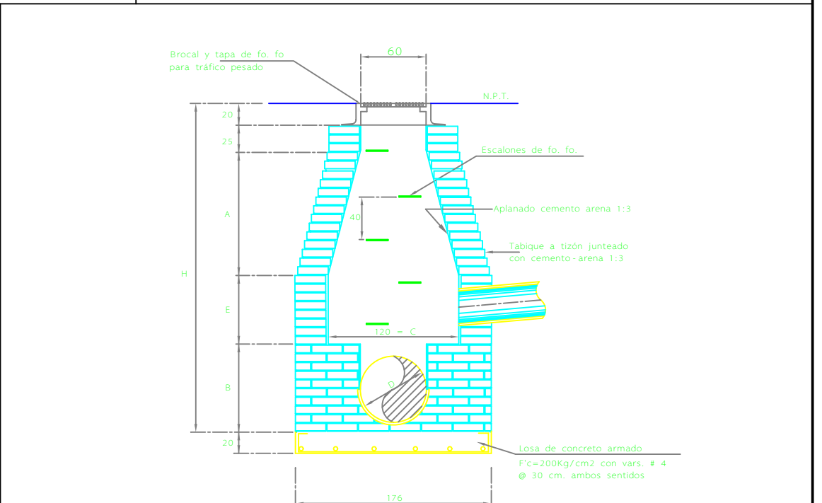
D-7 POZO DE VISITA TIPO COMUN CON CAIDA LIBRE PARA PROFUNDIDADES DE 1.50 A 2.50 METROS SIN ESC. REF: D-1/C-08
