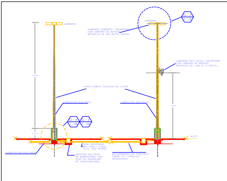
D-1 CONEXION DE REGISTRO A REGISTRO Y POSTE. ESC: SIN REF: D-1/C-10
