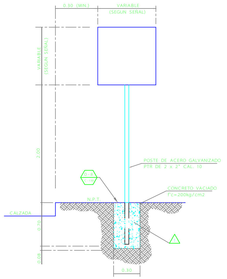
D-9 CIMENTACION DE SEÑAL DE UN POSTE SIN ESC. REF.: D-1 / C-13b
