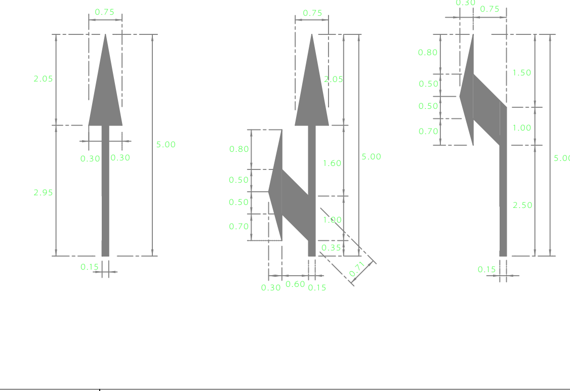
D-5 MODELO Y DIMENSION DE FLECHA EN PAVIMENTO PARA
