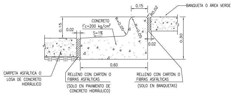
GUARNICIÓN TIPO 2 (PECHO DE PALOMA) PARA ISLETAS Y BANQUETAS
