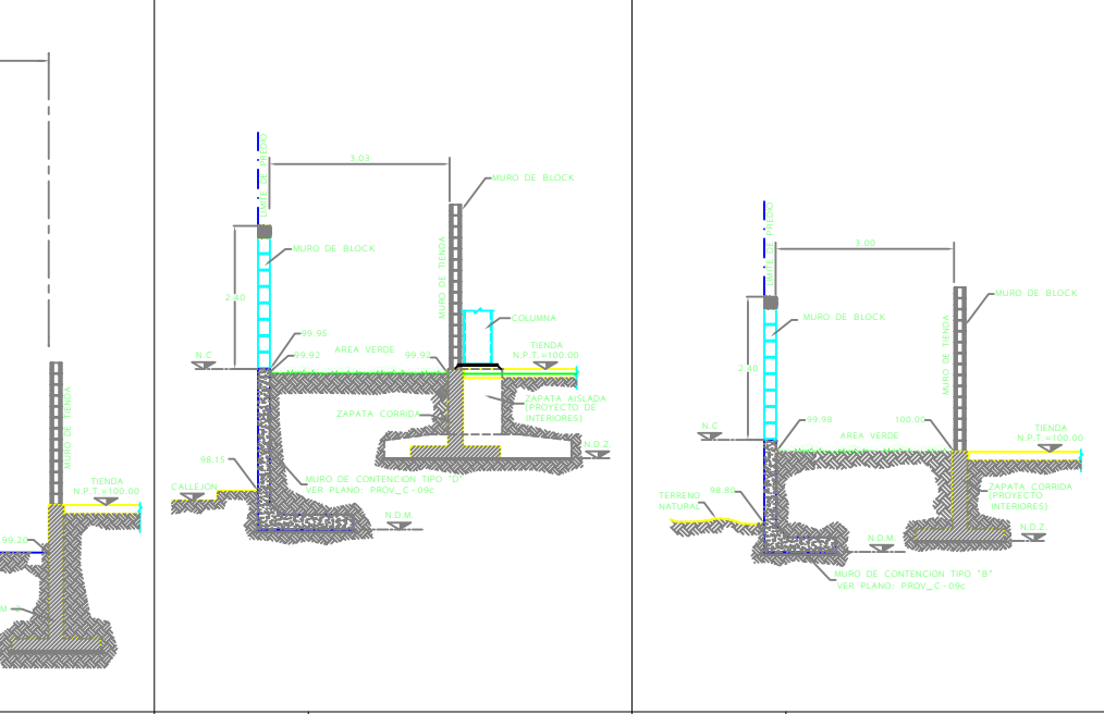
D-5 CORTE 4 - 4'
