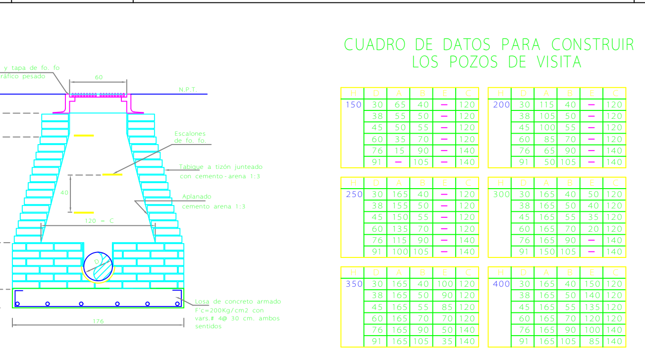
D-6 POZO DE VISITA TIPO COMUN PARA PROF. DE 1.5 A 2.5 m. SIN ESC. REF: D-1/C-08 Y D-4/C-08a
