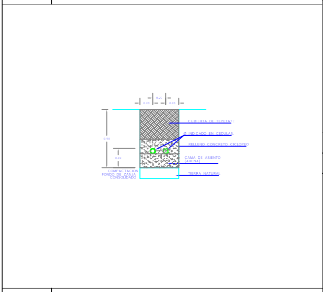
D-9 ZANJA PARA CONDUCTORES DE POSTES DE ALUMBRADO ESC: SIN REF: D-1/C-10
