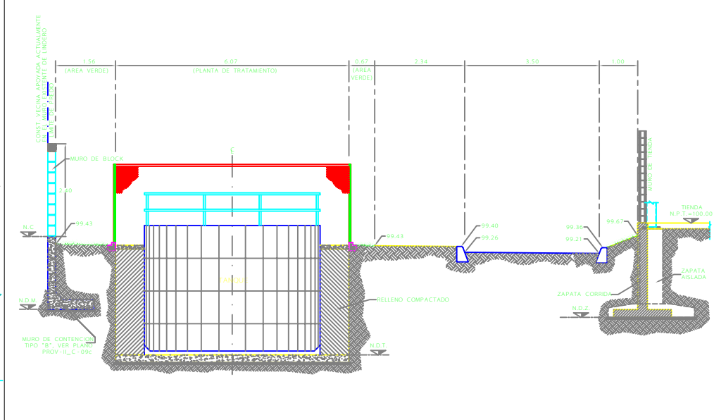
D-3 CORTE 2 - 2' ESC. 1:50 D-1/C-05
