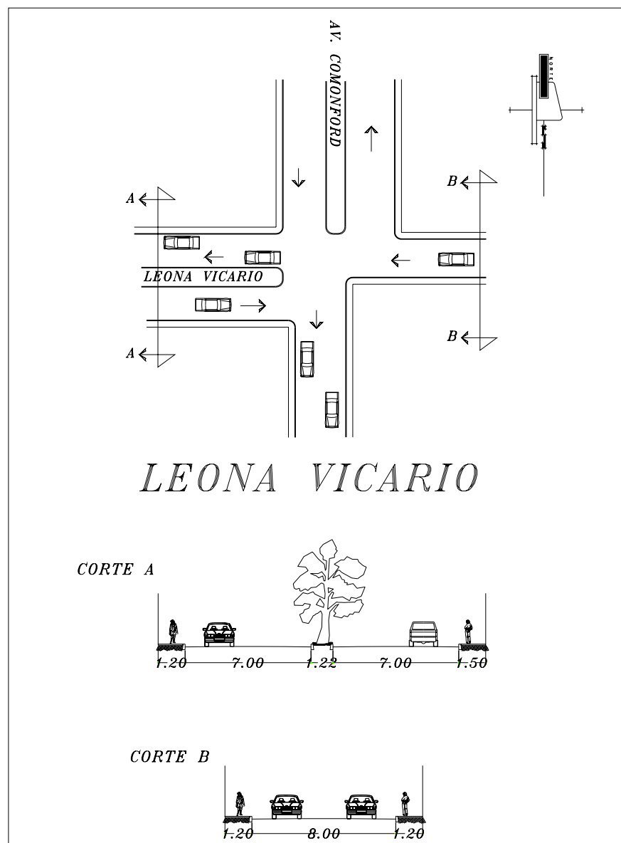
Figura II.4.3 Corte trasversal de la Av. Leona Vicario.
