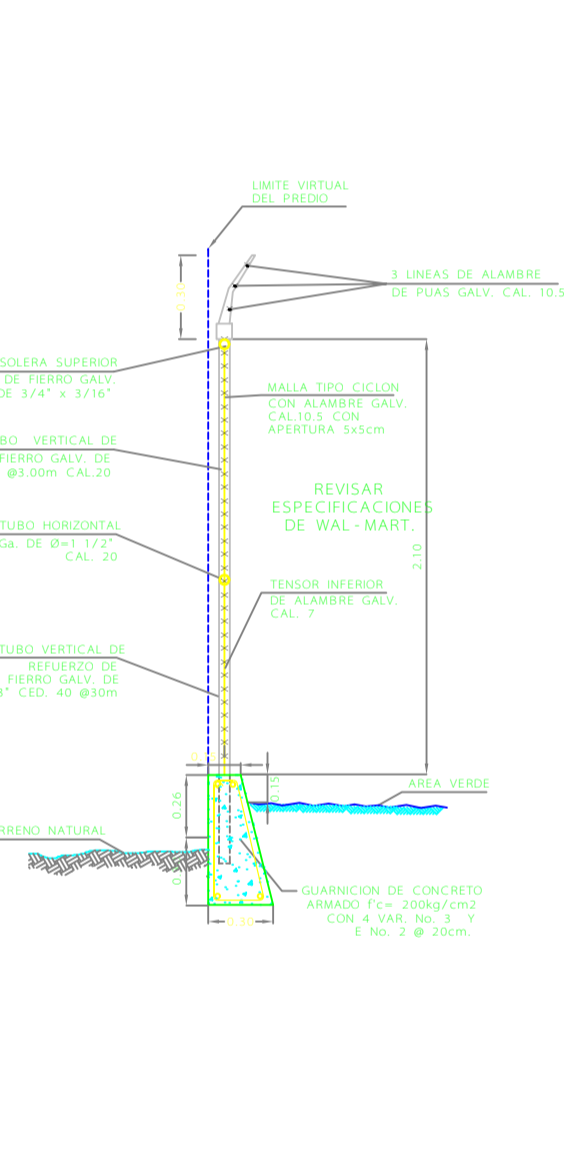
D-5a DETALLE DE MALLA CICLONICA
