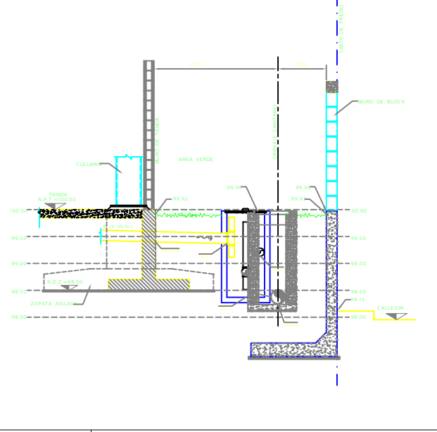
D-4 CORTE B - B'
