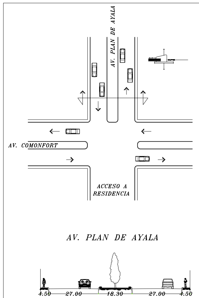
Figura II.4.2 Corte transversal de la Av. Plan de Ayala.
