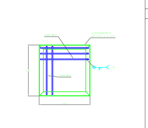
D-6 ARMADO DE TAPA SIN ESC. REF.: D-5/C-08b
