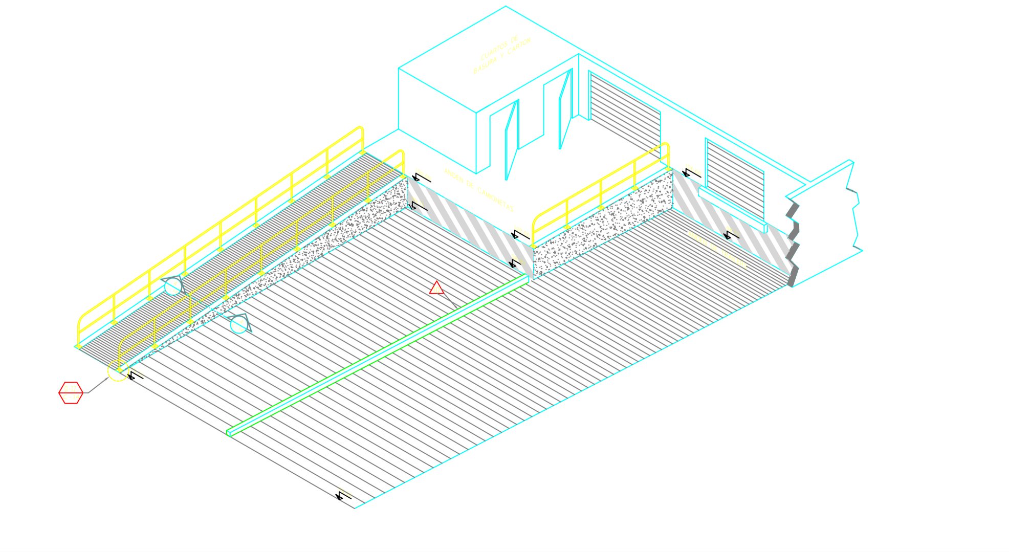
D-10 ISOMETRICO DEL PATIO DE MANIOBRAS
