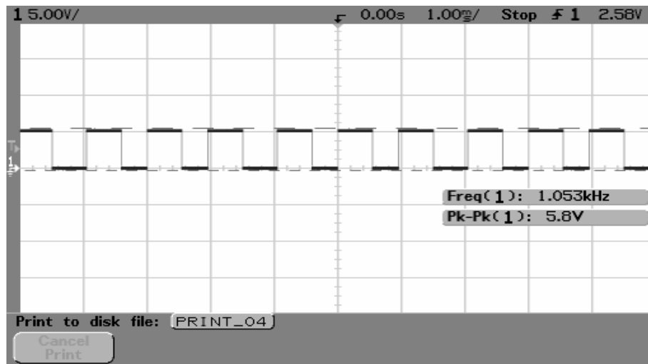
Figura 3.13. Oscilograma resultante al ser aplicadas las señales de la figura 3.12.
