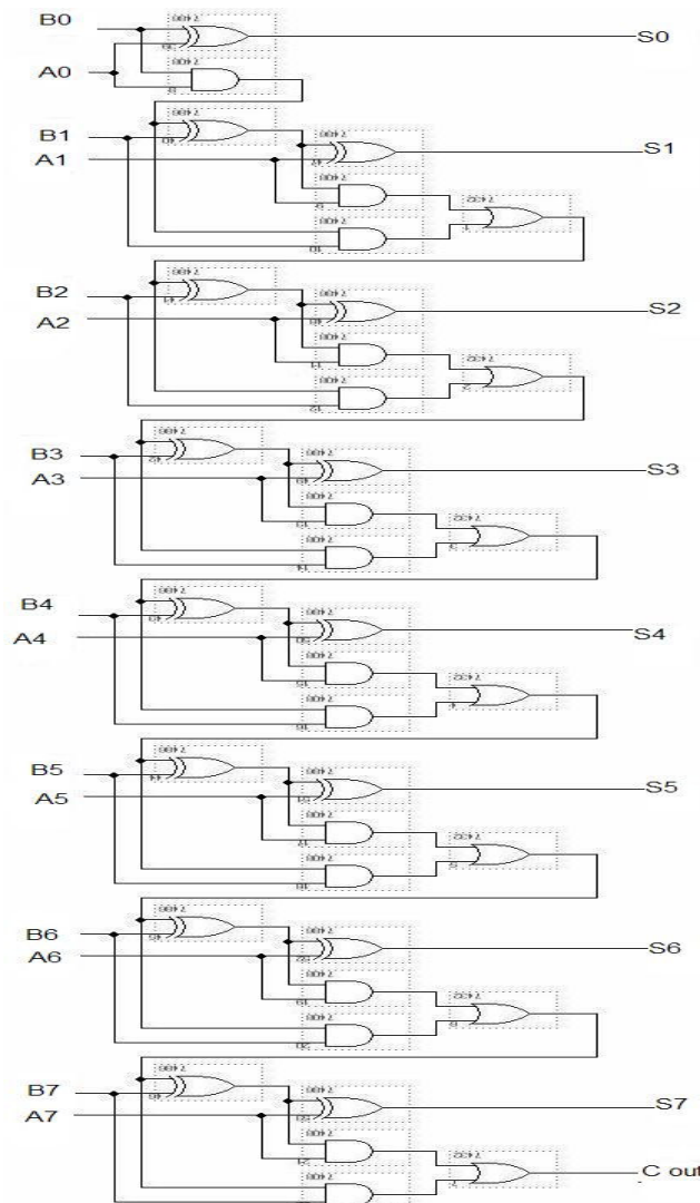
Figura 5.4. Circuito sumador de 8 bits.
