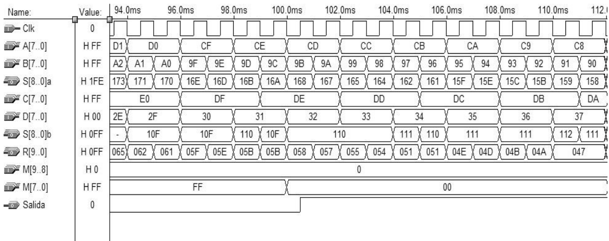
Figura 2.14b. Detalle de la operación del functor lógico para el periodo de 94 ms a 112 ms.
