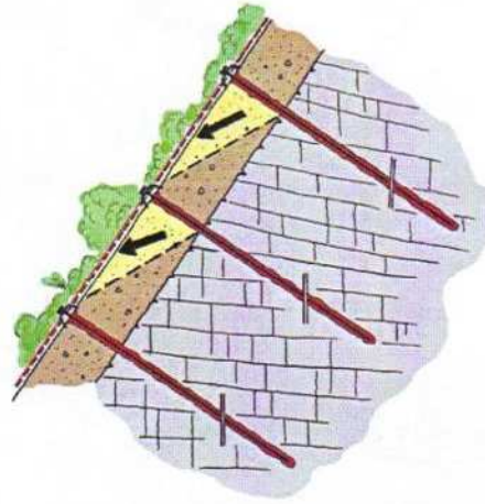
Inestabilidades locales entre anclajes
