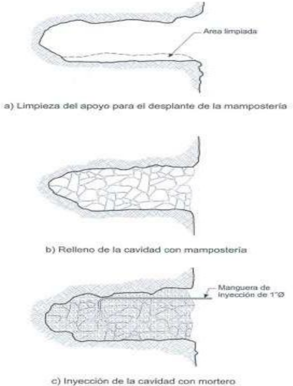
Figura 105. Relleno con mampostería de cavidades.
