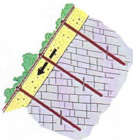
Inestabilidades superficiales paralelas al talud
