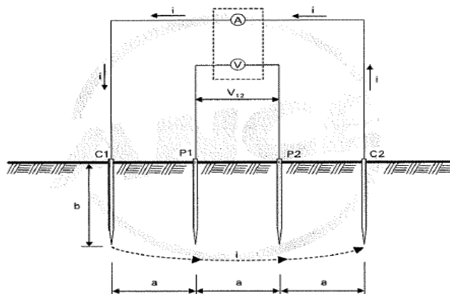
Ilustración 2. Método de conexión de los Cuatro Electrodos o Método de Wenner. Fuente: (NMX-J-549-ANCE-2005, 2005).
