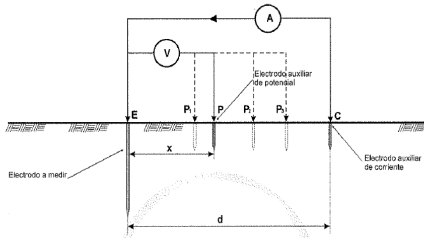
Ilustración 20. Método de caída de Tensión, Tomado de; NMX-J-549-ANCE-2005.
