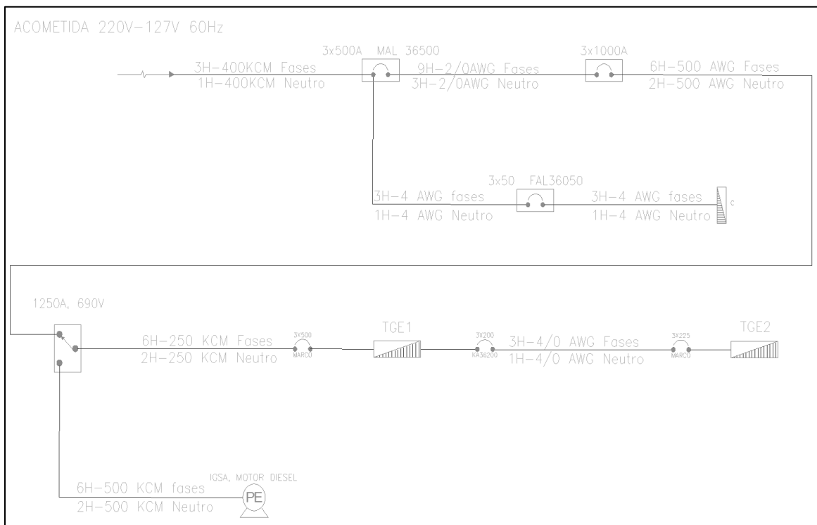
Ilustración 3. Diagrama Unifilar.
