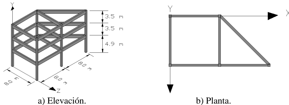
Figura 6.1 Estructura estudiada.
