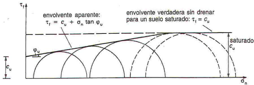
Figura 9 Esfuerzo total para resultados sin drenar
