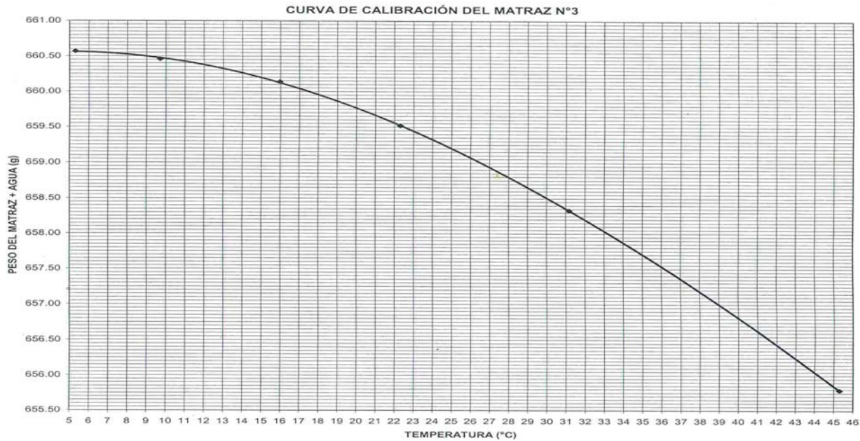
Gráfica 4 Curva de calibración del matraz 3 (Pozo1)
