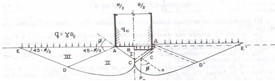
Figura 12 Mecanismo de falla de un cimiento continuo poco profundo según Terzaghi
