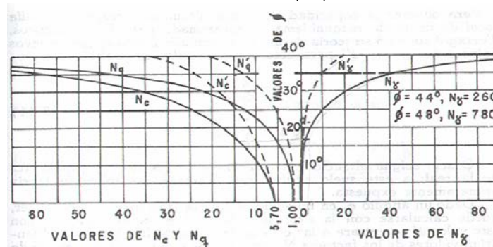
Figura 13 Factores de capacidad de carga
