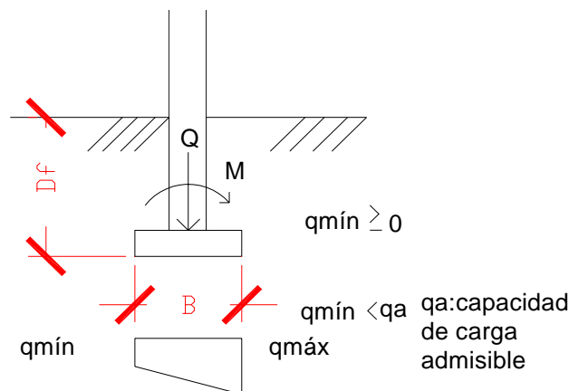
Figura 19 Zapata aislada
