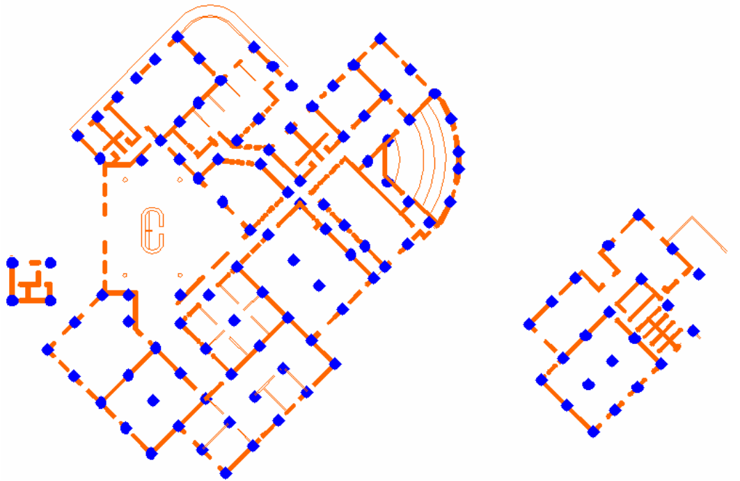
a) Estructura idealizada en planta del Centro Multidisciplinario
