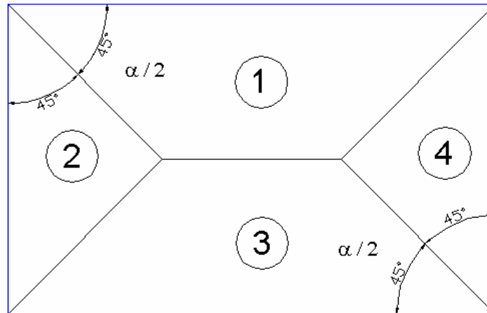
Figura 8 Procedimiento para dibujar áreas tributarias sobre traveses
