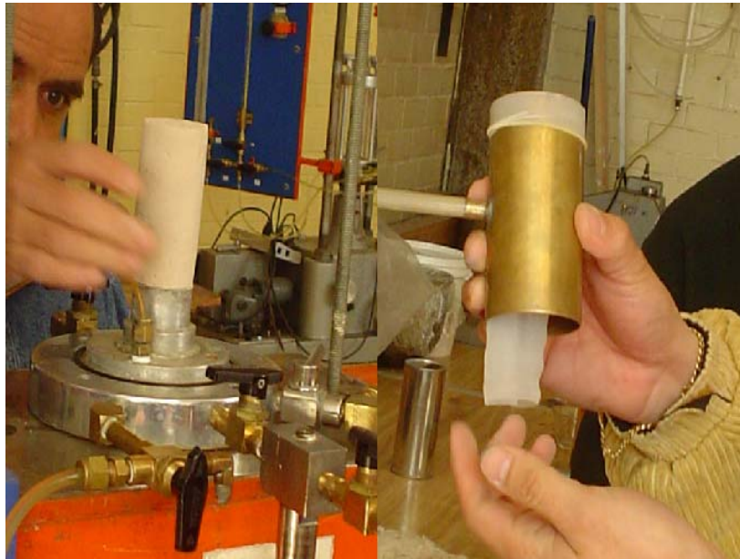
Fotografía 23 Colocación del espécimen y membrana
