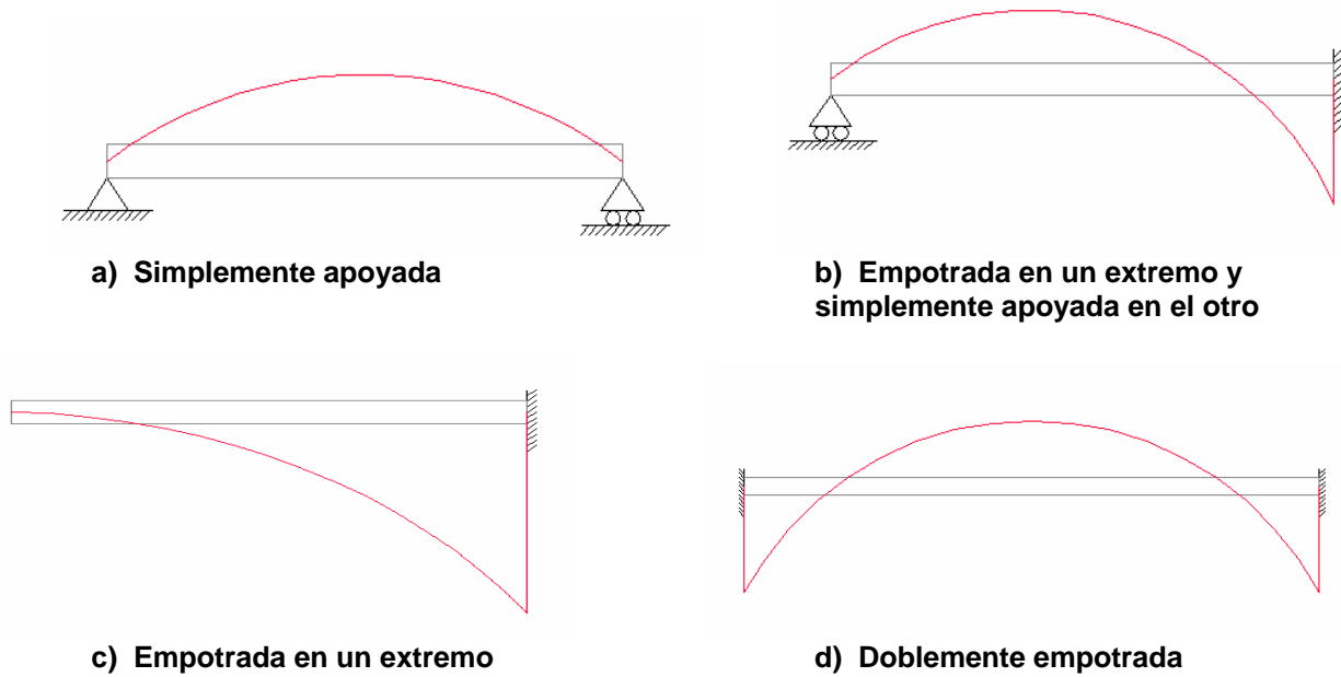
Figura 11 Comparativo de diagramas de momento flexionante
