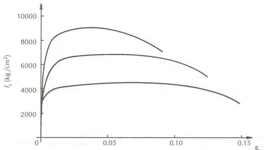
Figura 18 Curva esfuerzo-deformación de aceros laminados en frío
