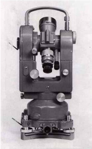
Figura 7 Teodolito universal Wild T2.
