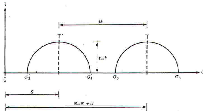
Figura 3 Representación del esfuerzo desviado
