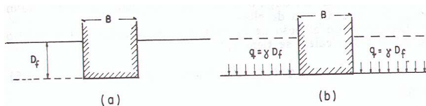
Figura 11 Equivalencia del suelo sobre el nivel de desplante de un cimiento con una sobrecarga debido a su peso
