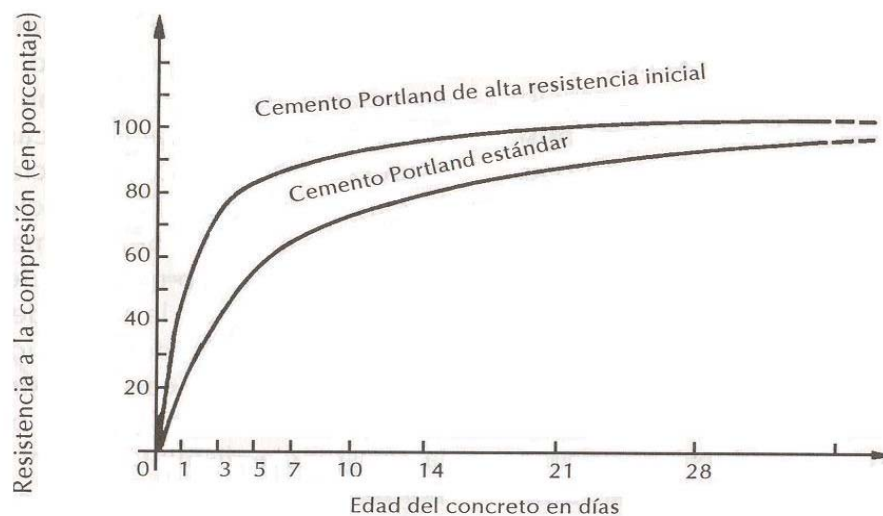
Figura 16 Variación de la resistencia con la edad y tipo de cemento
