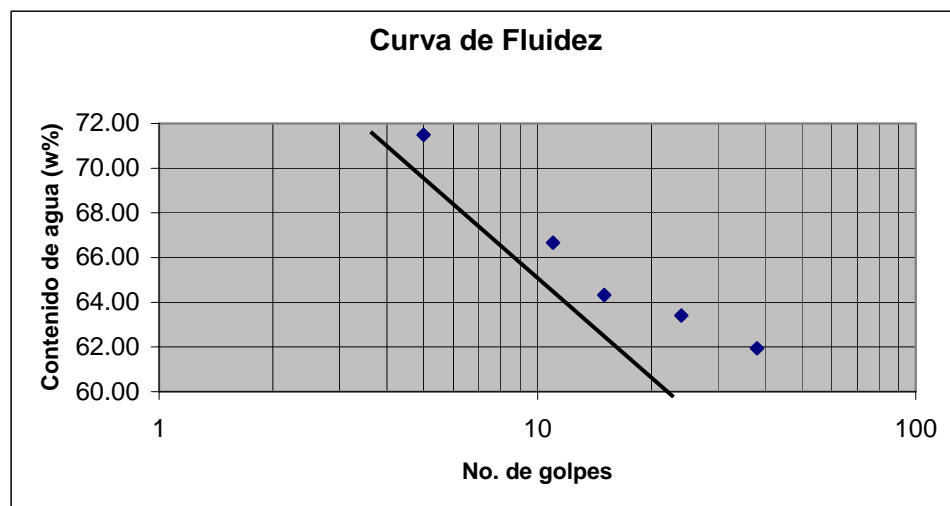
Gráfica 2 Curva de Fluidez del pozo 2
