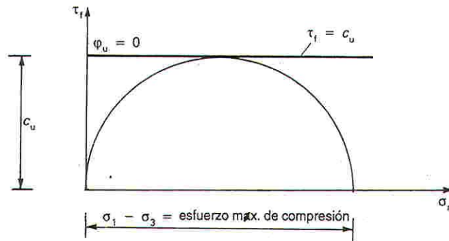
Figura 6 Prueba de compresión sin confinar
