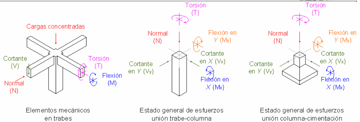
Figura 3 Fuerzas y acciones en los elementos estructurales
