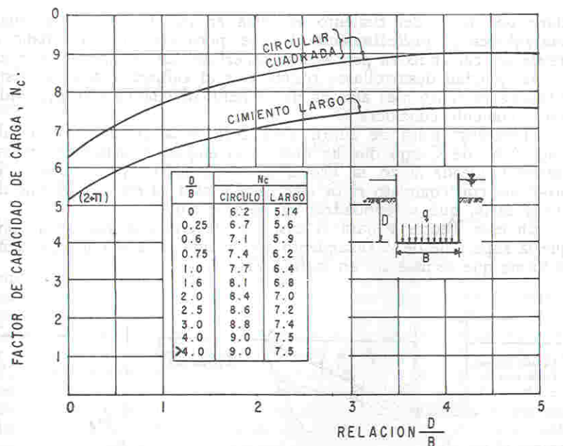
Figura 3 Valor de N_c para suelos cohesivos
