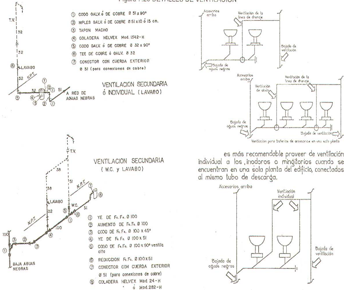
Figura 7.20 DETALLES DE VENTILACION
