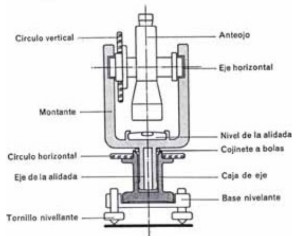
Figura 5 Representación esquemática de un teodolito.
