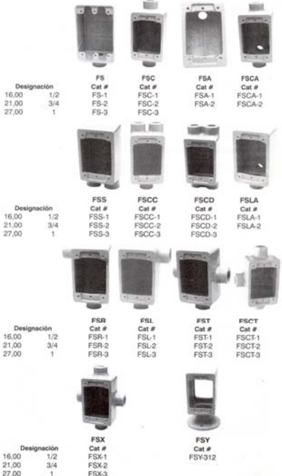
Figura 7 Cajas de conexión
