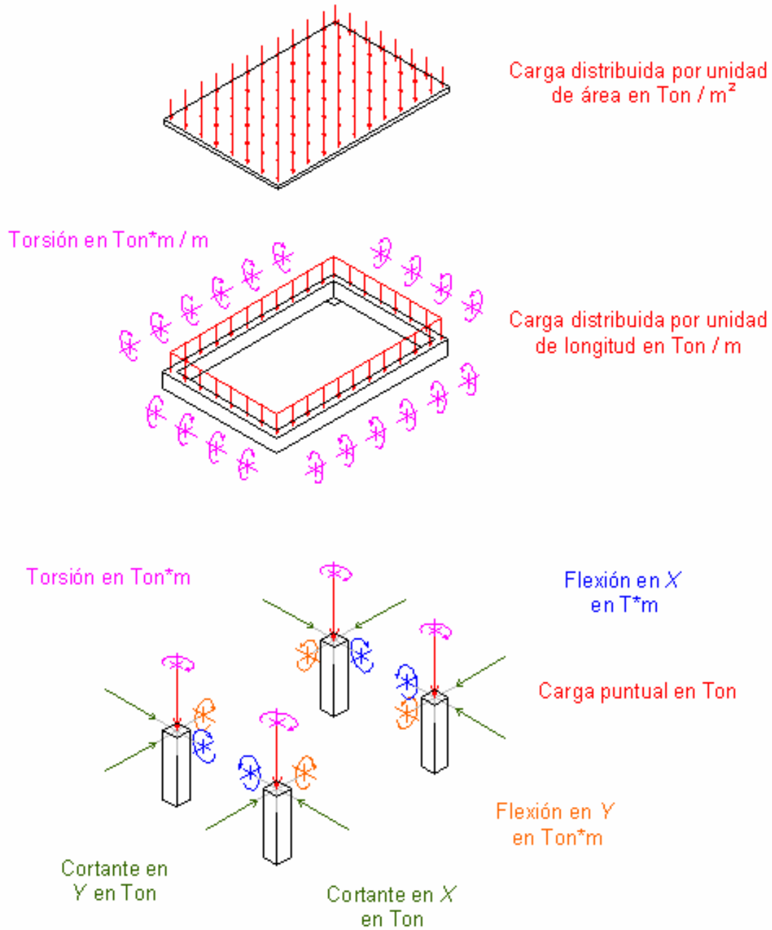
Figura 2 Bajada de cargas o transmisibilidad de efectos
