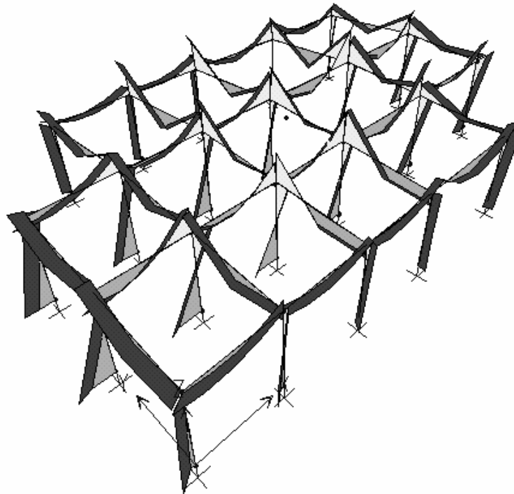
Figura 8 Diagrama de momentos eje 2-2
