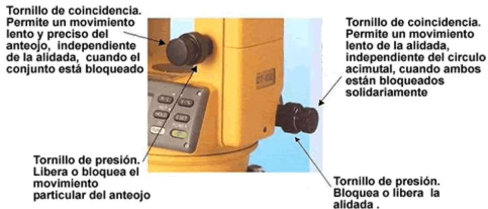
Figura 14 Tornillos
