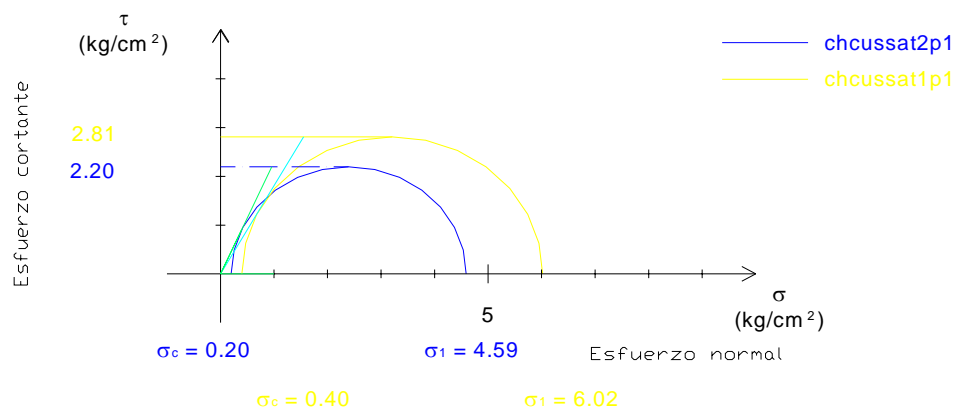
Gráfica 12 Grafica Esfuerzo- Deformación
