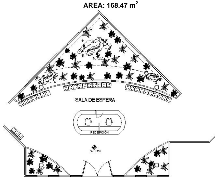
Figura 4 Sala de espera (planta)
