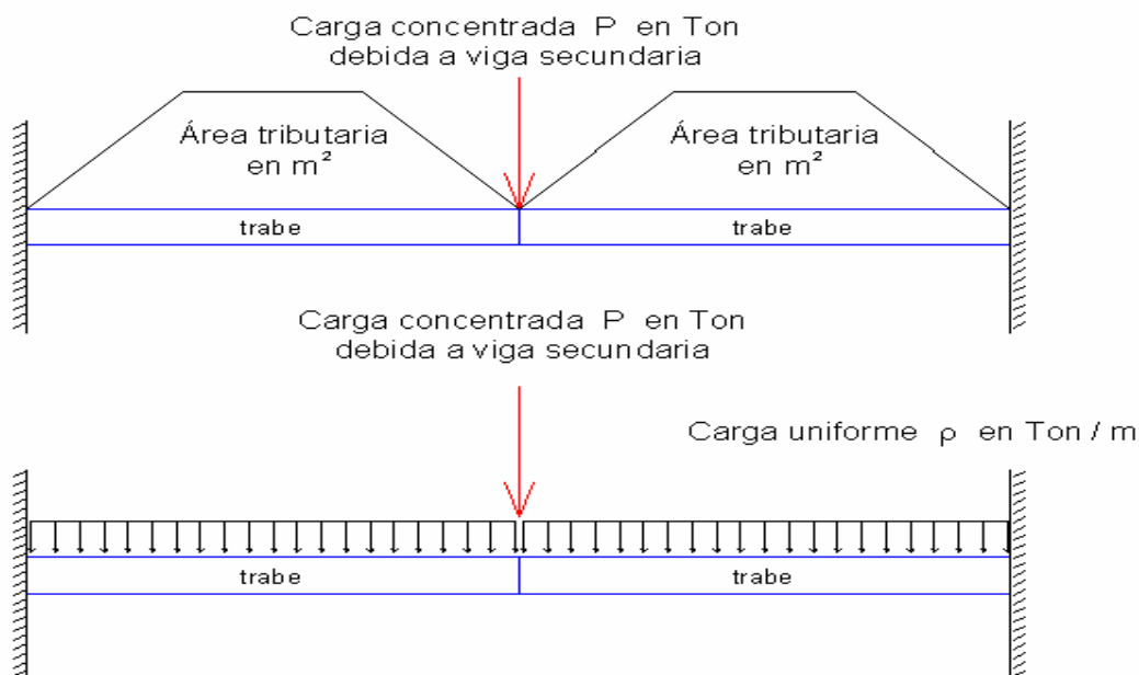
Figura 10 Esquema de una trabe de orilla con una viga secundaria
