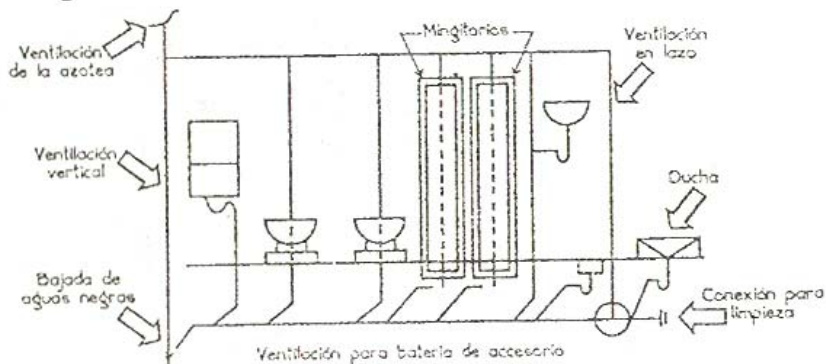
Figura 3 Ventilaciones
