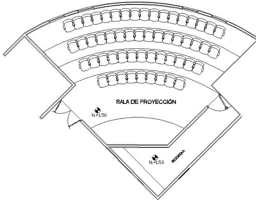
Figura 17 Sala de proyección (planta)
