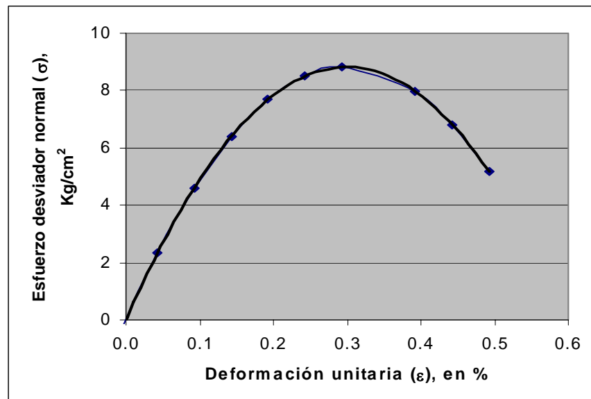
Gráfica 10 Curva esfuerzo-deformación
