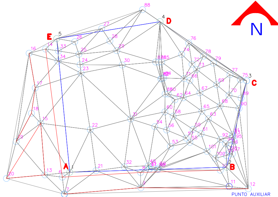
Figura 4 Estaciones, Punto Auxiliar y Puntos Asignados.
