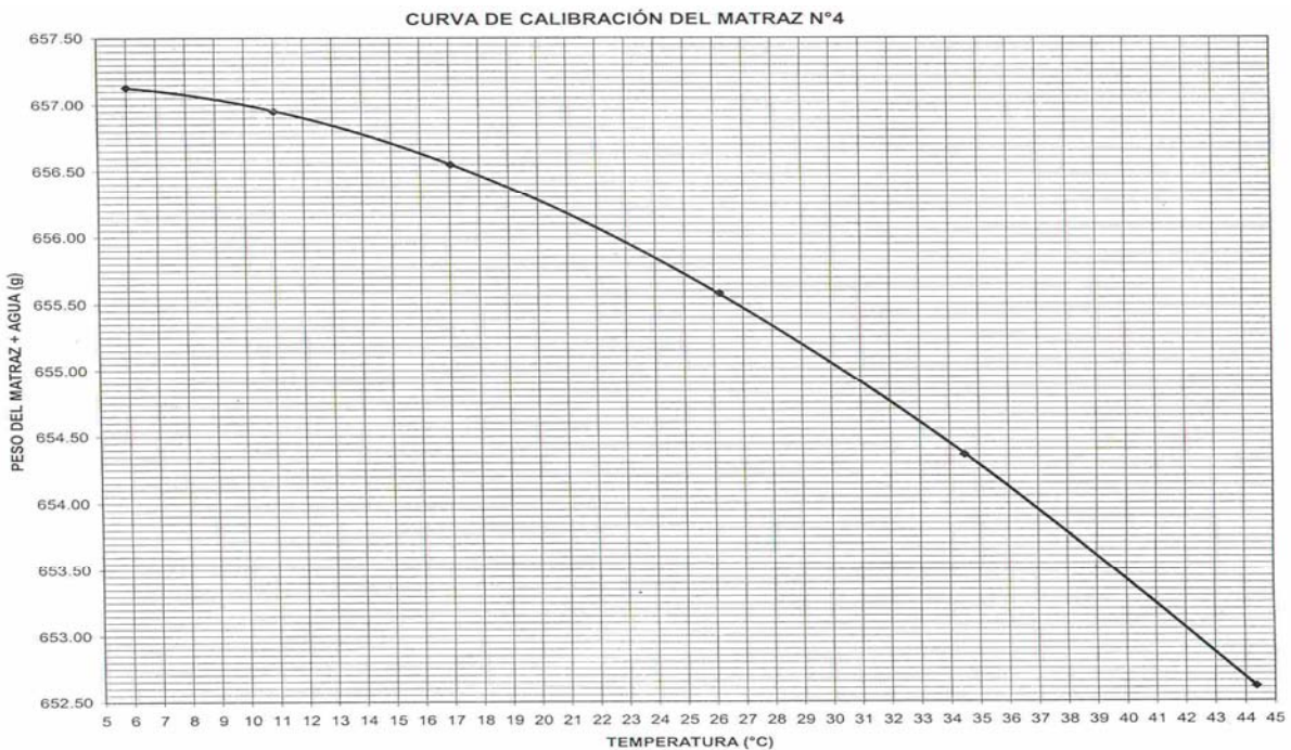
Gráfica 5 Curva de calibración del matraz 4 (Pozo2)
