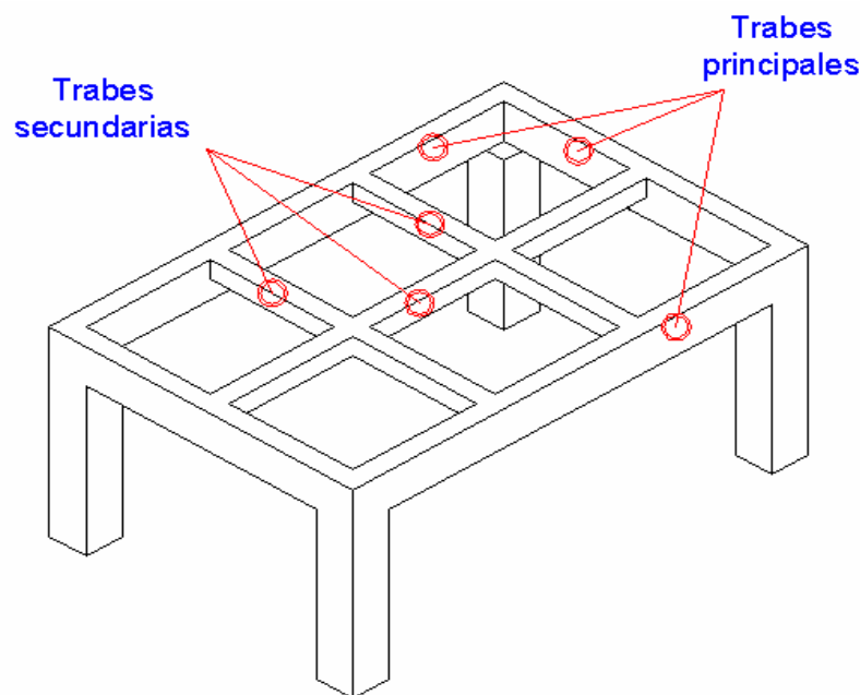
Figura 7 Travesas primarias y secundarias para grandes claros
