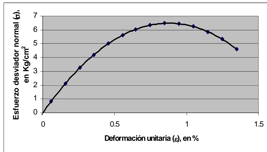
Gráfica 8 Curva esfuerzo-deformación
