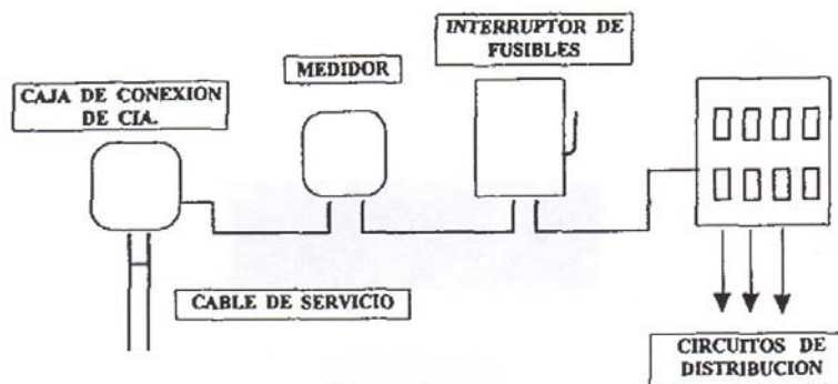
Figura 9 Instalación del transformador al circuito de distribución
