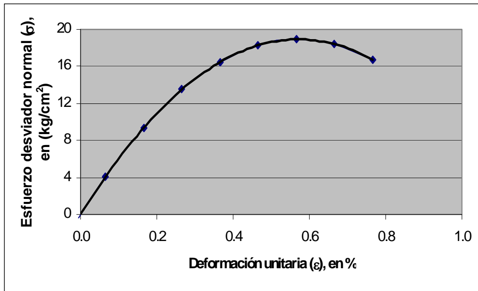
Gráfica 7 Curva esfuerzo-deformación
