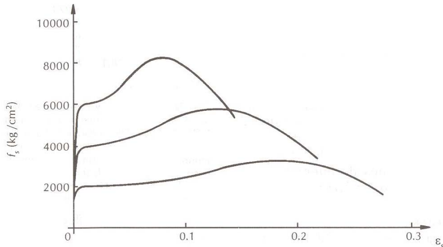
Figura 17 Curva esfuerzo-deformación de aceros laminados en caliente
