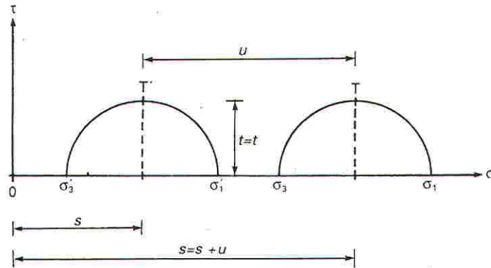
Figura 5 Teoría de falla de Mohr-Coulomb
