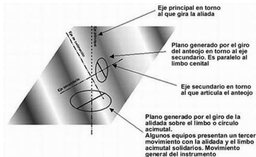
Figura 10 Ejes de la Estación total.
