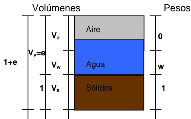
Figura 2 Esquema de una muestra de suelo
