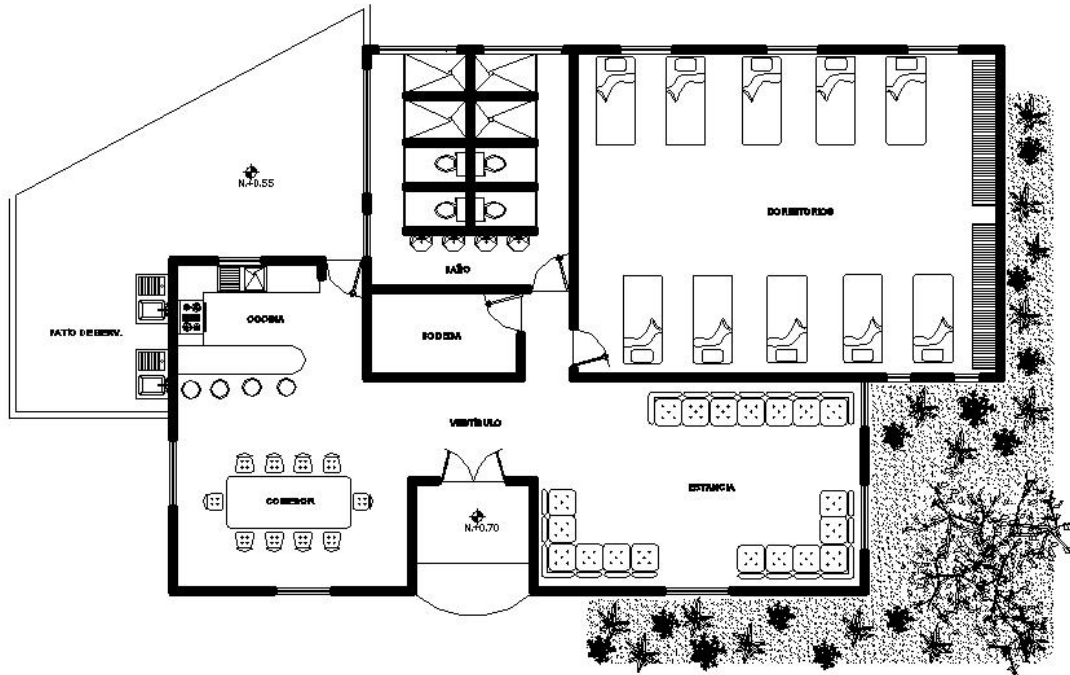
Figura 21 Dormitorios (planta)
