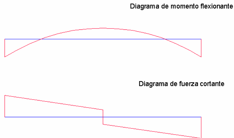
Figura 12 Elementos mecánicos de una trabe de orilla con una viga secundaria
