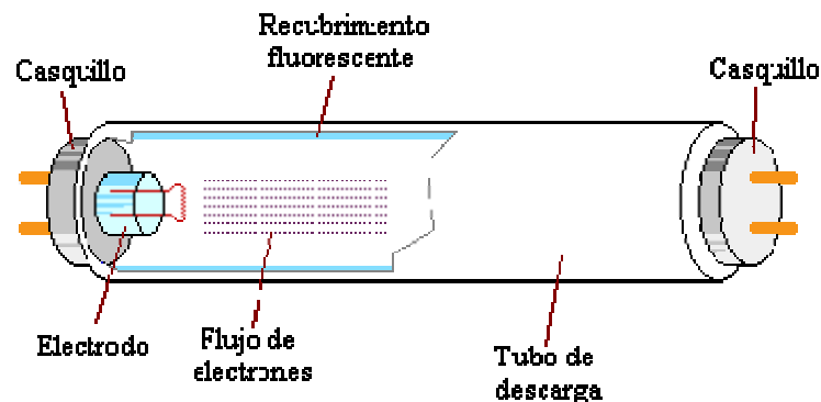
Figura 7 Lámpara fluorescente
