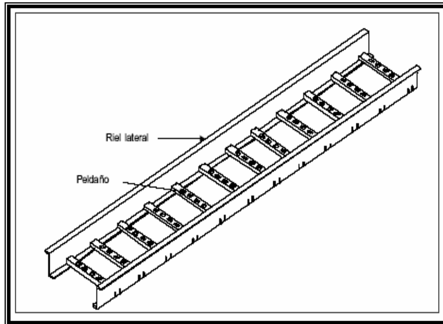
Fig. 9 Escalera portacables.
