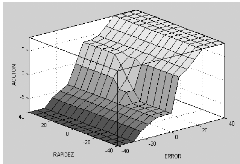
Figura 8.4 Superficie de control del controlador difuso diseñado para el sistema de nivel de líquido.
