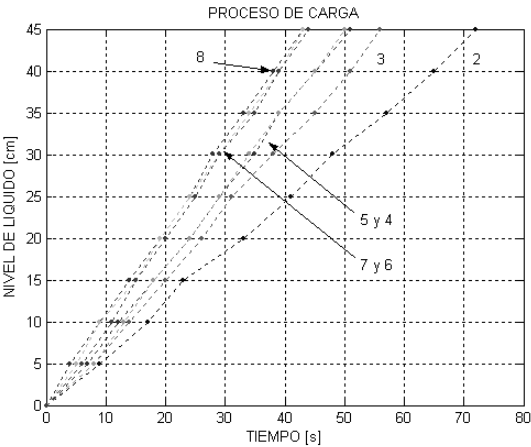
Figura 4 Proceso de llenado.
