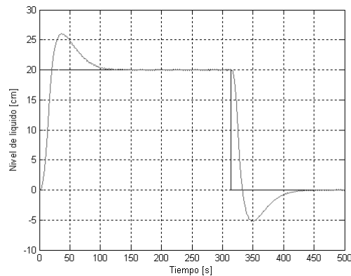
Figura 8.19 Respuesta escalón del sistema de nivel de líquido con el controlador PID diseñado mediante el método de límite de estabilidad.
