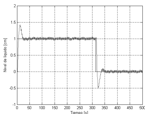
Figura B2 Respuesta escalón del sistema con los parámetros obtenidos del controlador PID con el método de limite de estabilidad.
