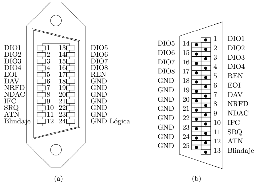
Figura 2.9: Conectores IEEE488, (a) americano, (b) europeo.
