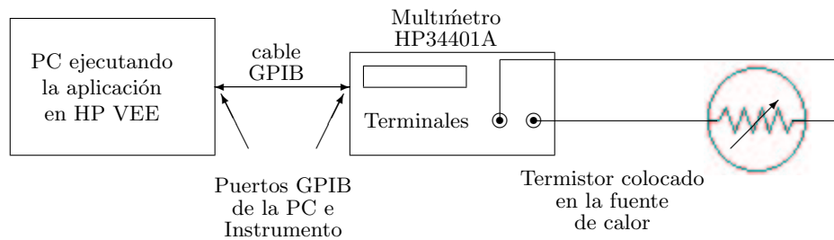
Figura 4.13: Conexión del Termistor NTC
