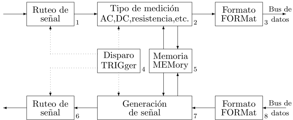
Figura A.1: Modelo de un instrumento programable
