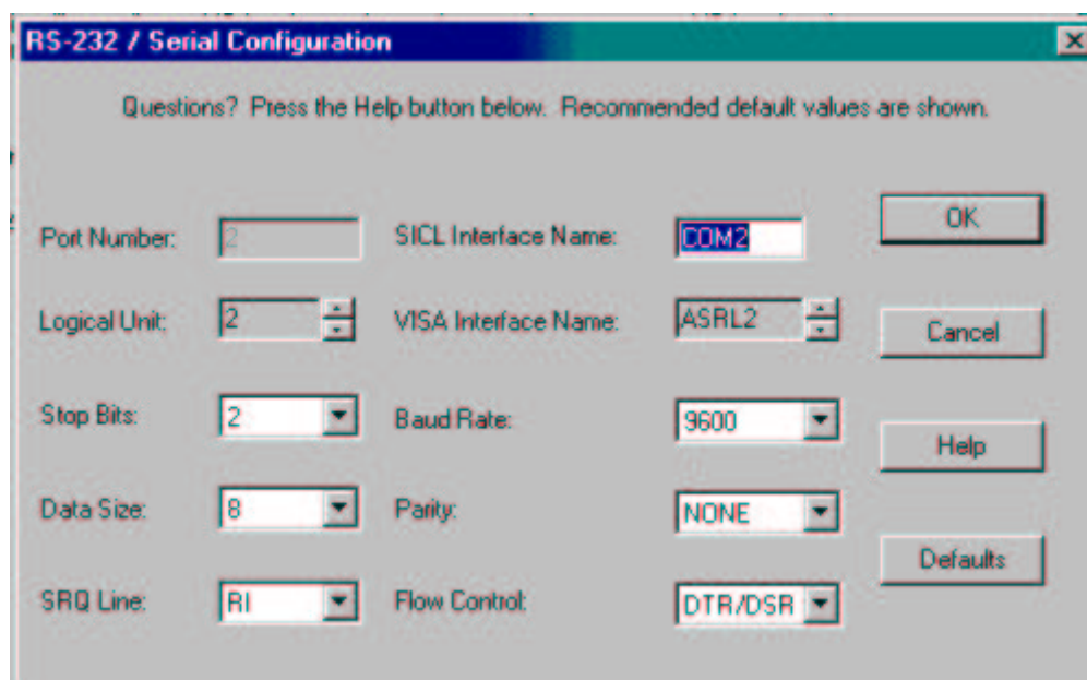
Figura 4.64: Parámetros de comunicación del puerto serie.
