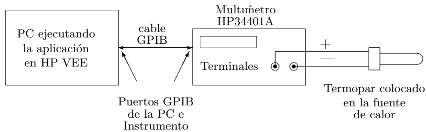
Figura 4.12: Conexión del Termopar tipo J
