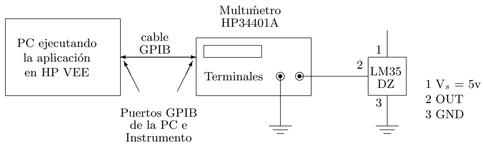
Figura 4.14: Conexión del LM35DZ
