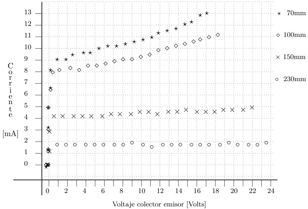
Figura 4.33: comportamiento del fototransistor.
