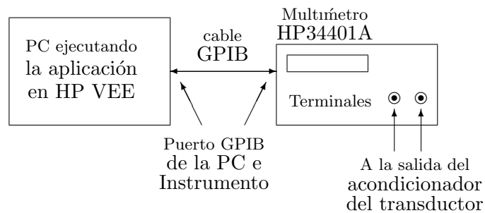
Figura 4.43: Esquema de conexión para visualizador.
