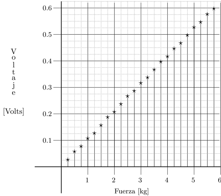
Figura 4.30: Gráfica Módulo G25 (fuerza).
