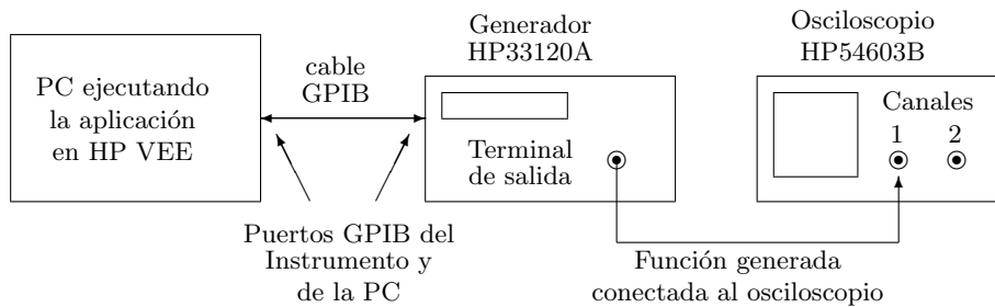
Figura 4.53: Esquema de conexión PC—Instrumento (HP33120A).
