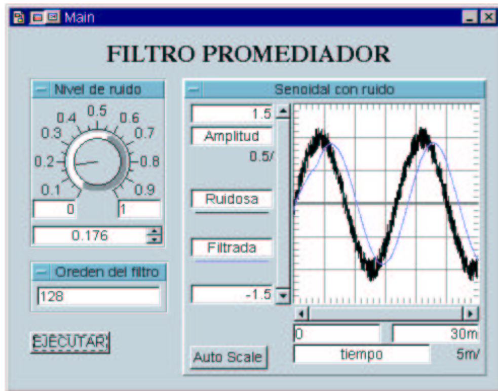
Figura 3.9: Panel de usuario del filtro promediador.
