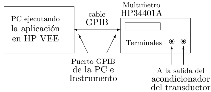
Figura 4.1: Esquema de conexión PC-Instrumento (HP34401A).
