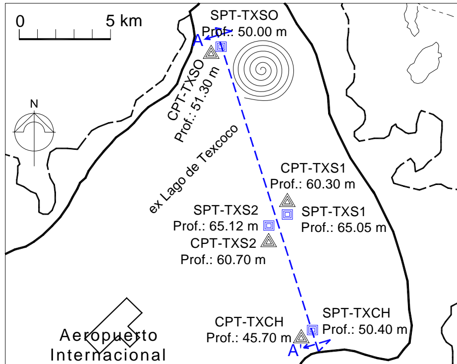
Figura 2.2. Ubicación de los sondeos de exploración del subsuelo
