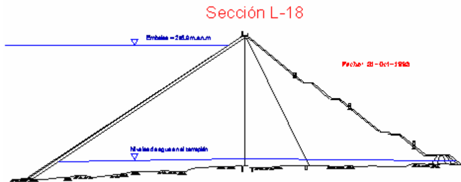
Fig. I. 32. Niveles de agua al final del primer llenado. Sección L-18.
