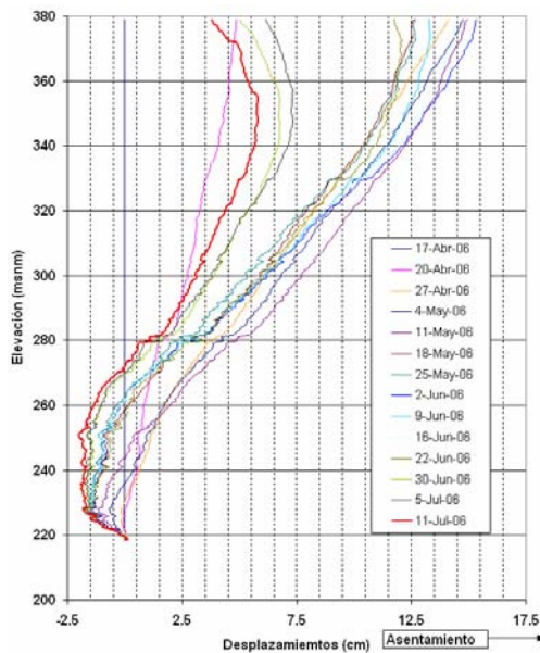
Fig. III.38. Desplazamientos normales a la cara de concreto. Inclínómetros inclinados. IL-21. Sección L-21.
