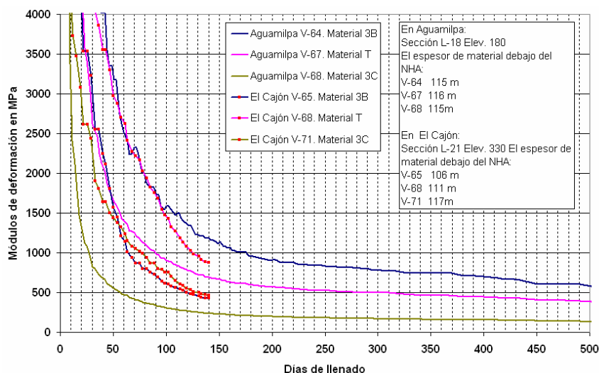
Fig. IV.79. Módulos de deformación (Penman).NHA. Tercera plataforma de instrumentación.
