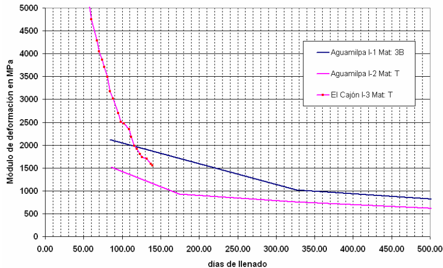
Fig. IV.83. Módulos de deformación. Inclínómetros en el terraplén. Materiales 3B y T.
