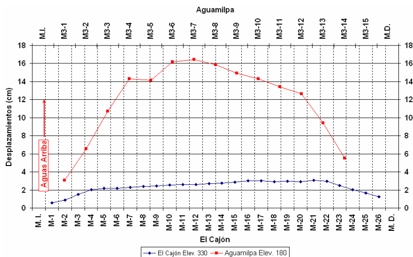
Fig. IV.75. Desplazamientos horizontales en referencias topográficas. Eje del río. Tercera plataforma de instrumentación.
