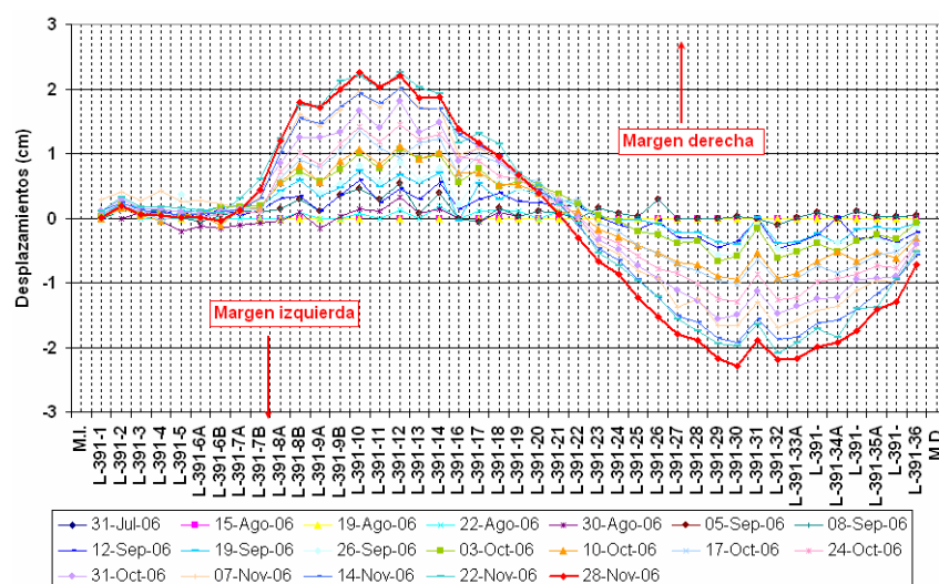
Fig. IV.39. Desplazamientos en la cara de concreto. Referencias topográficas. Eje de la cortina. Elev. 391.
