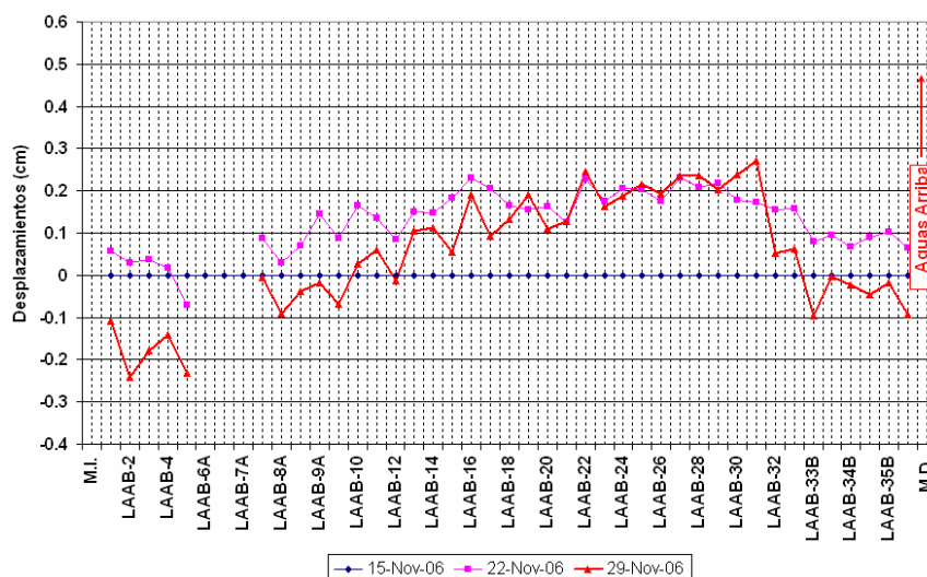
Fig. IV.39. Desplazamientos en la cara de concreto. Referencias topográficas. Eje del río. Parapeto aguas abajo.
