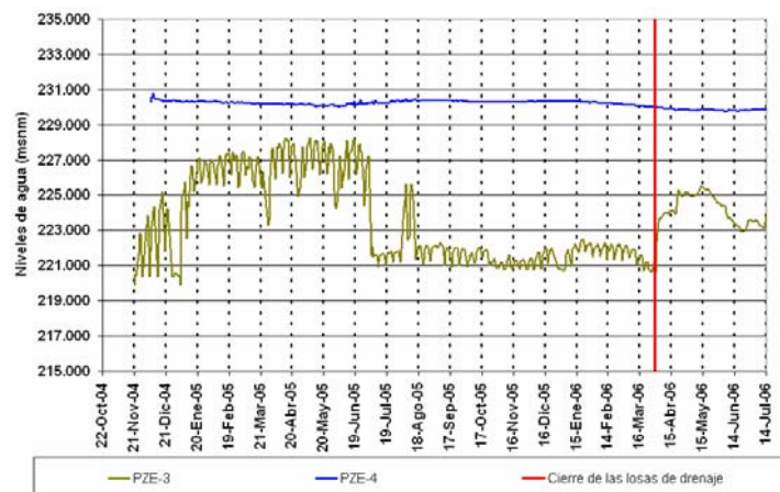
Fig. III.23. Niveles de agua en la sección L-18.
