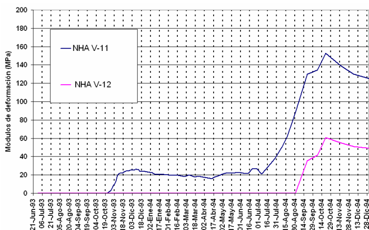
Fig. I. 24. Módulos de deformación (Fitzpatrick). Material T. Sección L-18. Elev. 90 m.s.n.m.
