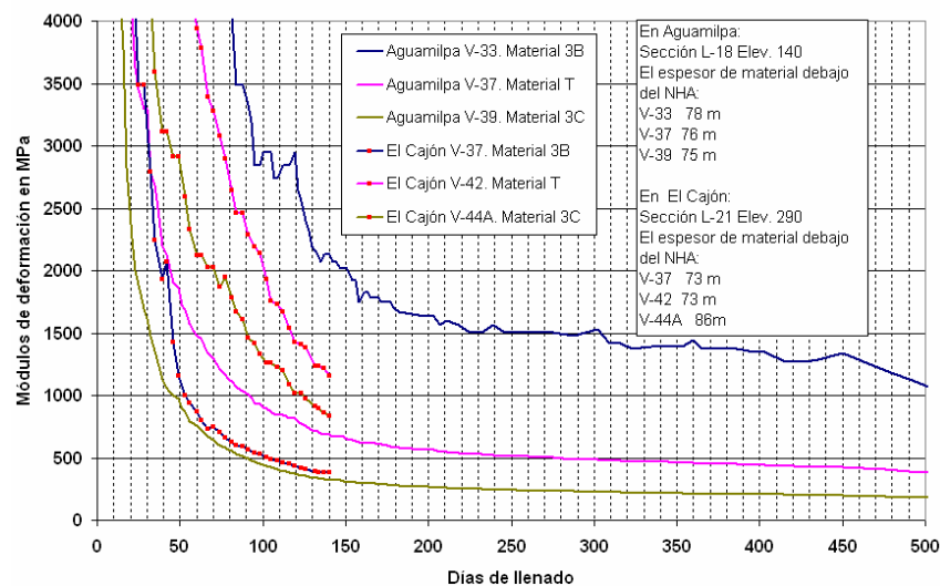
Fig. IV.78. Módulos de deformación (Penman).NHA. Segunda plataforma de instrumentación.
