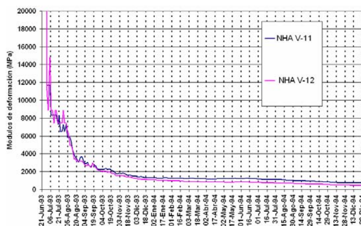
Fig. I. 19. Módulos de deformación (Penman). Material T. Sección L-18. Elev. 90 m.s.n.m.
