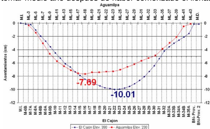
Fig. IV.67. Asentamientos en referencias topográficas. Corona. Aguas abajo.
