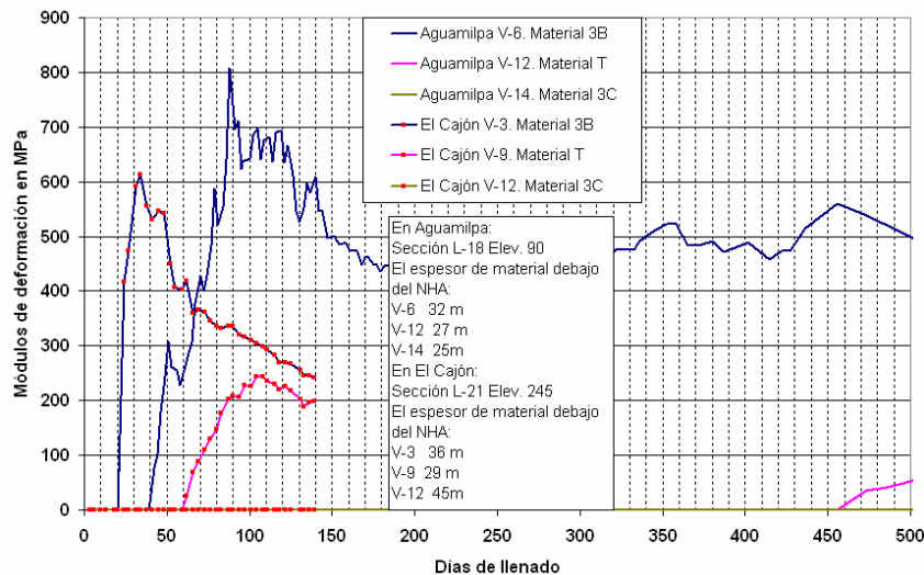
Fig. IV.80. Módulos de deformación (Fitzpatrick).NHA. Primera plataforma de instrumentación.
