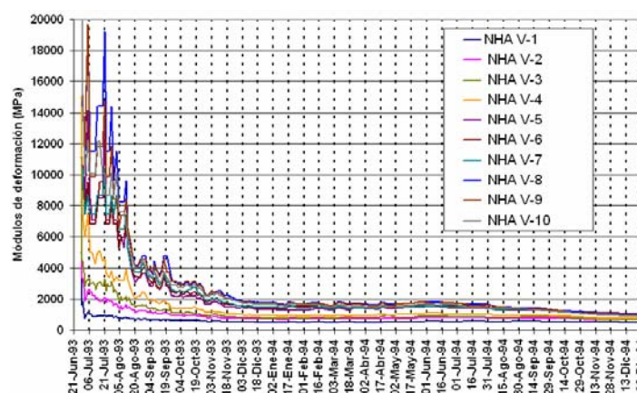
Fig. I. 18. Módulos de deformación (Penman). Material 3B. Sección L-18. Elev. 90 m.s.n.m.
