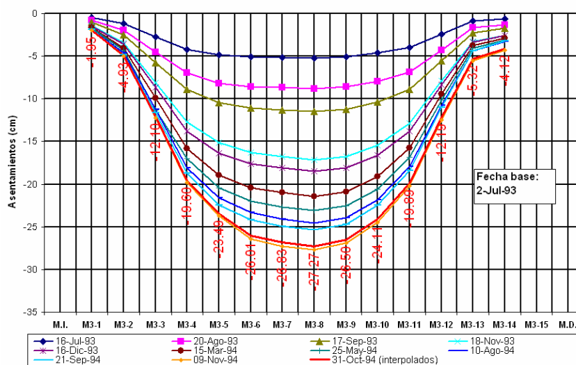
Fig. I. 11. Asentamientos en enrocamiento. Línea L-3. Elev. 180.
