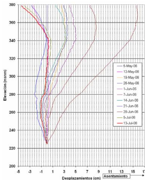
Fig. III.39. Desplazamientos normales a la cara de concreto. Inclínómetros inclinados. IL-26. Sección L-26.
