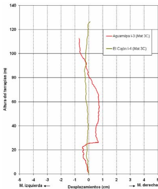
Fig. IV.72. Desplazamientos horizontales. Eje de la cortina. Inclinómetros instalados en el respaldo aguas abajo de la cortina. Sección máxima.
