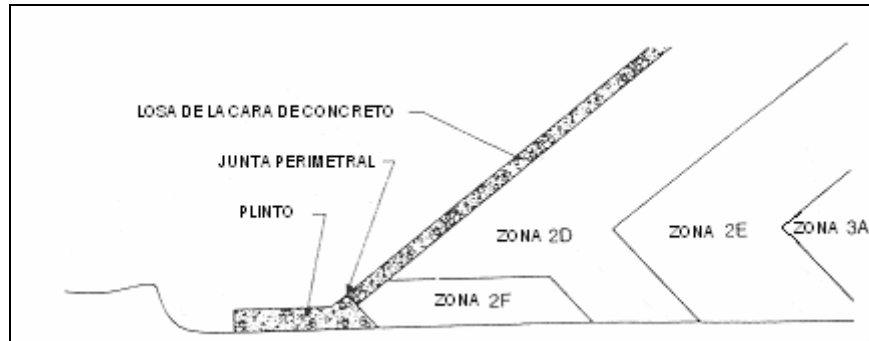
Fig. 2. Disposición del plinto, losa de concreto y material de recargue.
