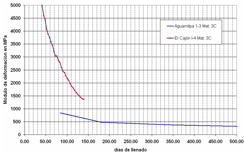
Fig. IV.84. Módulos de deformación. Inclínómetros en el terraplén. Material 3C.
