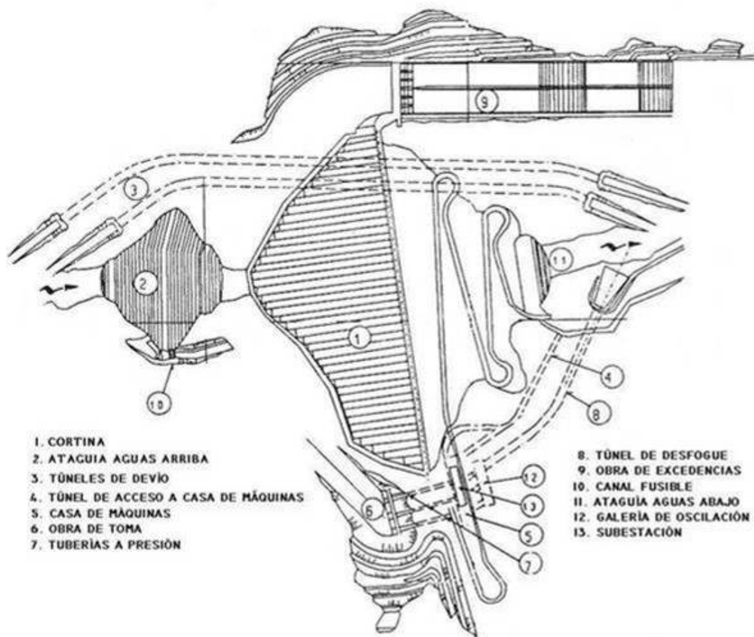
Fig. I.1. Esquema general de la C. H. Aguamilpa
