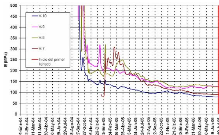
Fig. III.17. Módulos de deformación (Penman). Sección L-21. Elev. 245 m.s.n.m.
