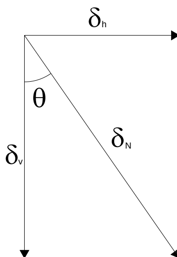
Fig. I. 22. Desplazamientos en el terraplén bajo la hipótesis de que la resultante es en dirección normal.
