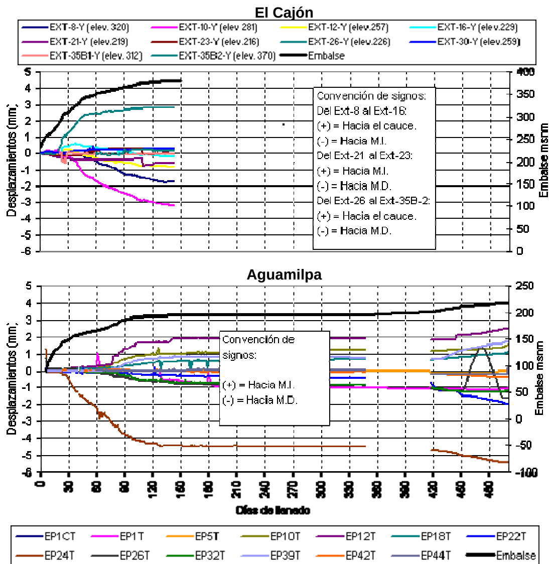
Fig. IV.93. Movimientos tangentes a la junta losa-plinto. Extensómetros tridimensionales.
