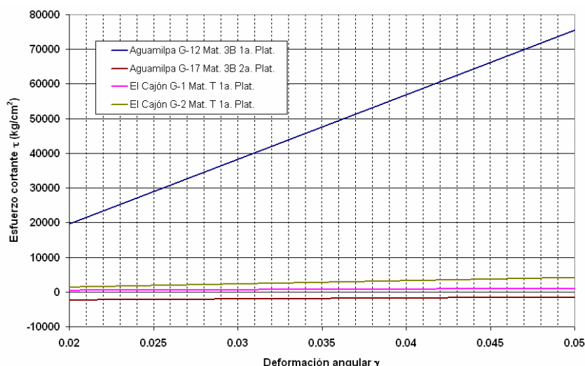
Fig. IV.86. Módulos de deformación. Módulo G. Grupos de Celdas de Presión y Extensómetros.
