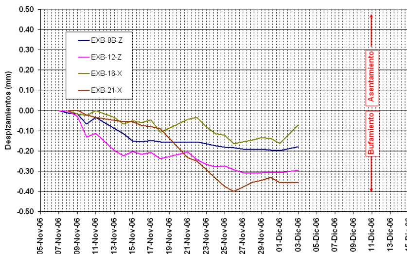
Fig. IV.48. Movimientos de asentamientos de la junta losa-parapeto. (Dirección Z). Extensómetros bidimensionales.
