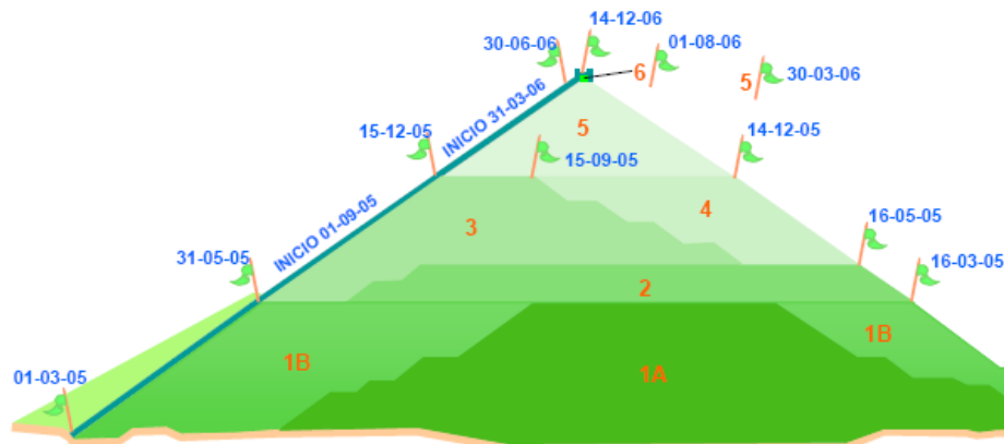
Fig. III. 1. Etapas de construcción del terraplén.
