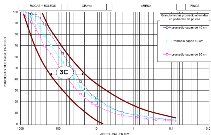
Fig. II.11. Granulometría Material 3C.
