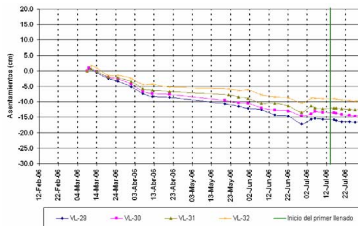
Fig. III.6. Asentamientos en losas concreto. Elev. 361. Losas centrales.
