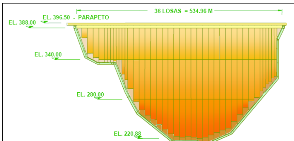
Fig. III. 2. Etapas de colado de la cara de concreto.
