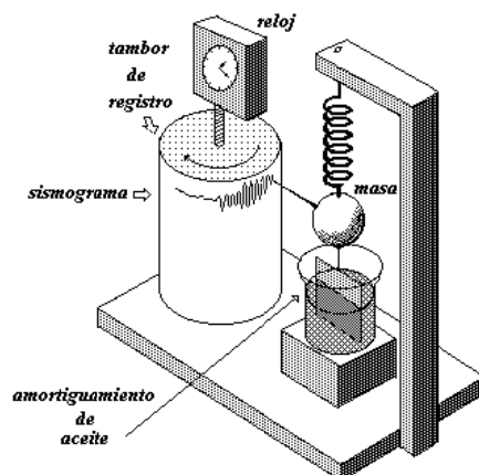
Figura 4.4.1. Sismógrafo
