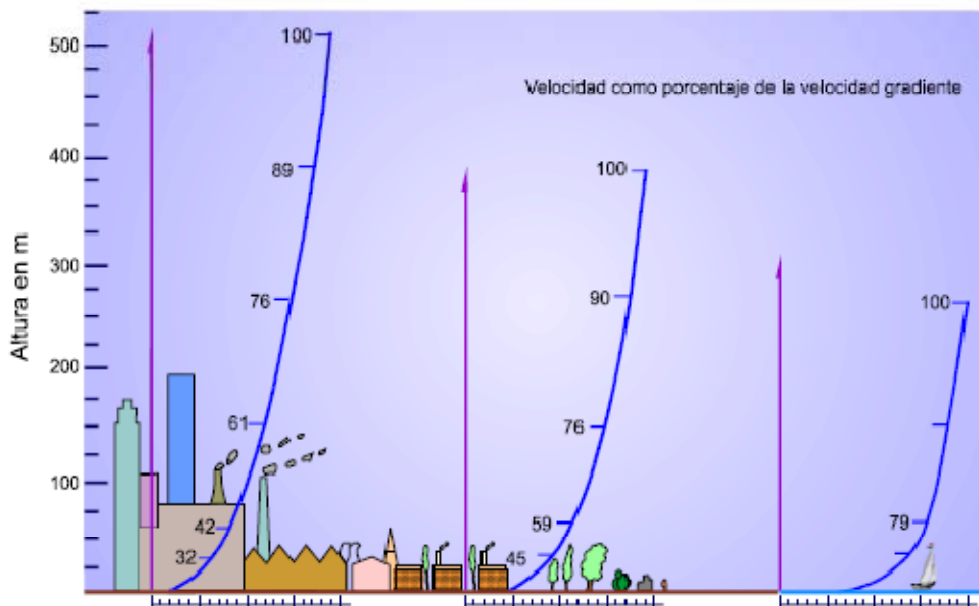
Figura 3.3.10.2. Variación de la velocidad del viento con la altura sobre terrenos de diferentes rugosidades.
