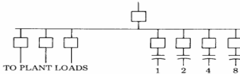
Figura 7.6 Capacitores conmutados en valores binarios
