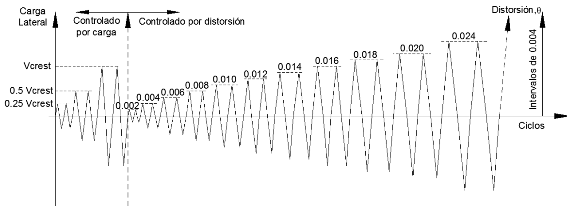
Figura 3.10. Protocolo de ensaye
