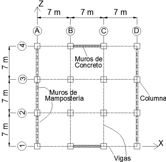
Figura 3.1. Configuración en planta de los prototipos.
