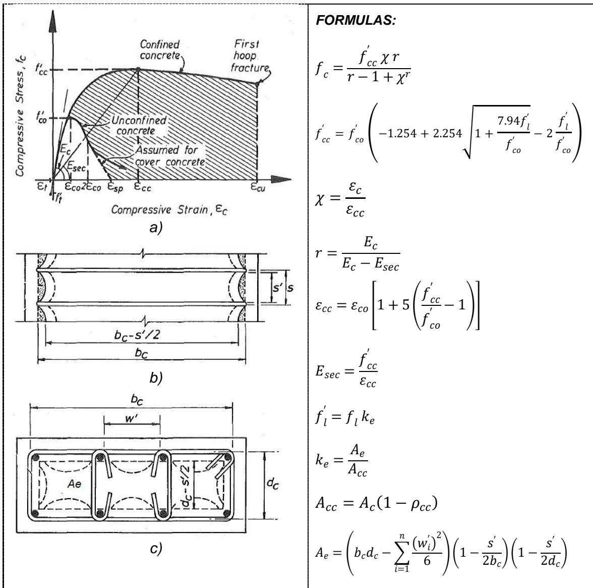
Figura A1.4. Modelo de Mander et. al (1988) para concreto confinado. a) Relación esfuerzo – deformación, b) propiedades geométricas que definen el modelo, vista en elevación, c) propiedades geométricas que definen el modelo, vista en planta.
