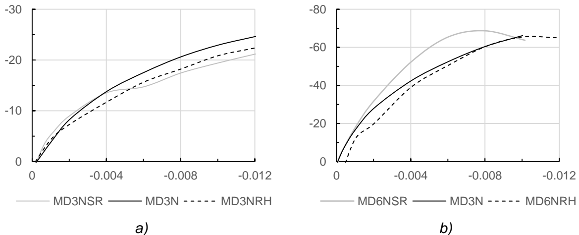
Figura 4.8. Gráficas envolventes momento flector M_z (kN-m) – Desplazamiento Lateral (mm) en SC1. a) Especímenes con columnas de menor tamaño, b) especímenes con columnas de mayor tamaño.
