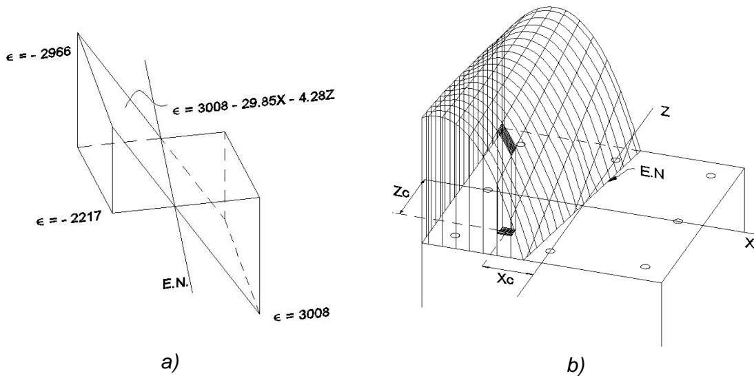
Figura A2.1 Deformaciones y esfuerzos en la sección transversal al pie de columna del espécimen MD3N a una distorsión \Delta = -0.01 . a) Plano promedio de deformaciones, b) diagrama de esfuerzos en la sección
