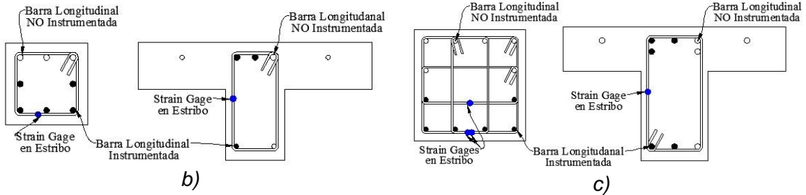
Figura 3.12. Instrumentación interna. a) Ubicación de los strain gages en los especímenes, b) ubicación de los strain gages en las secciones instrumentadas de los especímenes con columnas de menor tamaño, c) ubicación de los strain gages en las secciones instrumentadas de los especímenes con columnas de mayor tamaño.
