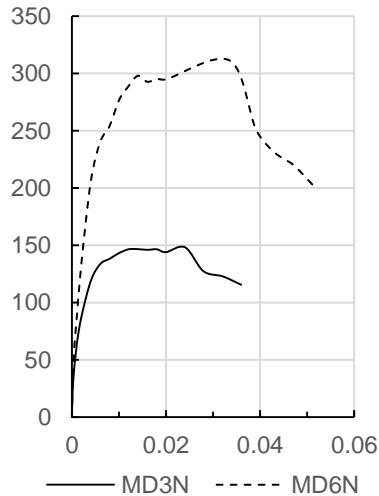
Figura 5.1. Curvas envolventes carga lateral (kN) – distorsión (mm/mm) de especímenes con diferente rigidez relativa muro/marco.
