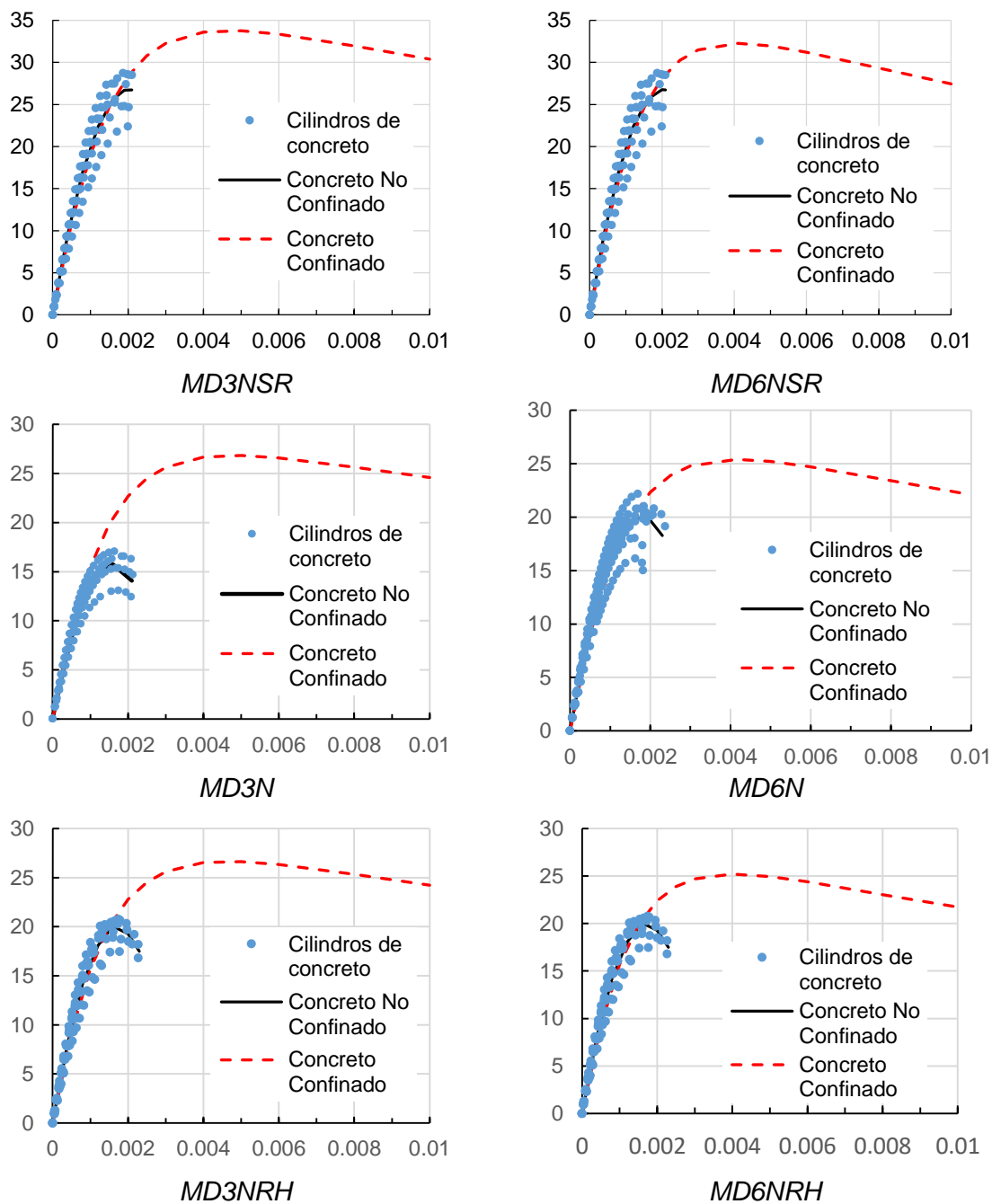
Figura A1.5. Graficas esfuerzo (MPa) – deformación (mm/mm) del concreto no confinado y confinado correspondiente al marco de cada espécimen
