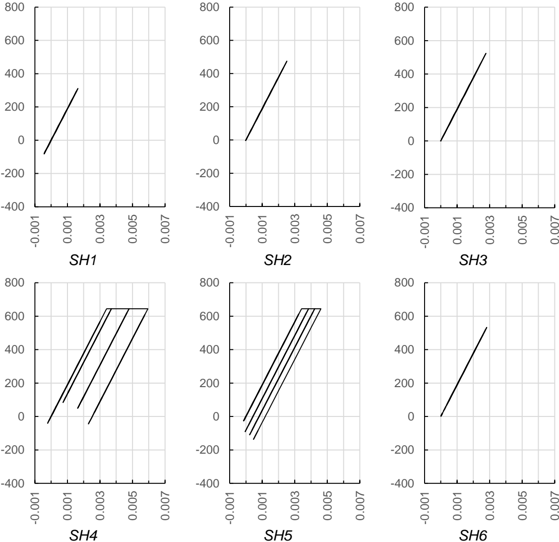
Figura A3.1. Curvas histeréticas esfuerzo (MPa) – deformación (mm/mm) del acero de refuerzo horizontal en el espécimen MD3NRH.
