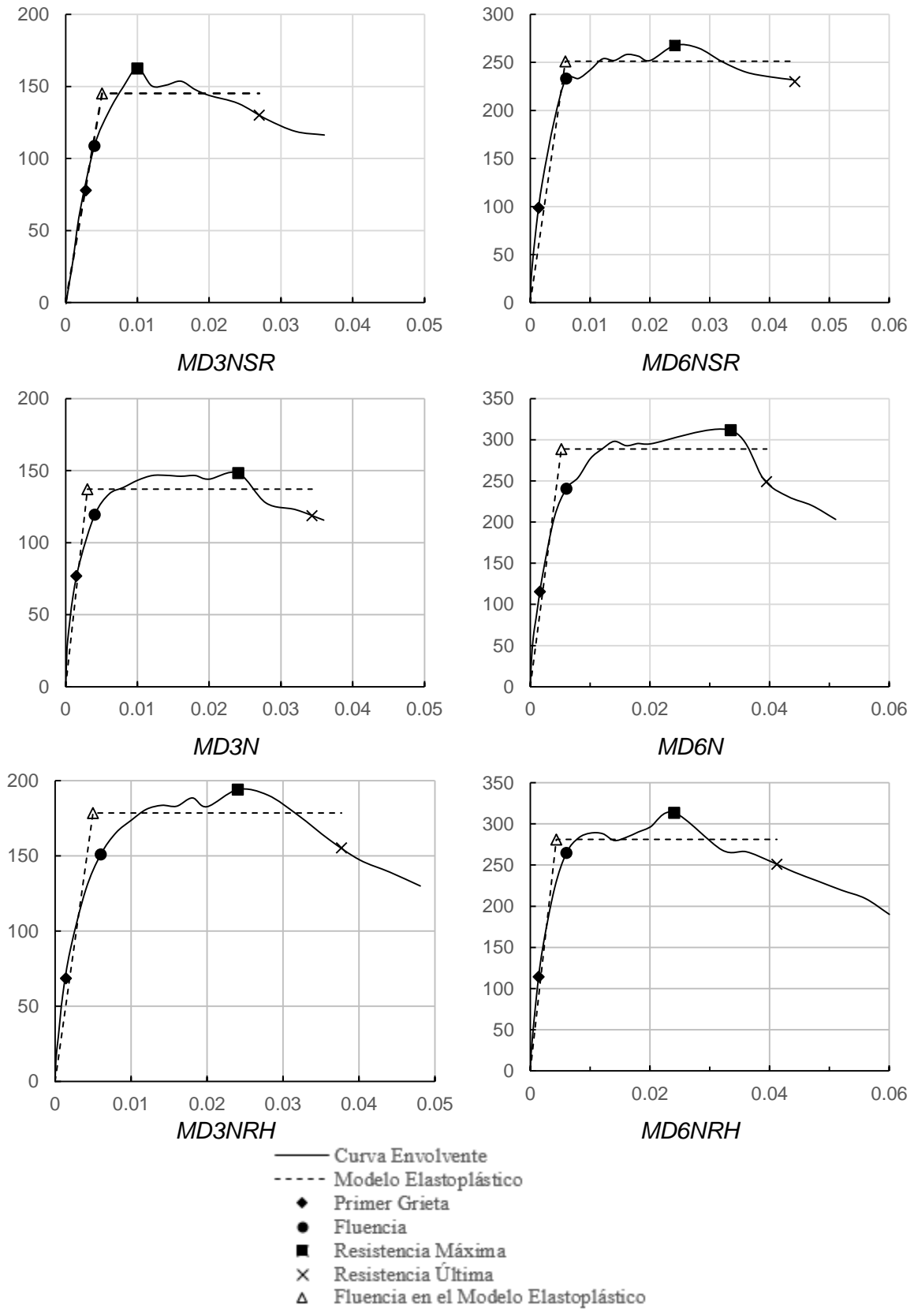
Figura 4.5. Curvas Envolventes positivas carga lateral (kN) - distorsión (mm/mm).
