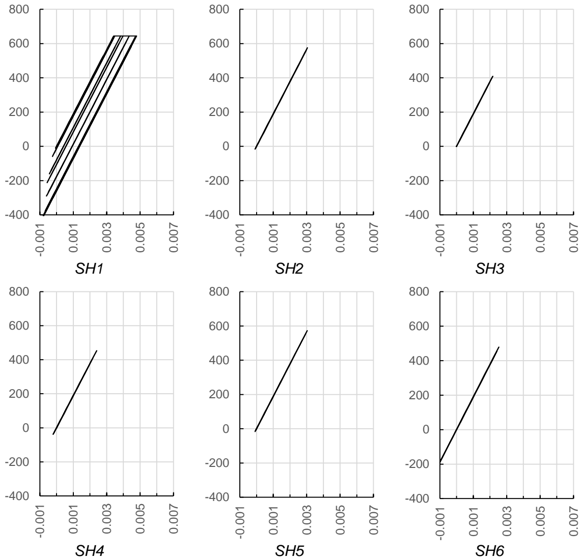
Figura A3.2. Curvas histeréticas esfuerzo (MPa) – deformación (mm/mm) del acero de refuerzo horizontal en el espécimen MD6NRH.
