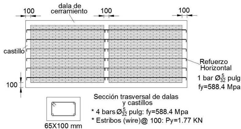
Figura 3.5. Detalles del refuerzo y dimensiones del muro diafragma con elementos de confinamiento
