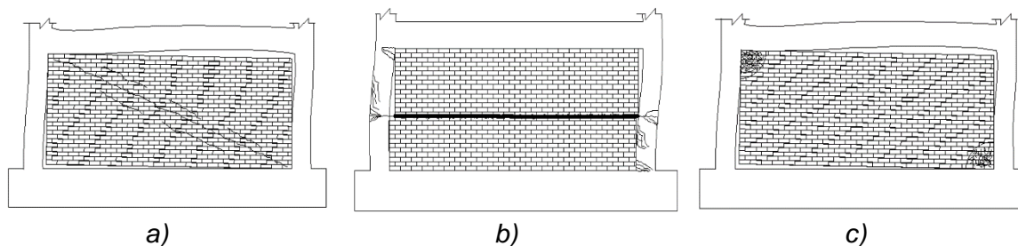
Figura 2.2. Daño en el muro. a) Agrietamiento por tensión diagonal, b) deslizamiento horizontal en las juntas, c) aplastamiento en las esquinas
