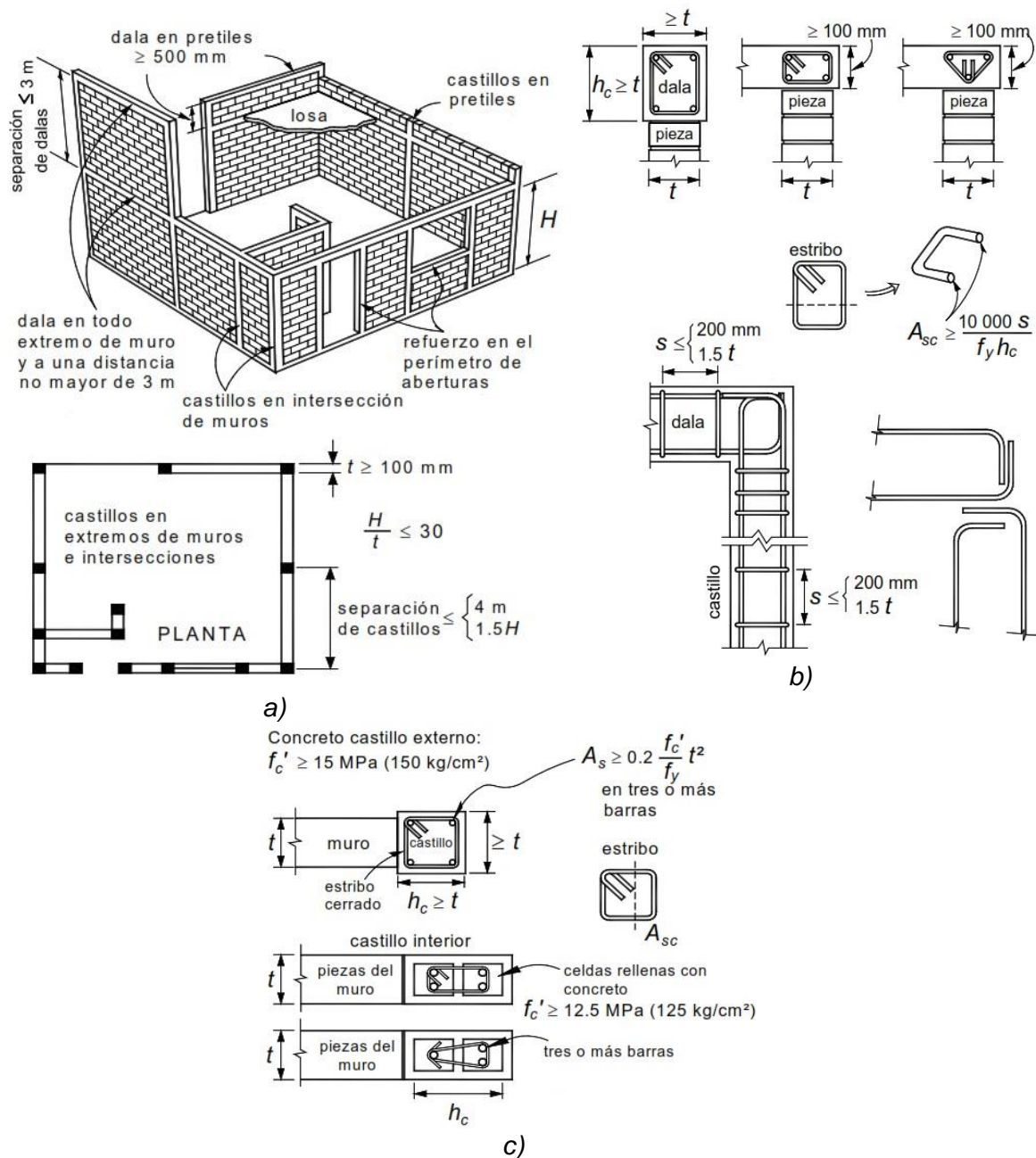
Figura 2.6. Requisitos para mampostería confinada (NTCM, 2004). a) Distribución de elementos de confinamiento en la estructura, b) refuerzo en dalas y castillos, vista en elevación, c) refuerzo en castillos, vista en planta.
