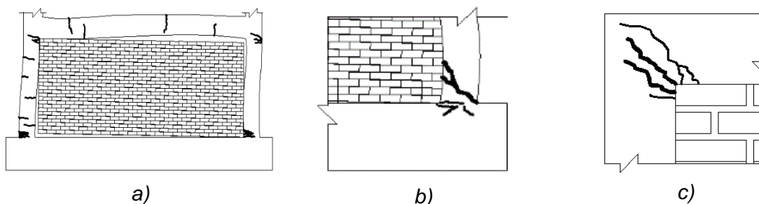
Figura 2.3. Daño en el marco. a) Grietas por flexión, b) falla de columna por cortante, c) falla en la unión viga-columna.
