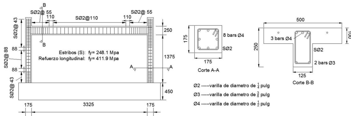
Figura 3.3. Detalles del refuerzo y dimensiones (en milímetros) del marco de los especímenes con columna de menor tamaño.
