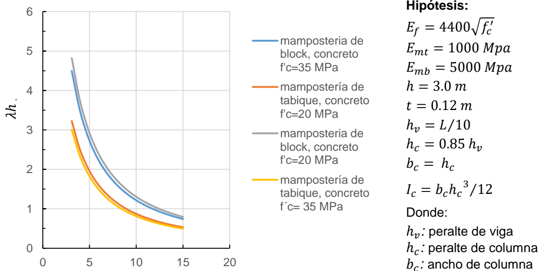
Figura 2.4. Gráficas \lambda h – Longitud del claro entre columnas (m) para materiales y dimensiones típicas de marcos de concreto rellenos con muros de mampostería.
