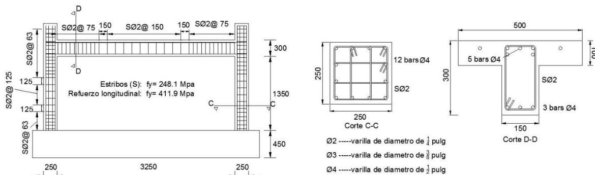
Figura 3.4. Detalles del refuerzo y dimensiones (en milímetros) del marco de los especímenes con columna de mayor tamaño.
