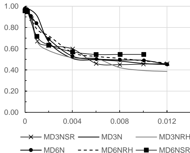
Figura 6.1. Curvas ( I_{Zcr}/I_{Zb} ) – distorsión (mm/mm) de las columnas.
