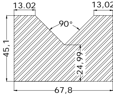
Figura 4. 31 Vertedor triangular
