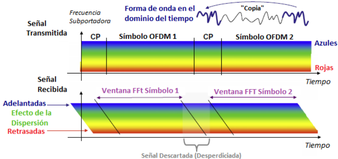
Fig. 2.6 Necesidad de introducir el CP; el canal afecta de forma diferente a las frecuencias que conforman la señal OFDM [35].
