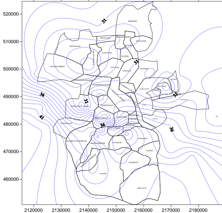
Isoyetas de Intensidad de Precipitación (mm/hr) para una duración de 30 minutos y periodo de retorno de 2 años
