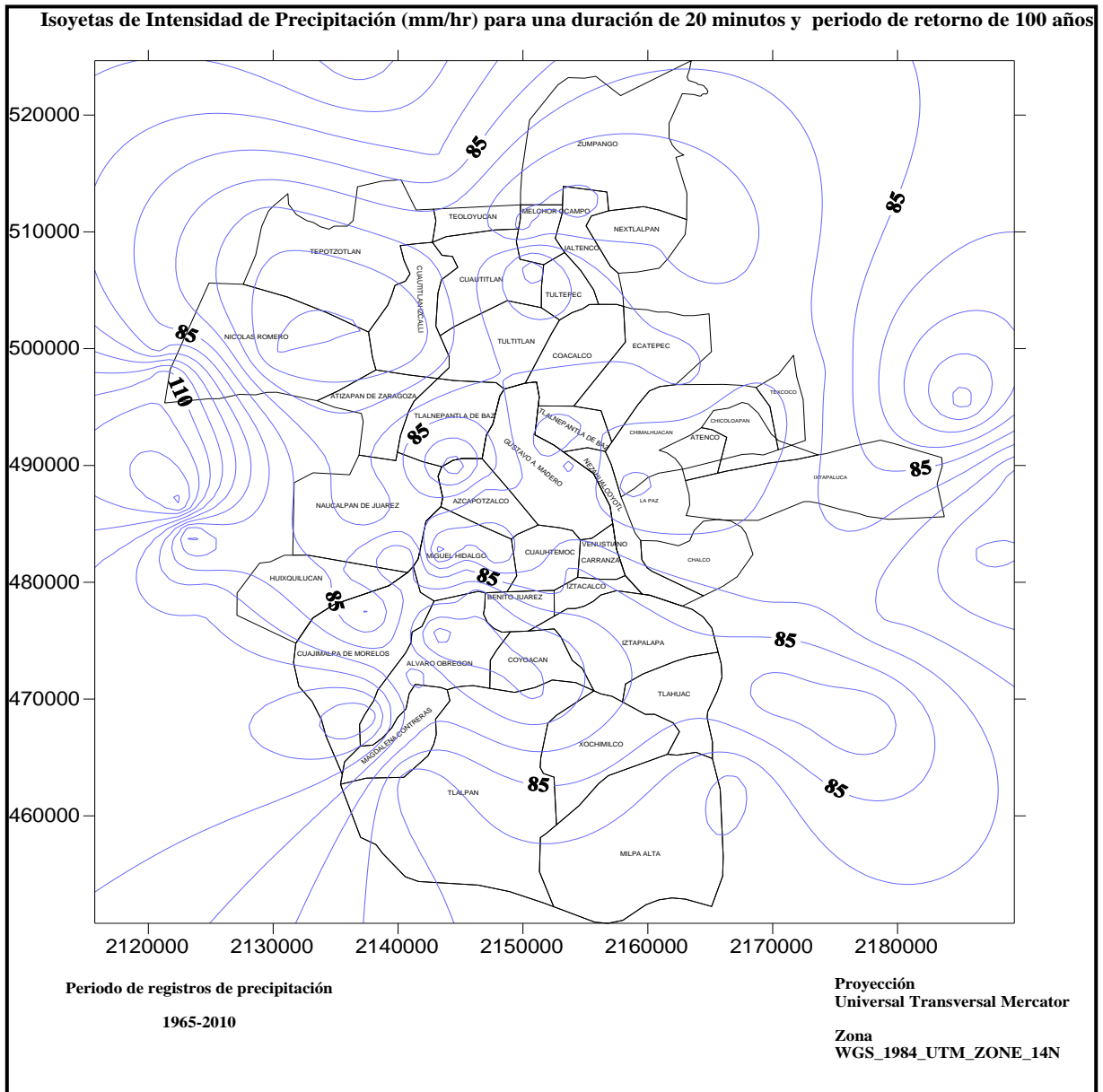
Figura 68. Isoyetas de precipitación para una duración de 20 minutos y periodo de retorno de 100 años elaborada para el área de estudio.
