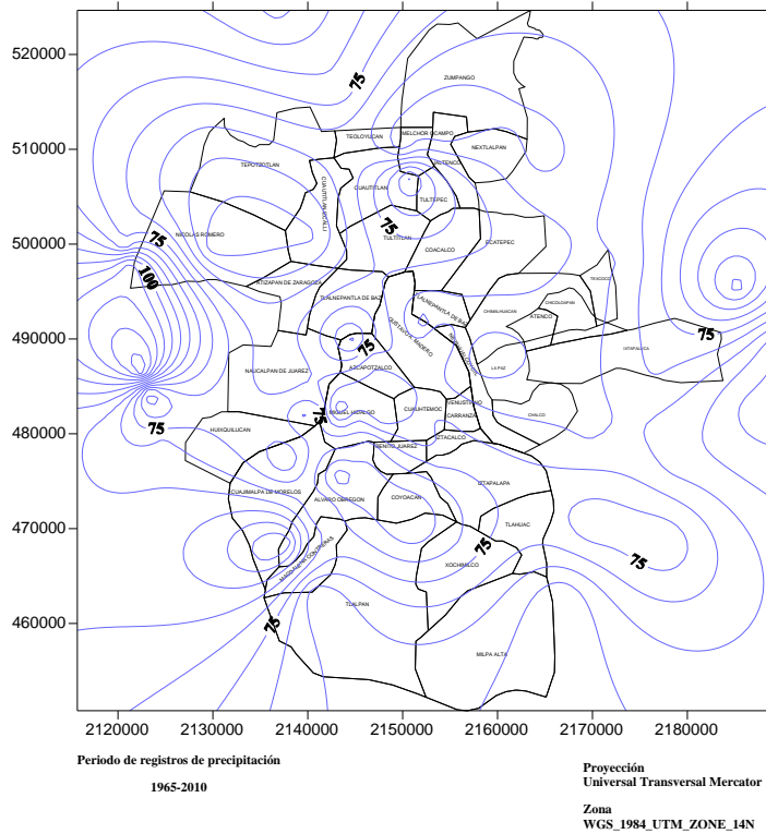
Isoyetas de Intensidad de Precipitación (mm/hr) para una duración de 50 minutos y periodo de retorno de 500 años
