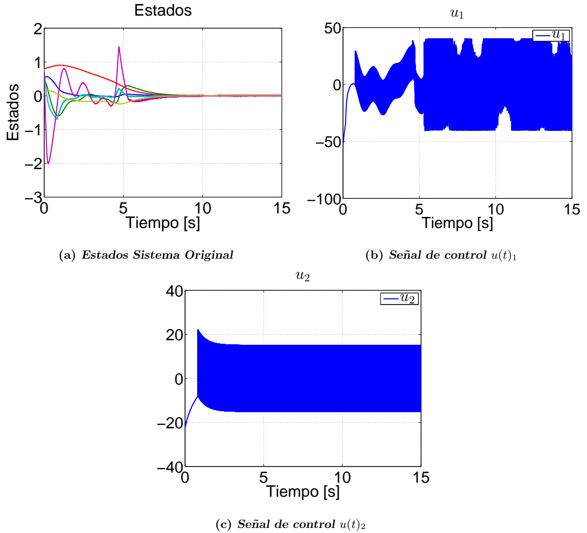
Figura 5.3: Sistema original
