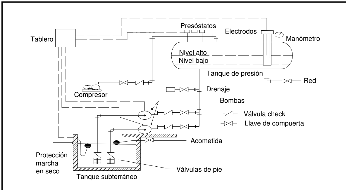
FIGURA V.2 “SISTEMAS HIDRONEUMÁTICOS”
