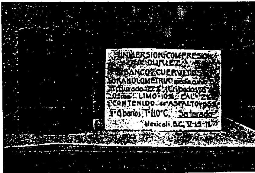
Foto 12. - PROBETA DURIEZ DESPUES DE LA SATURACION
