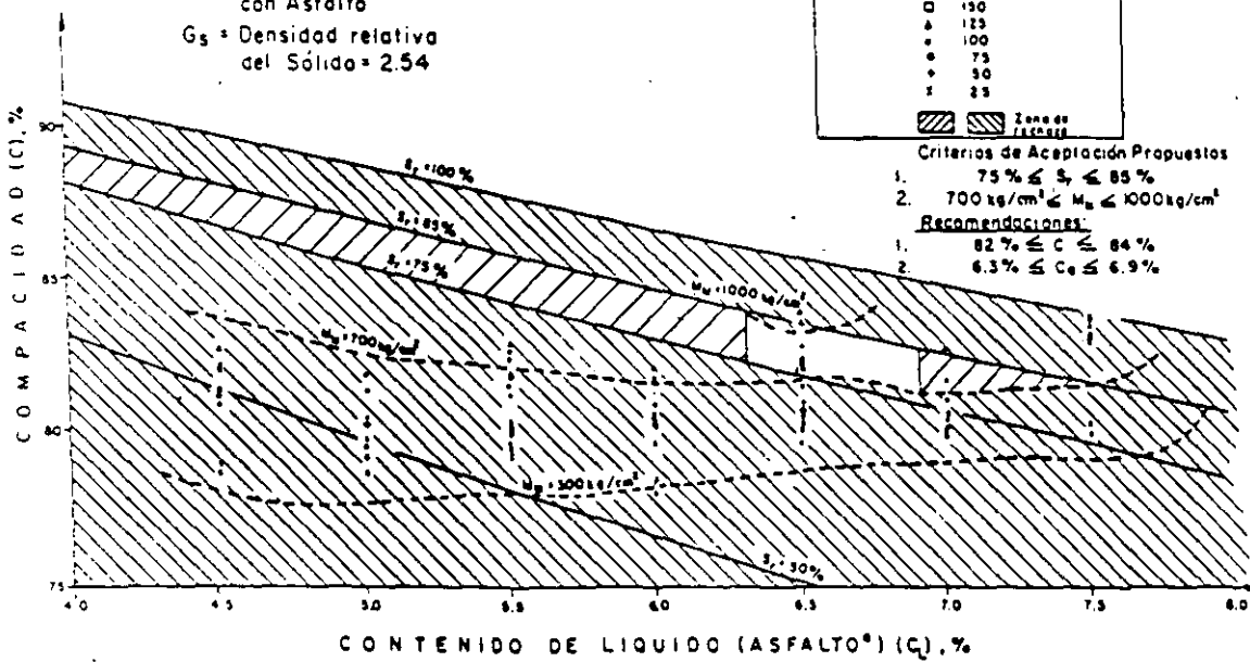
LAMINA 6.- Diagrama CAS.- Curvas de igual módulo Marshall (Refs. 6 y 7)
