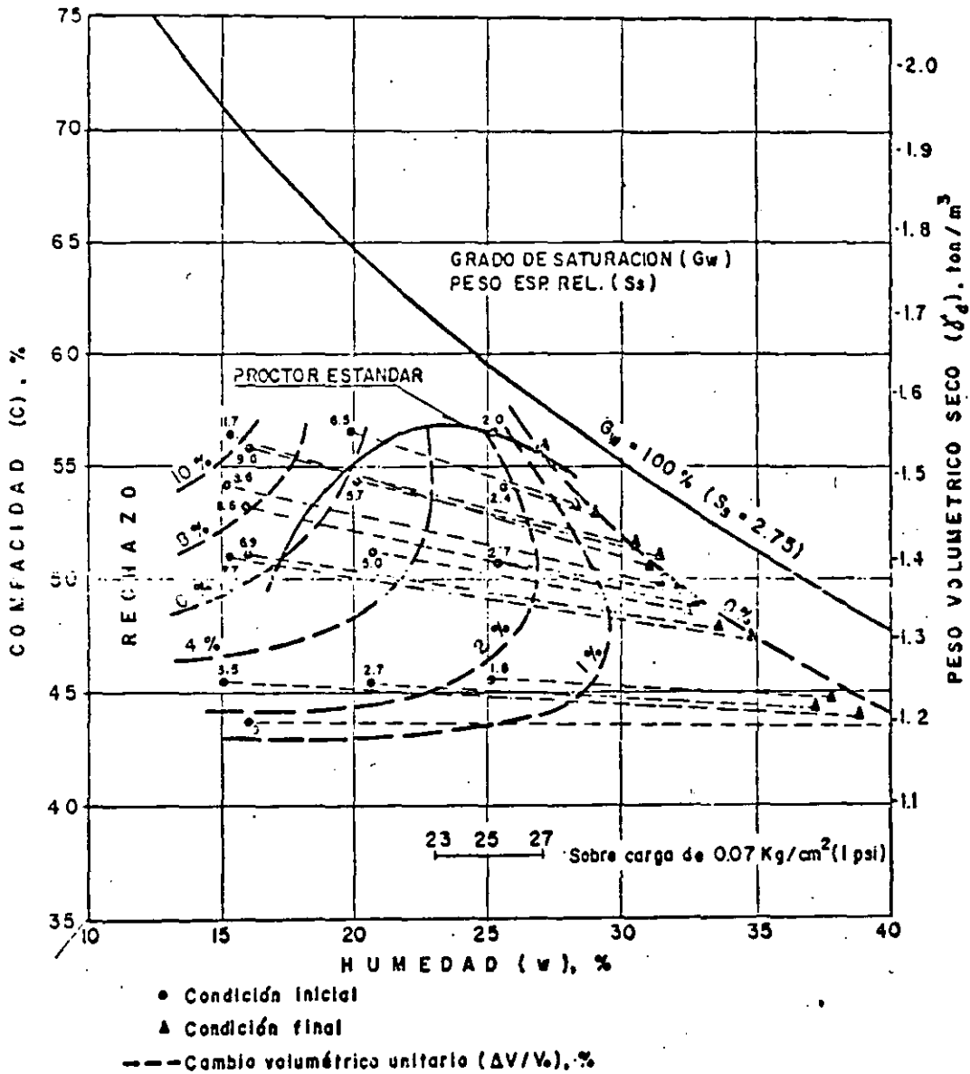
CAMBIOS VOLUMETRICOS EN UN SUELO COMPACTADO (SUELO A) LAMINA 21.- (Ref.12)
