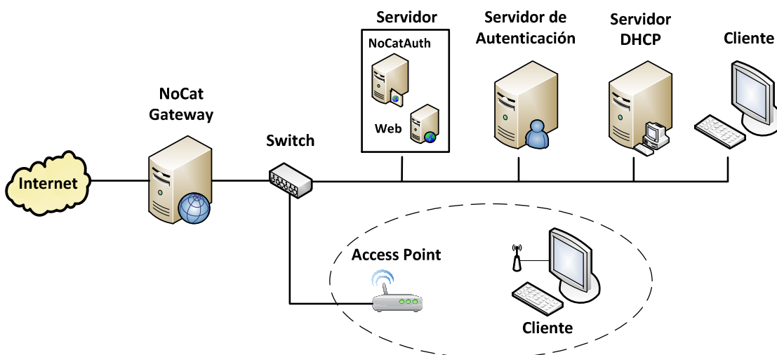
Figura 2.14 Arquitectura resultante (NoCat + servicios necesarios + red WLAN)
