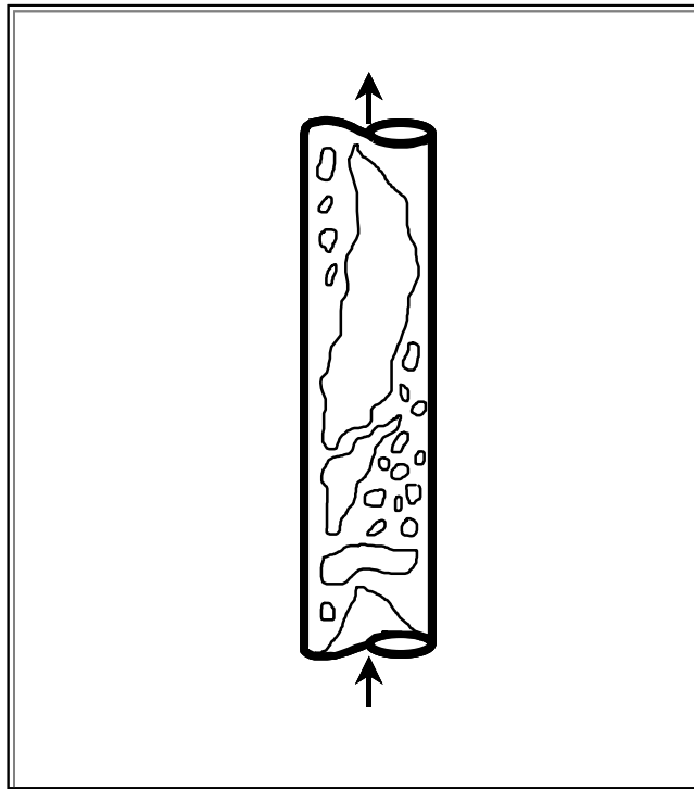
Fig. 2.3 Flujo disperso
