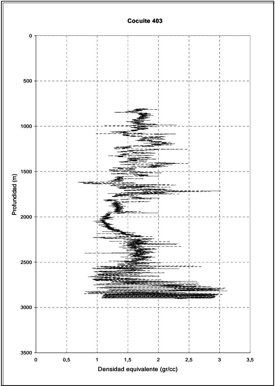
Fig. 4.17 Esfuerzo compresivo uniaxial del pozo Cocuite 403
