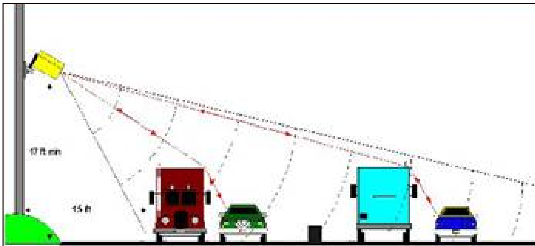
Figura 5.10 Esquema de detección del sensor RTMS
