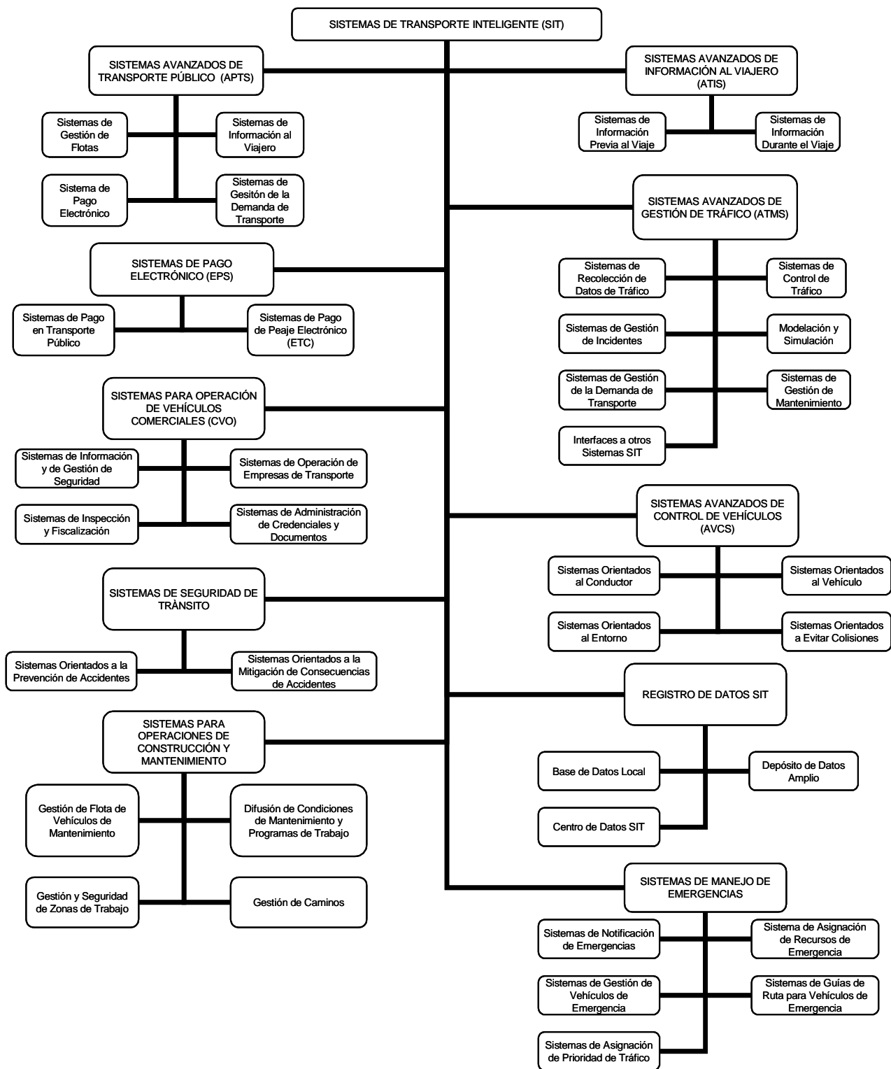
Figura 2.2 Diagrama de estructuración de los servicios que componen los SIT
