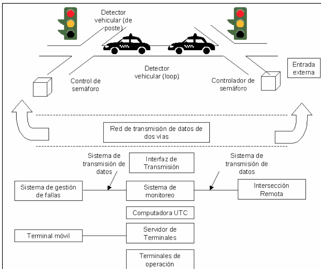
Figura 2.4 Sistema de Control de Tráfico Urbano
