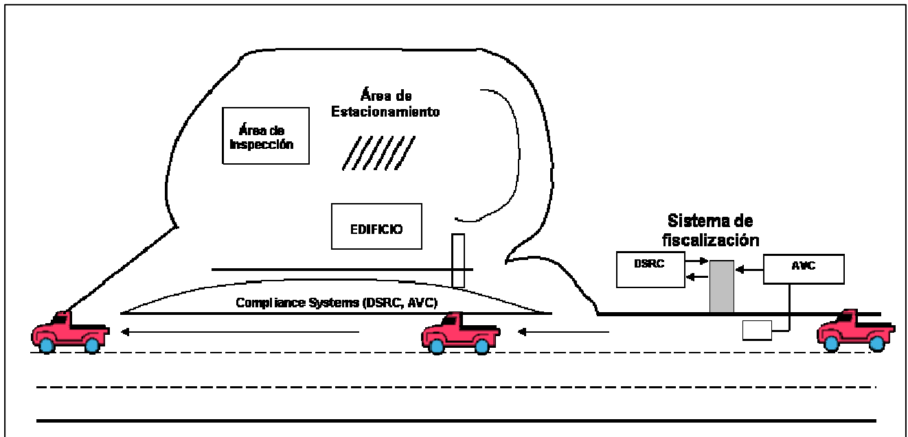
Figura 2.8 Concepto operativo de una estación de inspección
