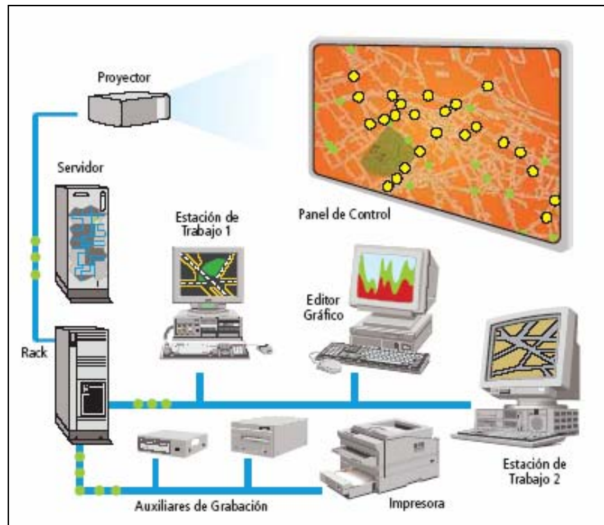
Figura 5.27 Sistemas Centralizados de Control de Semáforos
