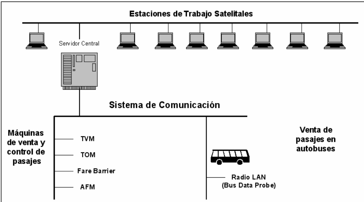
Figura 2.9 Arquitectura típica de un Sistema de Control Central
