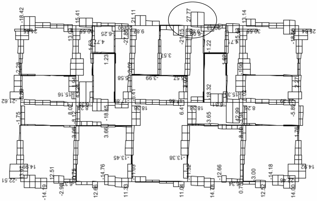
Figura IV.19 Se muestran los cortantes en planta baja. Se observa un comportamiento irregular de los cortantes pero con valores más grandes respecto al modelo con muros integrados. Se observa que el máximo cortante alcanza un valor de 27.77 ton en la zona marcada.
