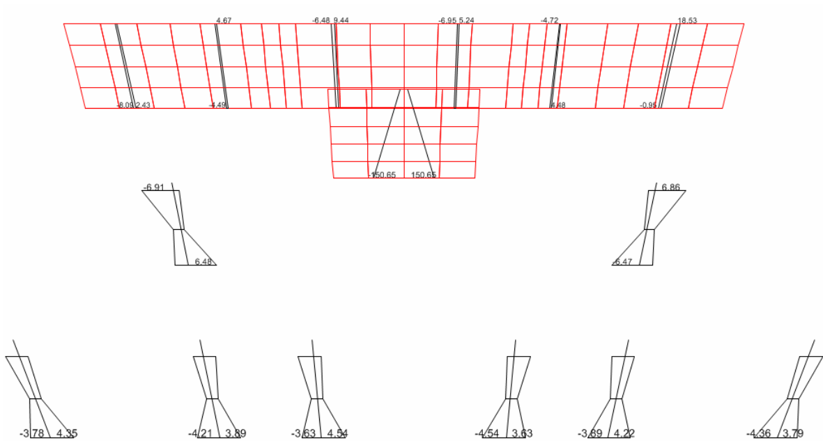
Figura IV.7 Se muestran los momentos en la planta baja. Se nota la gran cantidad de momento que toman los muros de concreto
