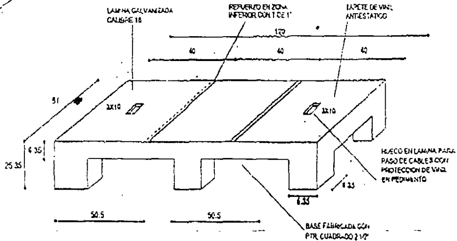
BASE PARA CONTENEDOR
