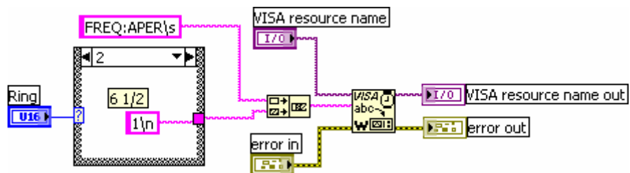
Figura 5.4 Diagrama de bloques del programa aper.vi
