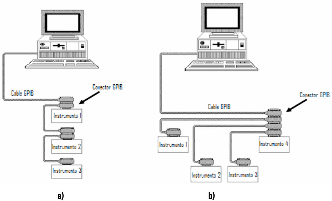
Figura 4.3 Topología de interconexión de un sistema de instrumentación con el bus GPIB. a) Conexión Lineal. b) Conexión estrella.
