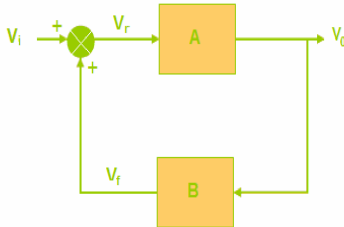
Figura 2.1 Oscilador senoidal
