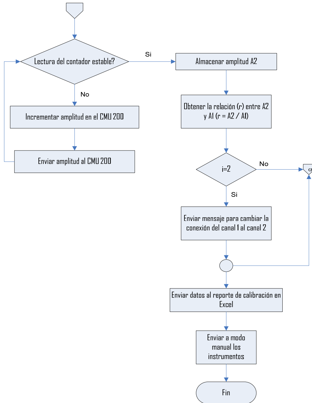
Figura 4.23 Diagrama de flujo para la automatización del procedimiento de verificación del atenuador x10 del contador Agilent 53132A
