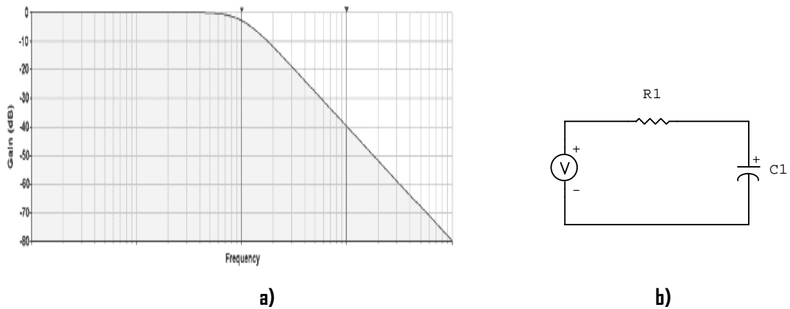
Figura 2.6 Filtro pasabajas. a) Comportamiento de un filtro pasabajas. b) Circuito simple de un filtro pasabajas.
