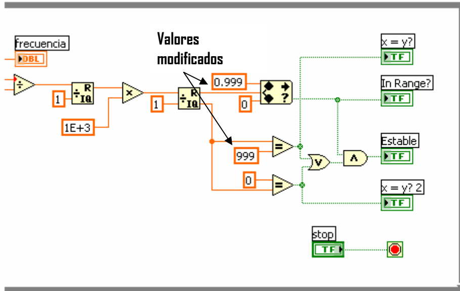
Figura 5.3 Detalle del diagrama de bloques para la detección de dato menos estable para el multímetro HP 34401.
