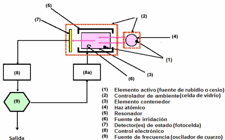
Figura 2.4 Estructura de un oscilador de rubidio o cesio.
