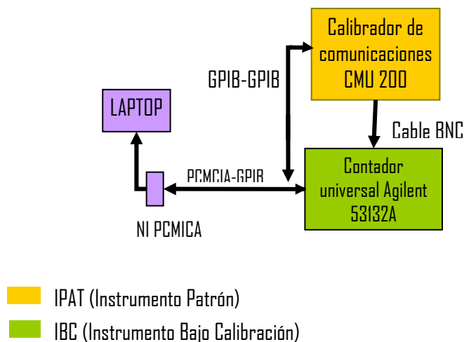
Figura 4.1 Arquitectura de automatización.
