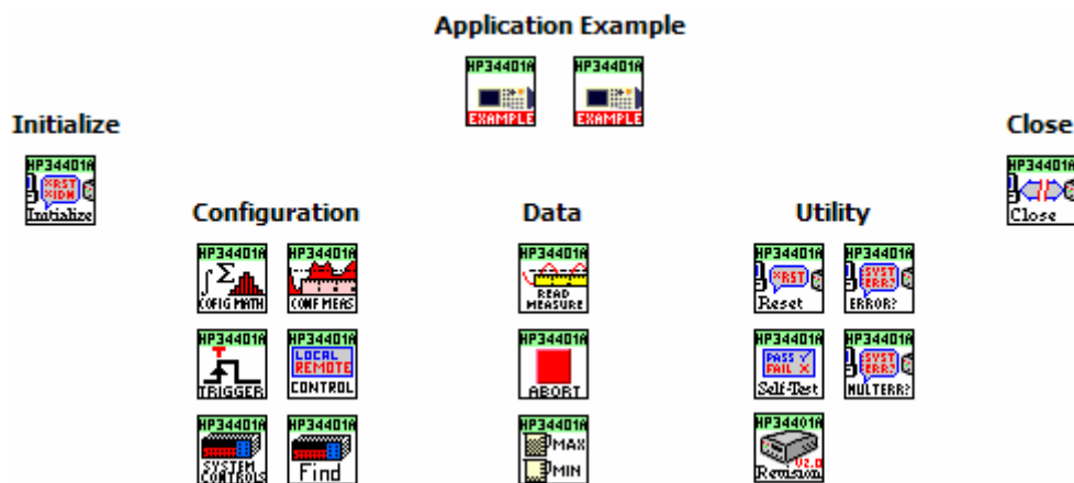
Figura 4.10 Árbol del multímetro Agilent 34401.
