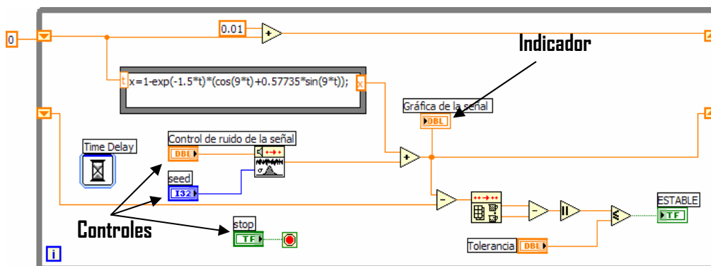
Figura 4.7 Diagrama de bloques del VI de detección de estado estable
