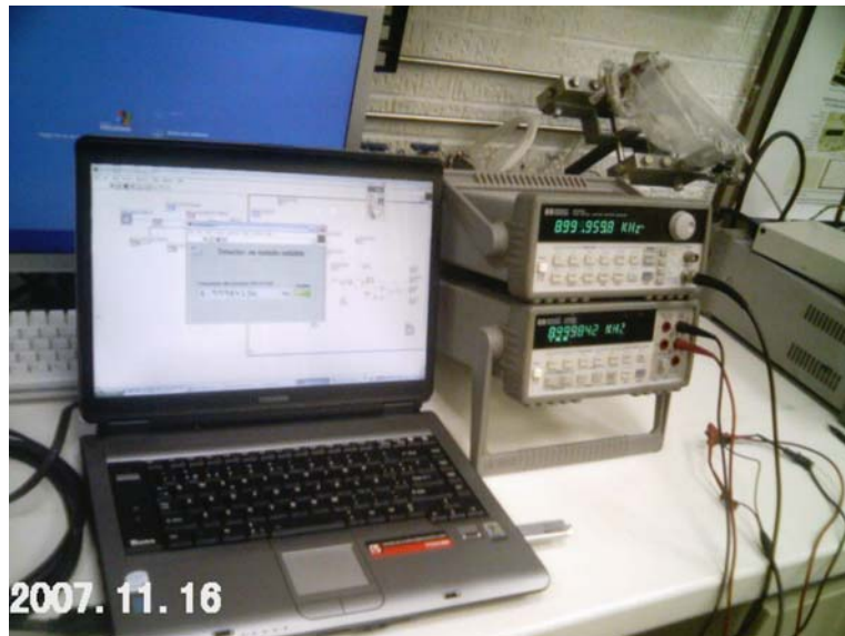
Figura 5.8 Sistema de instrumentación para probar el programa de "Detección de dato estable" en línea.
