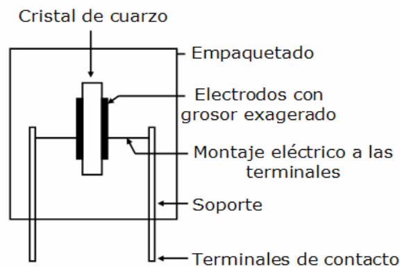
Figura 2.2 Montaje típico de un oscilador de cuarzo.
