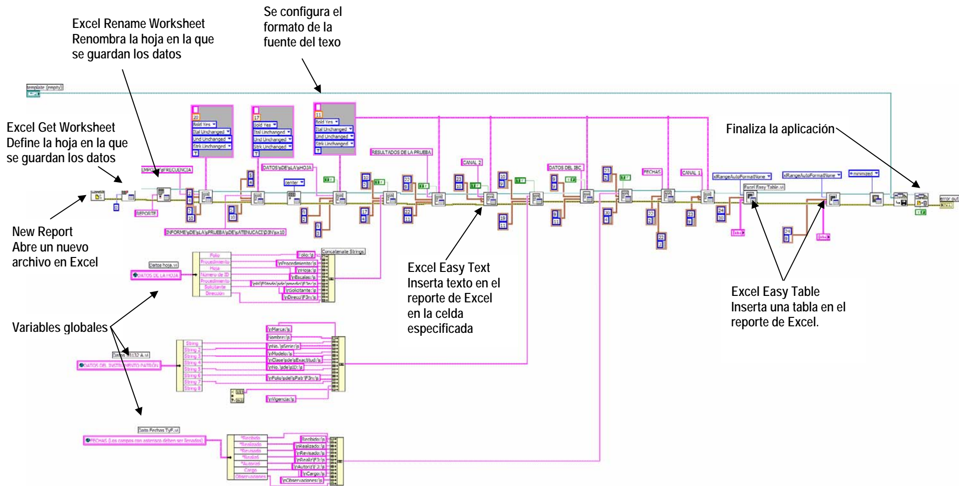
Figura 5.16 Diagrama de bloques del VI que escribe datos a Excel.
