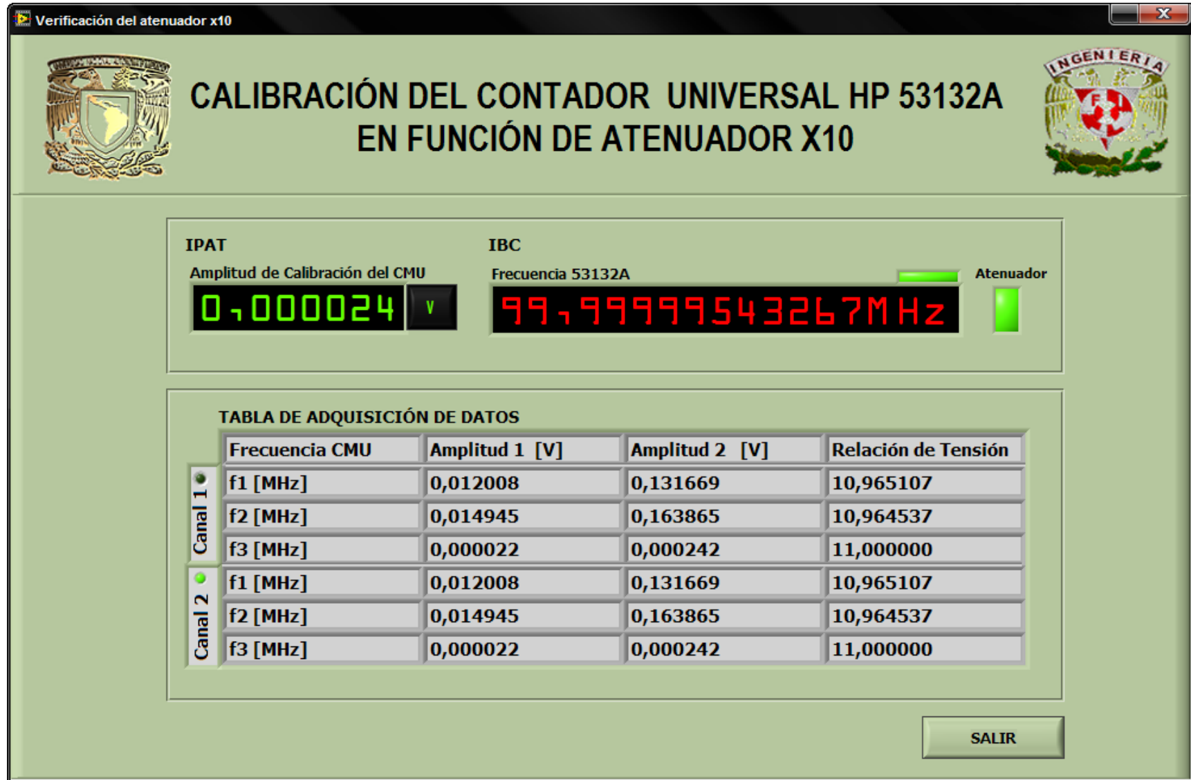
Figura 5.13 Panel frontal del programa de la verificación del atenuador x10 del Agilent 53132A con datos simulados.
