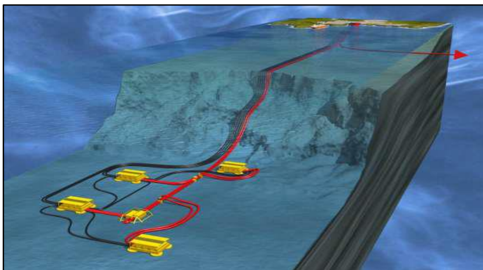
Figura 3.26 - Configuración submarina del campo Ormen Lange (CNH, 2011)
