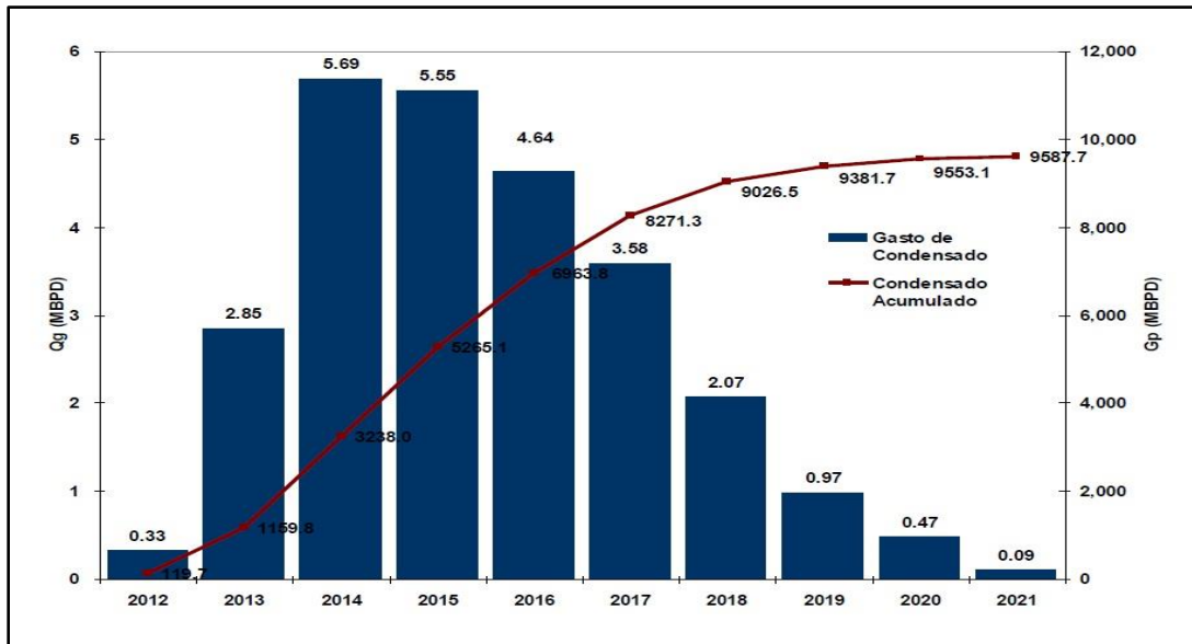
Figura 3.22 - Perfil de producción de condensados a venta (AI-PEP, 2009)
