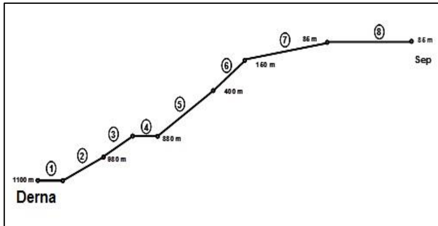
Figura 3.14 - Aproximación del perfil topográfico para el caso Tie-back a la estación de acondicionamiento de gas. (PEP-CNH, 2010)
