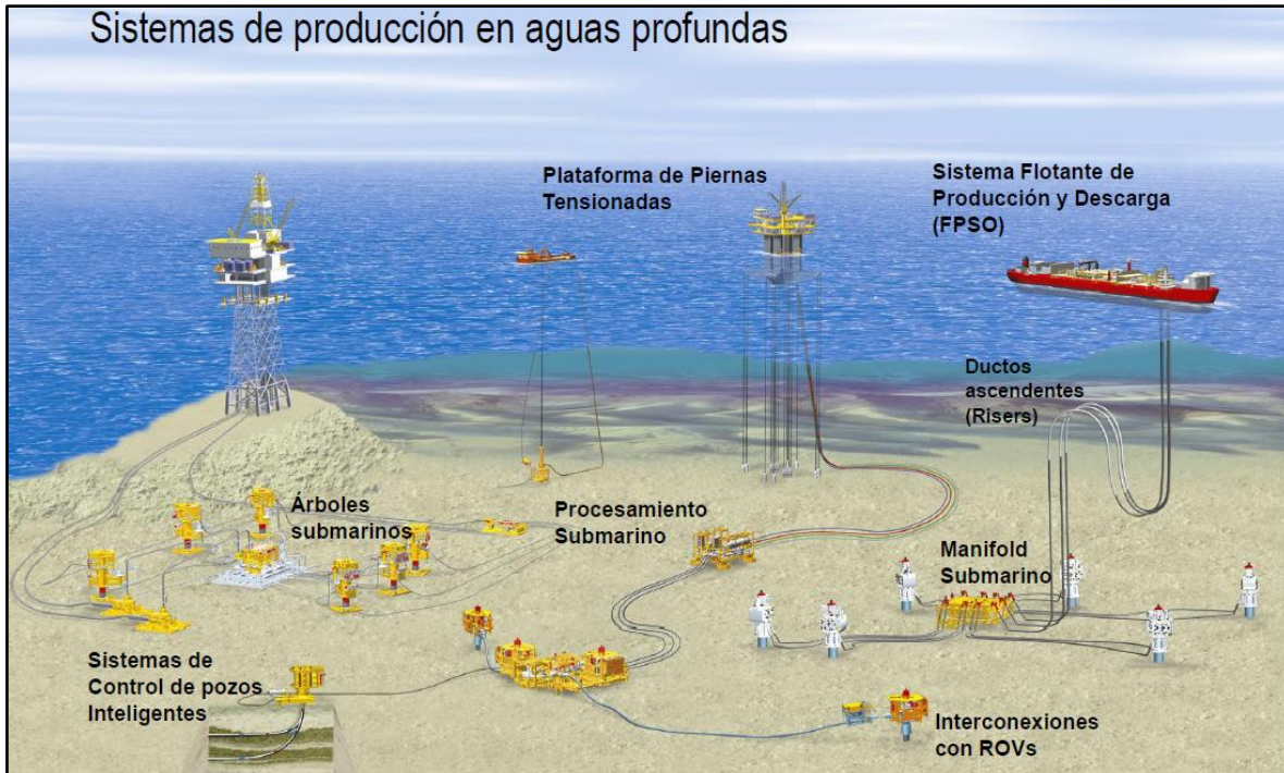
Figura 3.25 - Sistemas de producción en aguas profundas (Heredia Zavoni, 2012)
