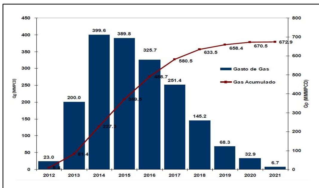
Figura 3.21 - Perfil de producción de gas a venta (AI-PEP, 2009)
