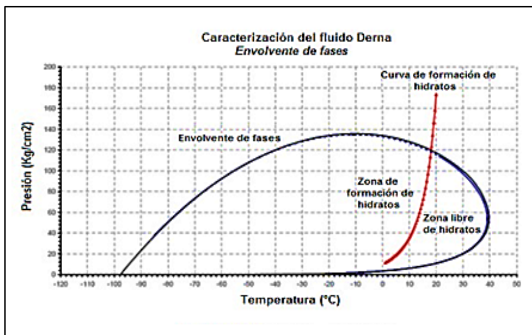
Figura 4.21 - Envlovente de fases y curva de formación de hidratos (PEP-CNH, 2010)
