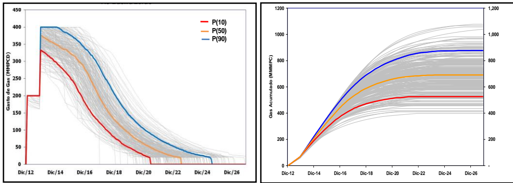
Figura 3.17 - Pronóstico de producción de gas de la alternativa 2 (PEP-CNH, 2010)
