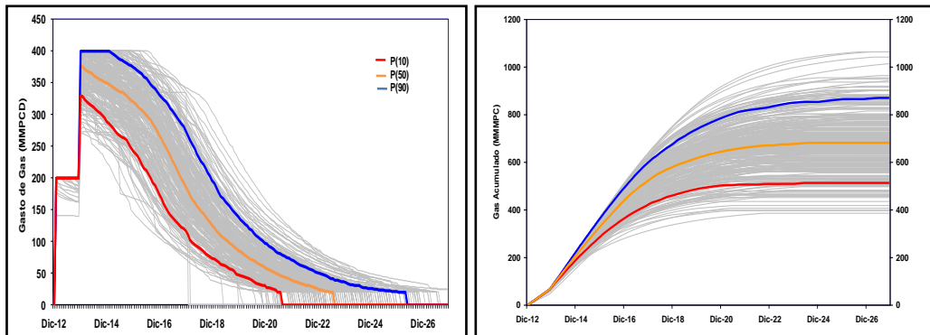
Figura 3.18 - Pronóstico de producción de gas de la alternativa 3 (PEP-CNH, 2010)
