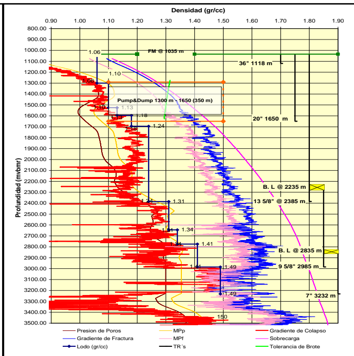
Figura 4.15 - Ventana operativa definida para el diseño del pozo tipo que va a un yacimiento en 5 etapas (PEP-CNH, 2010)
