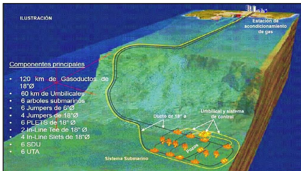
Figura 4.11 - Arquitectura submarina de la ruta de ductos y umbilicales (AI-PEP, 2009)
