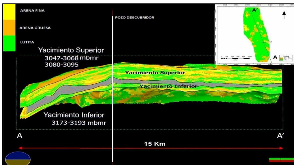
Figura 3.9 - Configuración estructural (AI-PEP, 2009)
