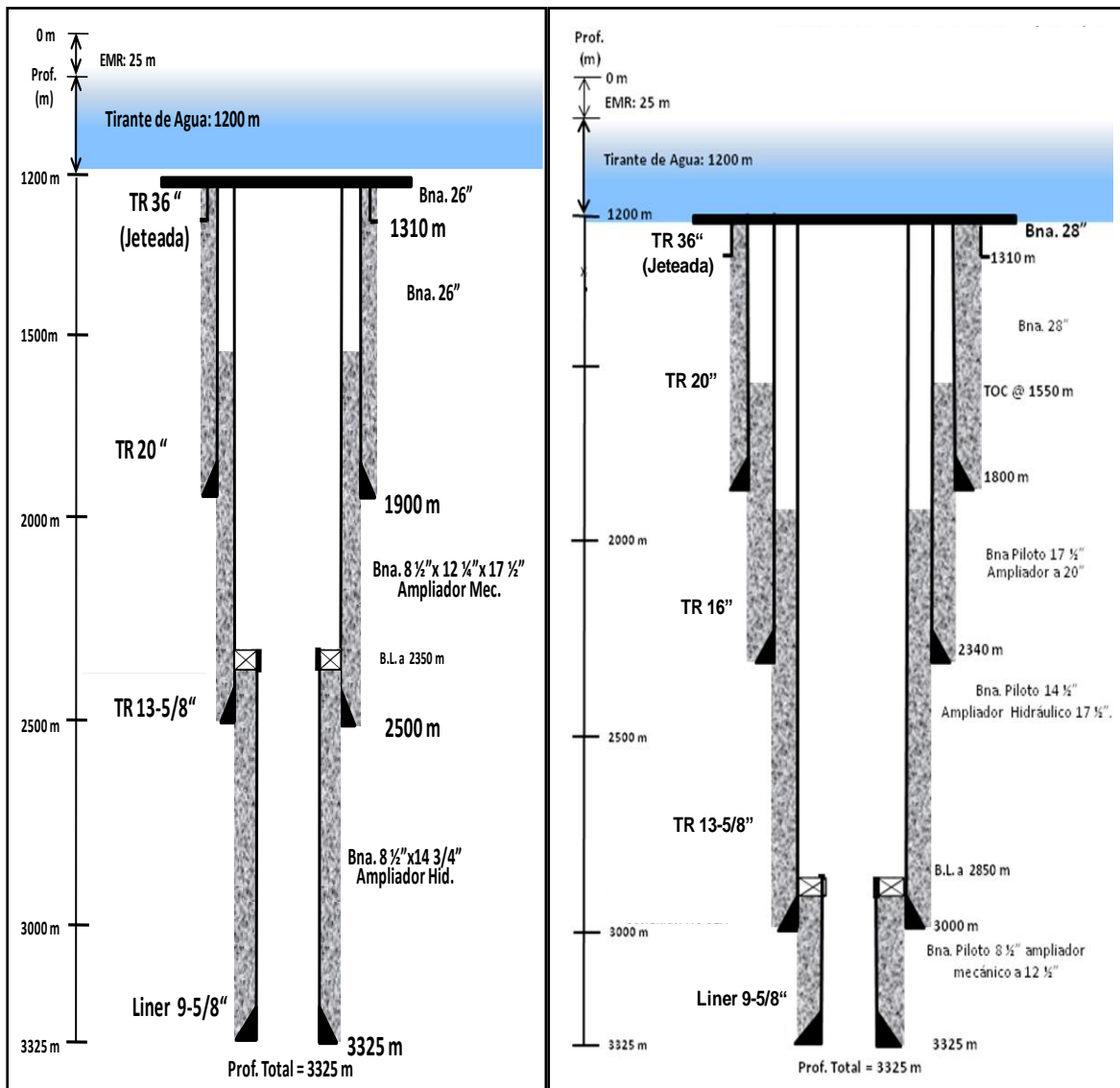
Figura 4.18 - Estado mecánico del pozo tipo que va a dos yacimientos en 4 etapas (PEP-CNH, 2010)
