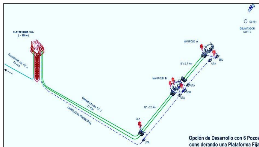
Figura 3.15 - Arreglo de infraestructura de Alternativa C (PEP-CNH, 2010)
