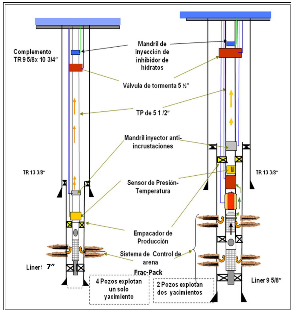
Figura 4.22 - Escenarios para la terminación de los pozos de desarrollo del Campo Derna (PEP-CNH, 2010)
