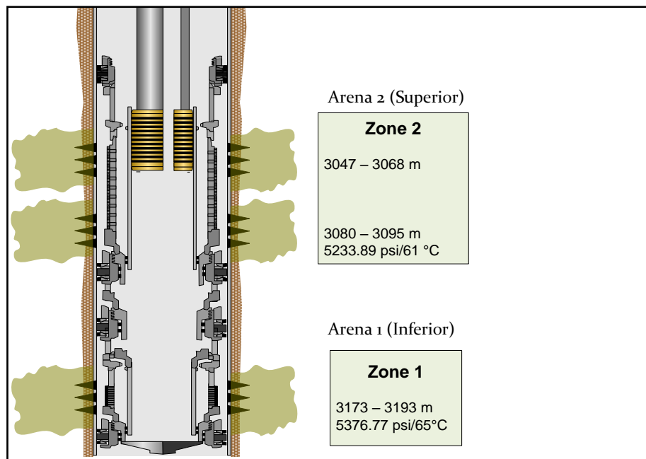
Figura 4.20 - Esquema de sistema de control de arena Frac-Pack (PEP-CNH, 2010)
