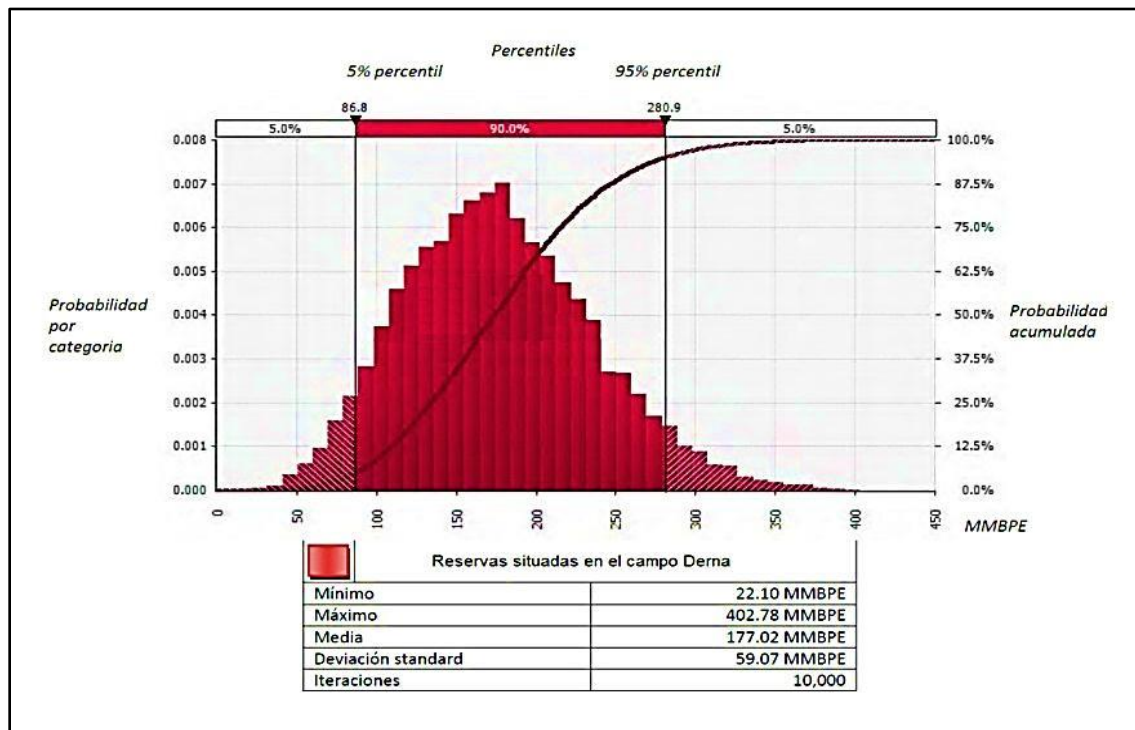
Figura 3.10 - Resultados del modelo de la simulación de reservas ubicadas en el campo Derna (Romero Mata, 2009)
