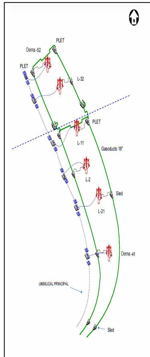
Figura 3.13 - Arreglo de infraestructura submarina de las alternativas A y B (AI-PEP, 2009)
