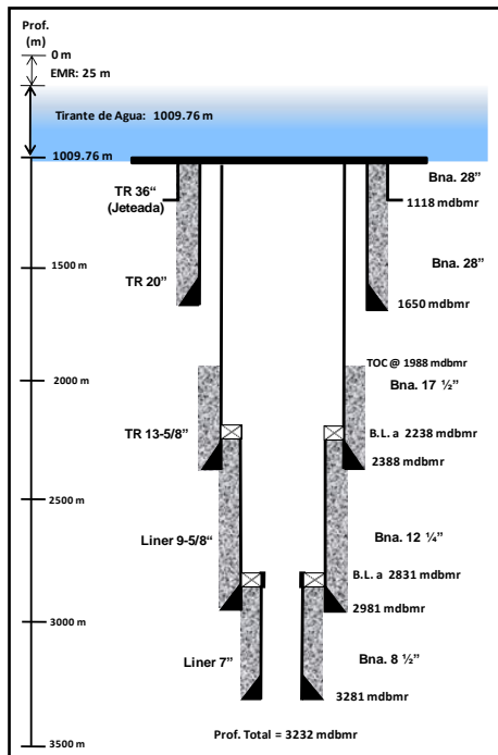
Figura 4.16 - Estado mecánico del pozo tipo que va a un yacimiento en 5 etapas (PEP-CNH, 2010)
