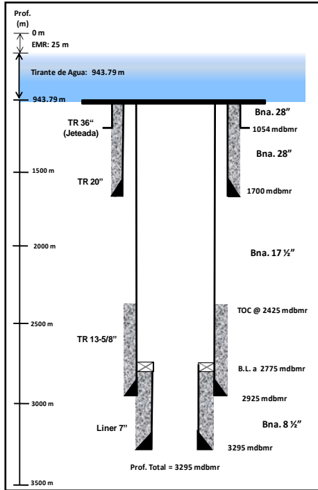
Figura 4.14 - Estado mecánico del pozo tipo que va a un yacimiento en 4 etapas (PEP-CNH, 2010)
