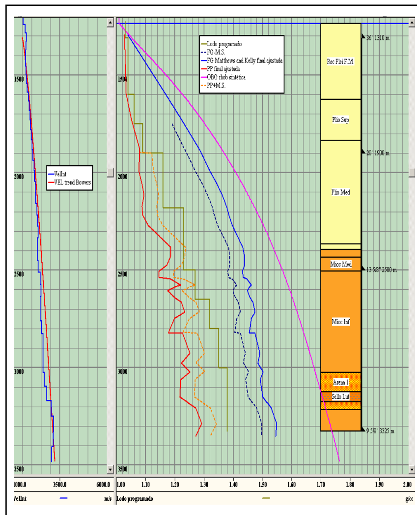
Figura 4.17 - Ventana operativa definida para el diseño de los pozos tipo que van a dos yacimientos (PEP-CNH, 2010)
