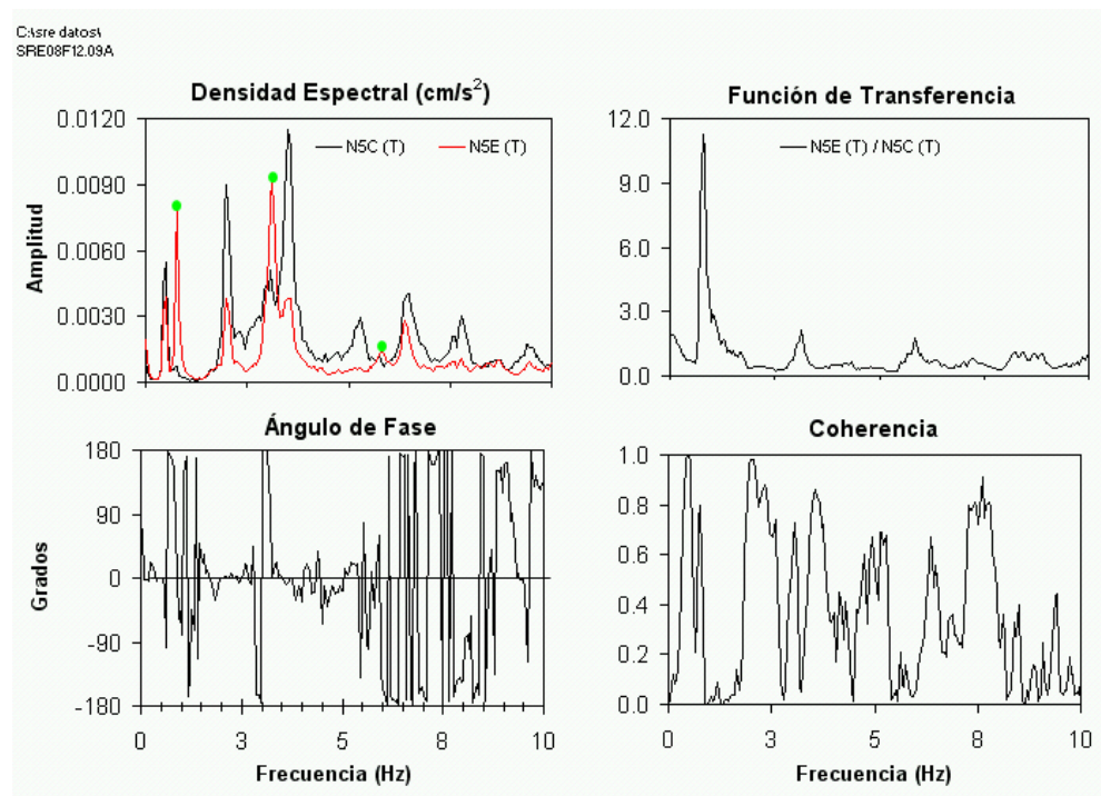
PRUEBA 08. ESPECTROS [N14-E/N14-C] DIRECCIÓN T
