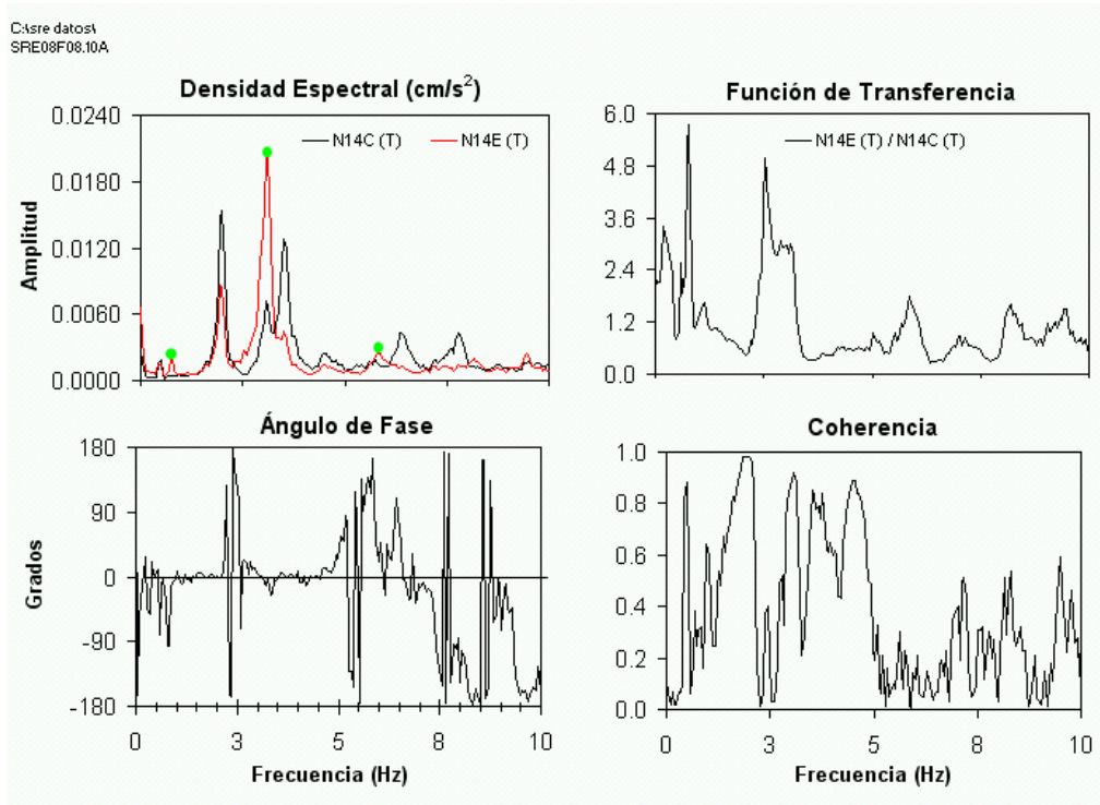
PRUEBA 08. ESPECTROS [N5-E/N5-C] DIRECCIÓN T
