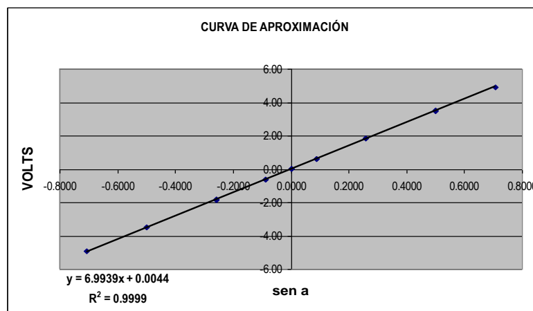
Fig. 2.16 Tabla y gráfica tipo de una calibración estática
