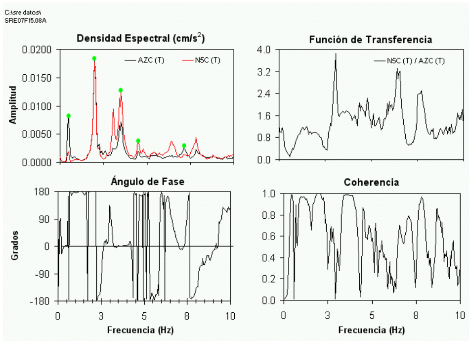
PRUEBA 07. ESPECTROS [AZ-C/N5-C] DIRECCIÓN T
