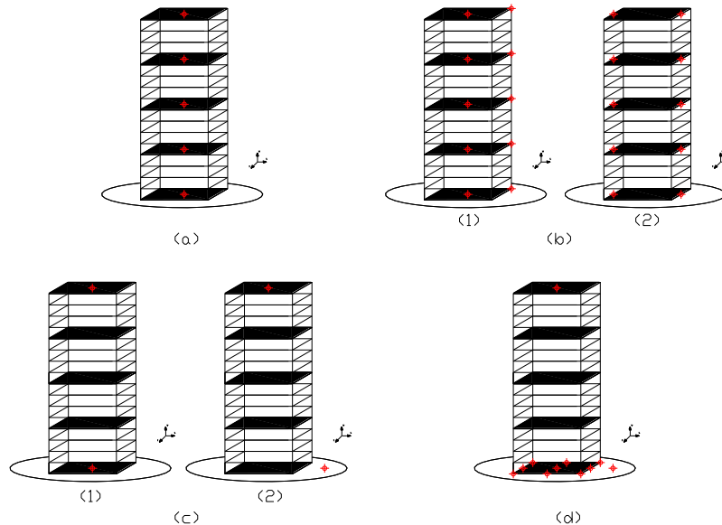
Fig. 2.21 Ubicación de acelerómetros según Tabla 2a
