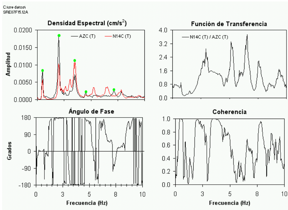
PRUEBA 07. ESPECTROS [AZ-C/N14-C] DIRECCIÓN T
