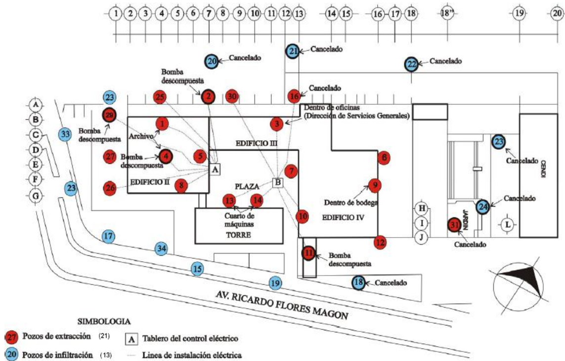
Fig. 1.14 Planta de localización de pozos de extracción e infiltración
