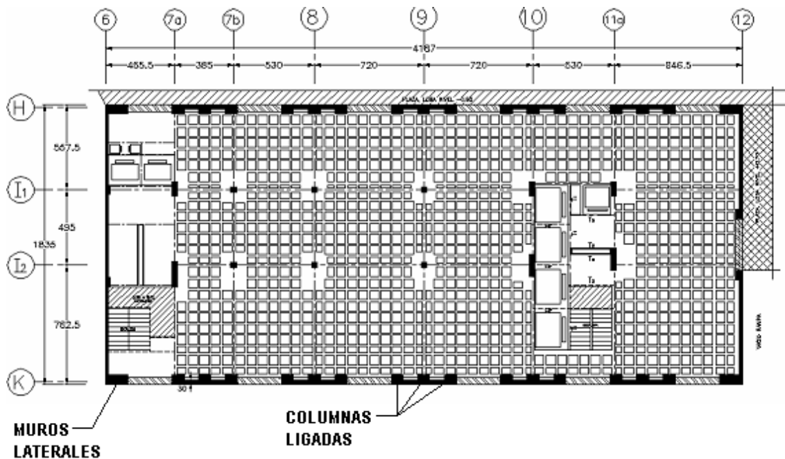
Fig. 1.9 Planta Baja (N+0.70 m)
