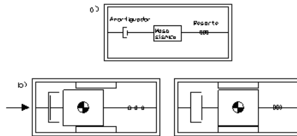
Fig. 2.3 Principio básico de funcionamiento de un transductor de aceleración: (a) Sistema masa-resorte, (b) Desplazamiento de la masa sísmica: con aceleración (izquierda); y con aceleración eliminada (derecha). (LÓPEZ MORALES, 2003)
