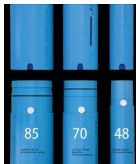
Fig. 4.5 Diámetros de fabricación de la tubería
