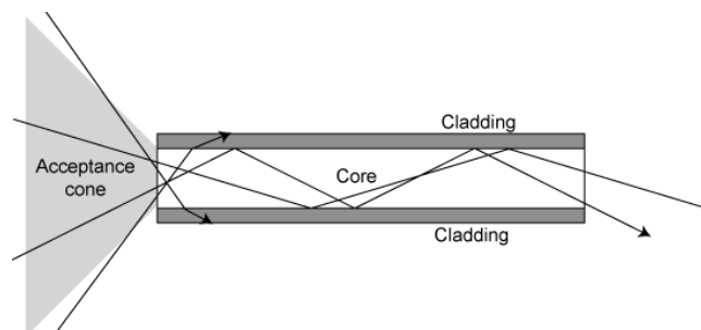
Fig. 4.14 Propagación de la luz a través de una fibra óptica multimodo
