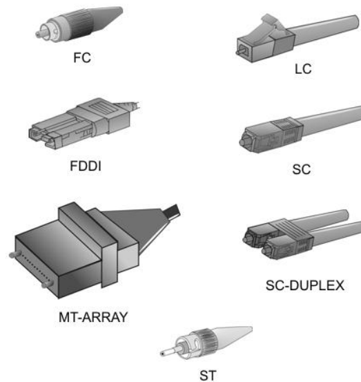
Fig. 4.16 Tipos de conectores de fibra óptica
