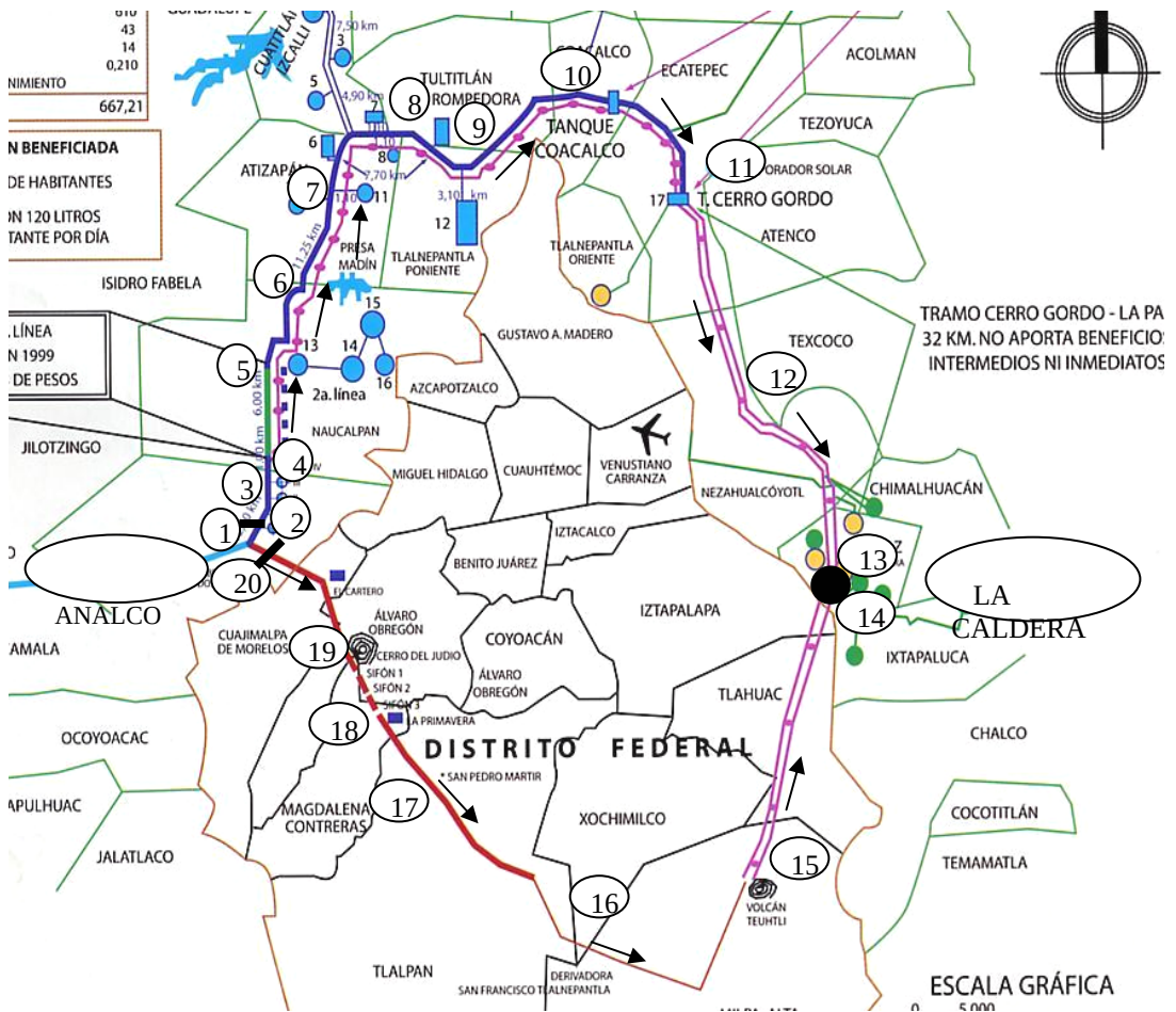
Fig. V.2 ACUAFÉRICO Y MACROCIRCUITO planta (Indicador para perfil)
