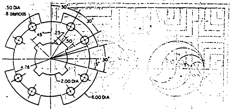
Fig. 2.89 Placa de fricción. Usando el plan A-2, trázelo a lápiz. Omite dimensiones y notas.
