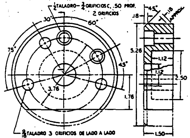
Fig. 2.90 Cubretapa. Usando el plan A-2, dibuje estas vistas a lápiz. Omite dimensiones y notas. Ver 17.8.
