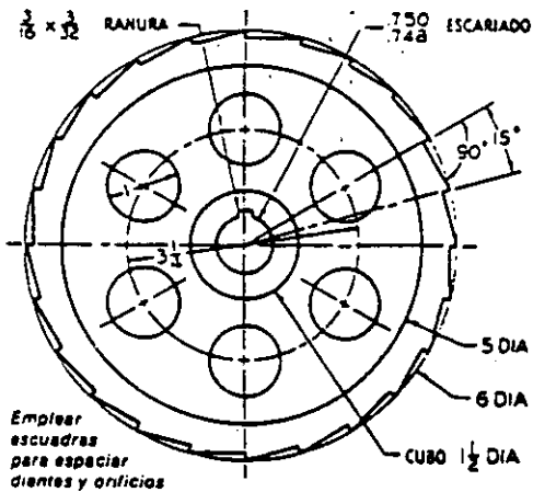
Fig. 2.93 Rueda dentada o de trinqueta. Empleando el plan A-2, dibuje a lápiz. Omite dimensiones y notas.
