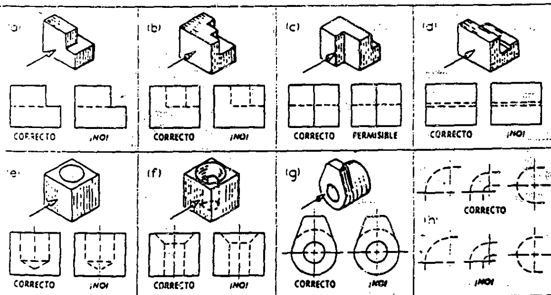
Fig. 5.43 Prácticas relativas a las líneas ocultas.
