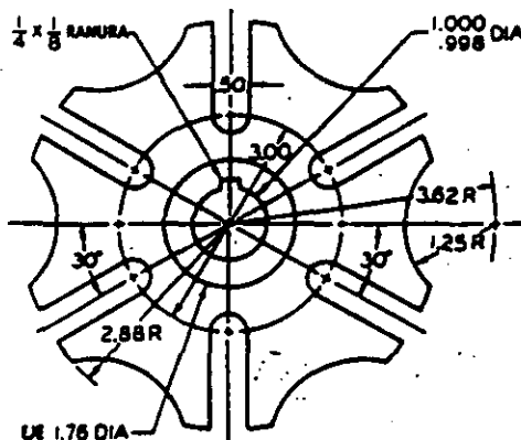
Fig. 2.91 Eje de levas tipo Ginebra. Empleando el plan A-2, dibuje a lápiz. Omite las dimensiones y las notas.
