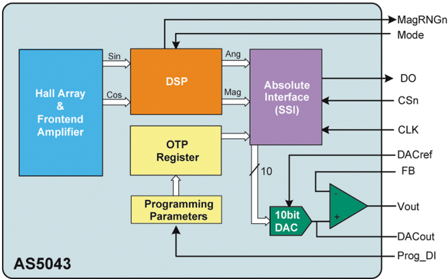
Figura A.16 Diagrama de bloques del codificador AS5043.
