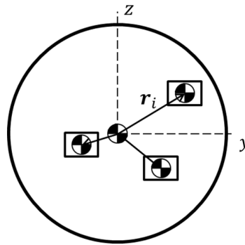
Figura 2.12 Esquema simplificado de un robot con arreglo de masas móviles.
