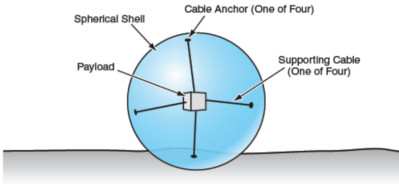
Figura 2.11 Diseño propuesto por J. Lux [15].
