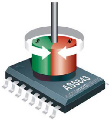
Figura A.15 Arreglo del codificador AS5043 e imán.
