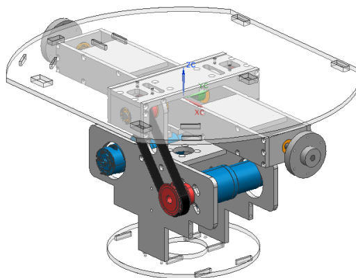
Figura 4.7 Péndulo con placas para montaje de componentes y dispositivos.
