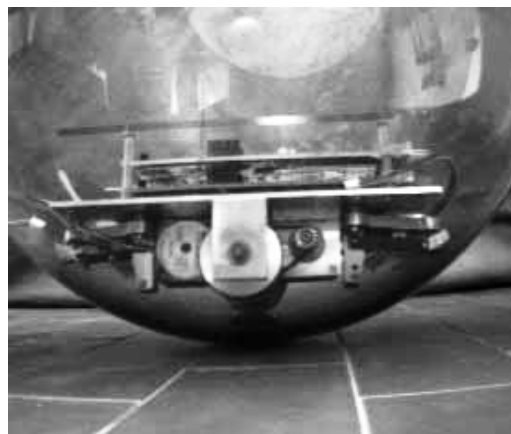
Figura 2.3 Diseño tipo “rueda de hámster” de Bicchi et al. [8].
