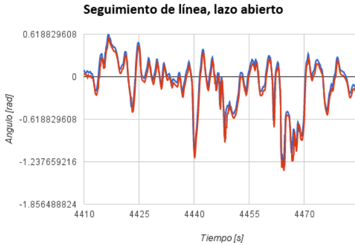
Figura 5.6 Roll del eje diametral, sin control, al moverse la esfera hacia “delante”.
