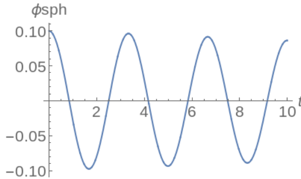
Figura 5.2 Comportamiento de \phi_{esf} sin control, por 10 s.
