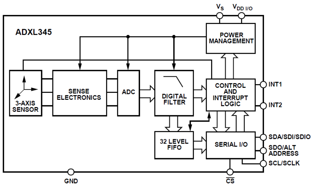
Figura A.19 Diagrama de bloques del acelerómetro ADXL345.
