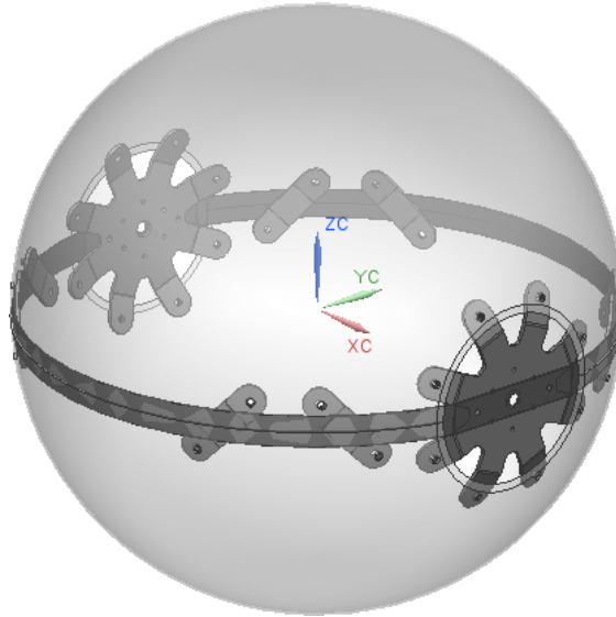
Figura 4.1 Esfera con placas de unión y anillo.
