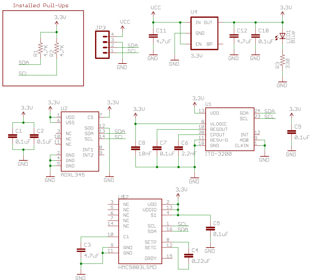
Figura A.18 Diagrama esquemático de la IMU 9DOF Sensor Stick, versión 13.
