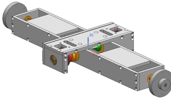
Figura 4.5 Estructura superior del péndulo.
