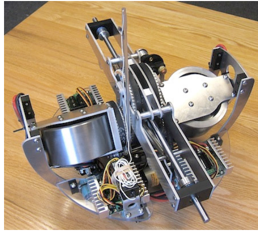
Figura 2.16 Ensamble de los CMG del prototipo de G. Schroll [19].
