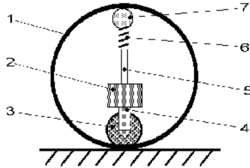
Figura 2.4 Diseño propuesto por A. Halme et ál. [10]
