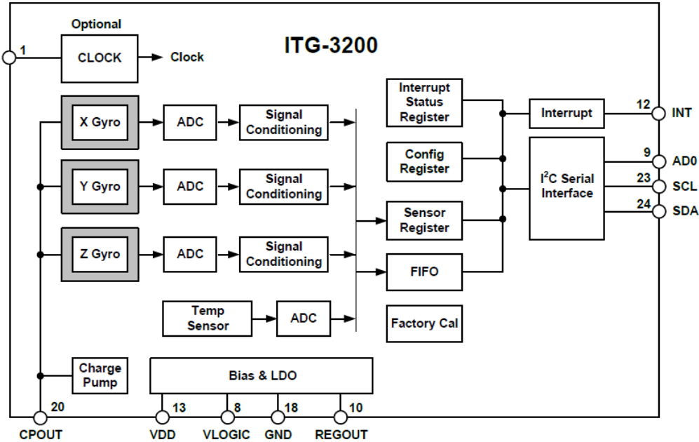
Figura A.20 Diagrama de bloques del giroscopio ITG3200.
