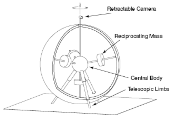
Figura 2.9 Robot Spherobot, desarrollado por R. Mukherjee et ál. [16].
