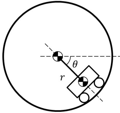
Figura 2.6 Diagrama simplificado de un robot esférico con IDU.
