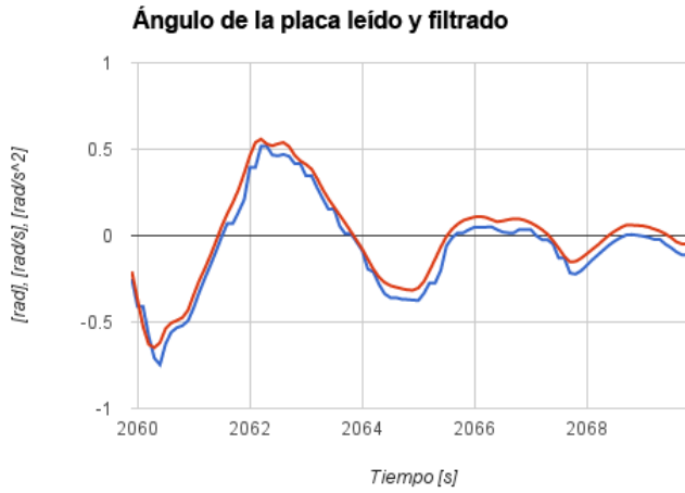
Figura 5.3 Roll de la placa, filtrado y sin filtrar, por 10 s.
