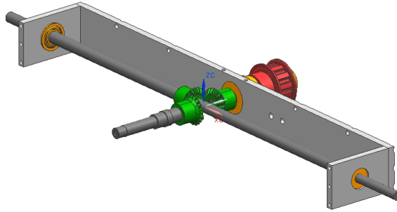
Figura 4.3 Arreglo diferencial de engranes.
