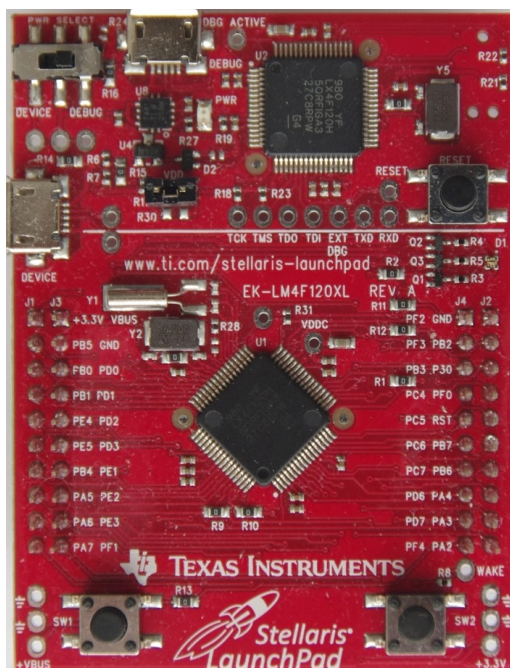
Figura A.23 Tarjeta de desarrollo Stellaris LMF4120.
