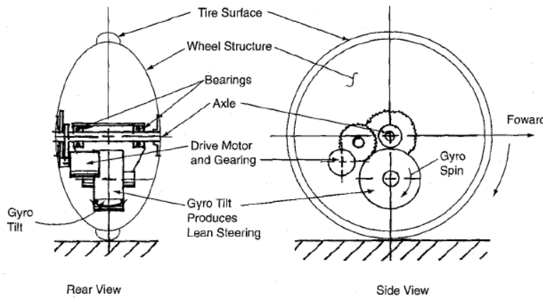
Figura 2.13 Robot Gyrover, desarrollado por H. Brown y Y. Xu [9].
