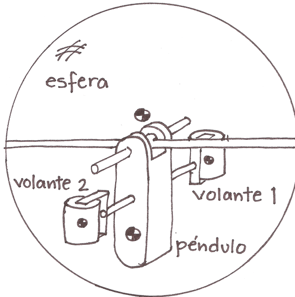
Figura 3.1 Diagrama del sistema del robot.
