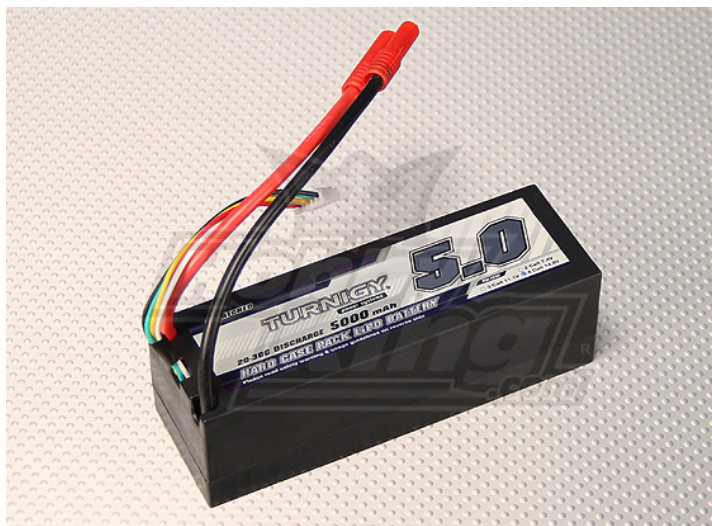
Figura A.14 Batería Hardcase Pack LiPo 4S 5000 mA·h.
