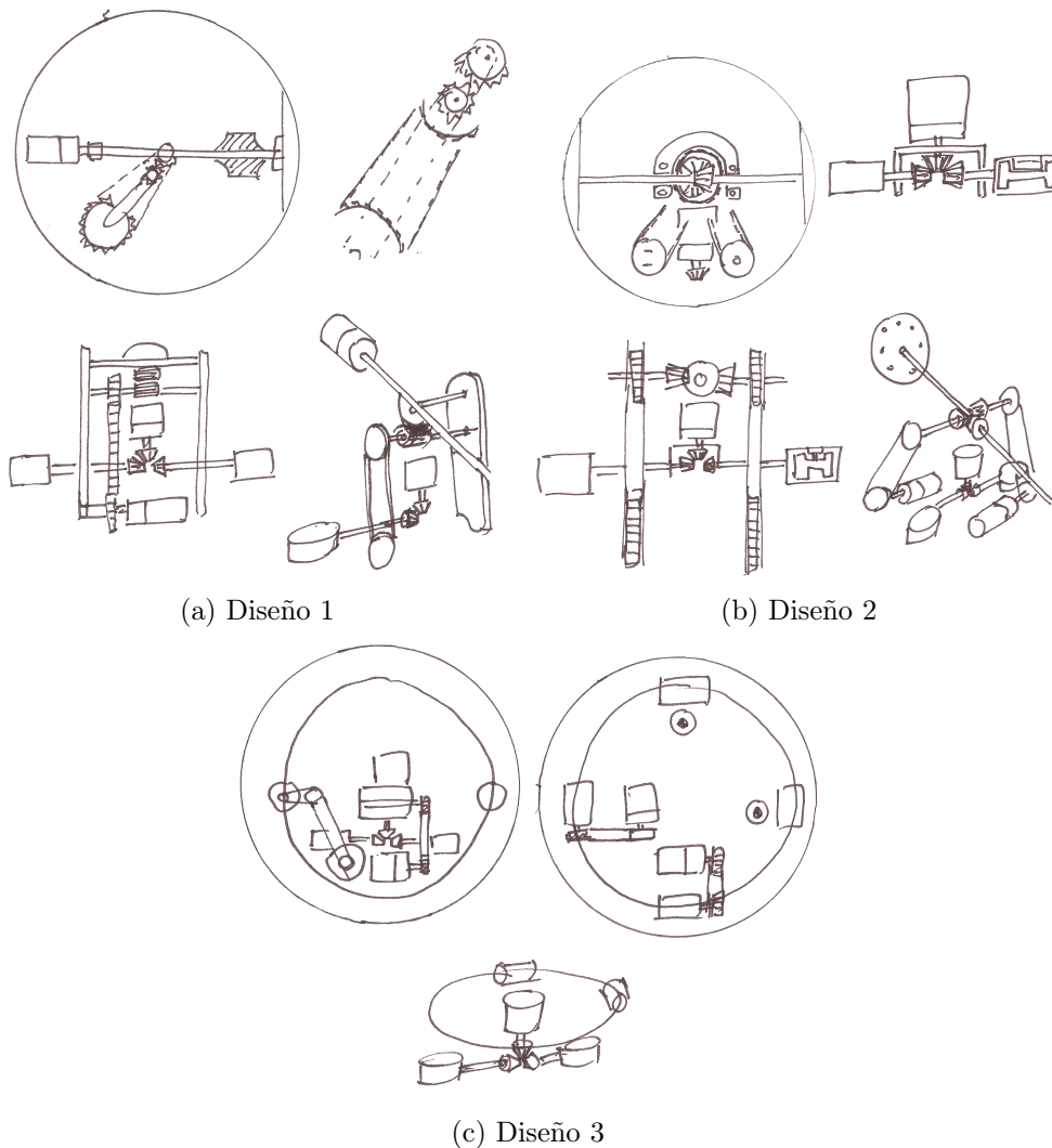
Figura 2.19 Bocetos de las propuestas de diseño mecánico.
