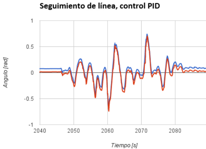
Figura 5.7 Roll del eje diametral, con control PID, al moverse la esfera hacia “delante”.
