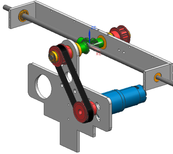
Figura 4.4 Transmisión por bandas dentadas de los motores al péndulo.
