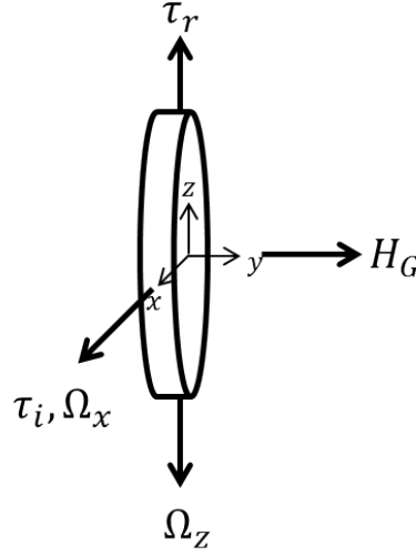
Figura 2.14 Diagrama de un volante de inercia vertical.
