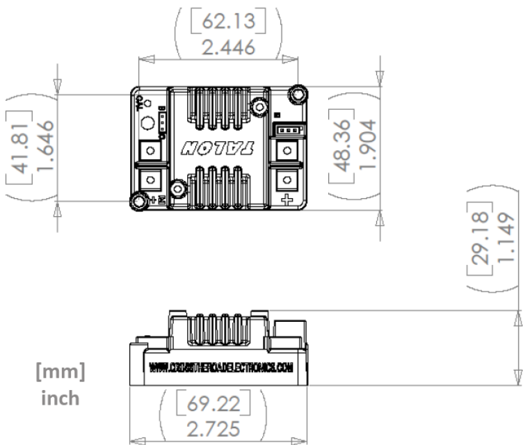
Figura A.12 Dimensiones del puente H Talon SR.
