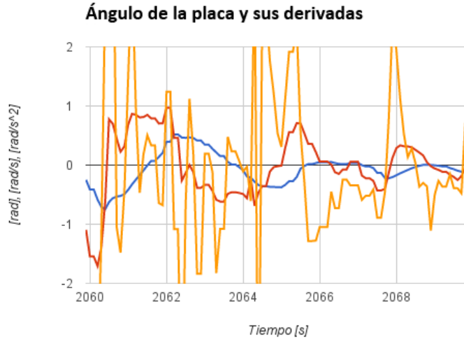
Figura 5.5 Roll de la placa, filtrado y sus primeras dos derivadas, por 10 s.
