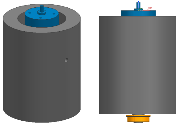
Figura 4.8 Volantes con motor brushless y rodamiento de apoyo
