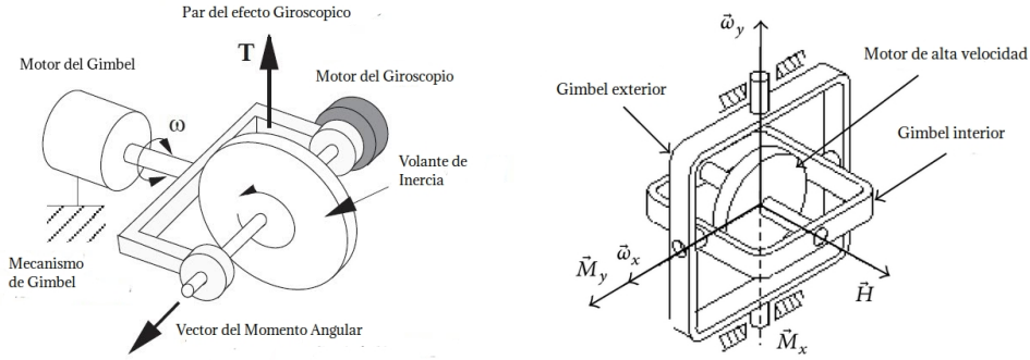
Figura 2.15 CMG simple (izquierda) y CMG doble (derecha).
