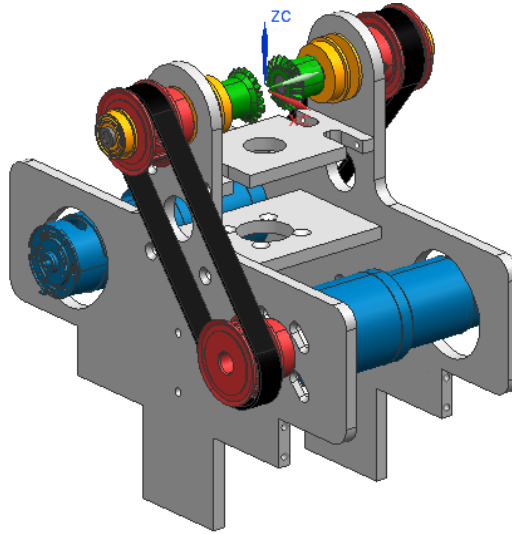
Figura 4.6 Estructura inferior del péndulo.
