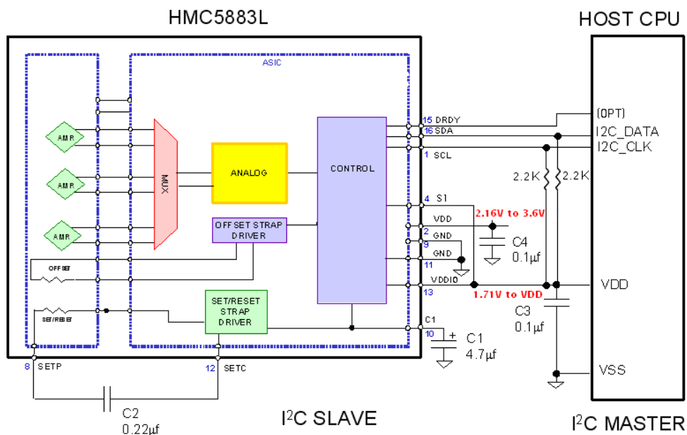
Figura A.21 Diagrama de bloques del magnetómetro HMC5883L.
