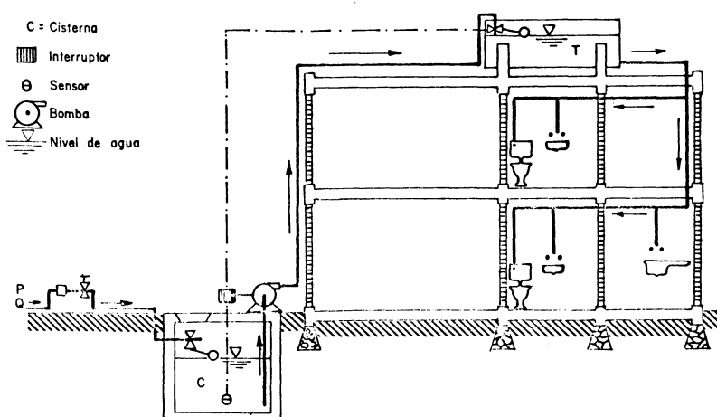
SISTEMA DE DISTRIBUCION DE AGUA CON CISTERNA, SISTEMA DE BOMBEO Y TANQUE ELEVADO
