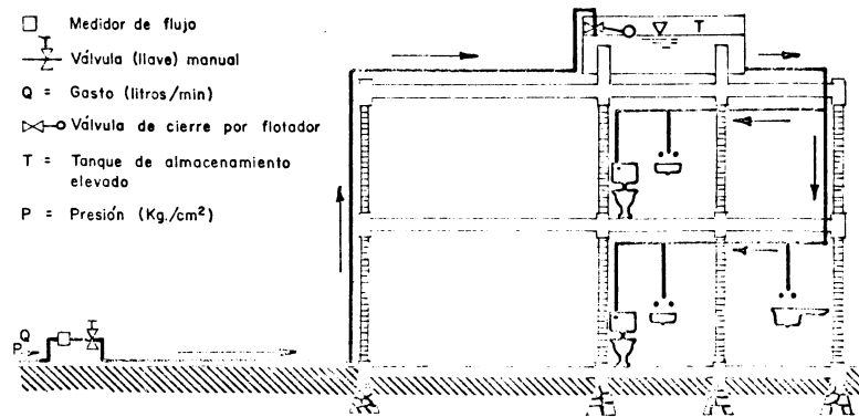
SISTEMA DE DISTRIBUCION DE AGUA CON TANQUE ELEVADO
