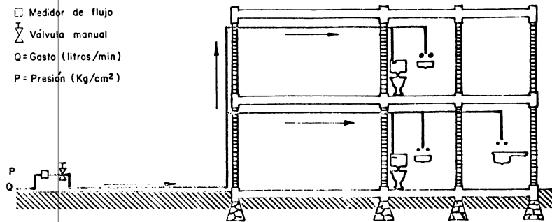
SISTEMA DE DISTRIBUCION DE AGUA EN UNA CASA HABITACION
