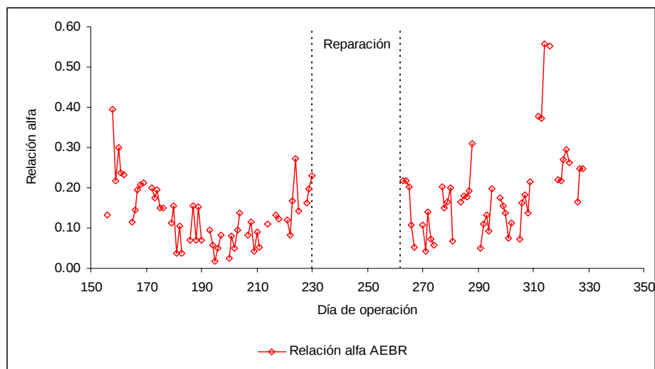
Figura 4.20. Evolución de la relación \alpha en el reactor AEBR
