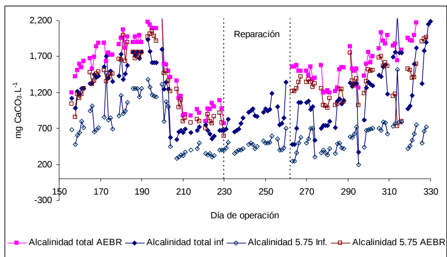
Figura 4.19. Alcalinidad total y a pH 5.75 en el reactor AEHR
