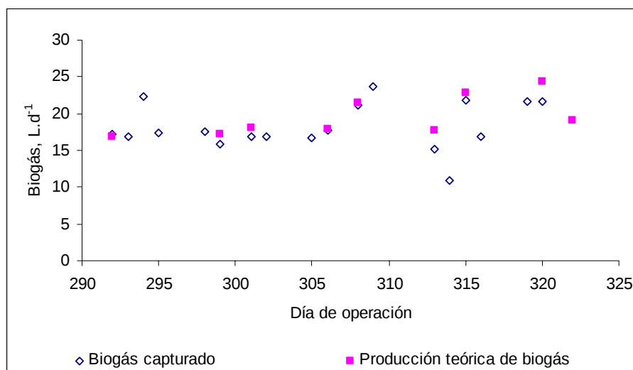
Figura 4.10. Producción de biogás. Reactor AEHR
