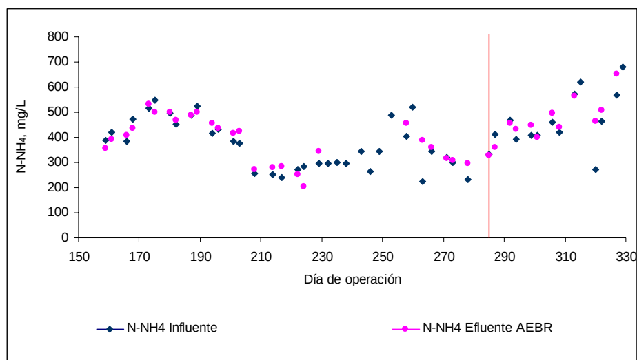
Figura 4.12. Concentraciones de \text{N-NH}_4^+ en el influente y efluente del reactor AEER
