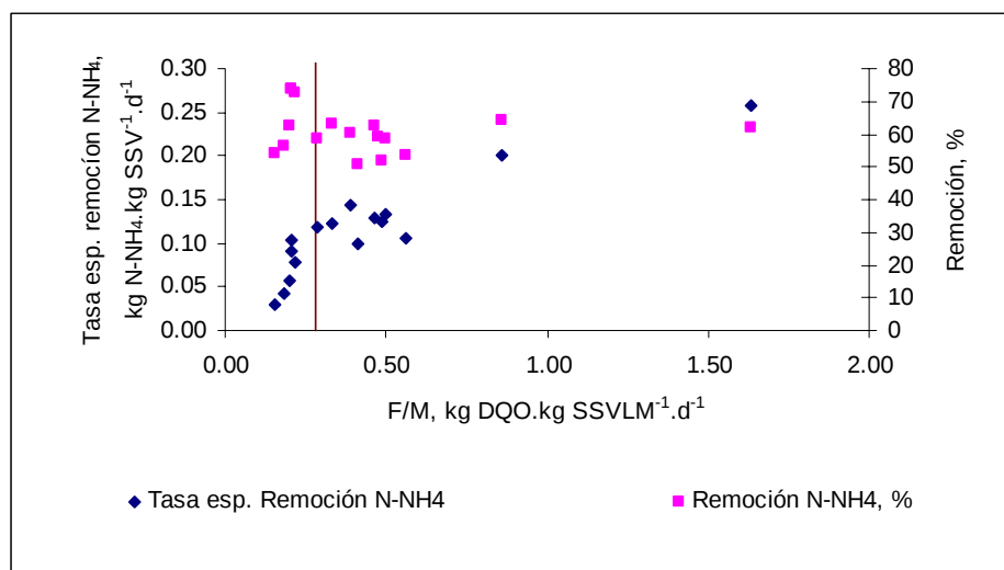
Figura 4.49. Variación en la tasa específica de remoción de \text{N-NH}_4 en los reactores de LA con respecto a la relación F/M
