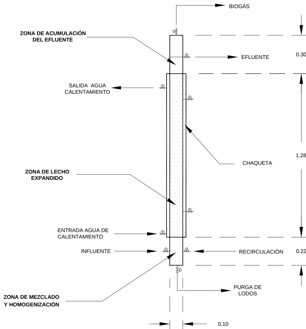
Figura 3.5. Esquema del reactor AEER
