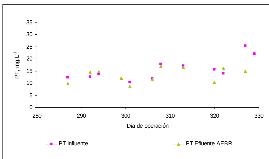
Figura 4.14. Concentración de PT en el influente y efluente del reactor AEBR
