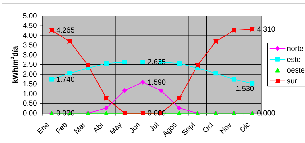
Figura 4.14 Irradiancia incidente en la fachada oeste del edificio protegida con parteso de 90° en Ecatepec de Morelos, Estado de México
