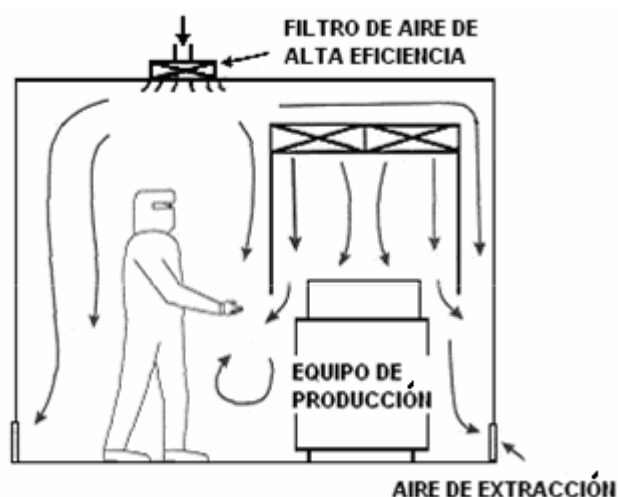
Figura 2.16 Cuarto limpio con flujo mezclado y con protección para áreas de proceso crítico
