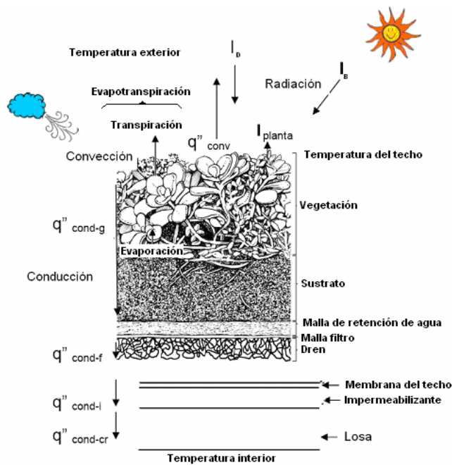
Figura 2.31 Factores que influyen en las ganancias de calor en los techos verdes
