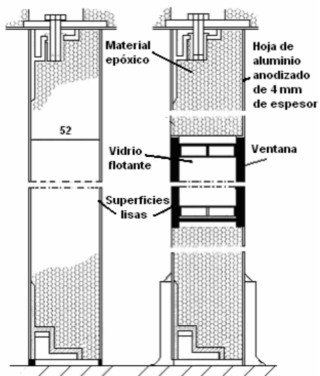
Figura 2.22 Muros prefabricados
