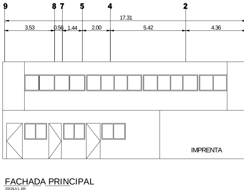
Figura 4.17 Fachada principal del edificio
