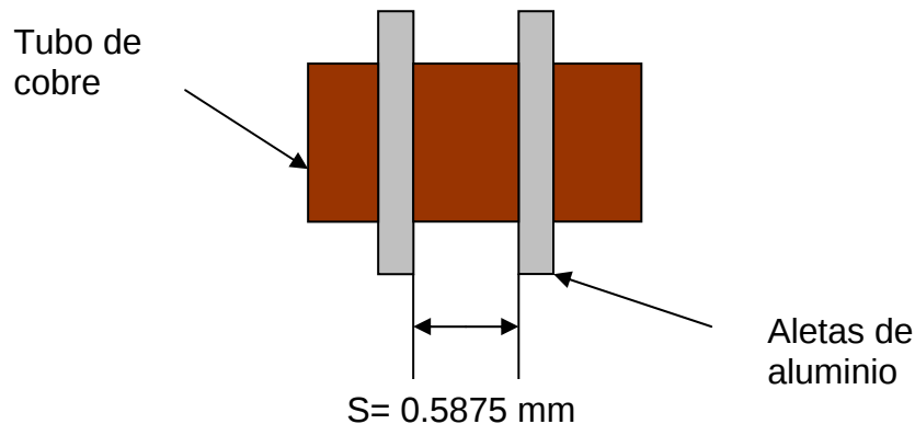
Figura 4.24 Espaciamiento entre aletas
