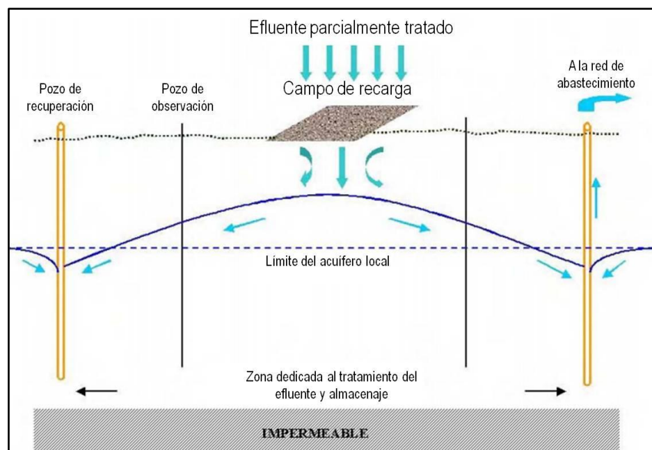
Figura 8. Esquema del Sistema de Tratamiento Suelo-Acuífero.
