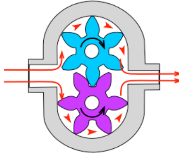
Figura 3.2. Bomba de engranes externos
