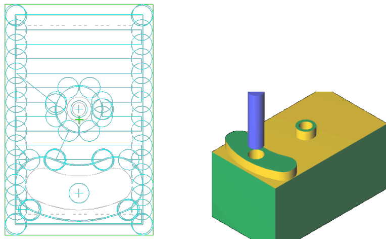
Figura 6.19. Patrón de corte generado y simulación del maquinado para el cilindro.
