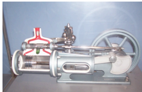
Figura 6.1. Motor de vapor de cilindro fijo.
