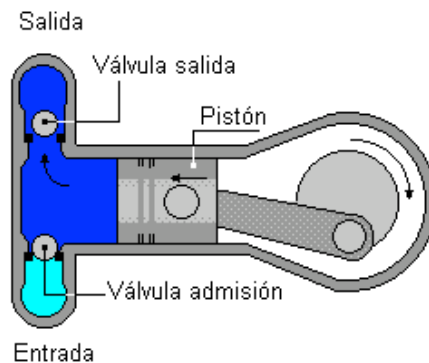
Figura 3.1. Bomba reciprocante
