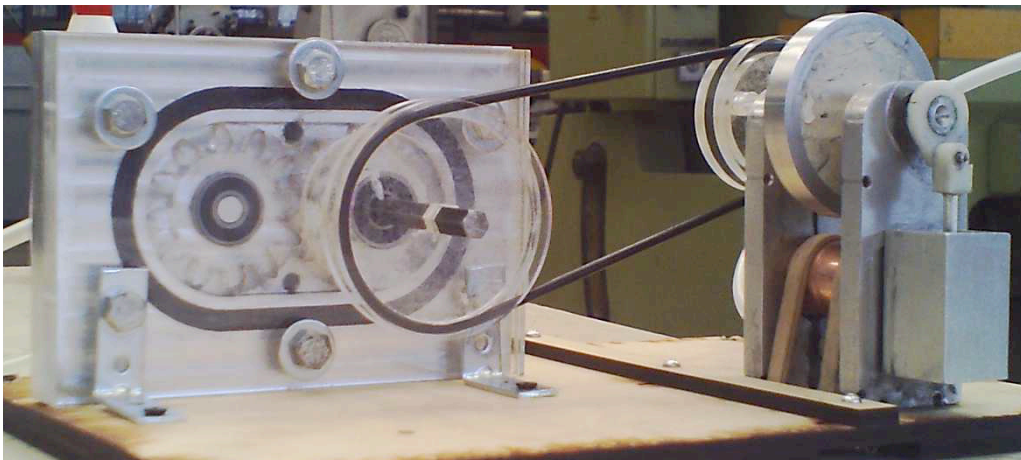
Figura 7.2. Conjunto motor-bomba
