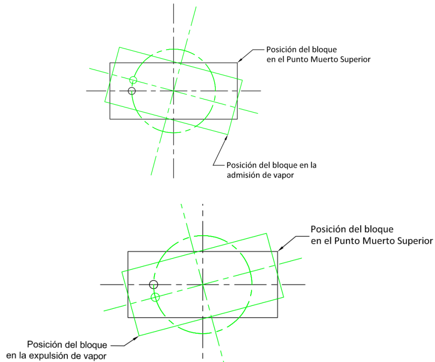
Figura 6.30. Oscilación del bloque
