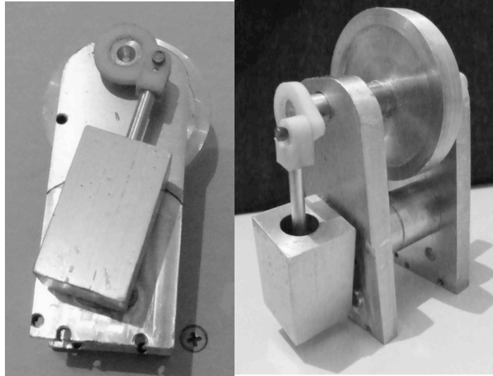
Figura 6.51. Ensamble final
