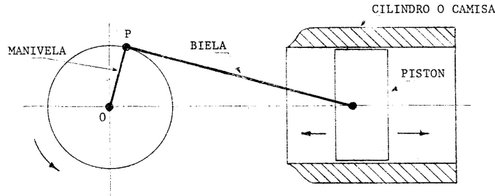
Figura 3.5 Modelo del motor de vapor
