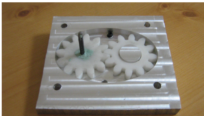
Figura 5.11. Ensamble de los engranes y la armadura
