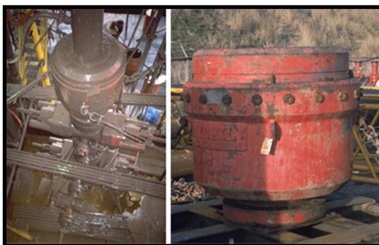
Figura I.2. Preventores Anulares
