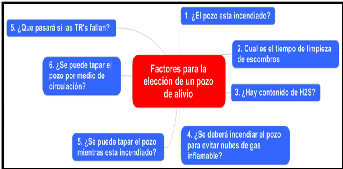
Figura 7.3. Factores para la elección de pozos de alivio (Alcorn, 2005)
