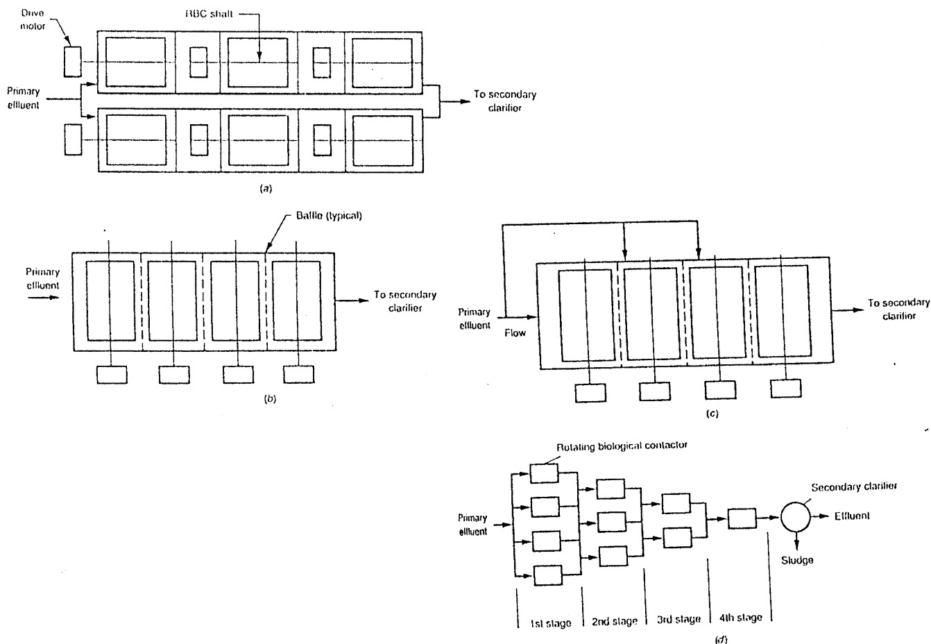
Fig.9.20 Arreglos para diferentes etapas de biodiscos
