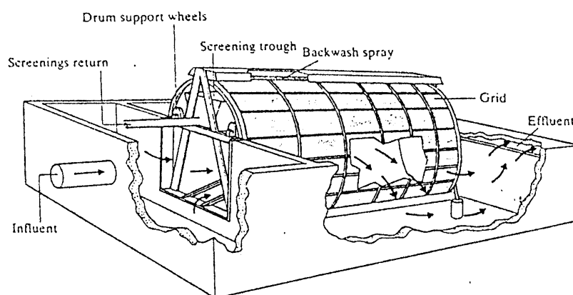
FIGURA 7.8 TAMIZ TIPO TAMBOR.
