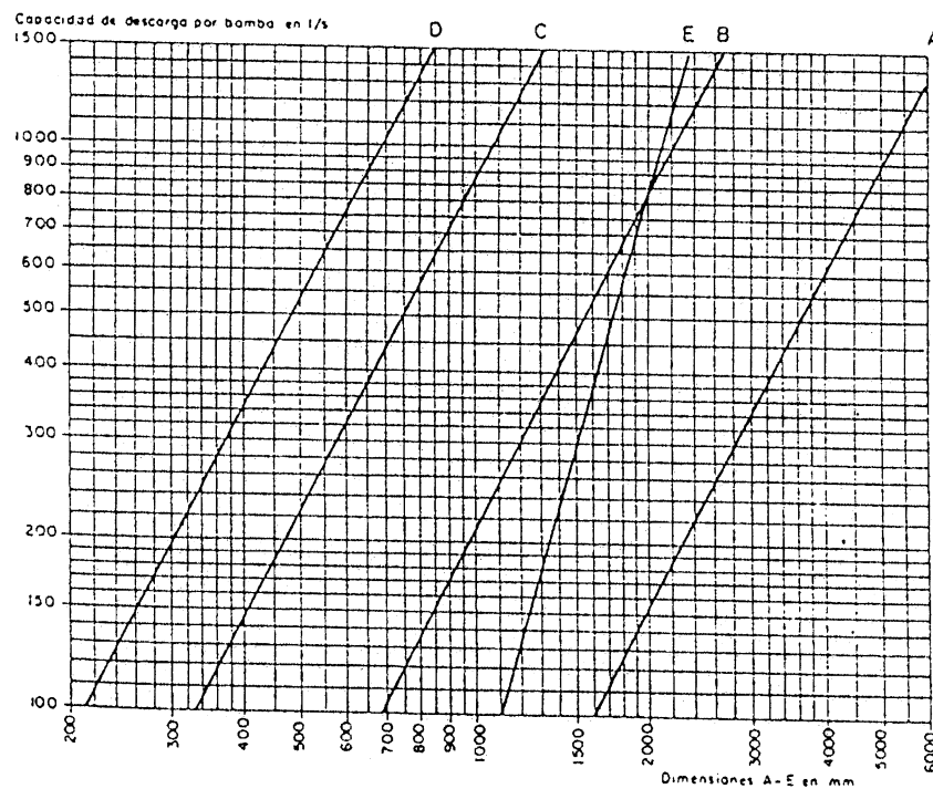
Fig. 5.34 Diagrama para determinar las dimensiones A-E
