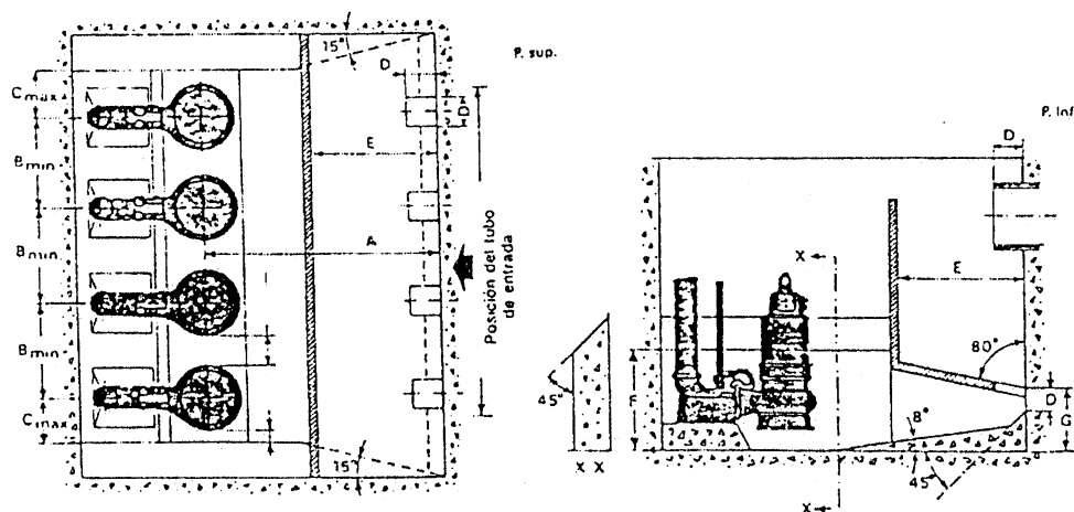
Fig. 5.32 Estación de bombeo en planta y alzado
