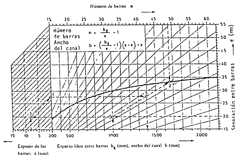
FIGURA 7.7 NOMOGRAMA DE MEDIDAS PARA CONSTRUCCIÓN DE REJAS.
