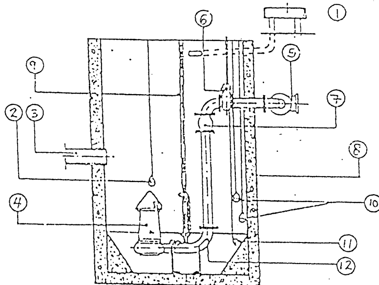
Fig. 5.3 Instalación en cárcamo húmedo con motor fuera del agua.
