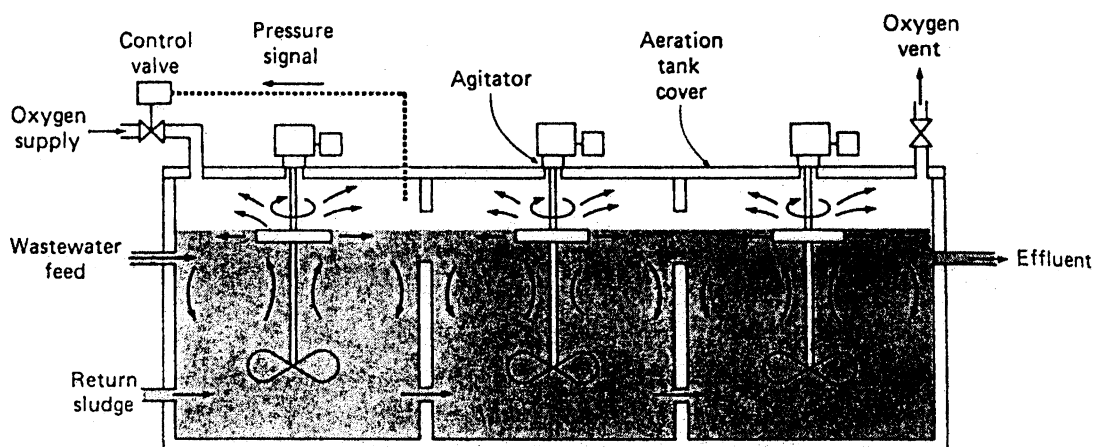
Fig. 9.14 Sistema de multietapas con oxígeno puro
