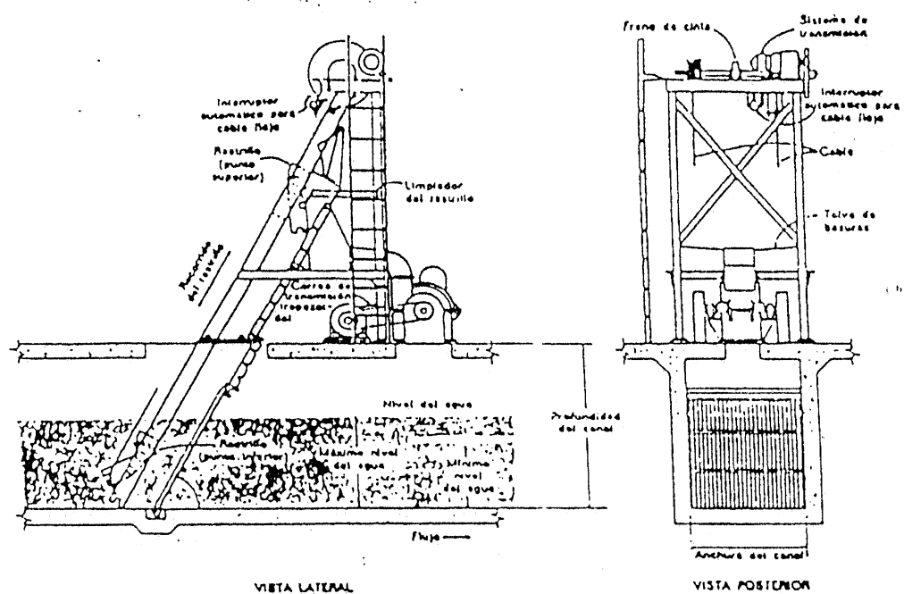
FIGURA 7.2 REJILLA MECÁNICA DE LIMPIEZA FRONTAL
