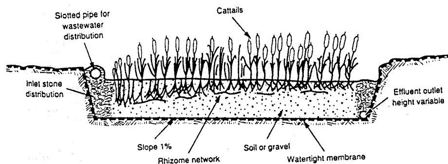
Fig. 11.6 Sección de un sistema de flujo subsuperficial
