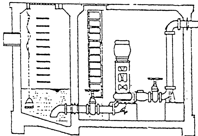
Fig. 5.2 Instalación de bomba de eje vertical en cárcamo seco.
