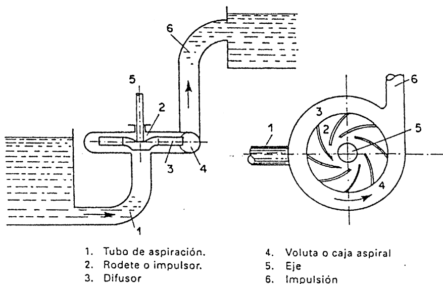
Figura 5.7 Bomba centrífuga
