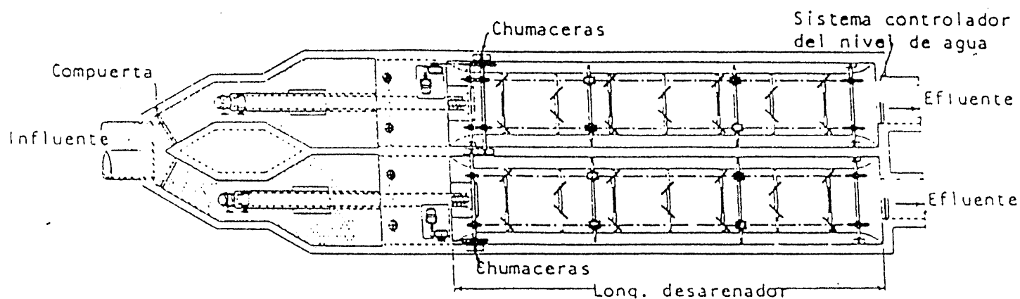
(a) PLANTA
