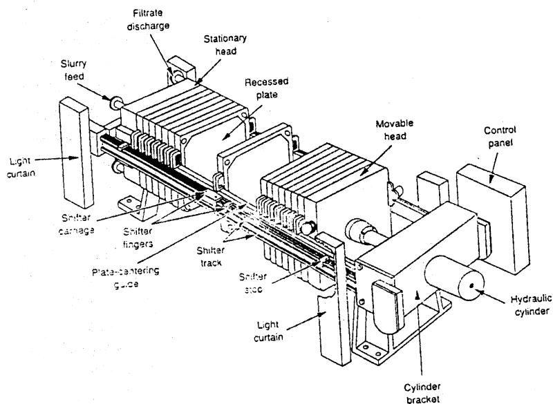
Fig. 12.13 Esquema de un filtro prensa de marco y placas
