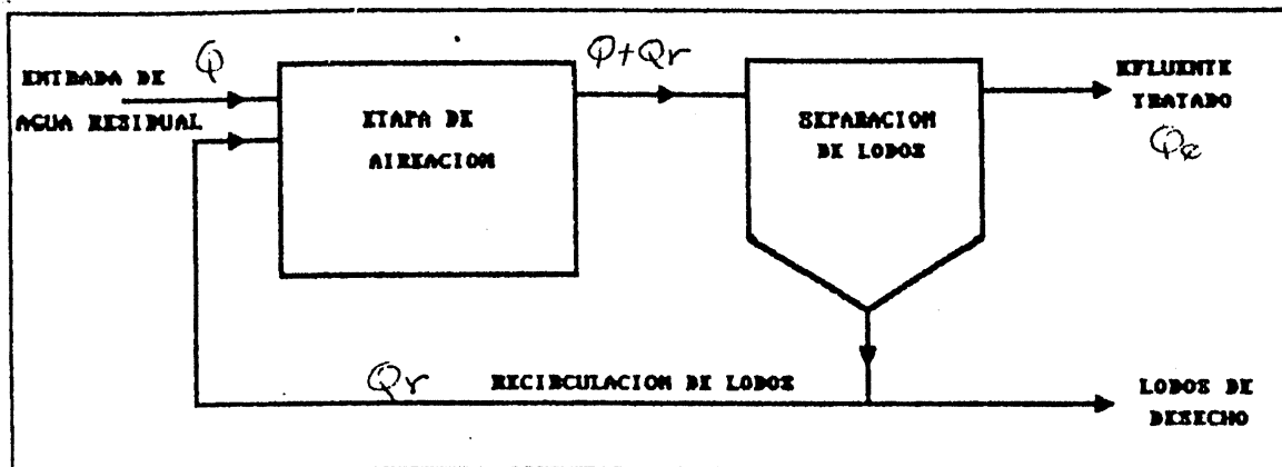
Figura 9.3 Características esenciales de los procesos de lodos activados
