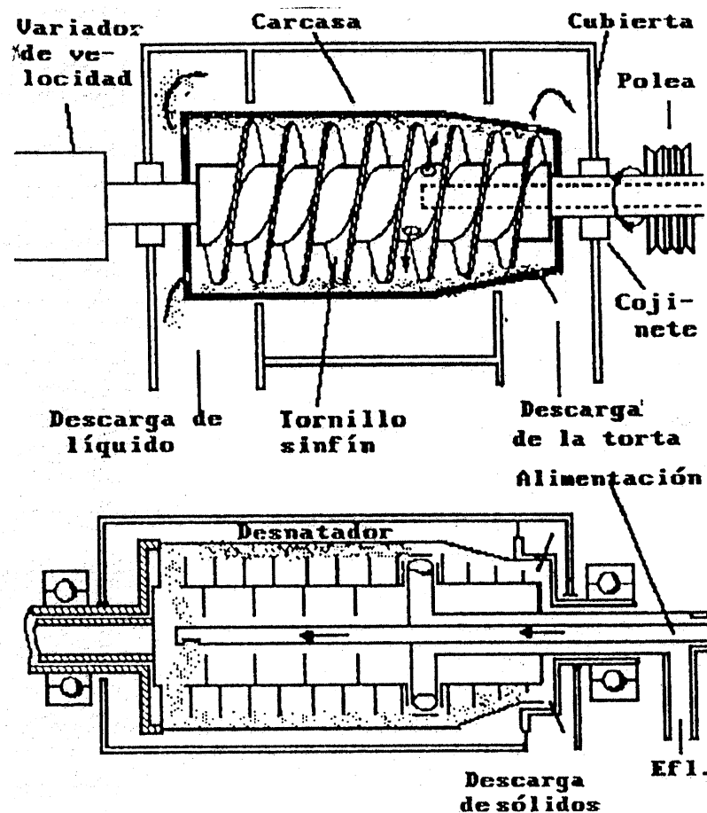
Fig. 12.12 Esquema de centrifuga de tornillo sinfín.
