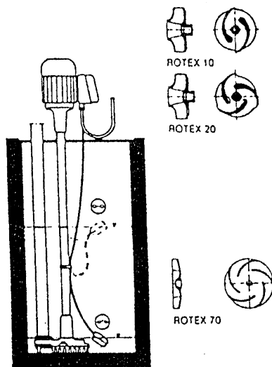
Fig. 5.21 Bombas e instalaciones (ROTEX)
