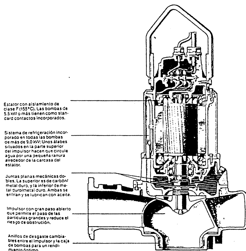
Fig. 5.12 Bomba con impulsor monocanal
