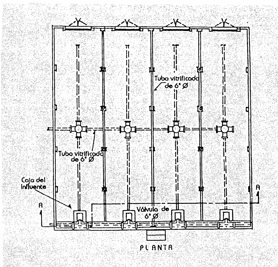
Fig. 12.9 Lecho de secado
