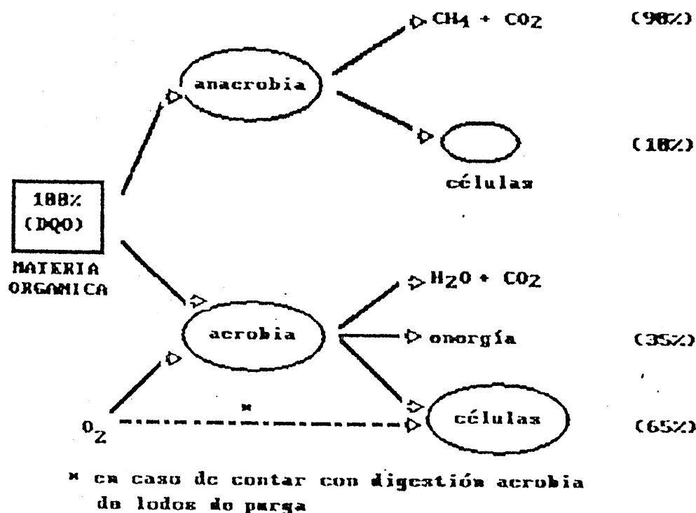
Fig. 9.27 Esquema del flujo de energía de los procesos biológicos de tratamiento de aguas residuales
