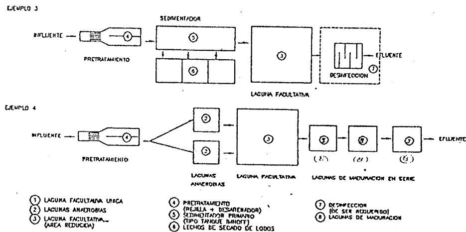
Fig.9.26 Eficiencia de Combinaciones Diversas.
