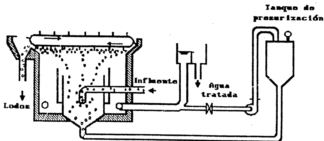
Fig. 12.3 Sistema de flotación para la separación de lodos.
