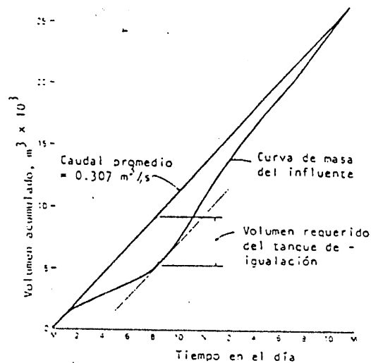
FIGURA 7.26 CURVA DE MASAS PARA LA DETERMINACIÓN DEL VOLUMEN DEL TANQUE DE IGUALACIÓN DEL EJEMPLO.
