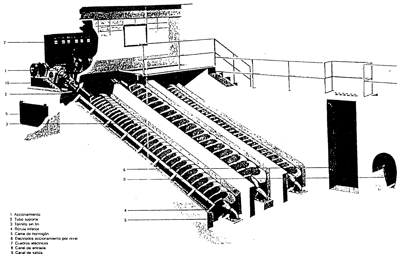
Fig. 5.20 Instalación completa con tornillos de Arquímedes
