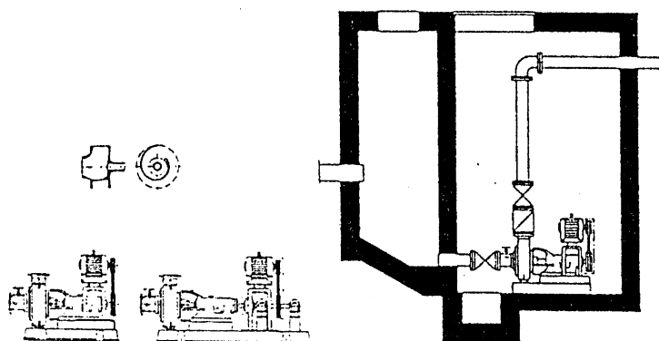
Fig. 5.24 Bombas e instalaciones (KRP) (KVR)
