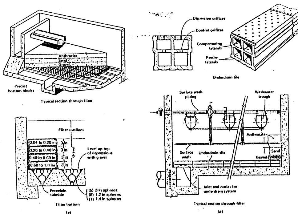
Fig. 10.6 Sistema de subdrenaje típico con capa de grava como soporte (a) y (b); sin soporte de cama de grava (c): (a) sistema de subdrenaje Wheeler y (b) Sistema de subdrenaje Leopold.
