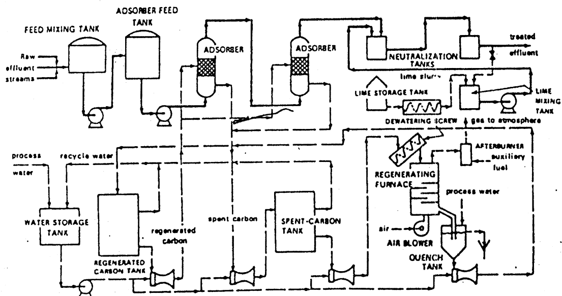
Fig. 10.8 Planta de adsorción y filtración con carbón activado para el tratamiento de residuos de plaguicidas.
