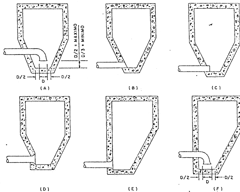
Fig. 5.5 Arreglos típicos para la instalación de la tubería de succión en el foso húmedo de las estaciones de bombas para aguas residuales.
