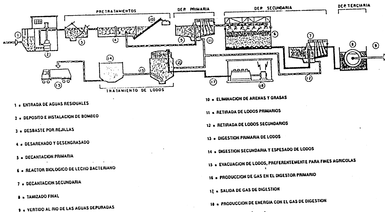
Fig. 6.2 Esquema de una depuradora convencional
