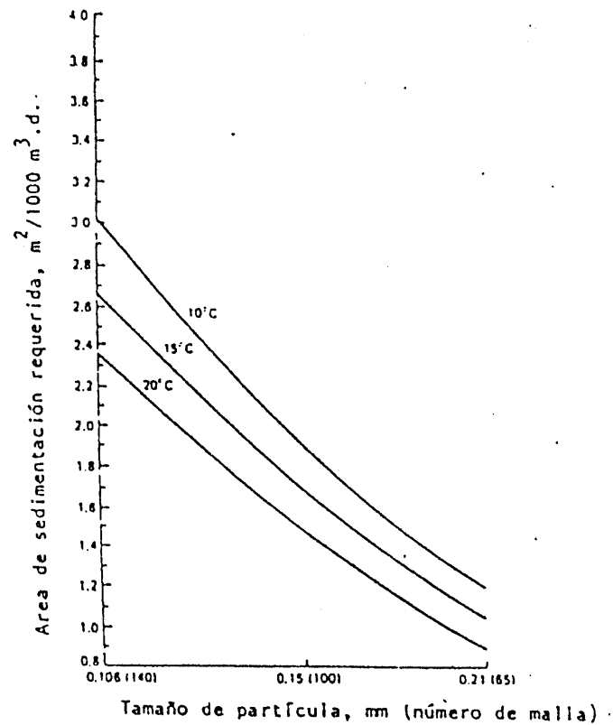
FIGURA 7.17 AREA REQUERIDA POR CADA 1000 M 3 DE AGUAS RESIDUALES PARA LA SEDIMENTACIÓN DE PARTÍCULAS CON GRAVEDAD ESPECIFICA = 2.65 A LAS TEMPERATURAS INDICADAS.
