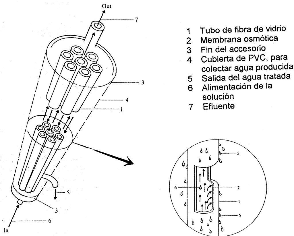
Fig. 10.11 Sistema de ósmosis inversa de configuración tubular
