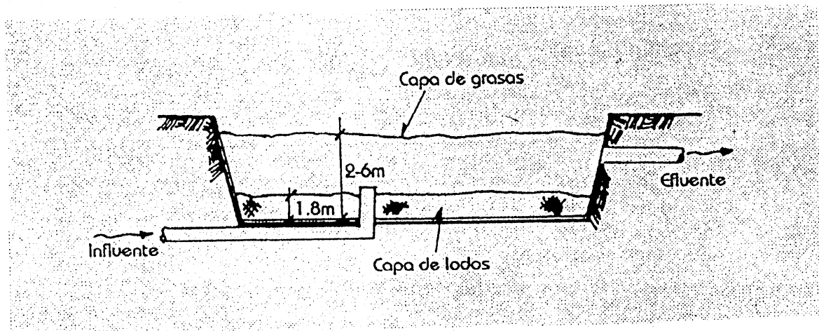
Fig. 9.23 Laguna anaerobia
