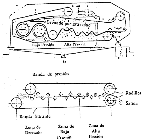
Fig. 12.14 Esquema de un filtro de lodos de banda típico
