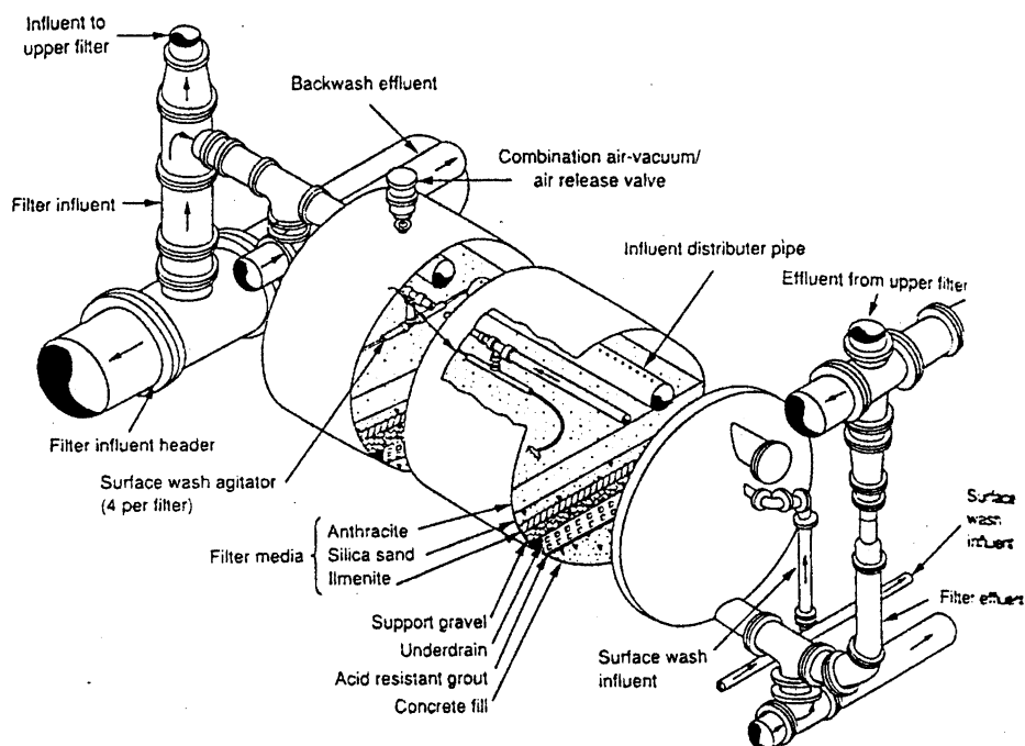
Fig. 10.5 Filtro a presión típico con cama filtrante multimedia y lavado de la superficie usado en el tratamiento de aguas residuales.
