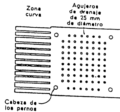
Vista en planta de la plataforma de desagüe
