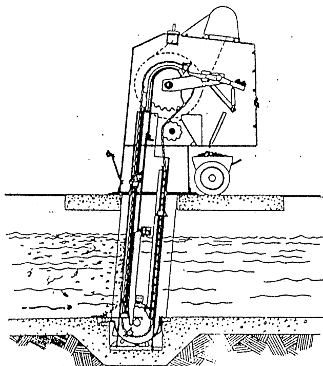
FIGURA 7.3 REJILLA MECÁNICA DE LIMPIEZA POSTERIOR
