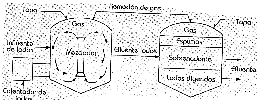
Fig. 12.5 Esquema de un proceso de digestión en dos pasos
