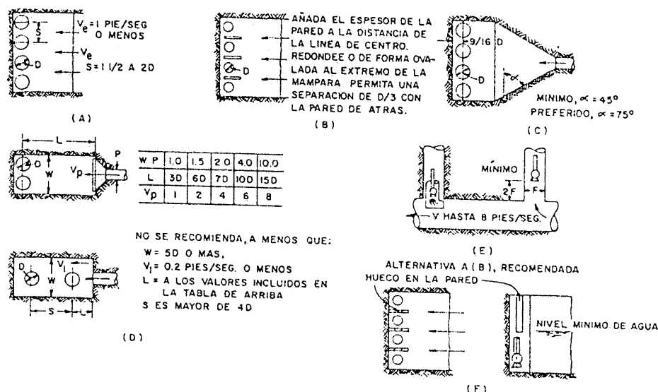
Fig. 5.33 Condiciones recomendadas para el canal de aproximación en instalaciones de bombas múltiples.
