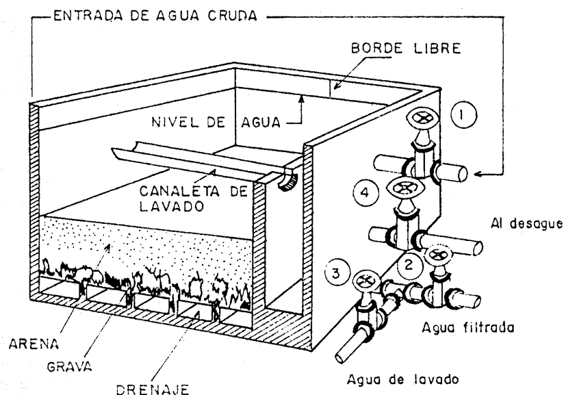
Fig. 10.4 Representación esquemática del funcionamiento de filtros de flujo descendente por gravedad de medio granular
