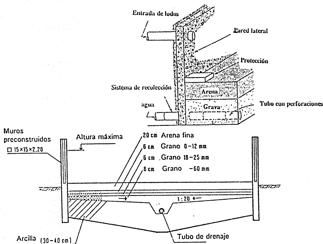
Fig. 12.8 Corte constructivo y granulometría de los lechos de arena
