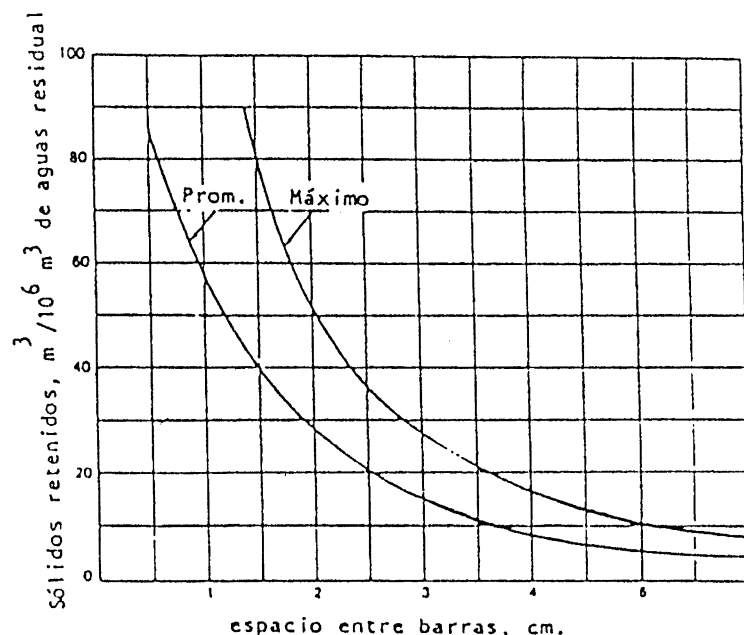
FIGURA 7.6 CANTIDADES DE SÓLIDOS RETENIDOS POR REJILLAS DE LIMPIEZA MECÁNICA
