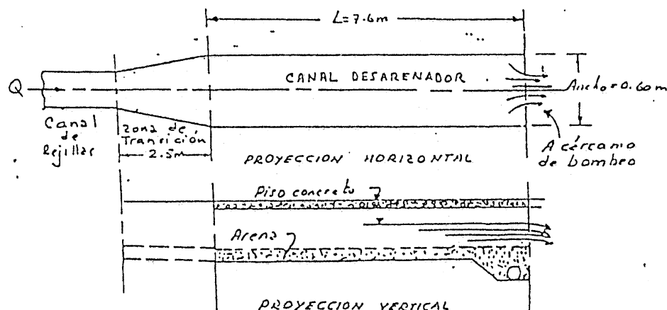
FIGURA 7.16 DESARENADOR DEL EJEMPLO VII.1
