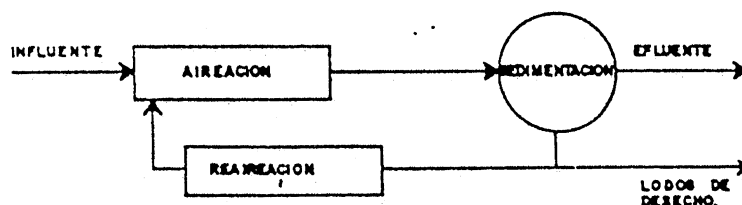
Fig. 9.13 Esquema del proceso de lodos activados con estabilización por contacto.
