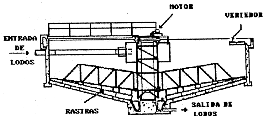
Fig. 12.2 Espesador cilíndrico de lodos (sedimentador).
