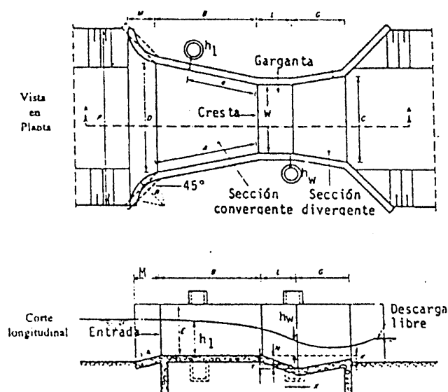
FIGURA 7.19 GEOMETRÍA DE UN CANAL PARSHALL
