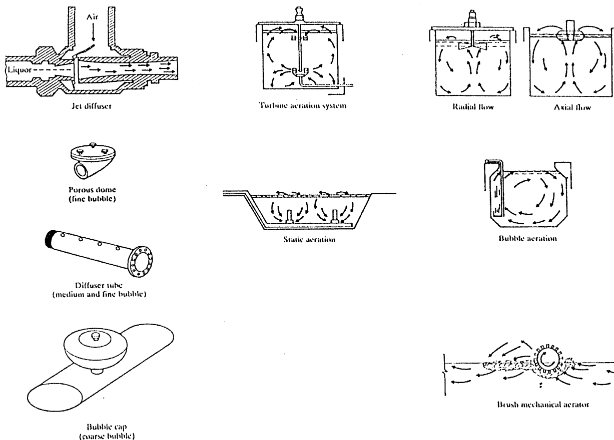
Fig. 9.10 Equipos aereadores
