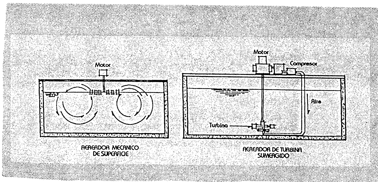
Fig. 9.6 Aireadores mecánicos
