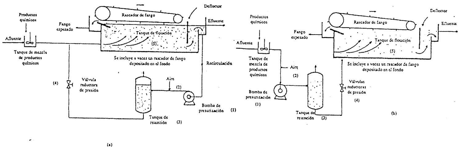
FIGURA 7.22 ESQUEMA DE TANQUES DE FLOTACIÓN CON AIRE(A) CON RECIRCULACIÓN, (B) SIN RECIRCULACIÓN
