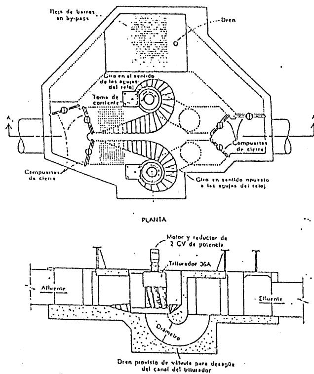
FIGURA 7.10 PLANTA Y SECCIÓN TRANSVERSAL DE UNA INSTALACIÓN DE TRITURACIÓN
