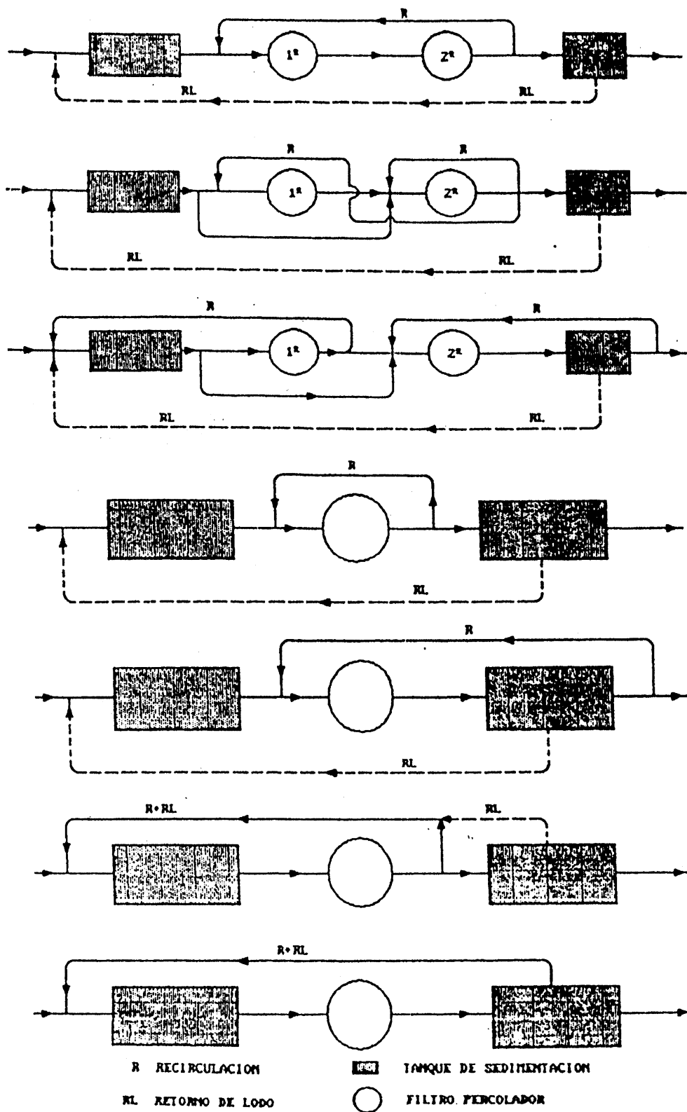
Fig. 9.19 Esquemas de diferentes arreglos de los filtros percoladores
