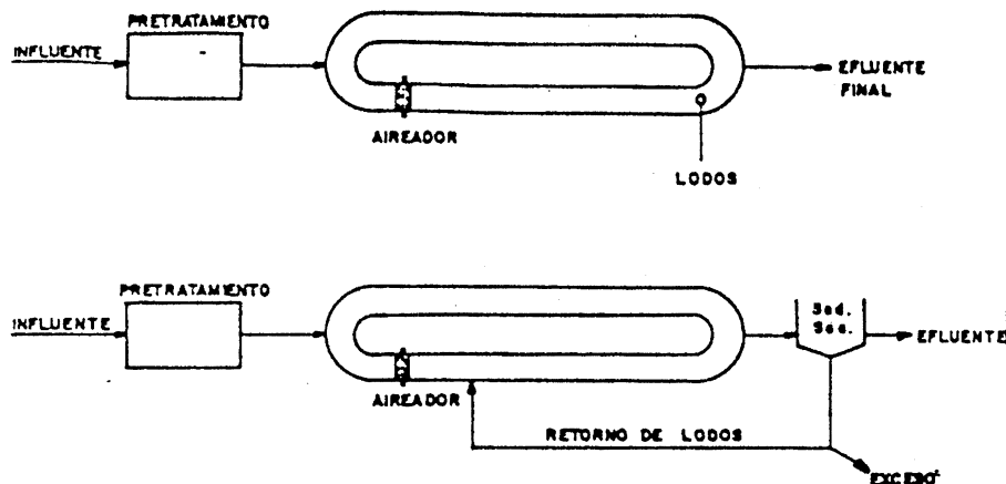
Fig. 9.15 Diagrama esquemático del proceso de zanjas de oxidación
