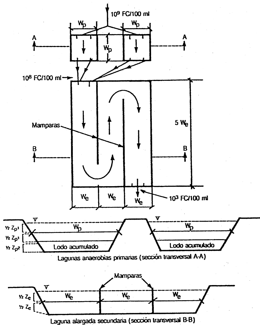
FIGURA 2. Esquema para el diseño de lagunas anaerobias primarias y lagunas alargadas secundarias en terrenos planos o ligeramente inclinados
