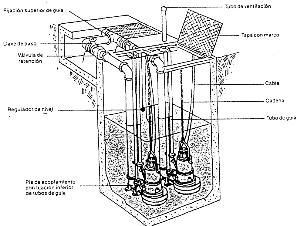
Fig. 5.13 Instalación de bombas con impulsosres monocanal tipo Flygt
