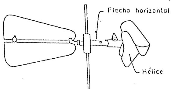
MEDIDOR DE CORRIENTE DE HELICE
