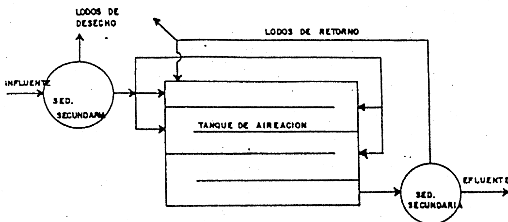
Fig. 9.12 Esquema del proceso de lodos activados con aireación por etapas.
