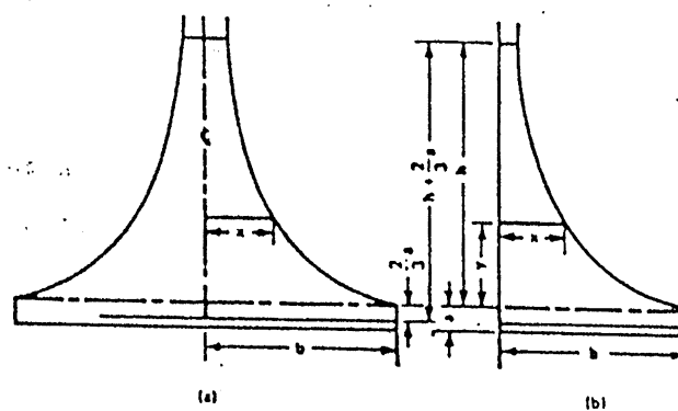
FIGURA 7.18 ELEMENTOS DE UN VERTEDOR PROPORCIONAL (A) Y DE UN VERTEDOR TIPO SUTRO (B)
