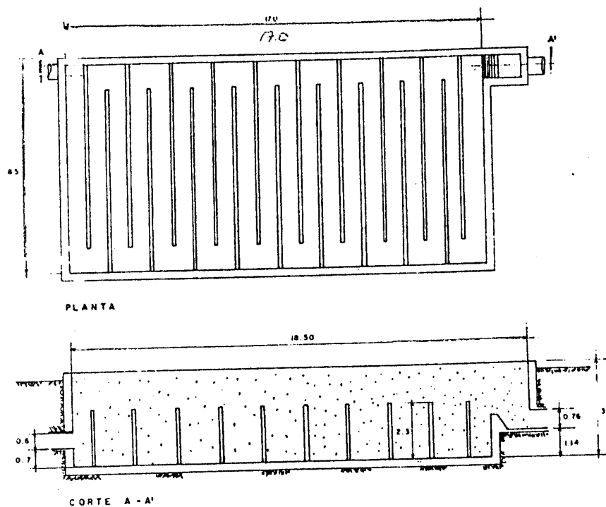
Fig. 10.2 Depósito longitudinal dividido con baffles con capacidad efectiva con relación largo-ancho mayor de 40-1 que suministra una distribución de cámara de contacto con tiempos de residencia aproximado al tipo flujo pistón.
