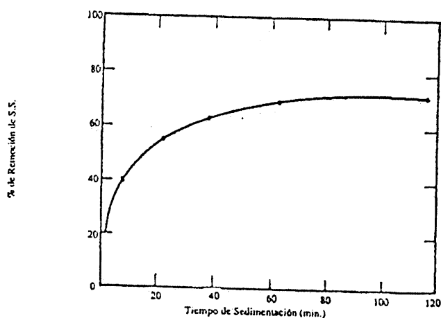
Fig. 8.12 Relación carga superficial-remoción sólidos
