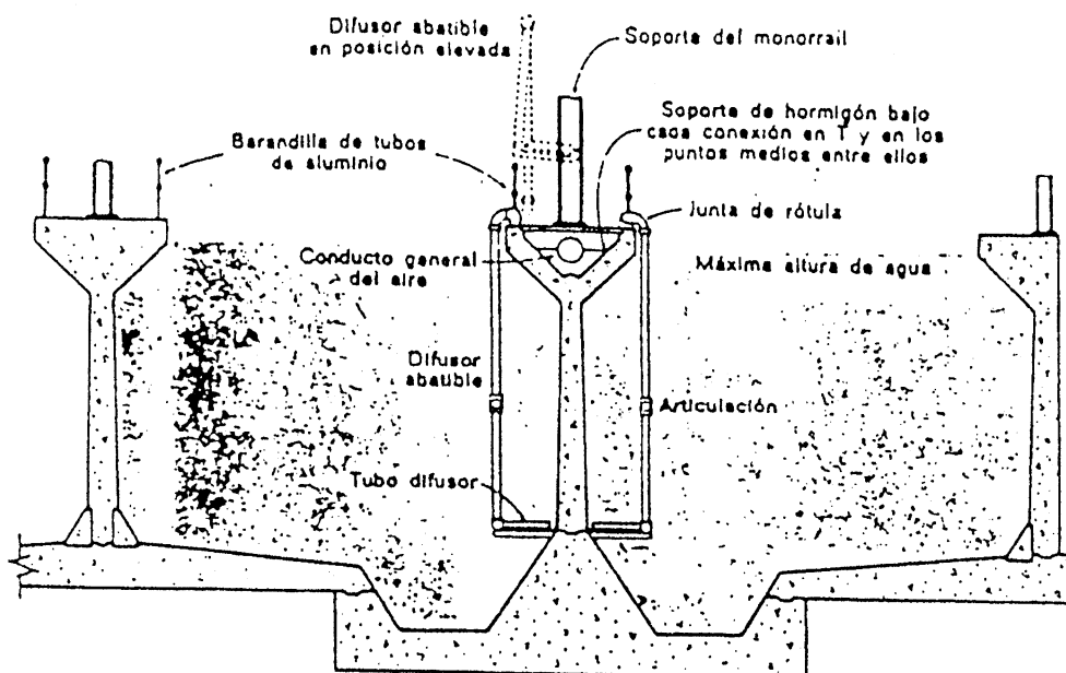
FIGURA 7.12 SECCIÓN TRANSVERSAL TÍPICA DE UN DESARENADOR AEREADO
