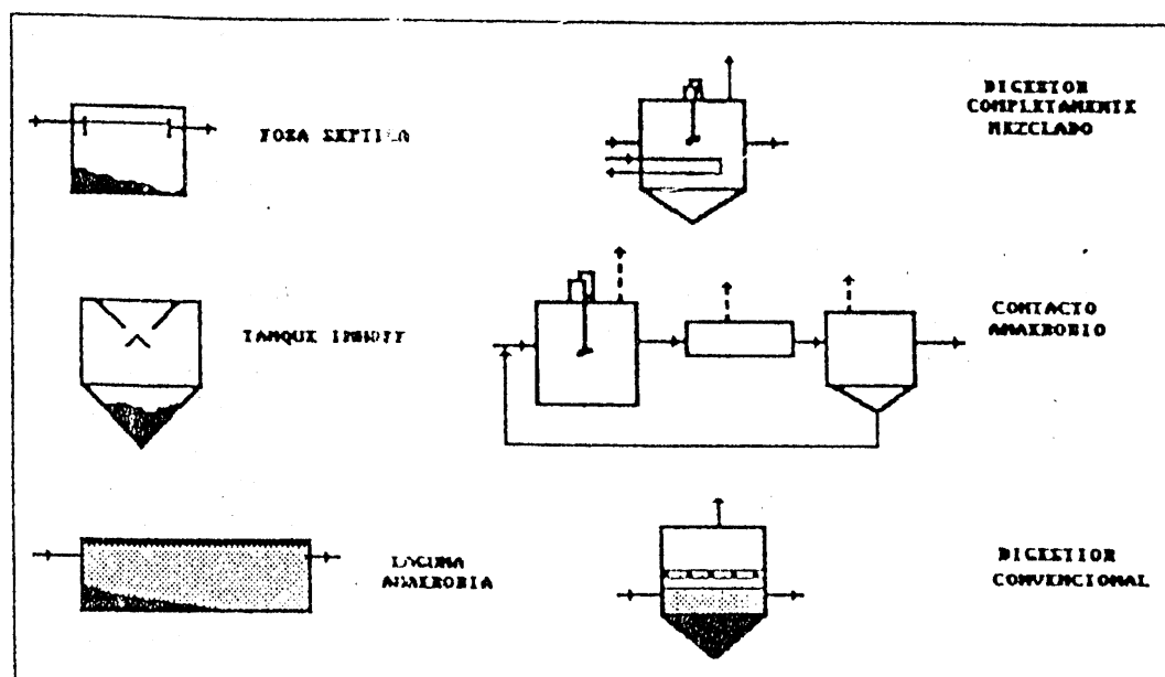
Fig. 9.28 Reactores anaerobios de la 1ª generación
