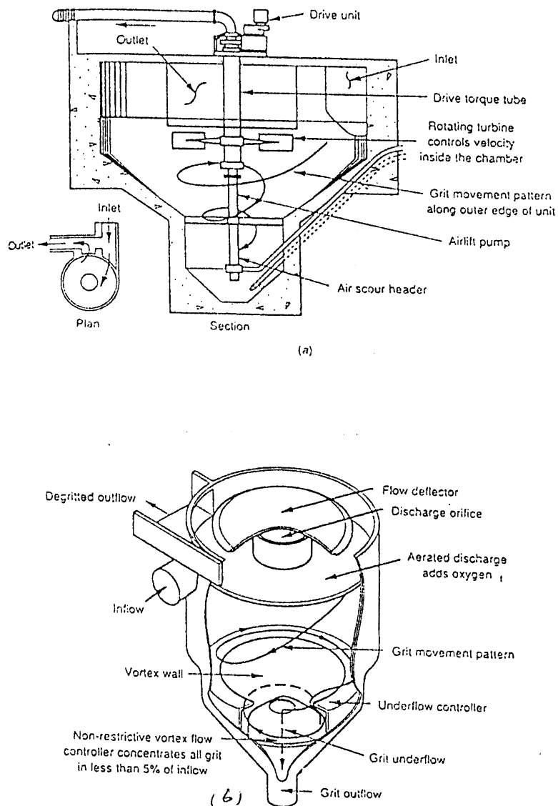
FIGURA 7.15 DOS EJEMPLOS DE DESARENADORES TIPO VORTICE
