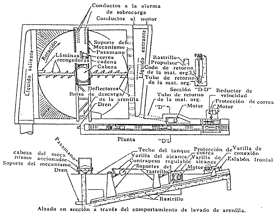
FIGURA 7.14 DESARENADOR DE SECCIÓN CUADRADA O TANQUE DE DETRITUS
