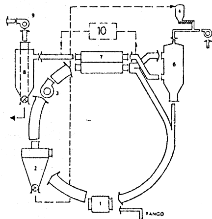
Diagrama del sistema de incineración (Tipo VON ROLL)
