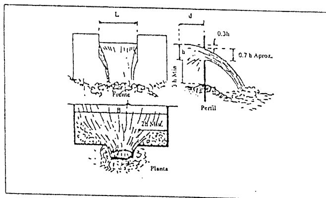
Fig. 4.6 Vertedor rectangular
