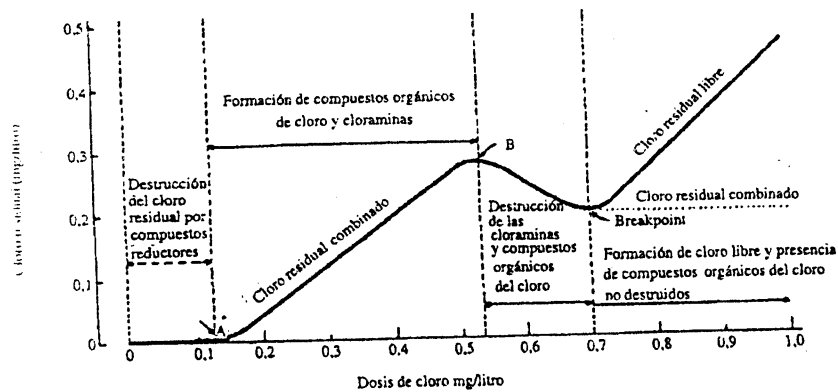
Fig. 10.1 Curva que generalmente se obtiene durante la cloración al punto de quiebre
