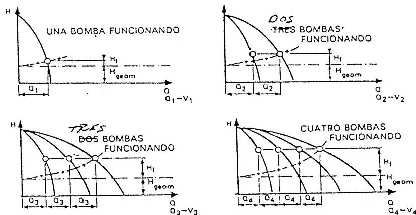
Fig. 5.36 Curvas de sistema esquemáticas
