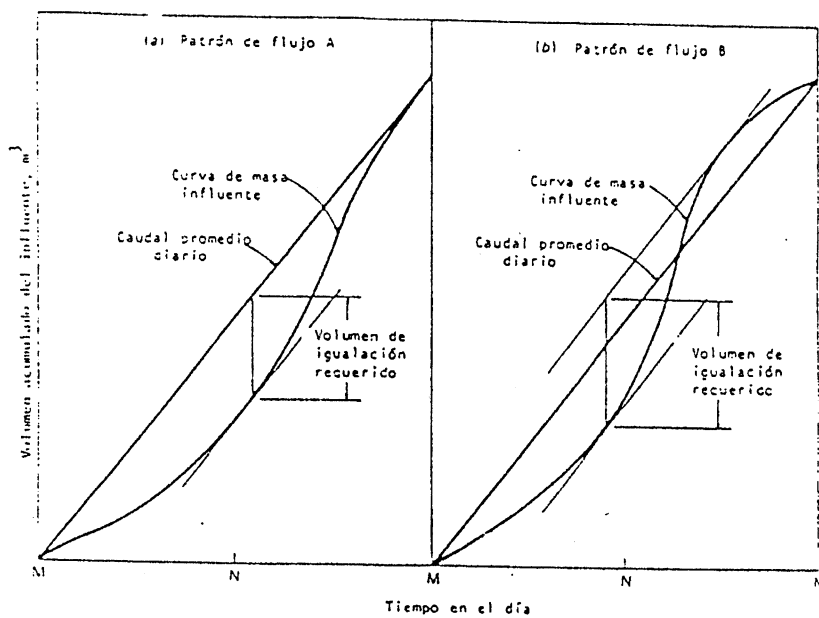
FIG. 7.25 CURVAS DE MASAS PARA LA DETERMINACIÓN DEL VOLUMEN DE IGUALACIÓN REQUERIDO PARA DOS PATRONES TÍPICOS DE FLUJO.
