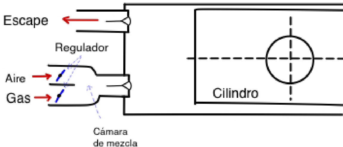
Figura 3.6. Configuración de regulación 4 (González, 2003).
