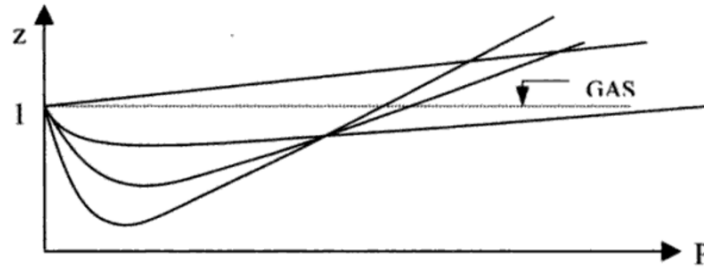
Figura 2.1. Factor de compresibilidad del N_2 para valores de P y T (Movilla Rosell, Movilla, & Rajadell Viciano, 2005)
