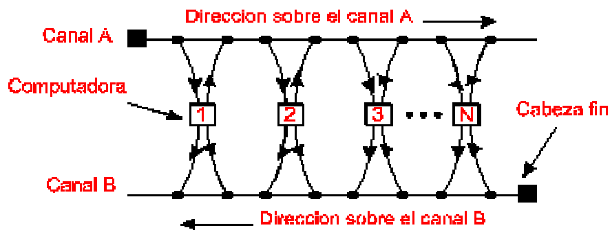
Figura 2.7.1.2 .1 DQDB
